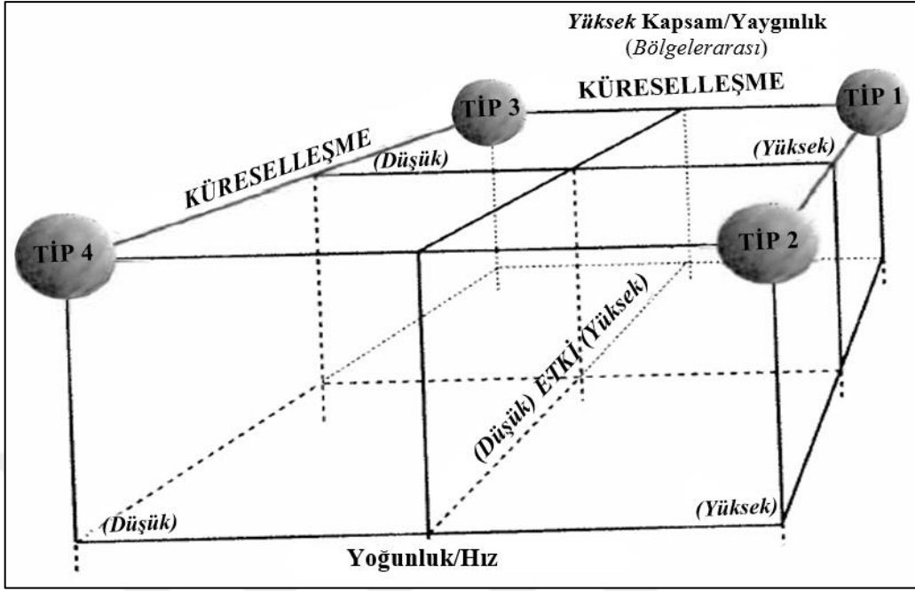
Şekil 4:Küreselleşmenin Tipolojisi
