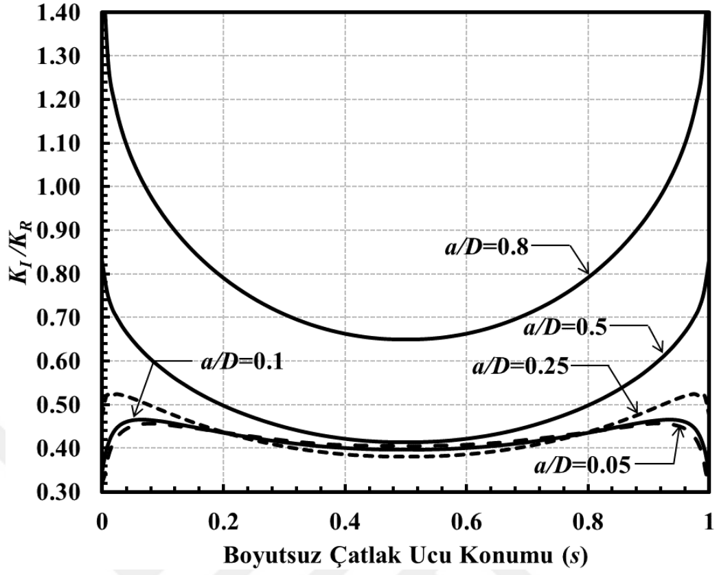
Şekil 3.268. Sabit a/c için çatlak önü boyunca boyutsuz K_I dağılımları (Eğilme gerilmesi) ( \alpha = 45^\circ , a/c=1 ).
