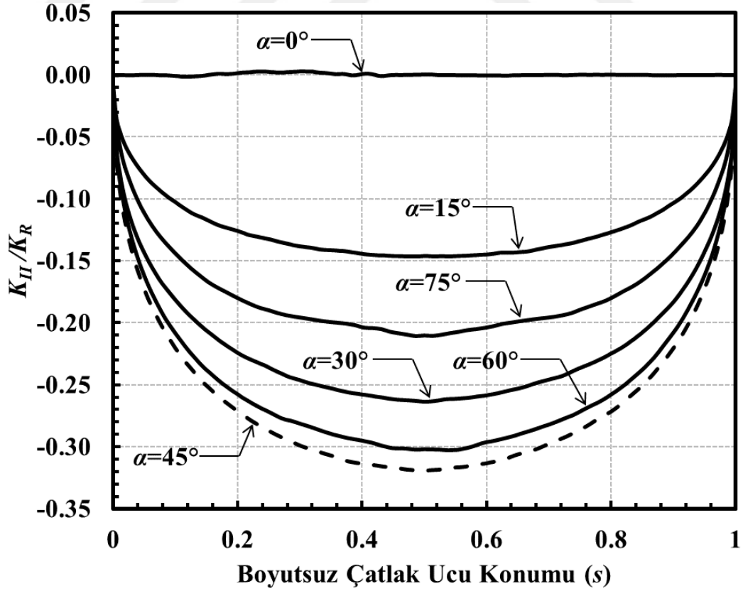
Şekil 3.103. a/c=0.25 , a/D=0.05 için çatlak önü boyunca boyutsuz K_{II} dağılımları (Eğilme gerilmesi).
