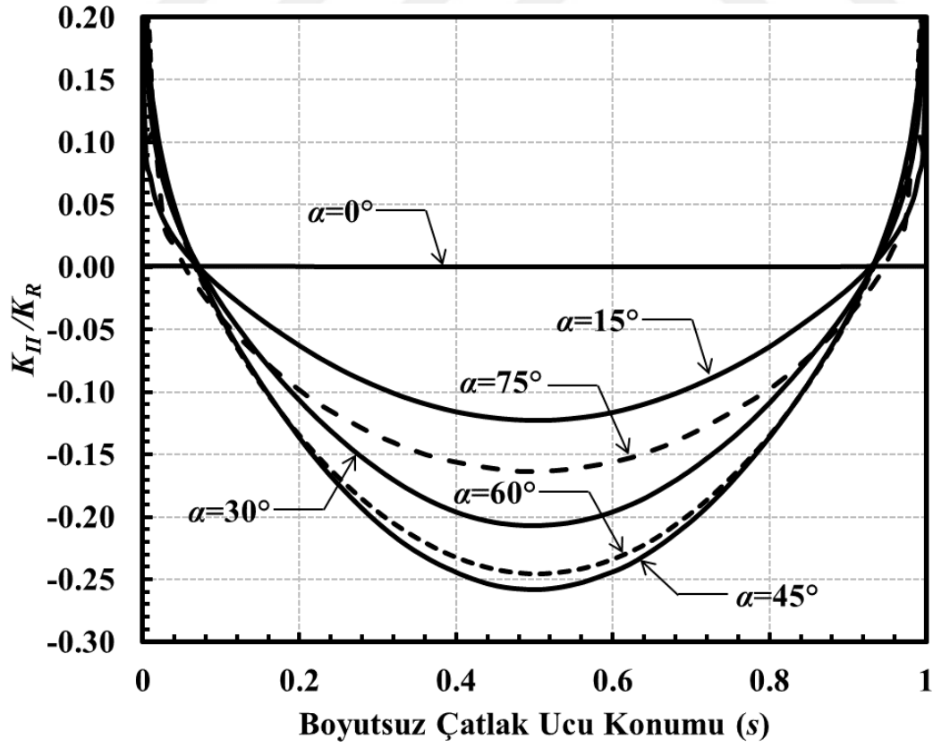
Şekil 3.133. a/c=1 , a/D=0.05 için çatlak önü boyunca boyutsuz K_{II} dağılımları (Eğilme gerilmesi).
