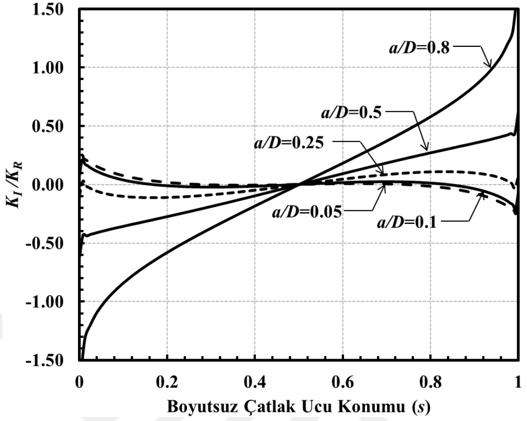
Şekil 3.280. Sabit a/c için çatlak önü boyunca boyutsuz K_I dağılımları (Burulma yükü) ( \alpha = 45^\circ , a/c = 1 ).
