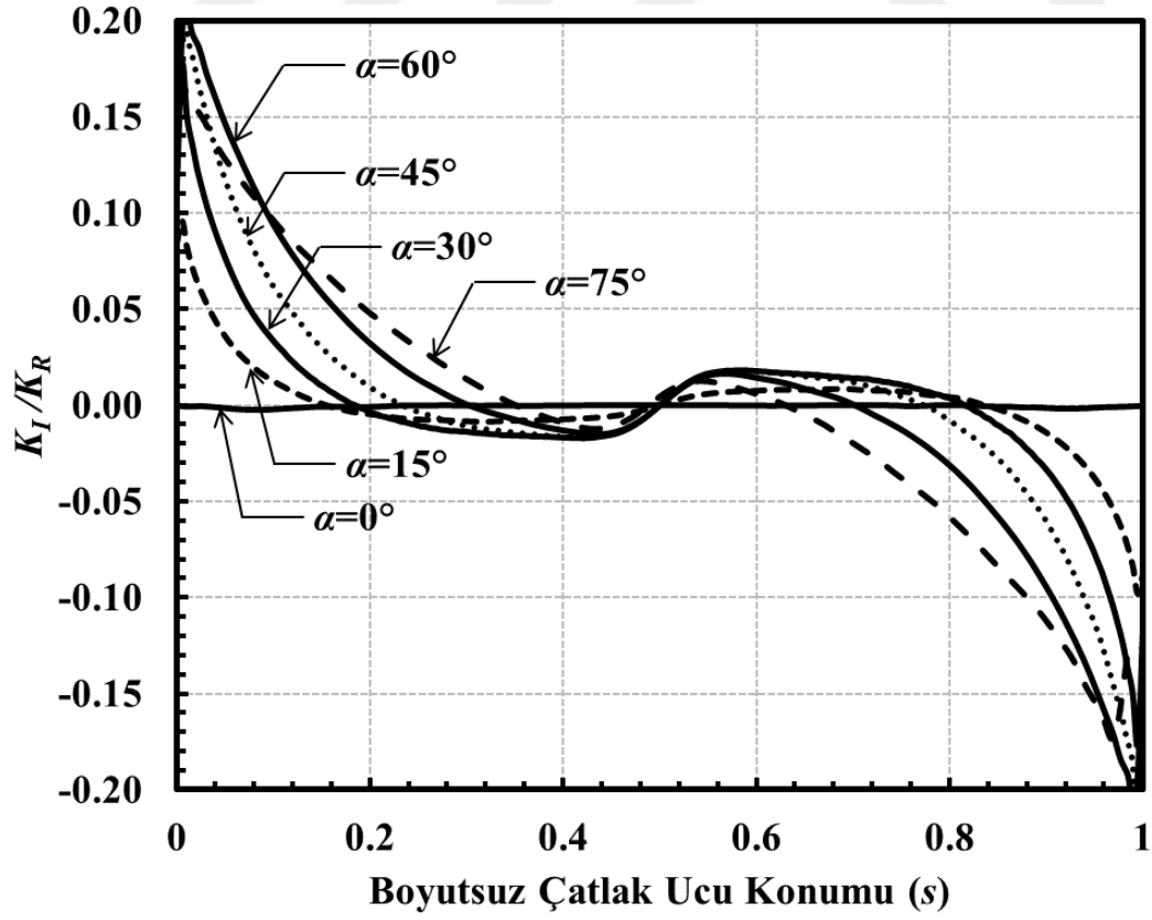
Şekil 3.230. a/c=2 , a/D=0.1 için çatlak önü boyunca boyutsuz K_I dağılımları (Burulma yükü).
