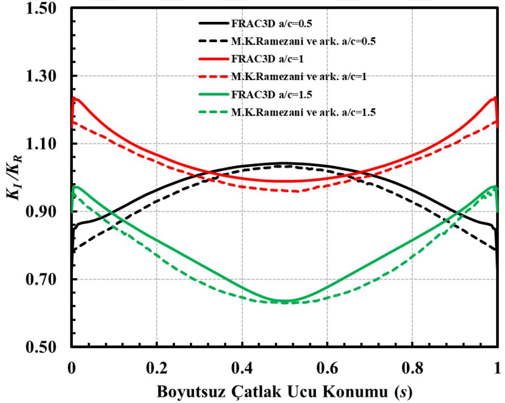
Şekil 3.23. a/D=0.05 , \beta=45^\circ değişik çatlak şekil oranları için boyutsuz K_I sonuçlarının kıyaslanması (Burulma yükü, [17]).
