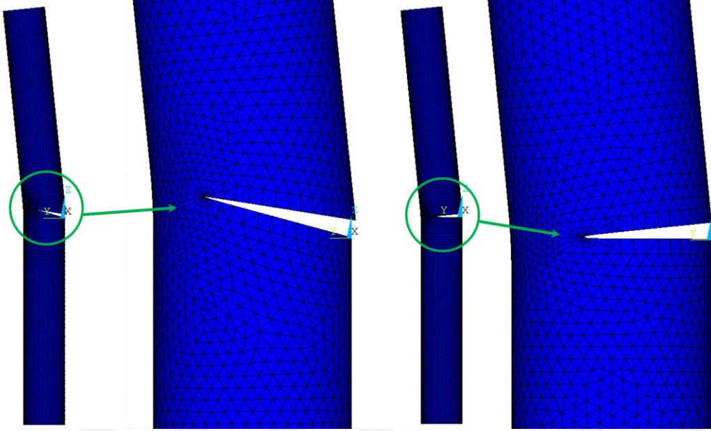
Şekil 4.1. a/c=0.5 , \alpha=15^\circ (solda), a/c=1 , \alpha=0^\circ (sağda) için eksenel gerilme yükü altında meydana gelen yapısal deformasyonlar [25].
