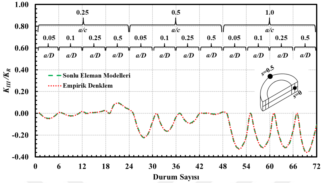
Şekil 4.11. Eksenel gerilme yükü altında silindirde bulunan a/c=0.25-1.0 şekil oranlarına sahip dönmüş yüzey çatlığının serbest yüzey noktası için ( s=0 ) boyutsuz K_{III} değerleri ile empirik denklem sonucunun karşılaştırılması.
