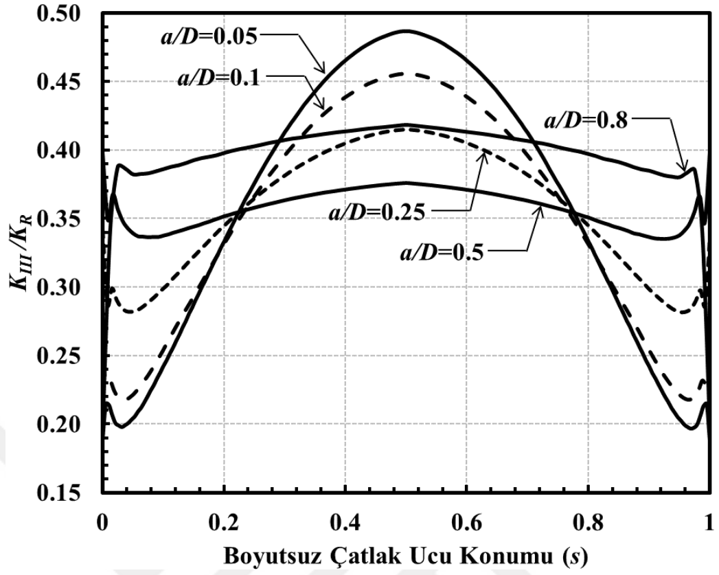
Şekil 3.288. Sabit a/c için çatlak önü boyunca boyutsuz K_{III} dağılımları (Burulma yükü) ( \alpha=45^\circ , a/c=1 ).
