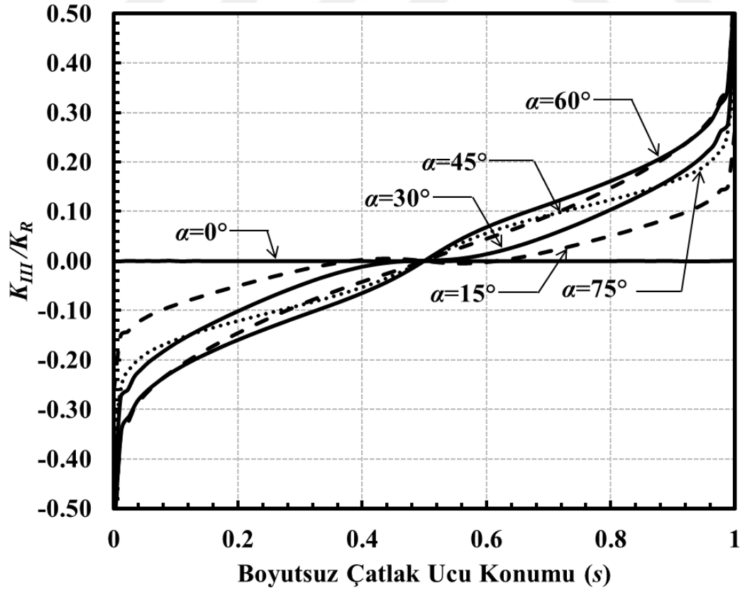
Şekil 3.161. a/c=2 , a/D=0.8 için çatlak önü boyunca boyutsuz K_{III} dağılımları (Eğilme gerilmesi).
