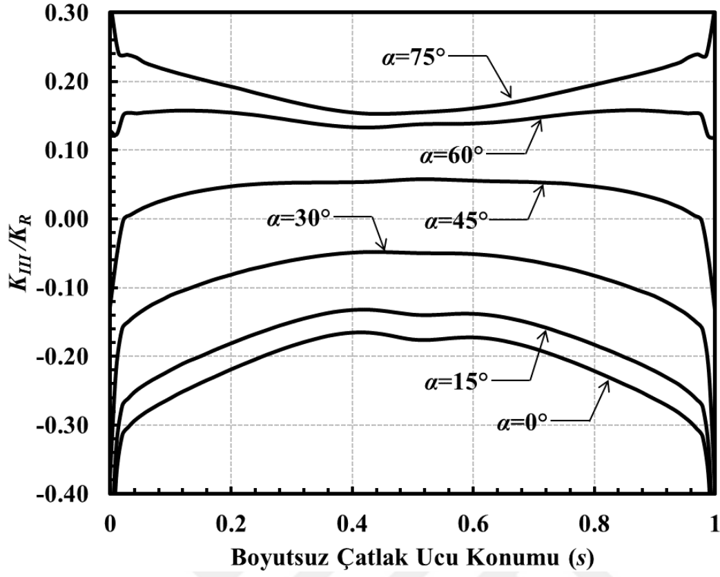
Şekil 3.241. a/c=2 , a/D=0.8 için çatlak önü boyunca boyutsuz K_{III} dağılımları (Burulma yükü).
