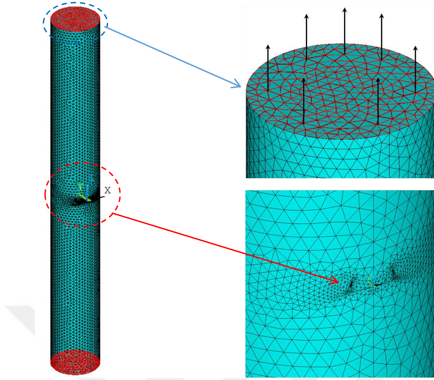
Şekil 3.26. a/c=1 , a/D=0.1 , \alpha =75^\circ olan dönmüş yüzey çatlağına sahip bir katı silindirin global sonlu elemanlar modeli, eksenel gerilme yüklemesi ve çatlak bölgesinin yakından görünümü.
