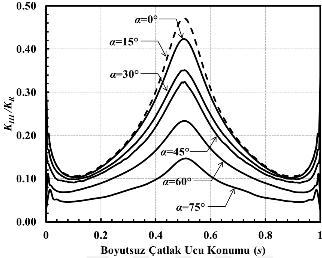
Şekil 3.253. a/c=2 , a/D=0.05 ve H/D=6 için çatlak önü boyunca boyutsuz K_{III} dağılımları (Burulma yükü).
