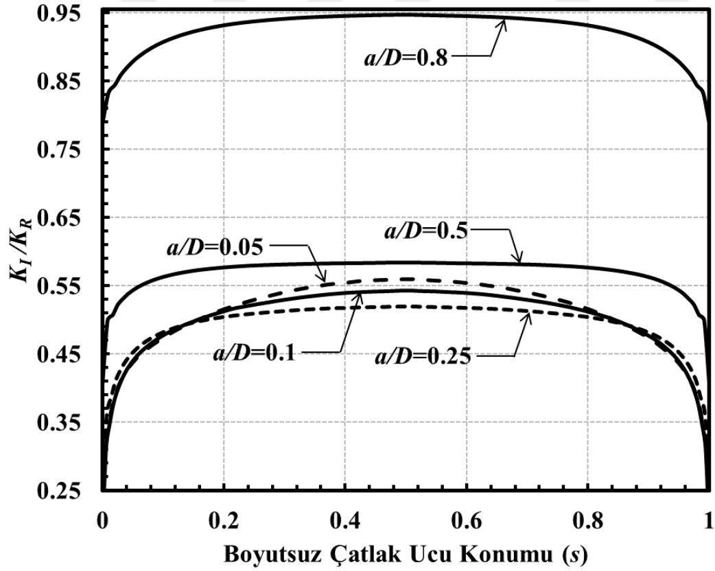
Şekil 3.267. Sabit a/c için çatlak önü boyunca boyutsuz K_I dağılımları (Eğilme gerilmesi) ( \alpha=45^\circ , a/c=0.5 ).
