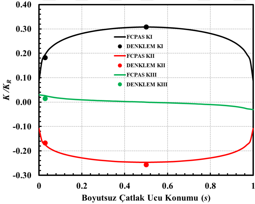
Şekil 4.27. a/c=0.3 , a/D=0.4 , \alpha=70^\circ için boyutsuz K dağılımları ile empirik denklem sonuçları (Eksenel gerilme).
