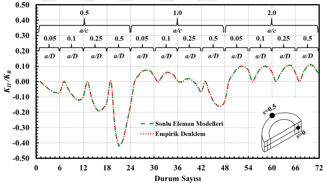
Şekil 4.10. Eksenel gerilme yükü altında silindirde bulunan a/c=0.5-2.0 şekil oranlarına sahip dönmüş yüzey çatlığının serbest yüzey noktası için ( s=0 ) boyutsuz K_{II} değerleri ile empirik denklem sonucunun karşılaştırılması.
