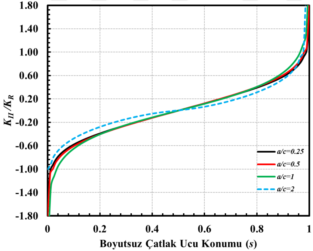
Şekil 3.329. Sabit a/D için çatlak önü boyunca boyutsuz K_{II} dağılımları (Burulma yükü) ( \alpha=45^\circ , a/D=0.8 ).
