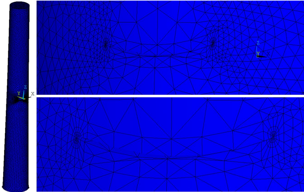
Şekil 3.180. a/c=2 , a/D=0.25 , \alpha =60 derece dönmüş çatlğa sahip katı silindire uygulanan burulma yükü sonucu oluşan deformasyon ve çatlak bölgesinin yakından görünümü.
