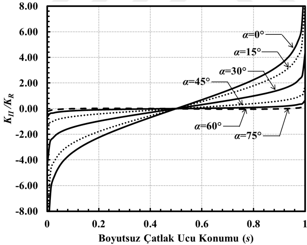
Şekil 3.210. a/c=0.5 , a/D=0.8 için çatlak önü boyunca boyutsuz K_{II} dağılımları (Burulma yükü).
