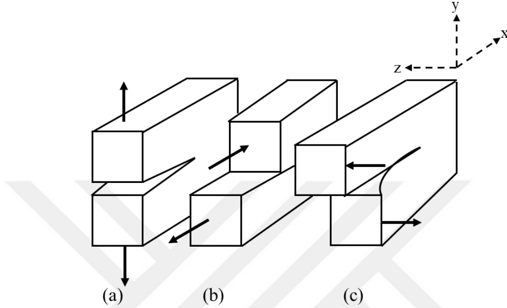
Şekil 1.1. Çatlak deformasyon modları, (a) açılma, (b) düzlem içi kayma ve (c) yırtılma modu.
