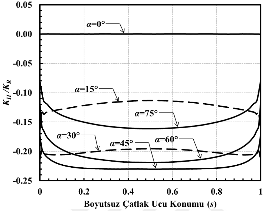
Şekil 3.112. a/c=0.25 , a/D=0.5 için çatlak önü boyunca boyutsuz K_{II} dağılımları (Eğilme gerilmesi).
