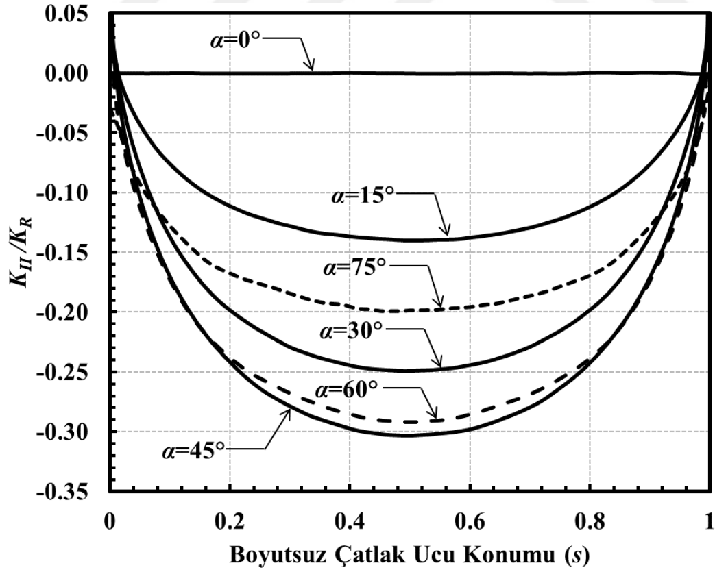
Şekil 3.165. a/c=0.5 , a/D=0.05 ve H/D=6 için çatlak önü boyunca boyutsuz K_{II} dağılımları (Eğilme gerilmesi).
