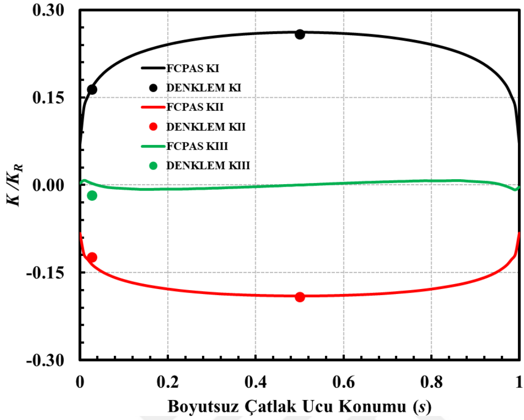
Şekil 4.50. a/c=0.45 , a/D=0.36 , \alpha=70^\circ için boyutsuz K dağılımları ile empirik denklem sonuçları (Eğilme gerilmesi).
