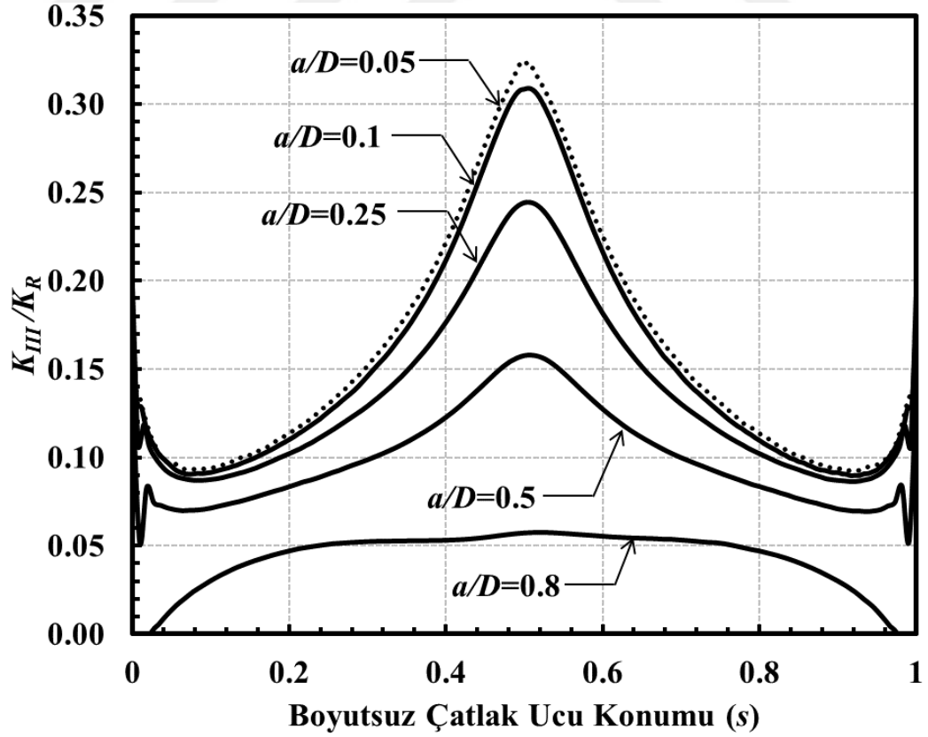
Şekil 3.289. Sabit a/c için çatlak önü boyunca boyutsuz K_{III} dağılımları (Burulma yükü) ( \alpha=45^\circ , a/c=2 ).
