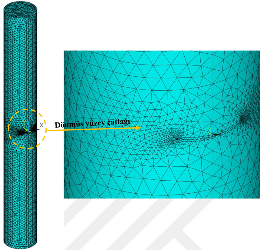
Şekil 3.6. Dönmüş yüzey çatlğına sahip katı bir silindirin bölüntülenmiş modeli ve çatlak bölgesinin yakından görünümü.
