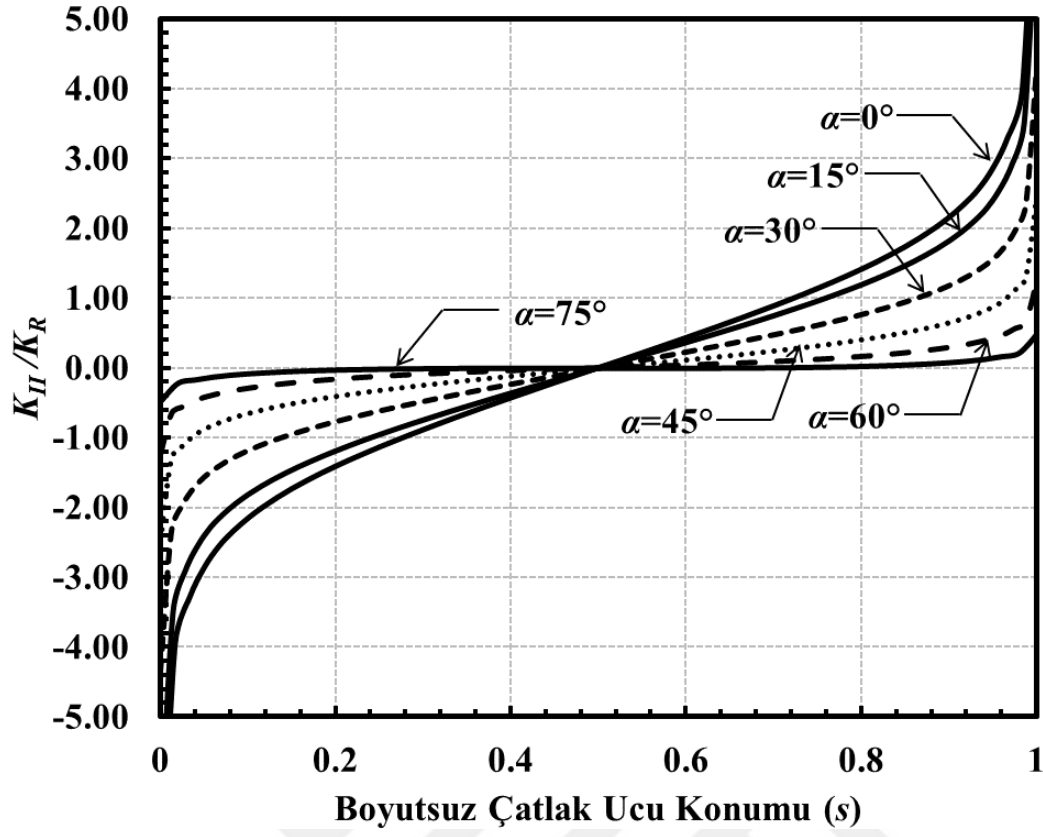
Şekil 3.225. a/c=1 , a/D=0.8 için çatlak önü boyunca boyutsuz K_{II} dağılımları (Burulma yükü).
