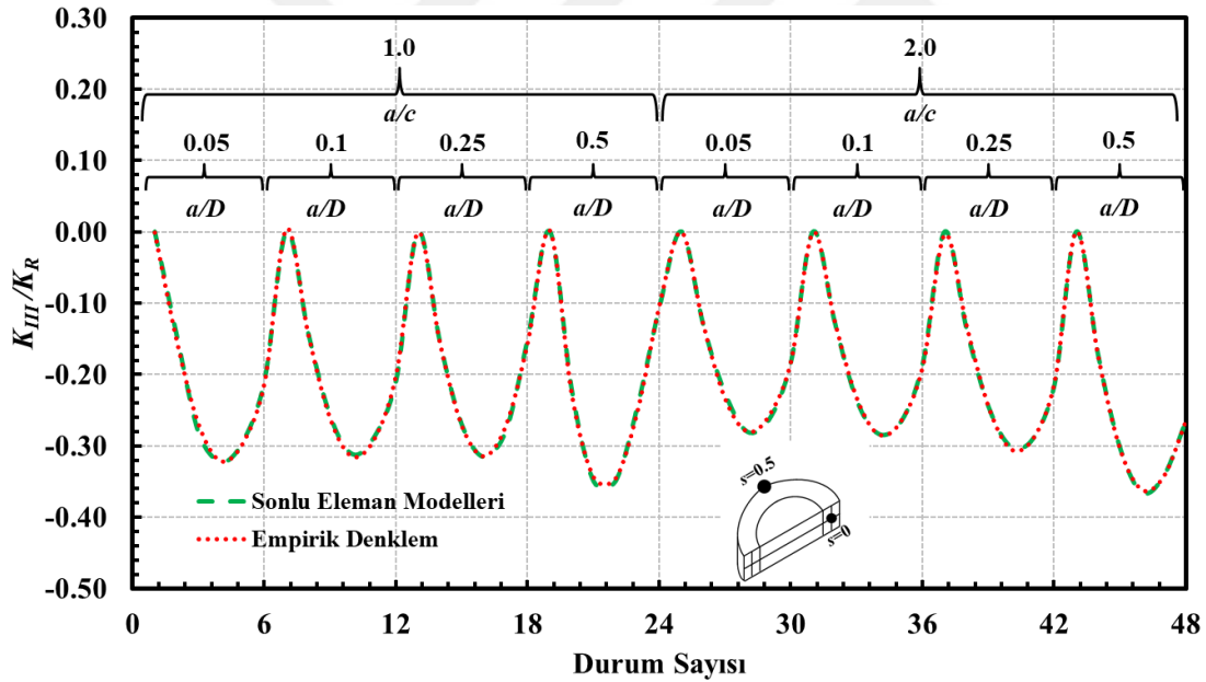
Şekil 4.12. Eksenel gerilme yükü altında silindirde bulunan a/c=1.0-2.0 şekil oranlarına sahip dönmüş yüzey çatlığının serbest yüzey noktası için ( s=0 ) boyutsuz K_{III} değerleri ile empirik denklem sonucunun karşılaştırılması.
