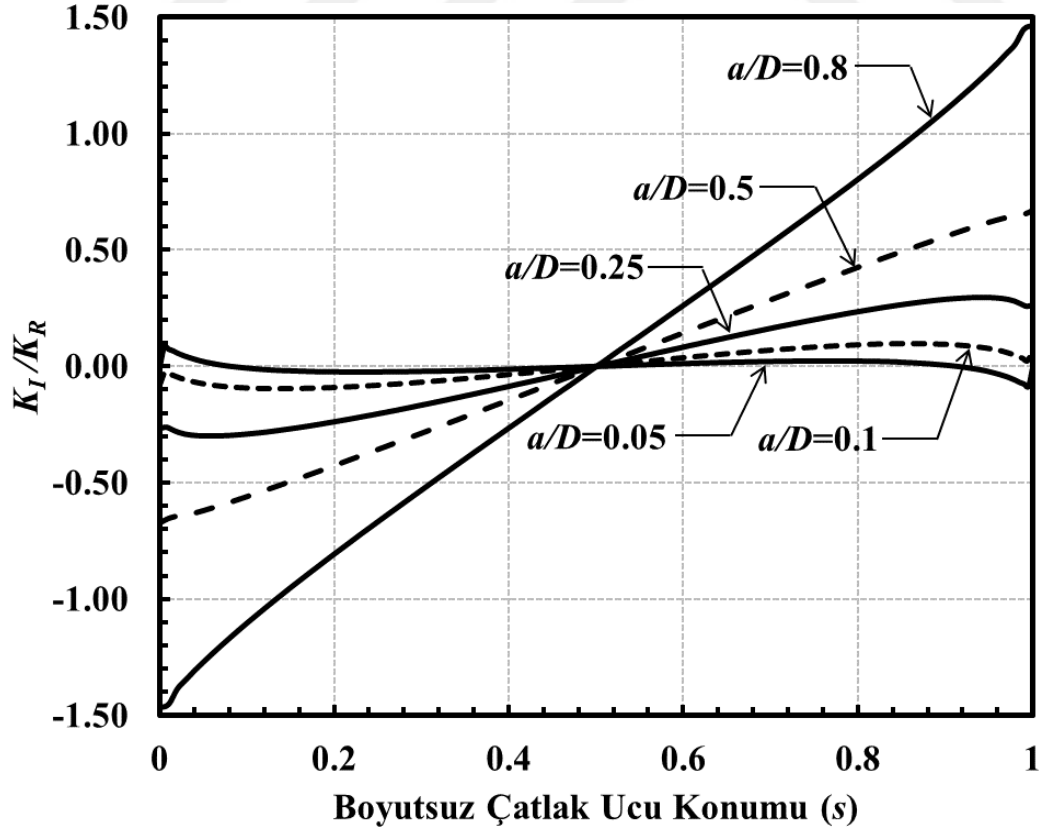
Şekil 3.279. Sabit a/c için çatlak önü boyunca boyutsuz K_I dağılımları (Burulma yükü) ( \alpha=45^\circ , a/c=0.5 ).
