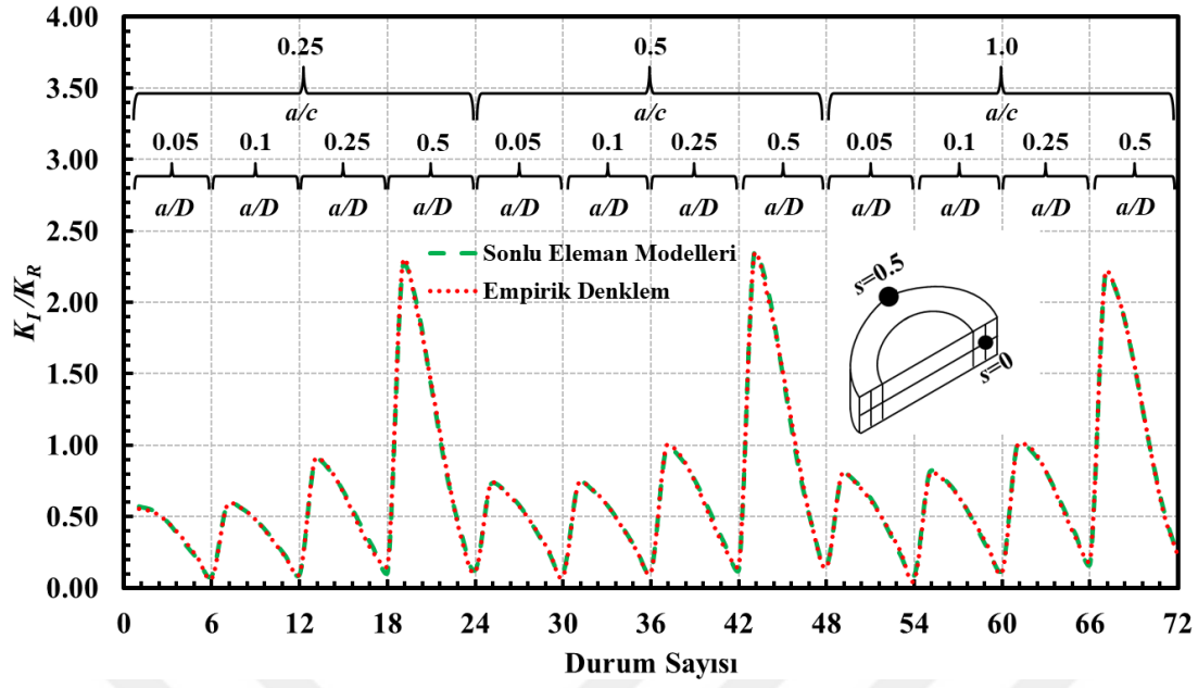
Şekil 4.7. Eksenel gerilme yükü altında silindirde bulunan a/c=0.25-1.0 şekil oranlarına sahip dönmüş yüzey çatlağının serbest yüzey noktası için ( s=0 ) boyutsuz K_I değerleri ile empirik denklem sonucunun karşılaştırılması.
