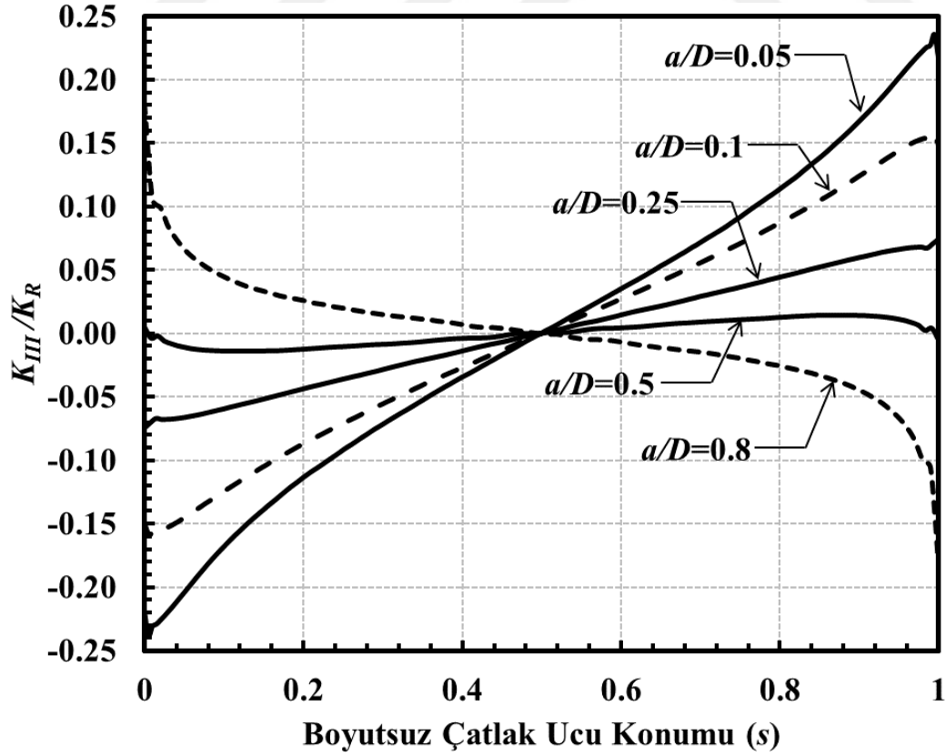
Şekil 3.275. Sabit a/c için çatlak önü boyunca boyutsuz K_{III} dağılımları (Eğilme gerilmesi) ( \alpha=45^\circ , a/c=0.5 ).
