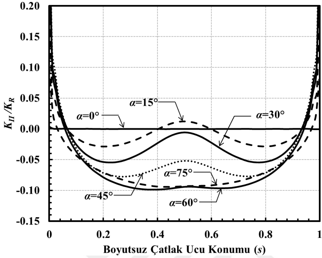
Şekil 3.160. a/c=2 , a/D=0.8 için çatlak önü boyunca boyutsuz K_{II} dağılımları (Eğilme gerilmesi).
