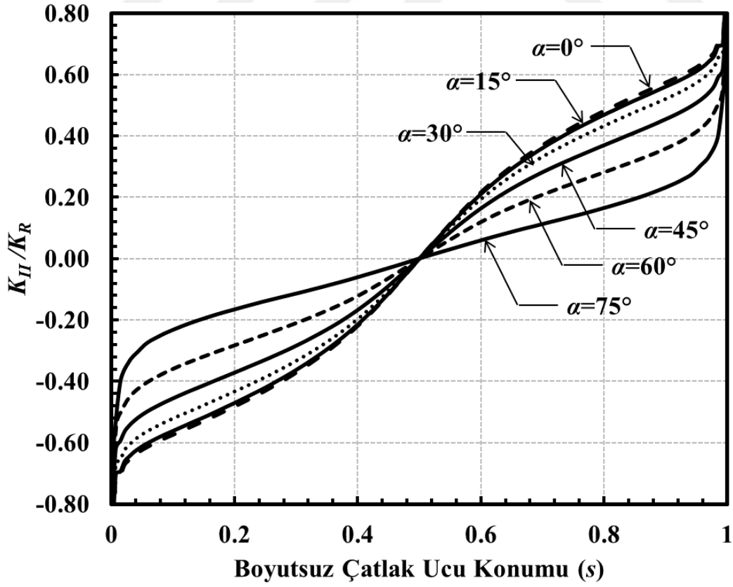
Şekil 3.234. a/c=2 , a/D=0.25 için çatlak önü boyunca boyutsuz K_{II} dağılımları (Burulma yükü).
