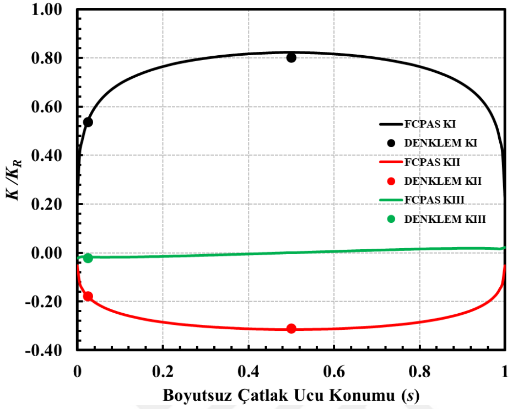
Şekil 4.26. a/c=0.3 , a/D=0.2 , \alpha=35^\circ için boyutsuz K dağılımları ile empirik denklem sonuçları (Eksenel gerilme).
