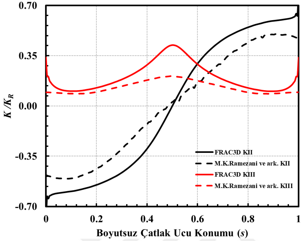
Şekil 3.24. a/c=2 , a/D=0.05 , \beta=0^\circ için boyutsuz K_{II} ve K_{III} sonuçlarının kıyaslanması (Burulma yükü, [18]).
