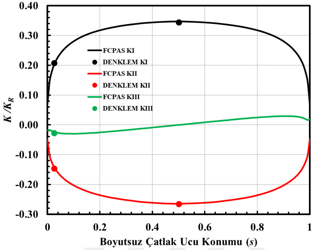
Şekil 4.30. a/c=0.4 , a/D=0.15 , \alpha=65^\circ için boyutsuz K dağılımları ile empirik denklem sonuçları (Eksenel gerilme).
