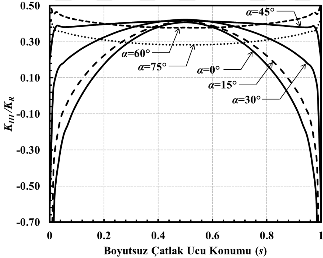
Şekil 3.226. a/c=1 , a/D=0.8 için çatlak önü boyunca boyutsuz K_{III} dağılımları (Burulma yükü).
