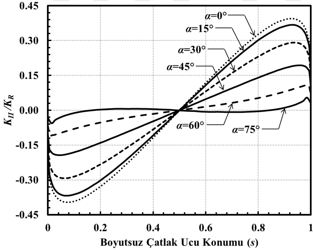
Şekil 3.186. a/c=0.25 , a/D=0.1 için çatlak önü boyunca boyutsuz K_{II} dağılımları (Burulma yükü).
