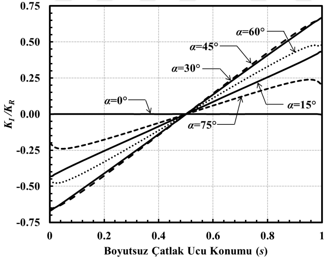
Şekil 3.206. a/c=0.5 , a/D=0.5 için çatlak önü boyunca boyutsuz K_I dağılımları (Burulma yükü).
