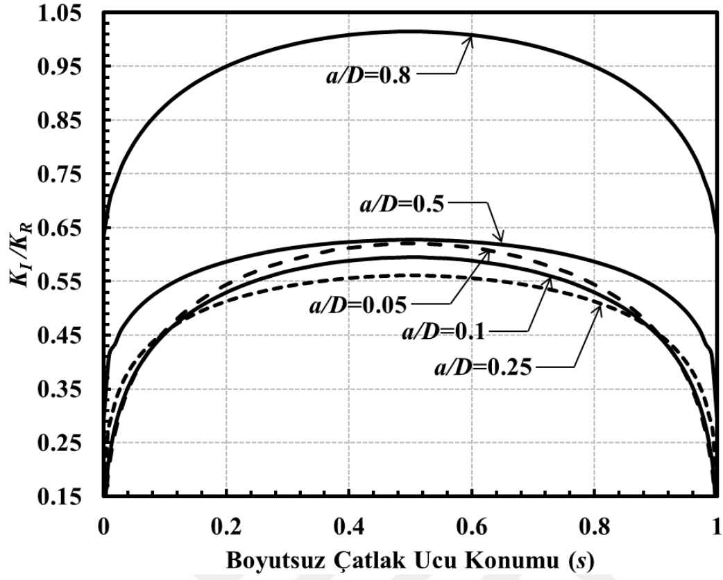
Şekil 3.266. Sabit a/c için çatlak önü boyunca boyutsuz K_I dağılımları (Eğilme gerilmesi) ( \alpha=45^\circ , a/c=0.25 ).
