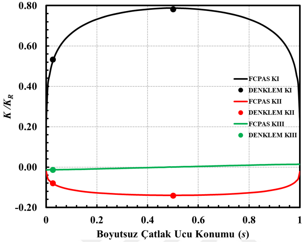
Şekil 4.46. a/c=0.3 , a/D=0.18 , \alpha=18^\circ için boyutsuz K dağılımları ile empirik denklem sonuçları (Eğilme gerilmesi).
