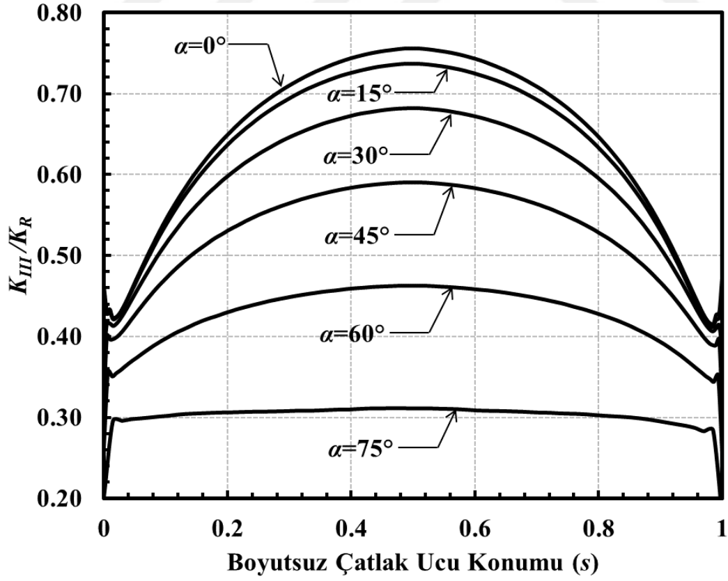
Şekil 3.246. a/c=0.5 , a/D=0.05 ve H/D=3 için çatlak önü boyunca boyutsuz K_{III} dağılımları (Burulma yükü).
