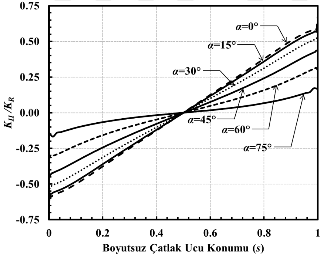
Şekil 3.198. a/c=0.5 , a/D=0.05 için çatlak önü boyunca boyutsuz K_{II} dağılımları (Burulma yükü).
