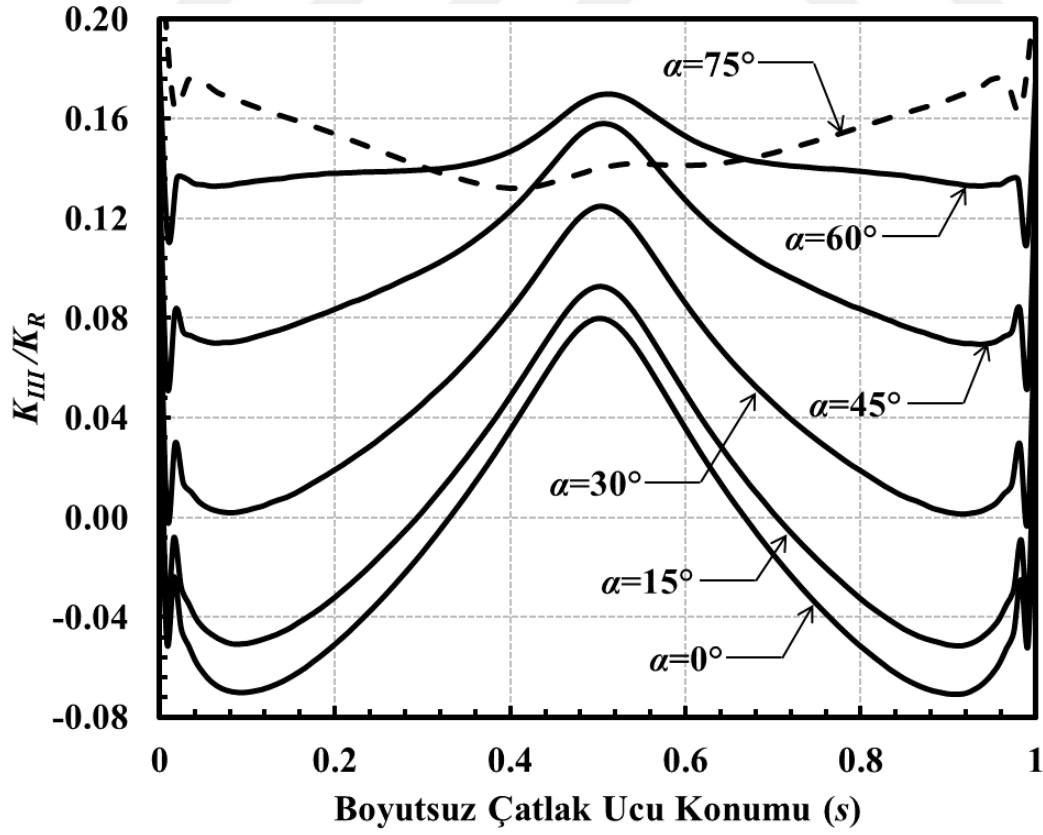
Şekil 3.238. a/c=2 , a/D=0.5 için çatlak önü boyunca boyutsuz K_{III} dağılımları (Burulma yükü).
