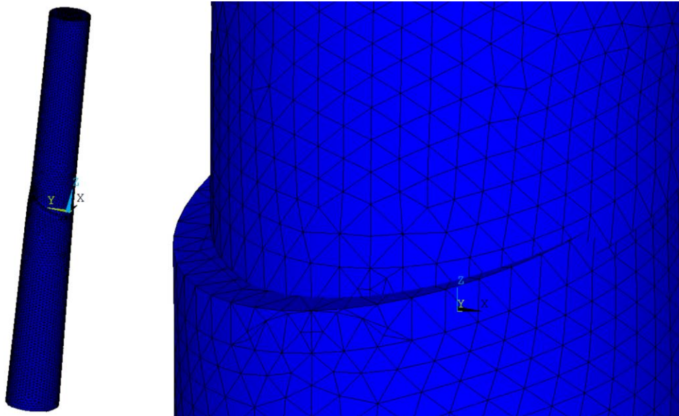
Őekil 3.177. a/c=0.5 , a/D=0.8 , \alpha =30 derece dnmř atlaėa sahip katı silindire uygulanan burulma yk sonucu oluřan deformasyon ve atlık blgesinin yakından grnm [25].
