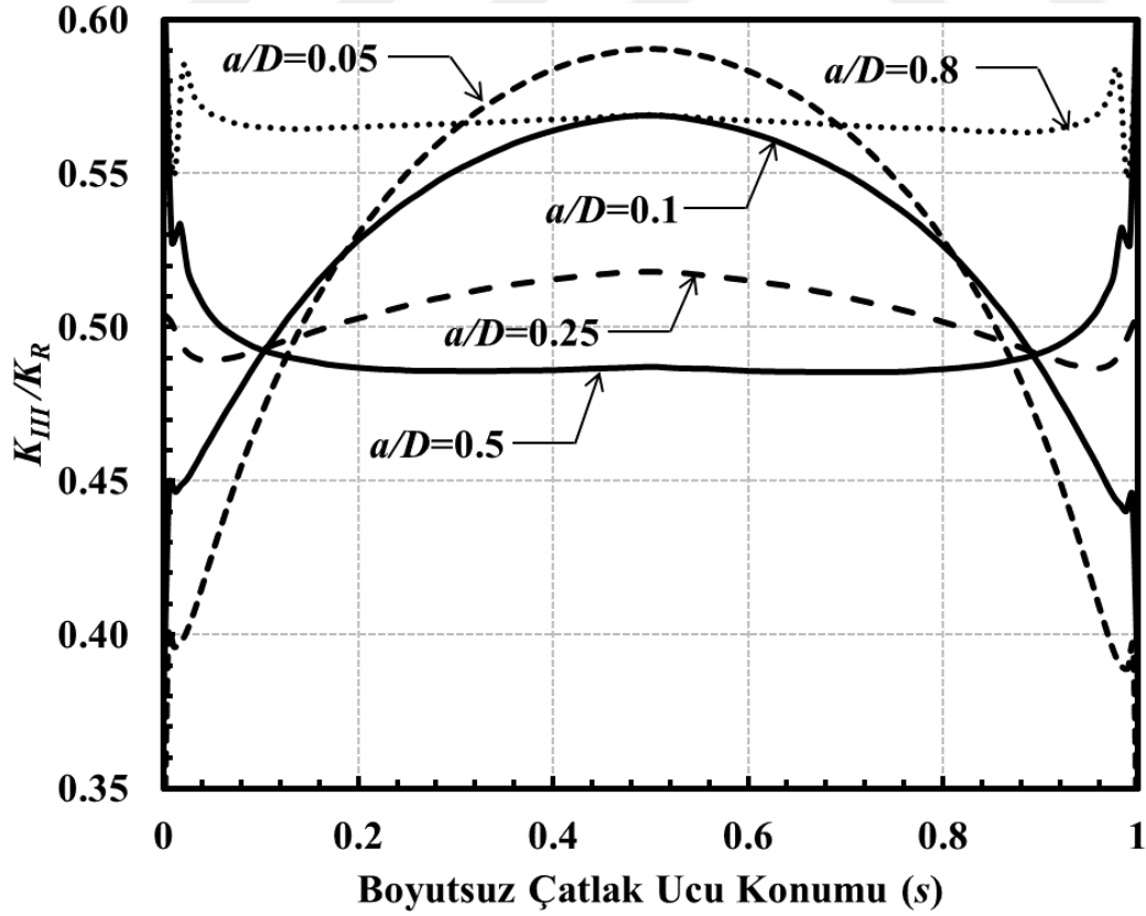
Şekil 3.287. Sabit a/c için çatlak önü boyunca boyutsuz K_{III} dağılımları (Burulma yükü) ( \alpha = 45^\circ , a/c = 0.5 ).
