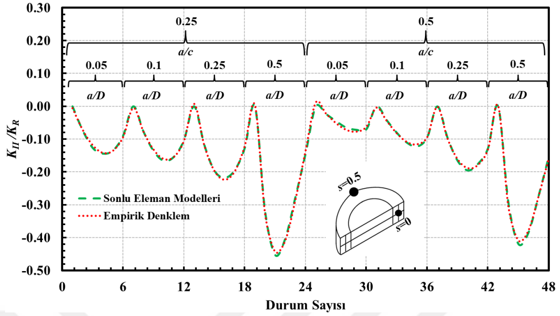
Şekil 4.9. Eksenel gerilme yükü altında silindirde bulunan a/c=0.25-0.5 şekil oranlarına sahip dönmüş yüzey çatlığının serbest yüzey noktası için ( s=0 ) boyutsuz K_{II} değerleri ile empirik denklem sonucunun karşılaştırılması.
