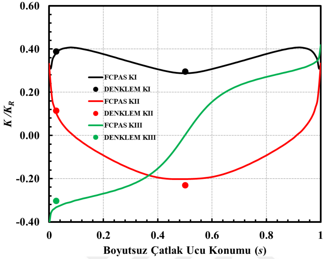
Şekil 4.42. a/c=1.5 , a/D=0.15 , \alpha=50^\circ için boyutsuz K dağılımları ile empirik denklem sonuçları (Eksenel gerilme).
