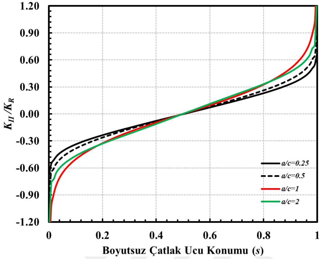
Şekil 3.328. Sabit a/D için çatlak önü boyunca boyutsuz K_{II} dağılımları (Burulma yükü) ( \alpha=45^\circ , a/D=0.5 ).
