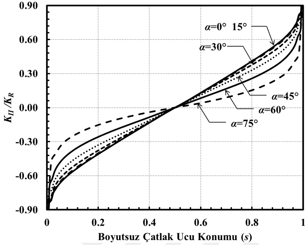
Şekil 3.237. a/c=2 , a/D=0.5 için çatlak önü boyunca boyutsuz K_{II} dağılımları (Burulma yükü).
