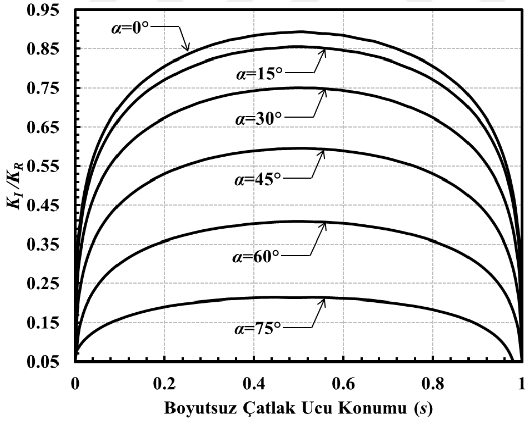
Şekil 3.105. a/c=0.25 , a/D=0.1 için çatlak önü boyunca boyutsuz K_I dağılımları (Eğilme gerilmesi).
