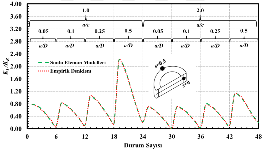
Şekil 4.8. Eksenel gerilme yükü altında silindirde bulunan a/c=1.0-2.0 şekil oranlarına sahip dönmüş yüzey çatlağının serbest yüzey noktası için ( s=0 ) boyutsuz K_I değerleri ile empirik denklem sonucunun karşılaştırılması.
