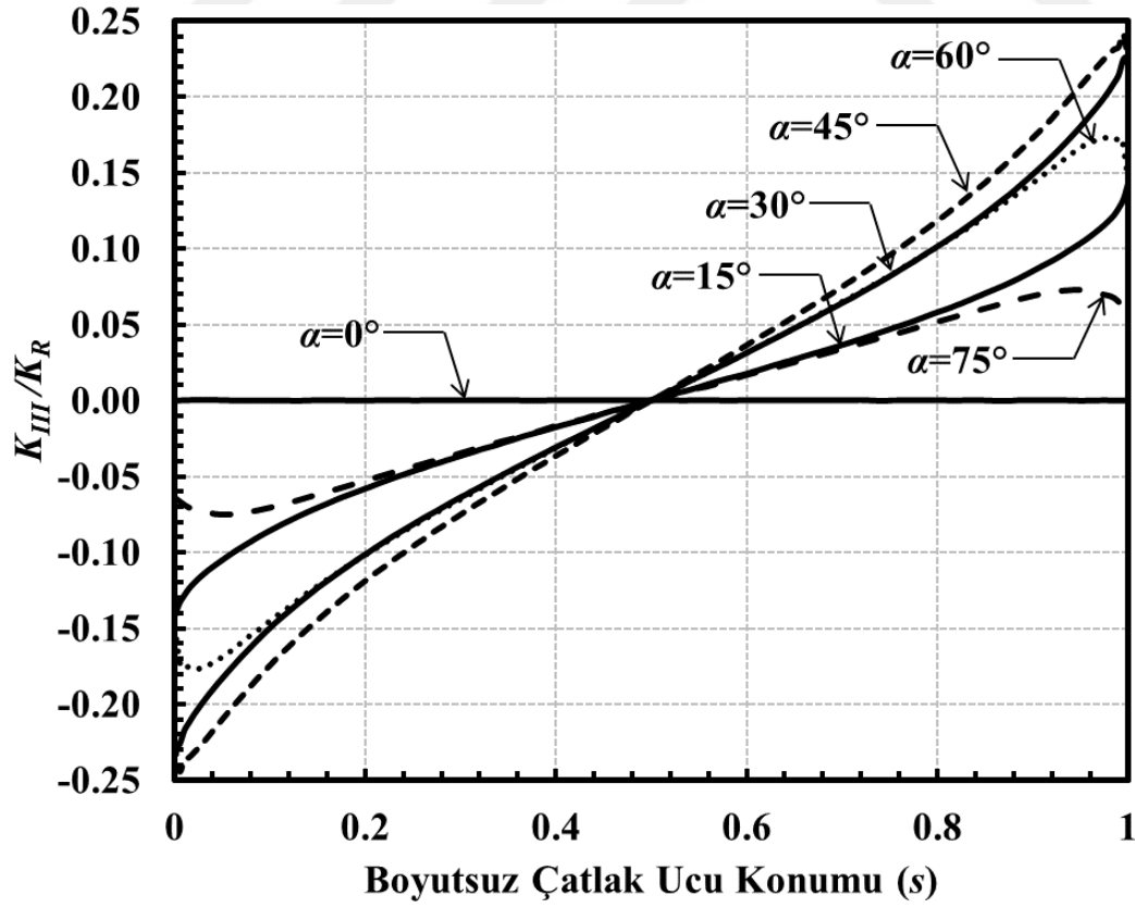
Şekil 3.45. a/c=0.5 , a/D=0.05 için çatlak önü boyunca boyutsuz K_{III} dağılımları (Eksenel gerilme).
