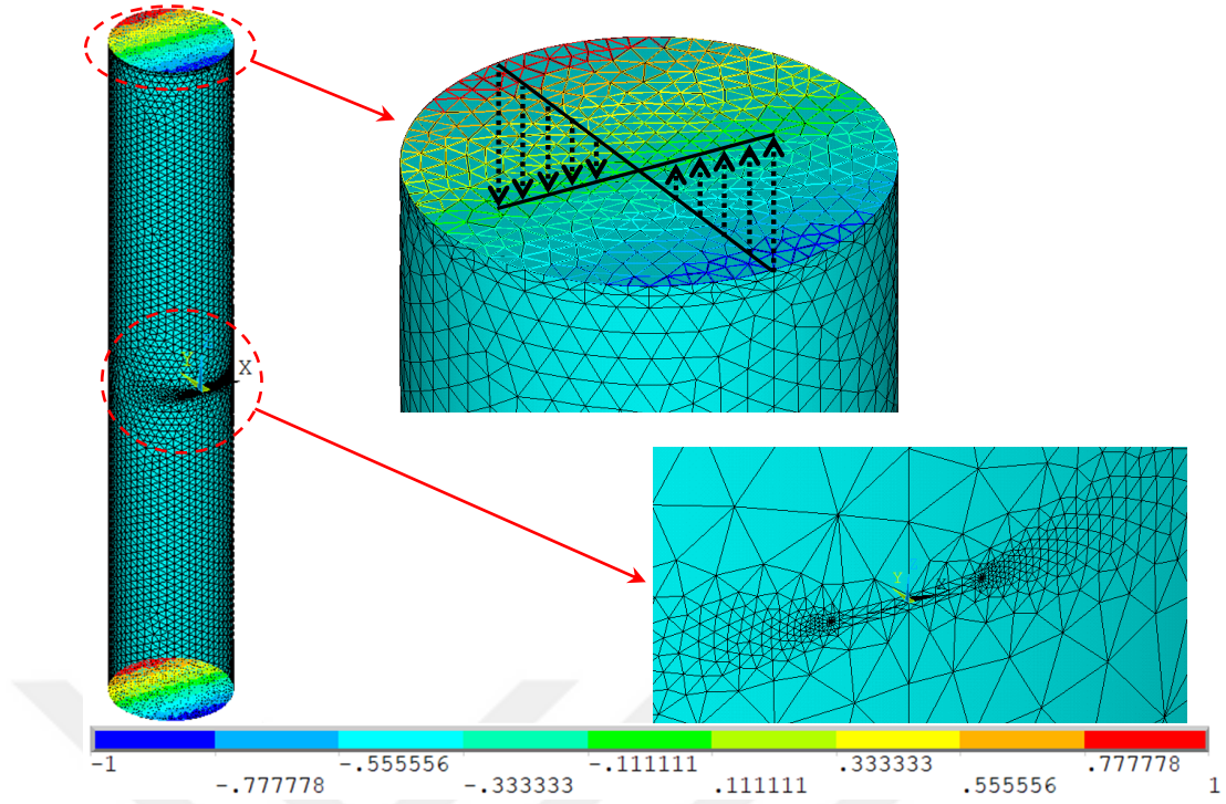
Şekil 3.100. a/c=1 , a/D=0.05 , \alpha =15^\circ olan dönmüş yüzey çatlakına sahip katı bir silindirin global sonlu elemanlar modeli, eğilme gerilme yüklemesi ve çatlak bölgesinin yakından görünümü.
