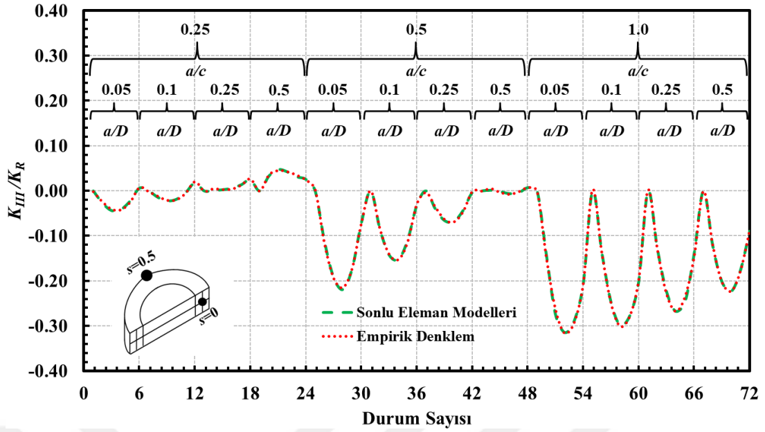
Şekil 4.17. Eğilme yükü altında silindirde bulunan a/c=0.25-1.0 şekil oranlarına sahip dönmüş yüzey çatlağının serbest yüzey noktası için ( s=0 ) boyutsuz K_{III} değerleri ile empirik denklem sonucunun karşılaştırılması.
