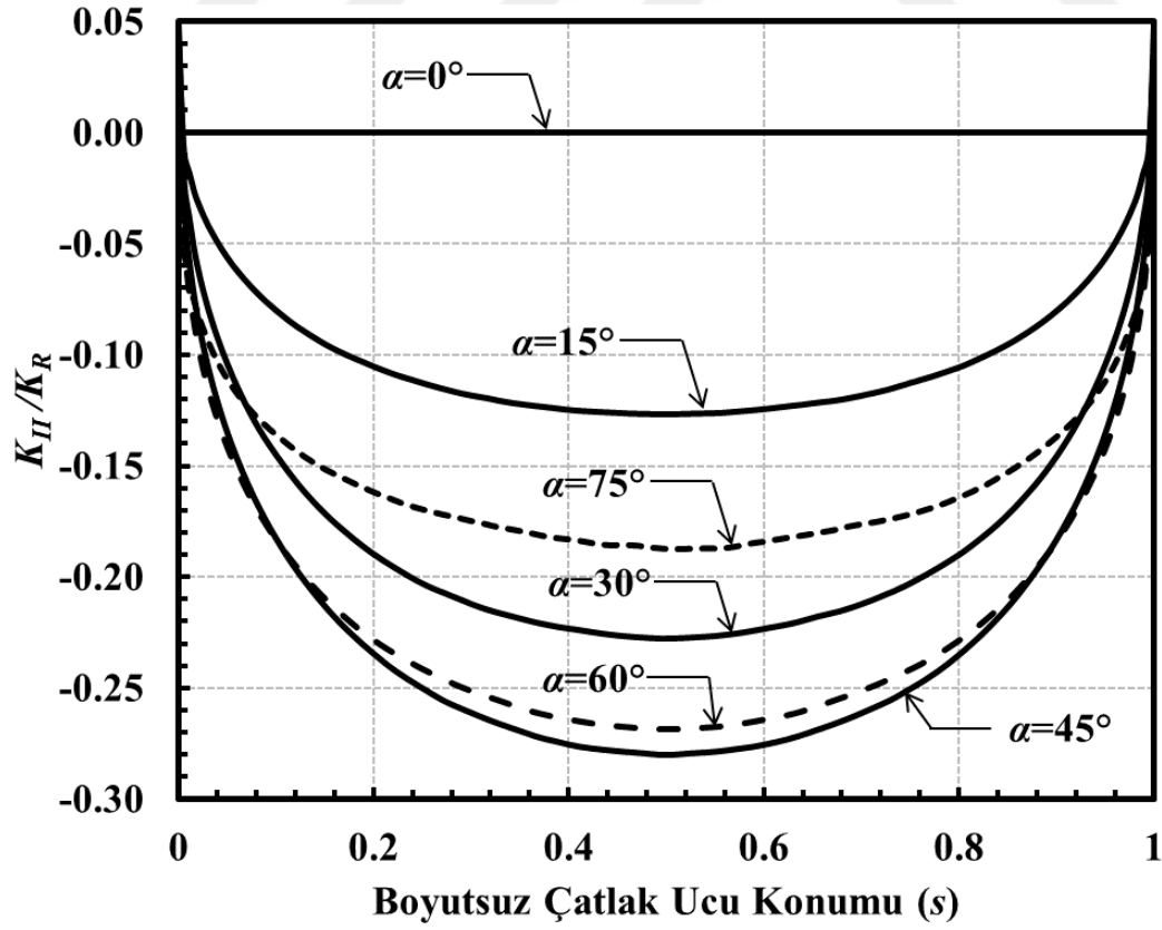
Şekil 3.121. a/c=0.5 , a/D=0.1 için çatlak önü boyunca boyutsuz K_{II} dağılımları (Eğilme gerilmesi).
