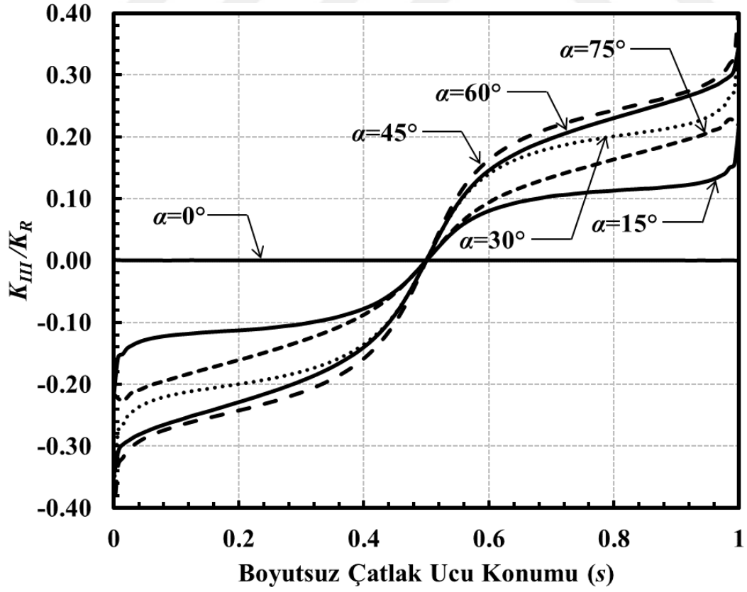
Şekil 3.81. a/c=2 , a/D=0.25 için çatlak önü boyunca boyutsuz K_{III} dağılımları (Eksenel gerilme).
