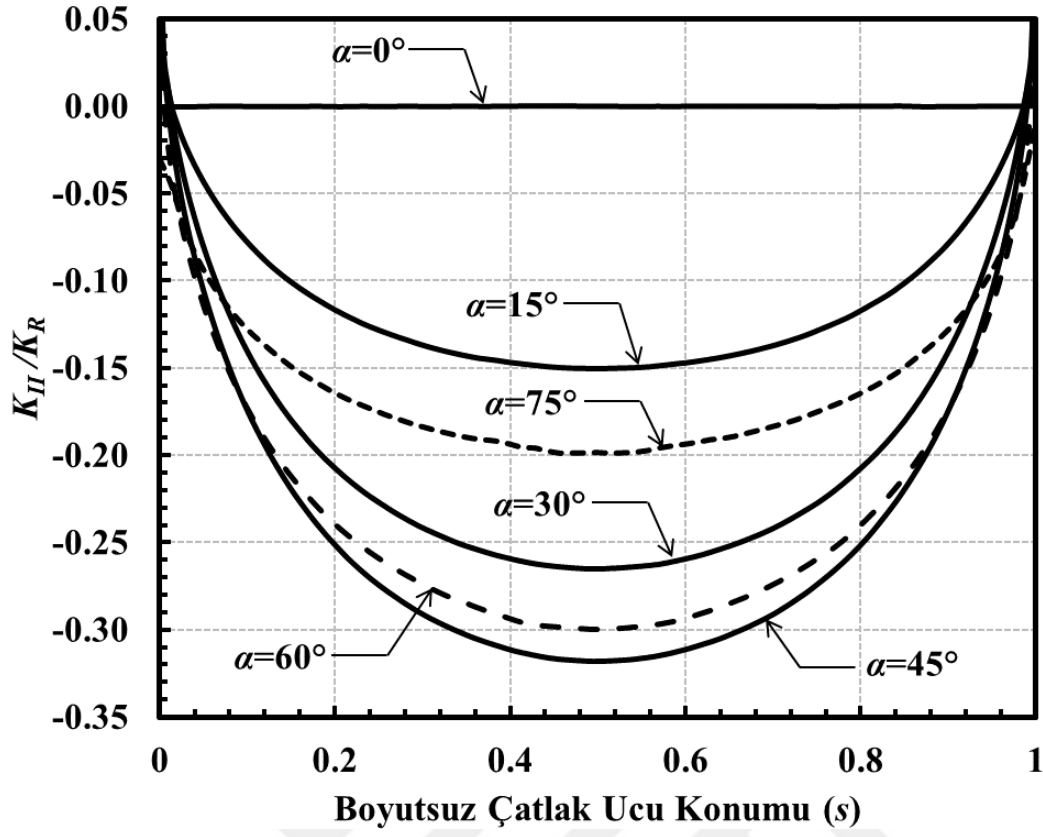
Şekil 3.44. a/c=0.5 , a/D=0.05 için çatlak önü boyunca boyutsuz K_{II} dağılımları (Eksenel gerilme).
