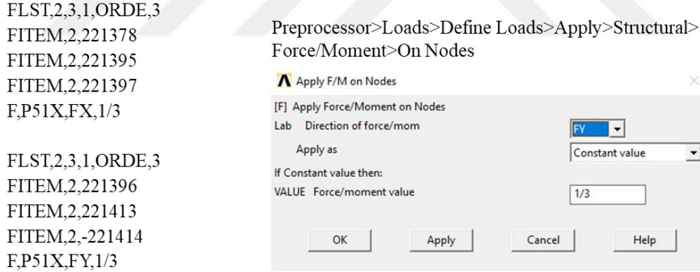
Şekil 5.28. Burulma yükü için düğümlerden kuvvet tanımlanması.
