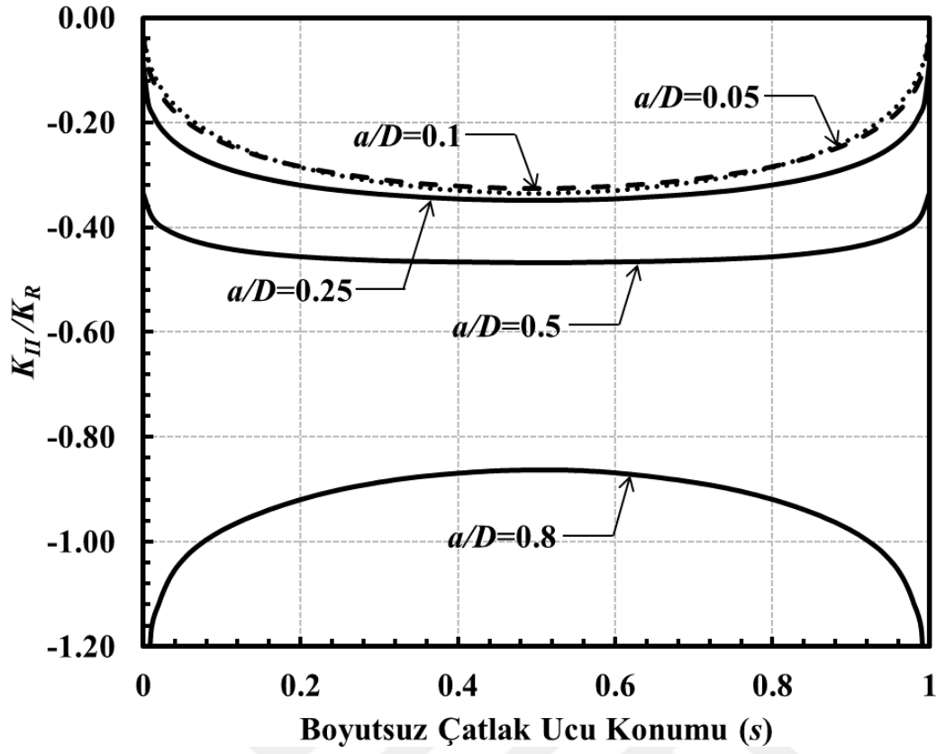
Şekil 3.258. Sabit a/c için çatlak önü boyunca boyutsuz K_{II} dağılımları (Eksenel gerilme) ( \alpha=45^\circ , a/c=0.25 ).
