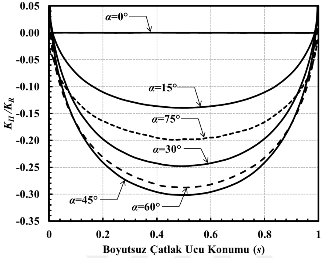
Şekil 3.164. a/c=0.5 , a/D=0.05 ve H/D=3 için çatlak önü boyunca boyutsuz K_{II} dağılımları (Eğilme gerilmesi).
