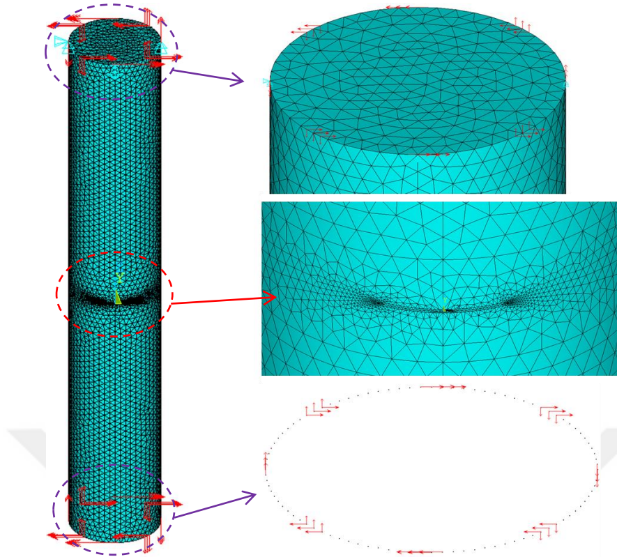
Şekil 3.174. a/c=0.25 , a/D=0.05 , \alpha =15^\circ olan dönmüş yüzey çatlağına sahip katı silindirin global sonlu elemanlar modeli, burulma yükü için kuvvet dağılımlarının ve çatlak bölgesinin yakından görünümü.
