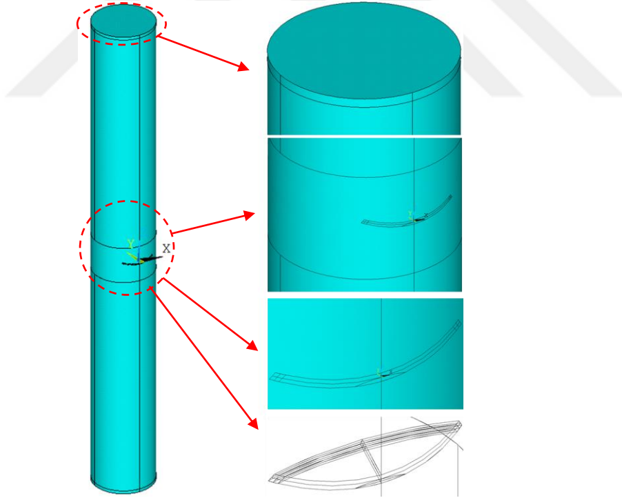
Şekil 3.5. Eğilme yükü için oluşturulan silindir tasarımı ve çatlak tünel hacmi modeli.
