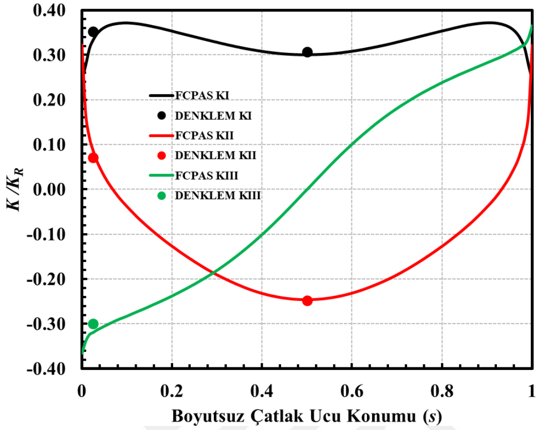
Şekil 4.38. a/c=1.2 , a/D=0.14 , \alpha=55^\circ için boyutsuz K dağılımları ile empirik denklem sonuçları (Eksenel gerilme).
