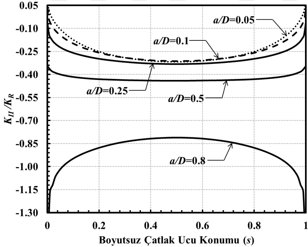
Şekil 3.259. Sabit a/c için çatlak önü boyunca boyutsuz K_{II} dağılımları (Eksenel gerilme) ( \alpha=45^\circ , a/c=0.5 ).
