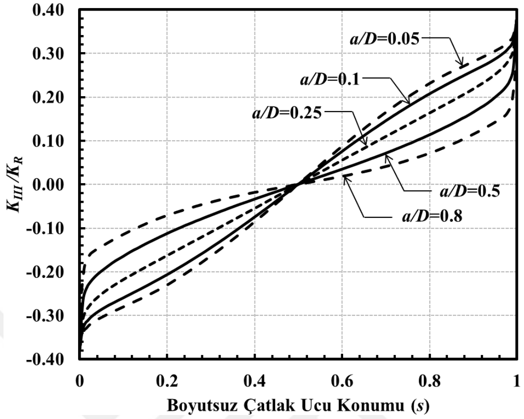
Şekil 3.276. Sabit a/c için çatlak önü boyunca boyutsuz K_{III} dağılımları (Eğilme gerilmesi) ( \alpha=45^\circ , a/c=1 ).
