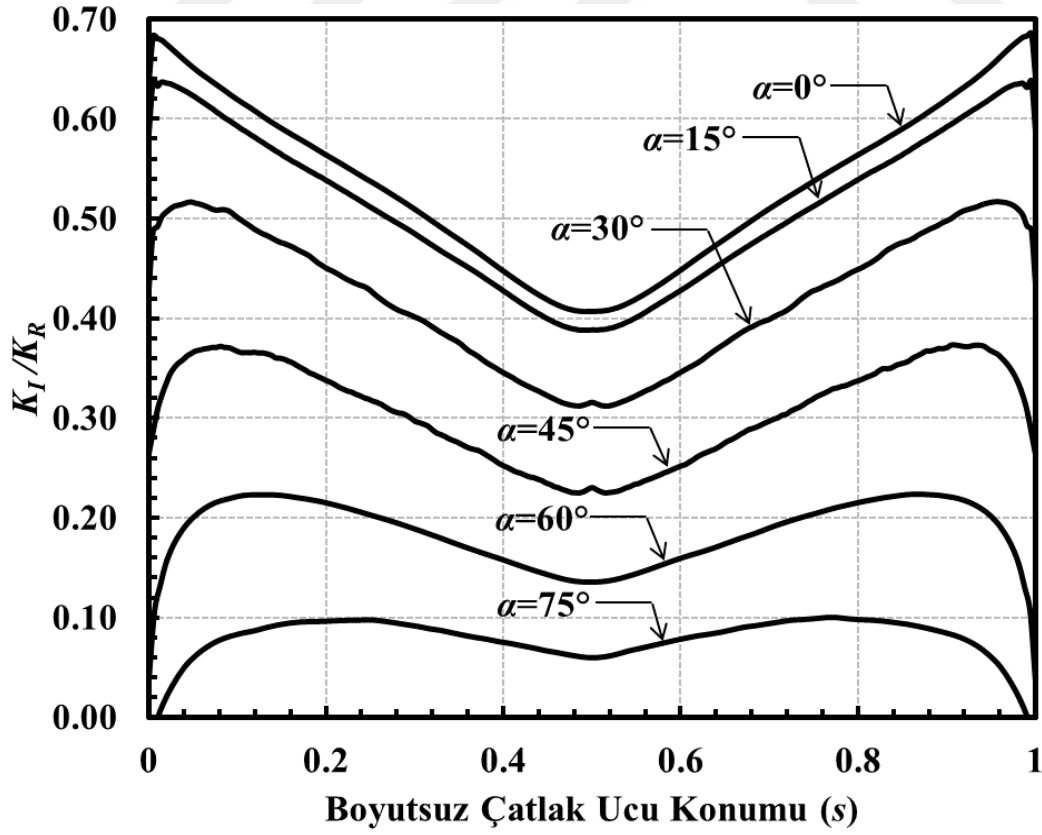
Şekil 3.169. a/c=2 , a/D=0.05 ve H/D=6 için çatlak önü boyunca boyutsuz K_I dağılımları (Eğilme gerilmesi).
