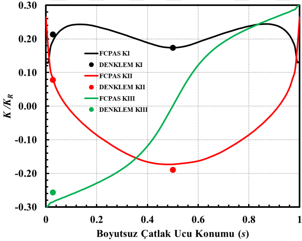
Şekil 4.43. a/c=1.5 , a/D=0.15 , \alpha=65^\circ için boyutsuz K dağılımları ile empirik denklem sonuçları (Eksenel gerilme).
