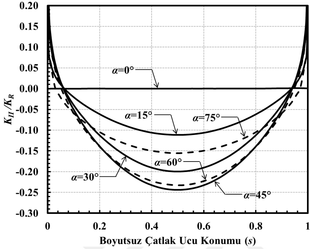
Şekil 3.136. a/c=1 , a/D=0.1 için çatlak önü boyunca boyutsuz K_{II} dağılımları (Eğilme gerilmesi).
