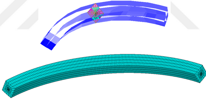
Şekil 5.16. Çatlak tünel hacminin oluşturulması.
