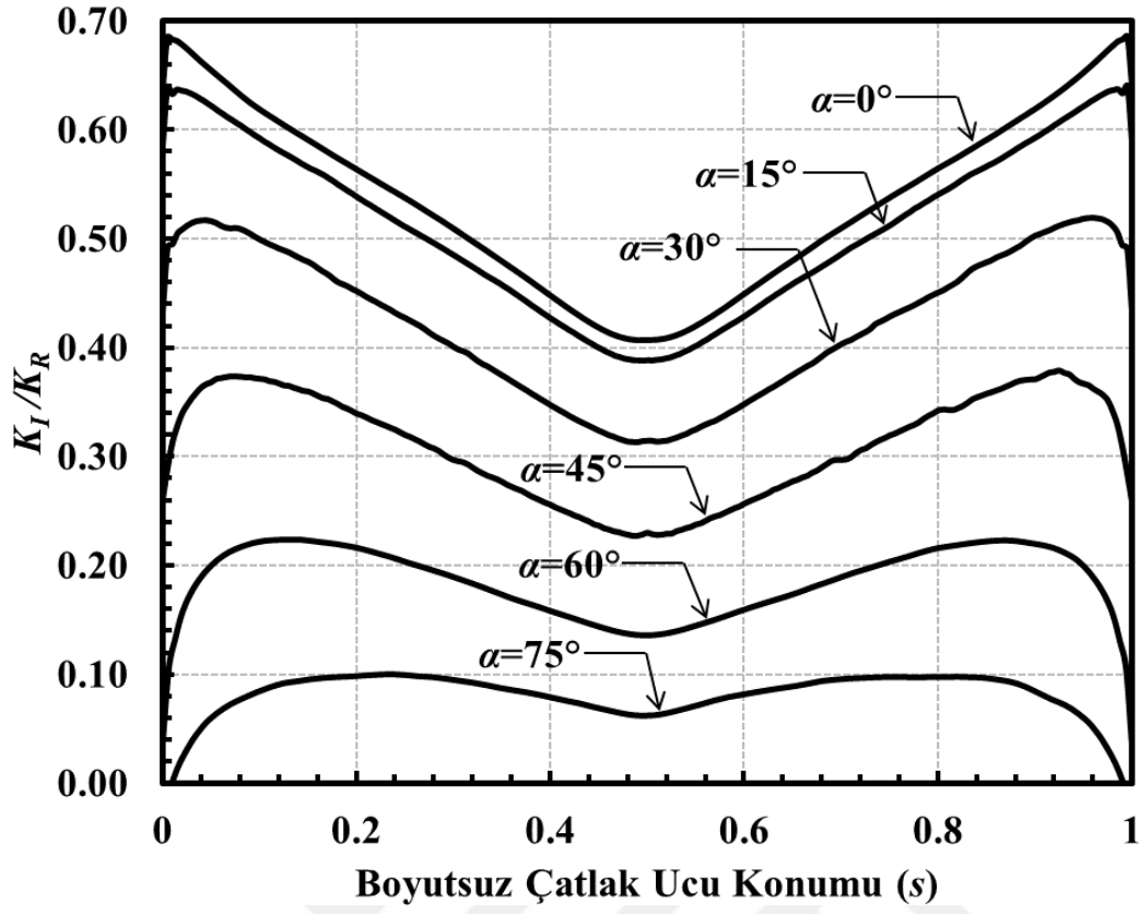
Şekil 3.168. a/c=2 , a/D=0.05 ve H/D=3 için çatlak önü boyunca boyutsuz K_I dağılımları (Eğilme gerilmesi).
