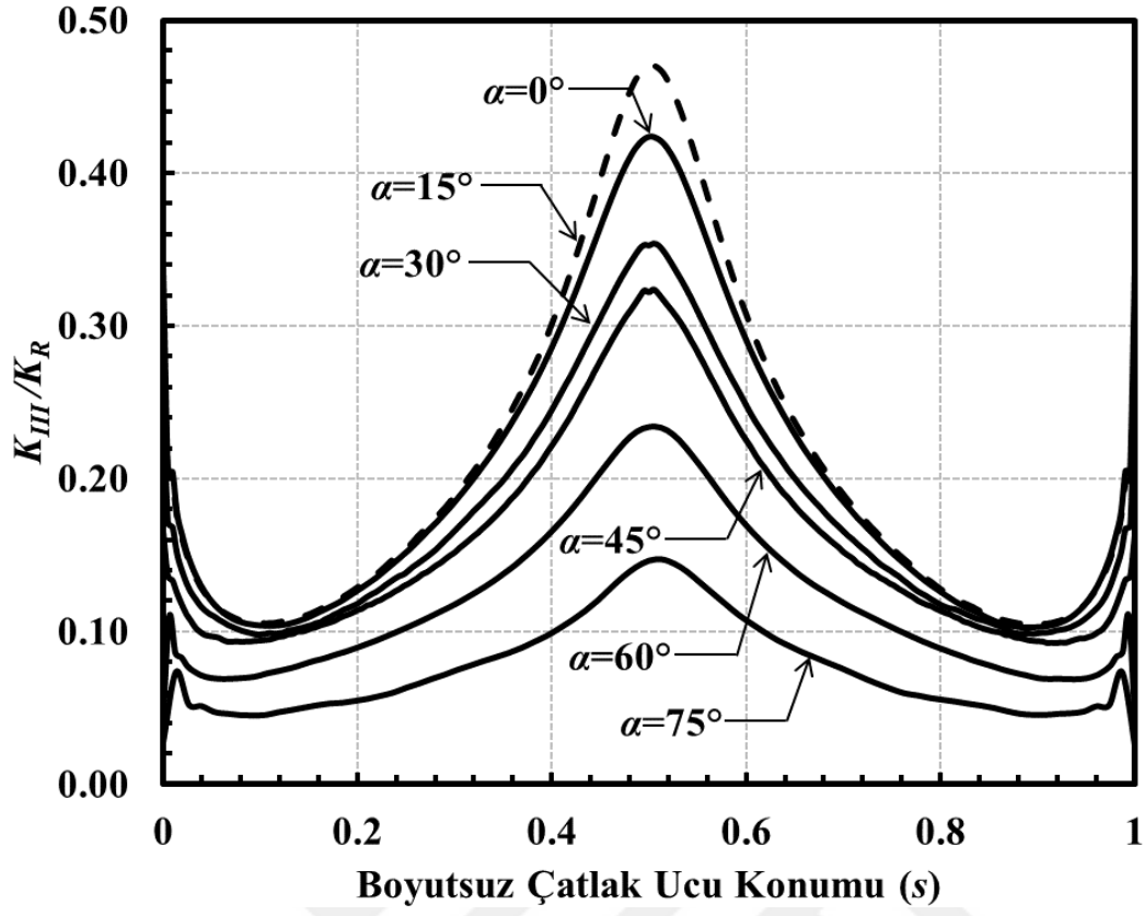
Şekil 3.229. a/c=2 , a/D=0.05 için çatlak önü boyunca boyutsuz K_{III} dağılımları (Burulma yükü).
