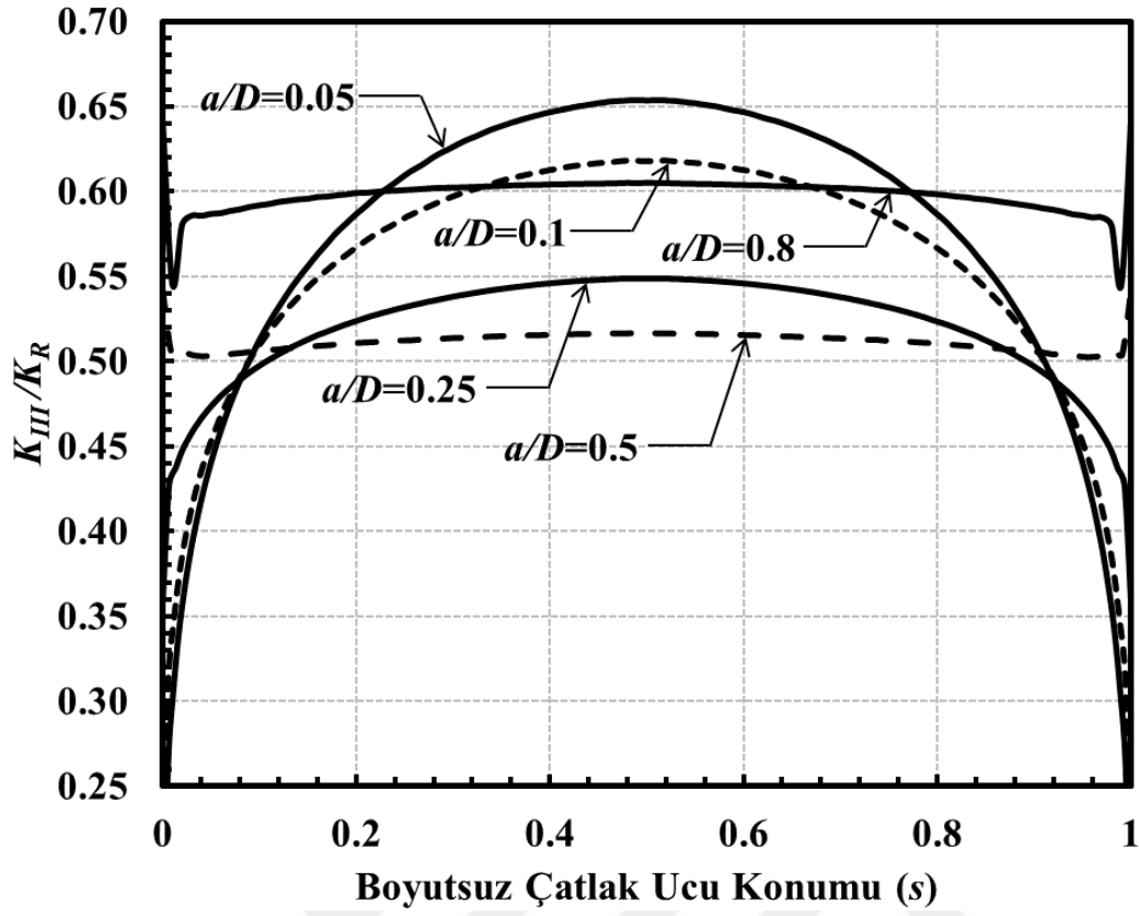
Şekil 3.286. Sabit a/c için çatlak önü boyunca boyutsuz K_{III} dağılımları (Burulma yükü) ( \alpha = 45^\circ , a/c = 0.25 ).
