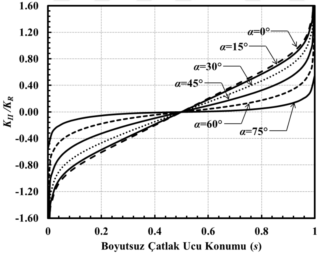
Şekil 3.222. a/c=1 , a/D=0.5 için çatlak önü boyunca boyutsuz K_{II} dağılımları (Burulma yükü).
