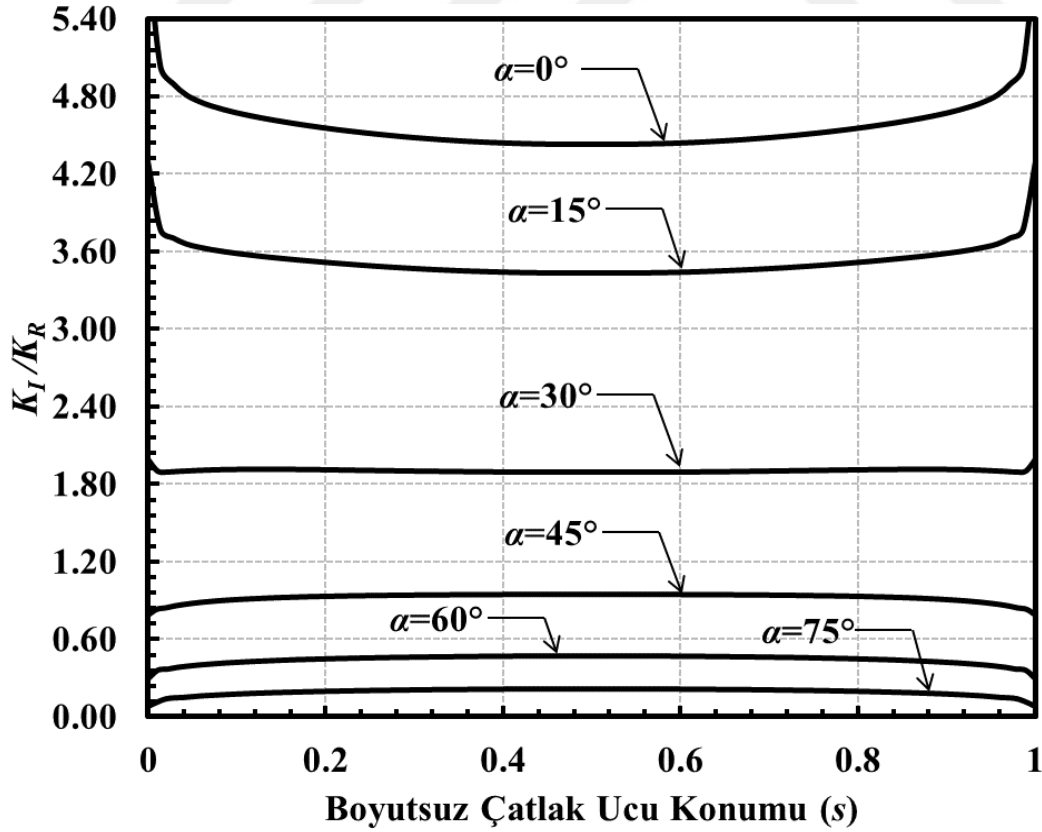
Şekil 3.129. a/c=0.5 , a/D=0.8 için çatlak önü boyunca boyutsuz K_I dağılımları (Eğilme gerilmesi).
