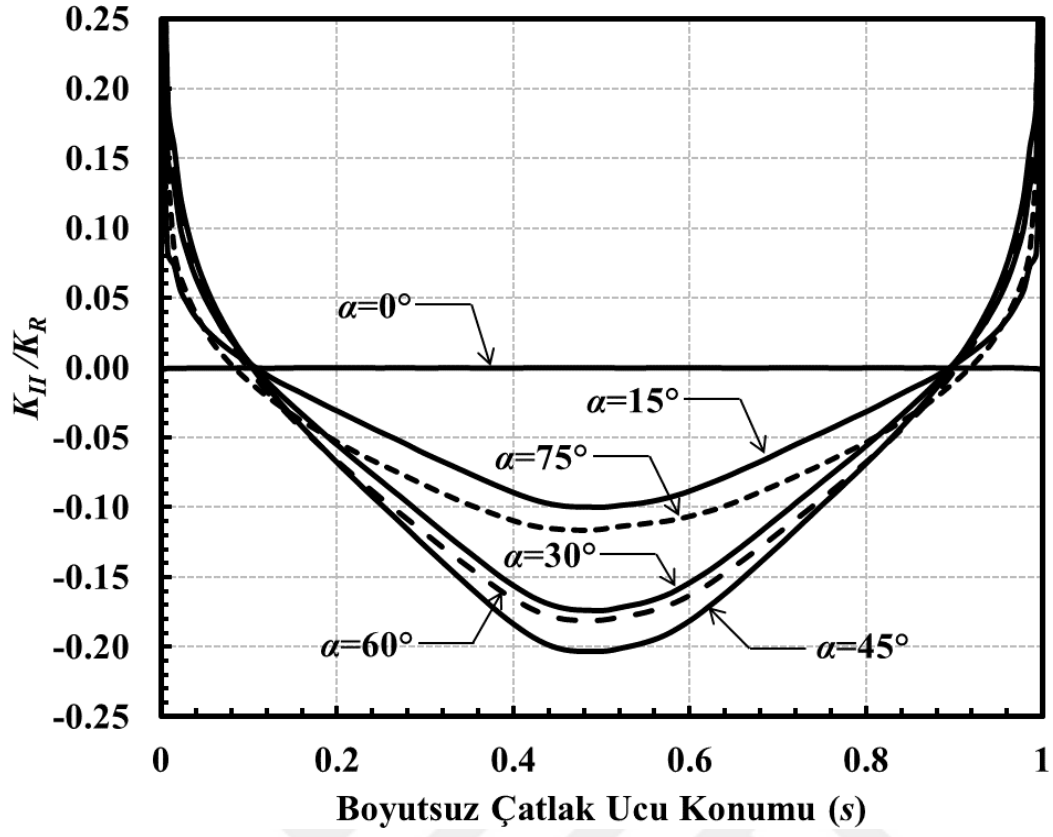
Şekil 3.80. a/c=2 , a/D=0.25 için çatlak önü boyunca boyutsuz K_{II} dağılımları (Eksenel gerilme).
