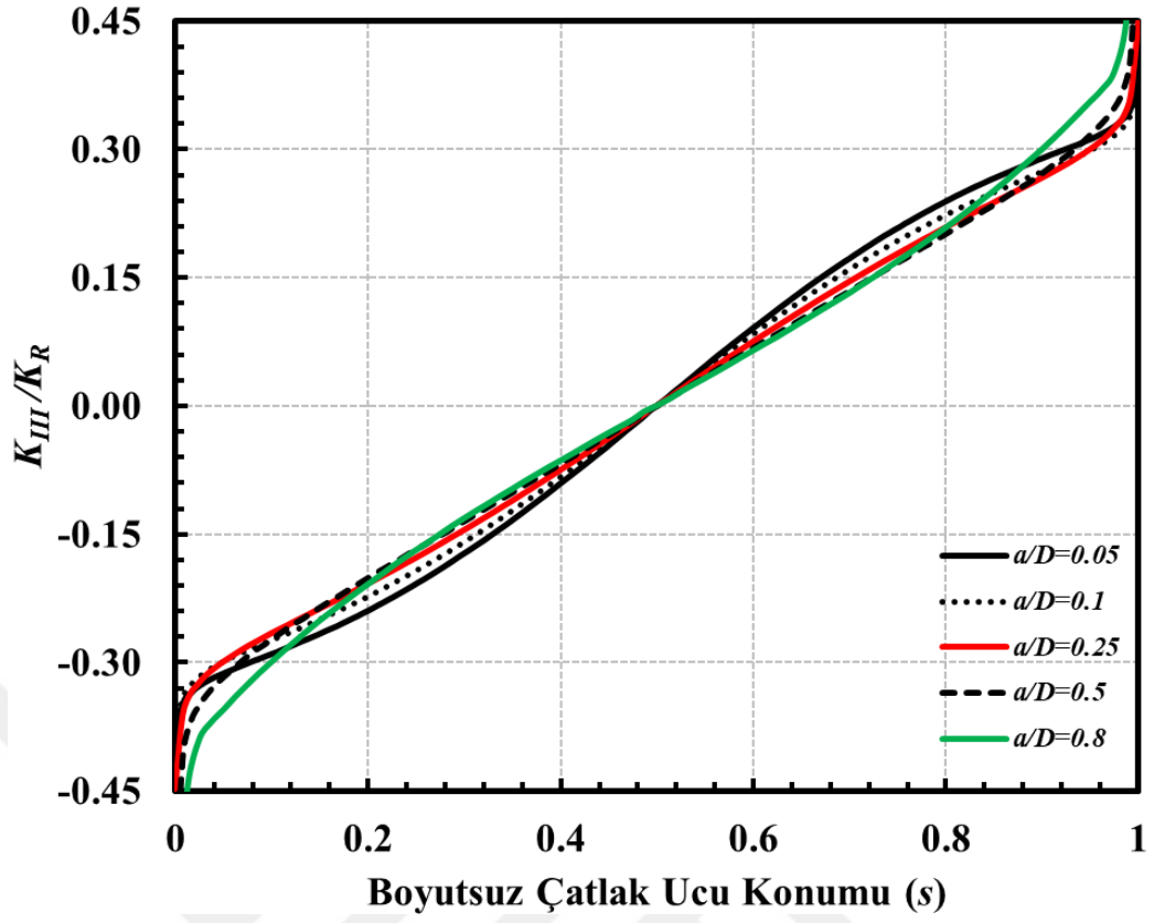
Şekil 3.264. Sabit a/c için çatlak önü boyunca boyutsuz K_{III} dağılımları (Eksenel gerilme) ( \alpha=45^\circ , a/c=1 ).
