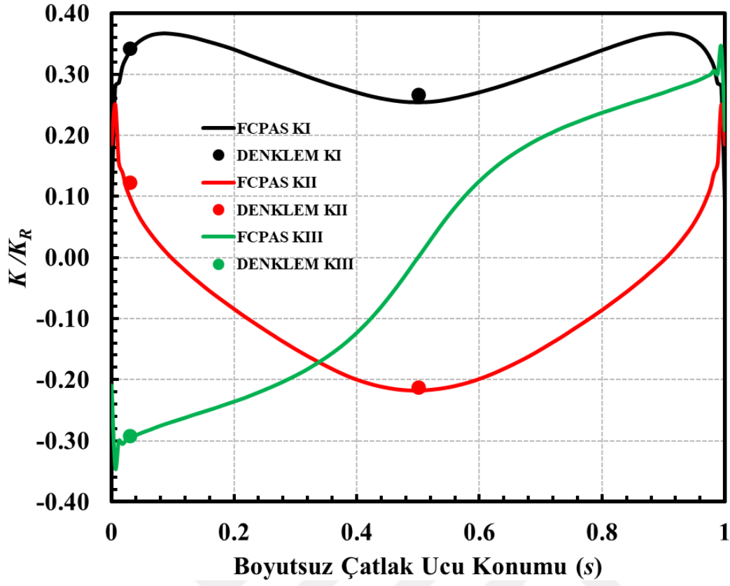
Şekil 4.62. a/c=1.5 , a/D=0.08 , \alpha=50^\circ için boyutsuz K dağılımları ile empirik denklem sonuçları (Eğilme gerilmesi).
