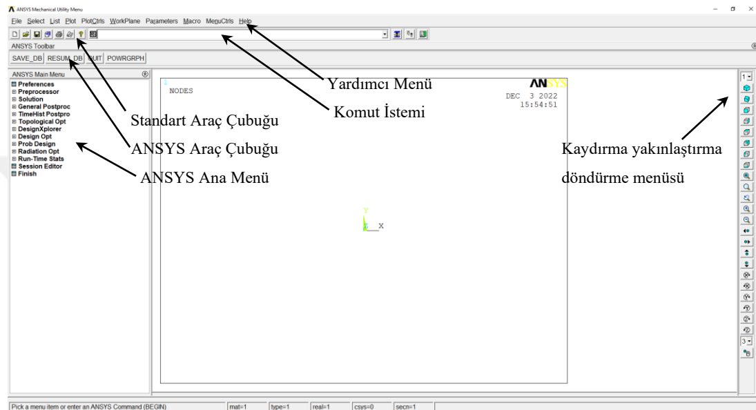
Şekil 5.1. ANSYS Mechanical APDL (Parametrik Tasarım Dili) kullanıcı arayüzü.
