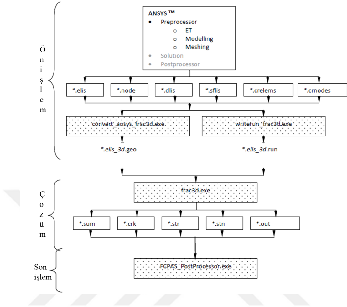
Şekil 3.10. FCPAS ile kırılma analizi basamakları [26].
