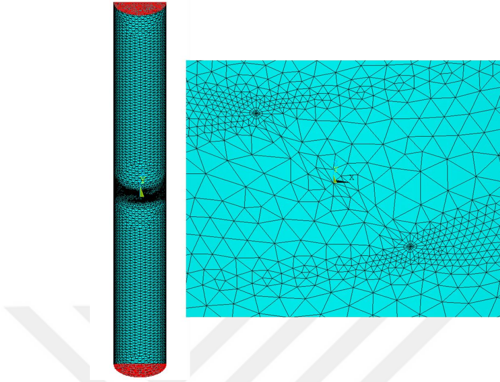
Şekil 3.16. a/c=1 , a/D=0.1 , \beta=45^\circ boyutlarına sahip eğik dairesel yüzey çatlaklı içeren katı silindirin simetrik sonlu eleman modeli ve çatlak önü yakın görüntüsü.
