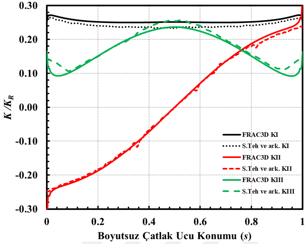
Şekil 3.20. a/c=1 , a/D=0.05 , \beta =45^\circ için boyutsuz K_I , K_{II} ve K_{III} sonuçlarının kıyaslanması (Eksenel gerilme, [19]).
