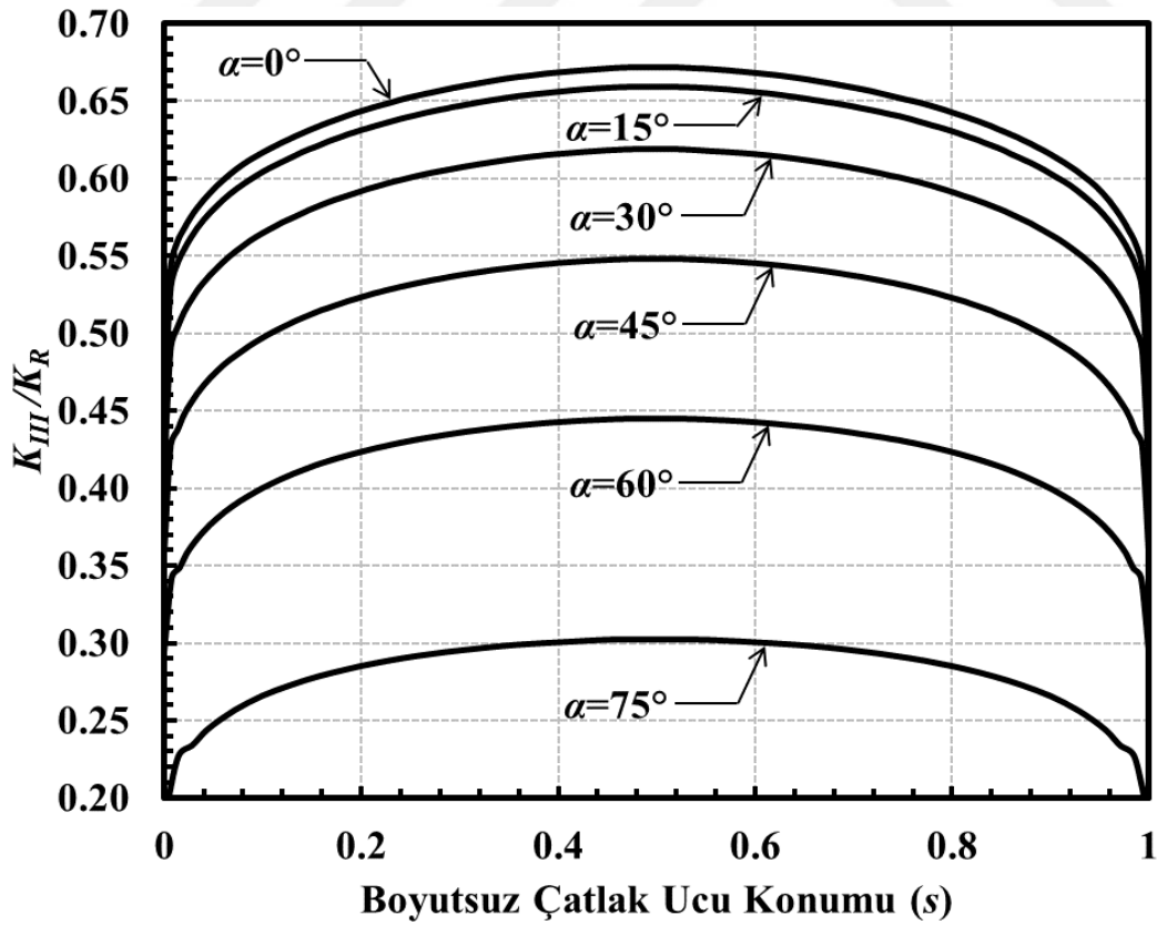
Şekil 3.190. a/c=0.25 , a/D=0.25 için çatlak önü boyunca boyutsuz K_{III} dağılımları (Burulma yükü).
