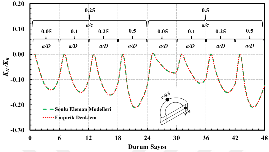
Şekil 4.15. Eğilme yükü altında silindirde bulunan a/c=0.25-0.5 şekil oranlarına sahip dönmüş yüzey çatlağının serbest yüzey noktası için ( s=0 ) boyutsuz K_{II} değerleri ile empirik denklem sonucunun karşılaştırılması.
