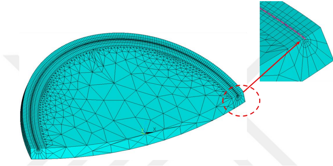
Şekil 4.6. Çatlak önü serbest yüzey bölgelerinin ağ yapıları.
