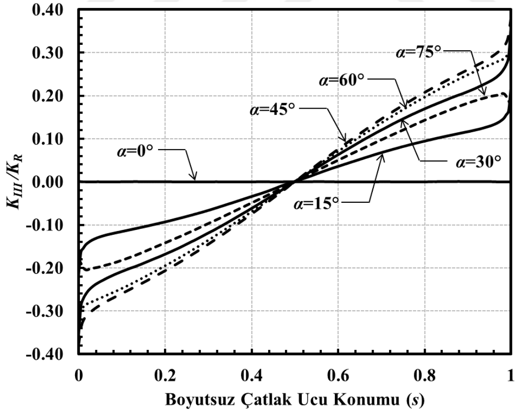
Şekil 3.137. a/c=1 , a/D=0.1 için çatlak önü boyunca boyutsuz K_{III} dağılımları (Eğilme gerilmesi).
