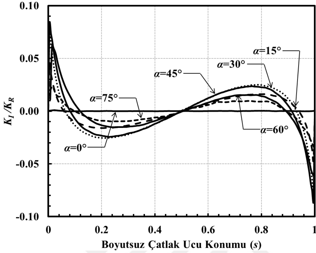
Şekil 3.197. a/c=0.5 , a/D=0.05 için çatlak önü boyunca boyutsuz K_I dağılımları (Burulma yükü).
