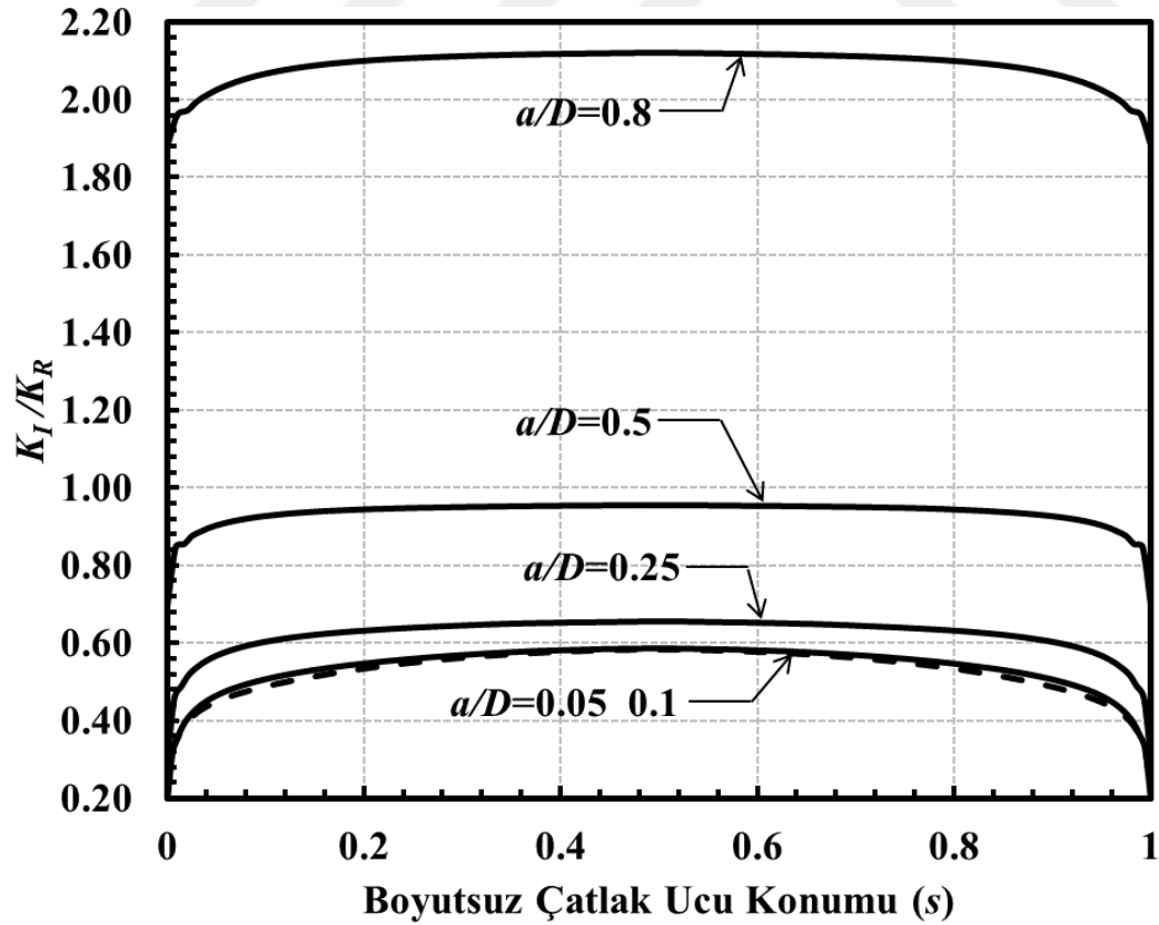
Şekil 3.255. Sabit a/c için çatlak önü boyunca boyutsuz K_I dağılımları (Eksenel gerilme) ( \alpha=45^\circ , a/c=0.5 ).
