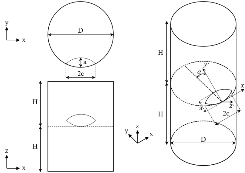
Şekil 3.1. Silindir üst görünüş, ön görünüş, silindir yüzeyine konumlandırılan eliptik dönmüş yüzey çatlak ve problemi tanımlayan parametreler.
