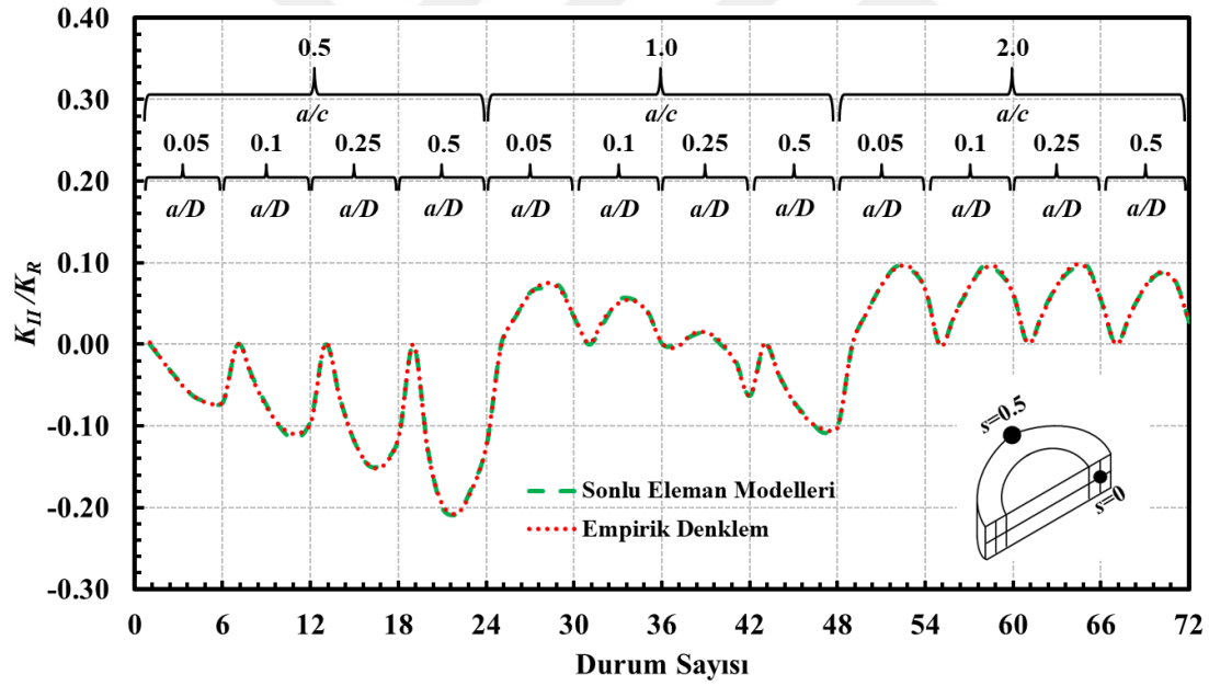
Şekil 4.16. Eğilme yükü altında silindirde bulunan a/c=0.5-2.0 şekil oranlarına sahip dönmüş yüzey çatlağının serbest yüzey noktası için ( s=0 ) boyutsuz K_{II} değerleri ile empirik denklem sonucunun karşılaştırılması.
