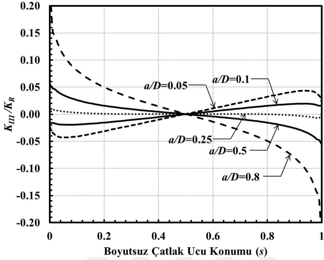
Şekil 3.274. Sabit a/c için çatlak önü boyunca boyutsuz K_{III} dağılımları (Eğilme gerilmesi) ( \alpha=45^\circ , a/c=0.25 ).
