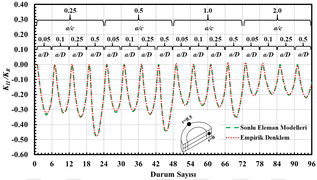
Şekil 4.22. Eksenel gerilme yükü altında silindirde bulunan dönmüş yüzey çatlaklarının çatlak ucu derinlik noktası için ( s=0.5 ) boyutsuz K_{II} değerleri ile empirik denklem sonucunun karşılaştırılması.
