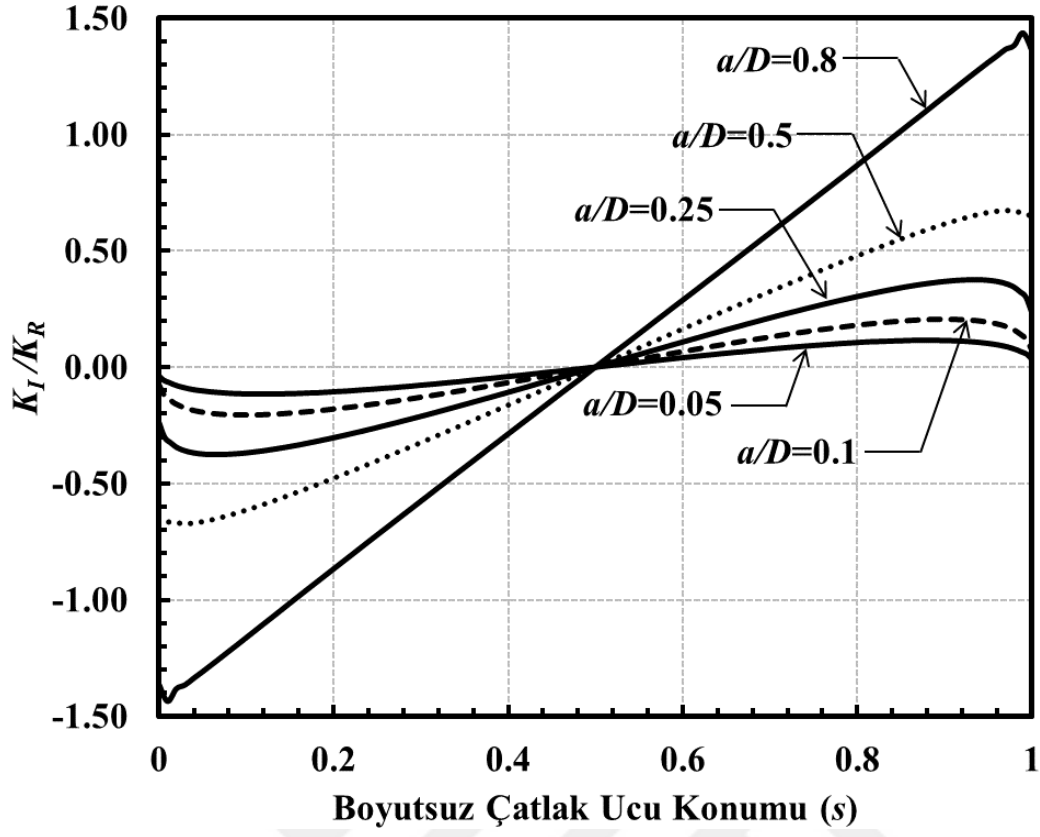
Şekil 3.278. Sabit a/c için çatlak önü boyunca boyutsuz K_I dağılımları (Burulma yükü) ( \alpha=45^\circ , a/c=0.25 ).
