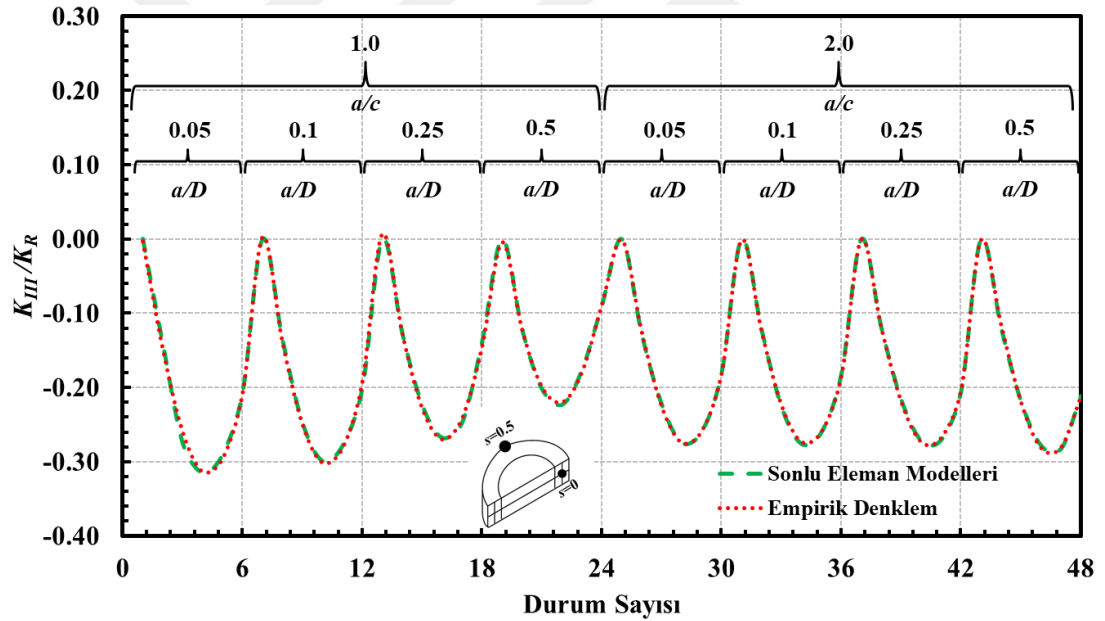
Şekil 4.18. Eğilme yükü altında silindirde bulunan a/c=1.0-2.0 şekil oranlarına sahip dönmüş yüzey çatlağının serbest yüzey noktası için ( s=0 ) boyutsuz K_{III} değerleri ile empirik denklem sonucunun karşılaştırılması.
