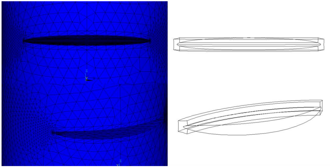
Şekil 3.27. Eksenel gerilme yükü altında yatay düzlem ile 0^\circ açı yapan yüzey çatlağının açılma durumu[25].
