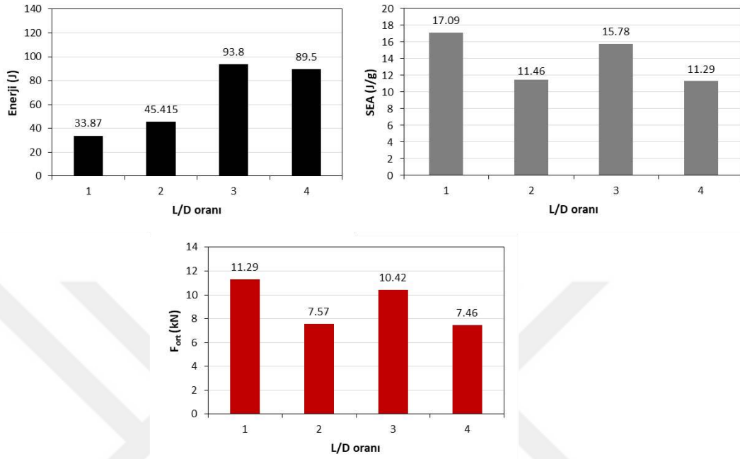
Grafik 7.19. L/D oranına bağlı olarak %25 deformasyon için %10 B_4C takviyeli Al profillerde elde edilen E, F_{ort} ve SEA değerleri
