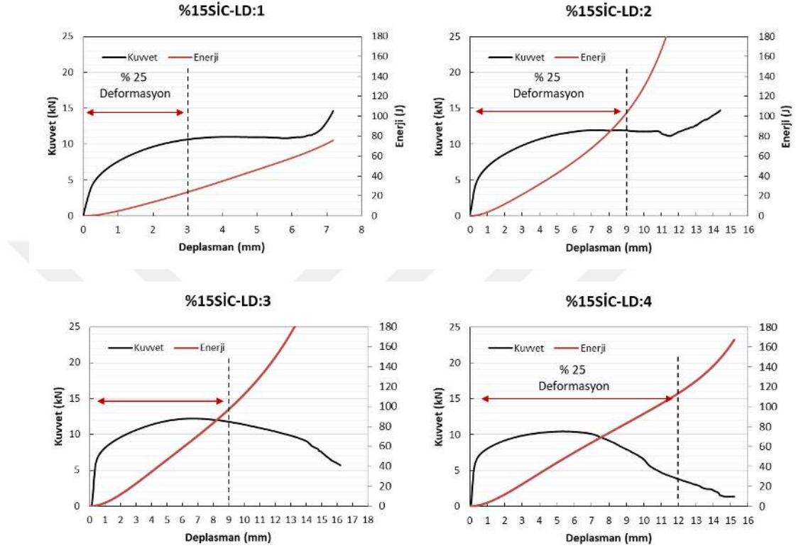
Grafik 7.9. %15 SiC takviyeli alüminyum profillerin yük-deplasman eğrileri
