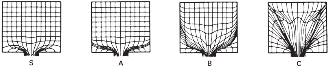
Şekil 3.5. Ekstrüzyonda dört farklı akış türü (Saha, 2000).
