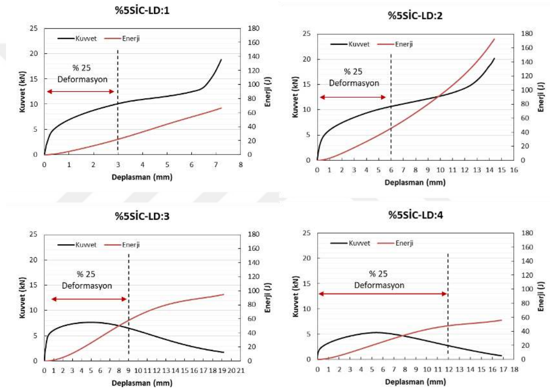
Grafik 7.5. %5 SiC takviyeli alüminyum profillerin yük-deplasman eğrileri
