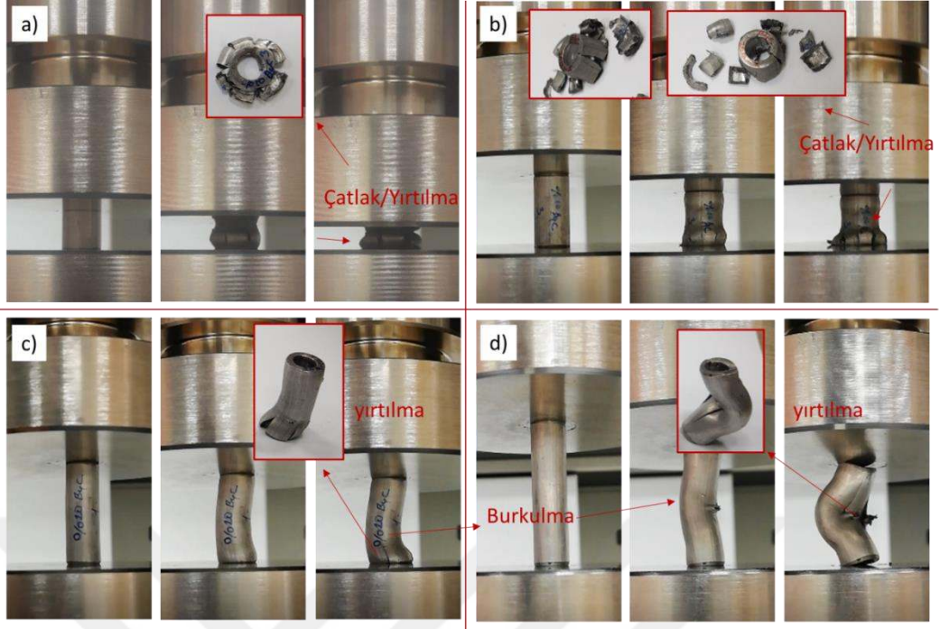
Fotoğraf 7.18. %20 B 4 C takviyeli Al profillerin deformasyon davranışları, a) L/D:1, b) L/D:2, c) L/D:3 ve d) L/D:4
