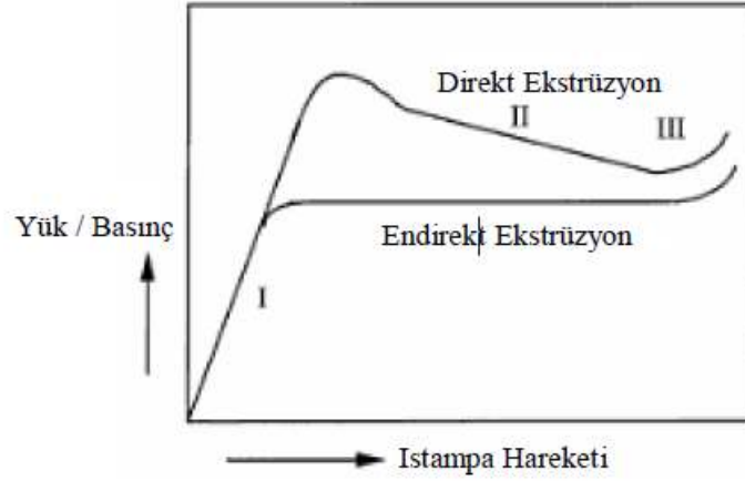
Şekil 3.4. Direkt ve endirekt ekstrüzyon proseslerinde yük veya basıncın istampa hareketiyle değişimi (Saha, 2000).
