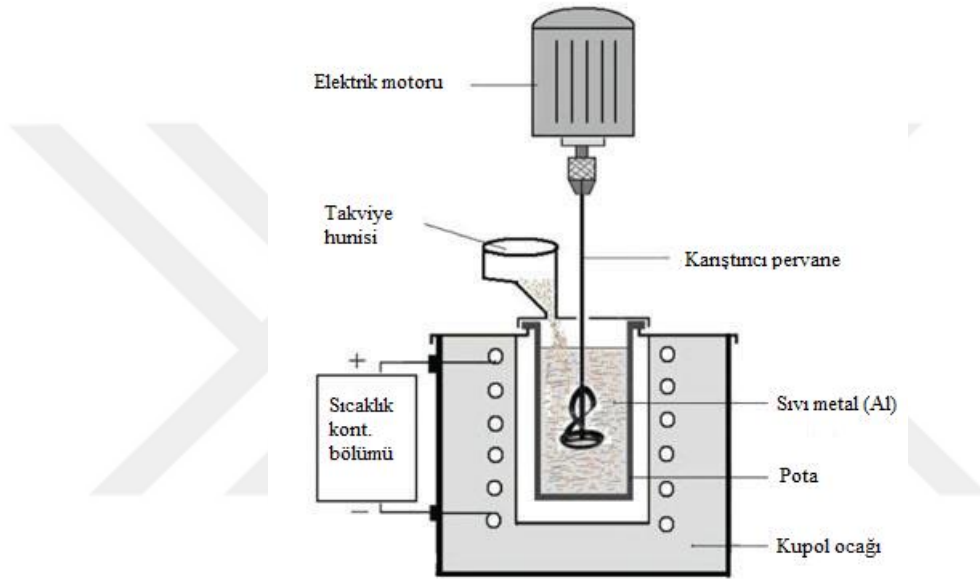
Şekil 2.3. Karıştırırmalı dökümün şematik gösterimi (Calin, Pul ve Pehlivanlı, 2002).
