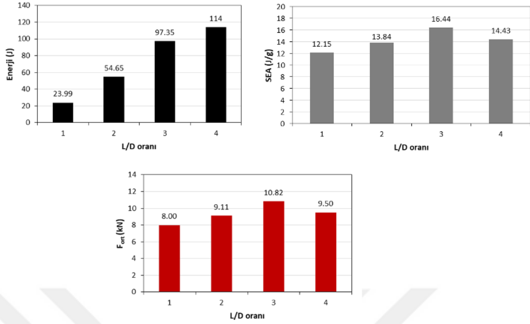
Grafik 7.10. L/D oranına bağlı olarak %25 deformasyon için %15 SiC takviyeli Al profillerde elde edilen E, Fort ve SEA değerler
