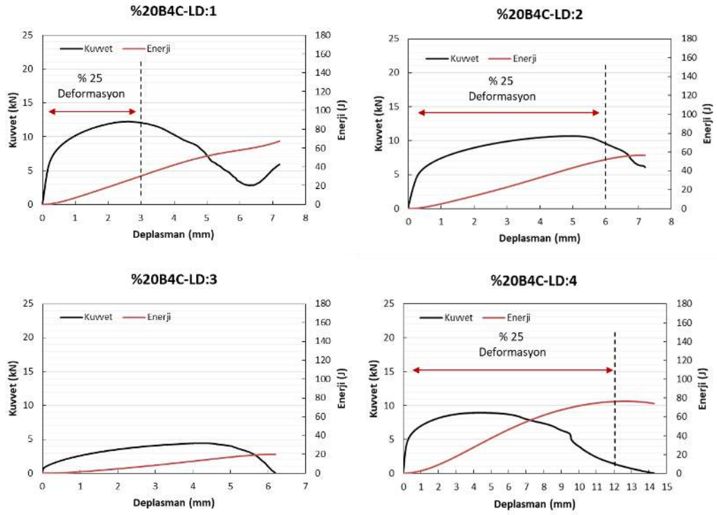
Grafik 7.22. %20 B 4 C takviyeli alüminyum profillerin yük-deplasman eğrileri
