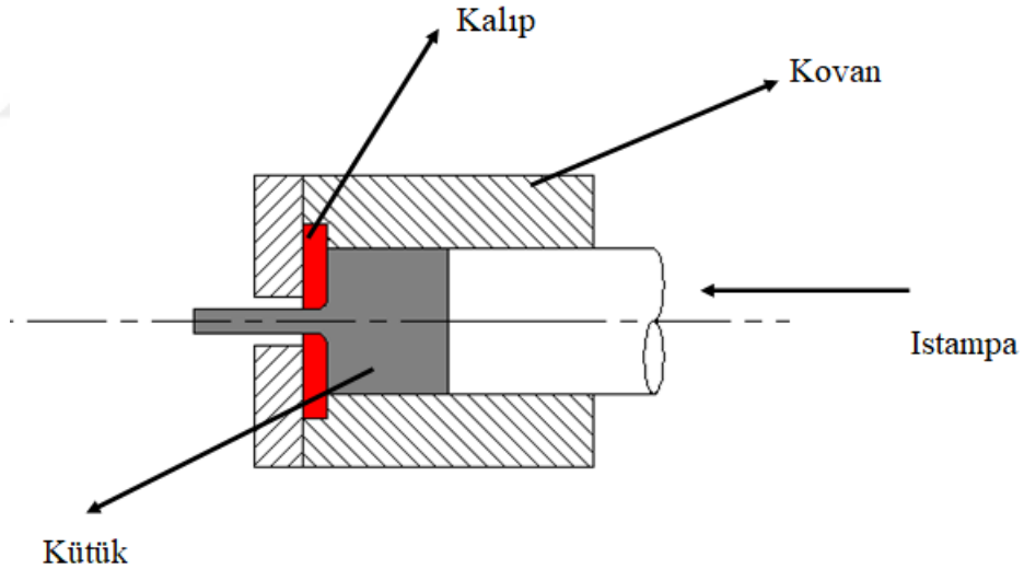
Şekil 3.2. Direkt ekstrüzyon işleminin şematik gösterimi (Kalkan, 2011).
