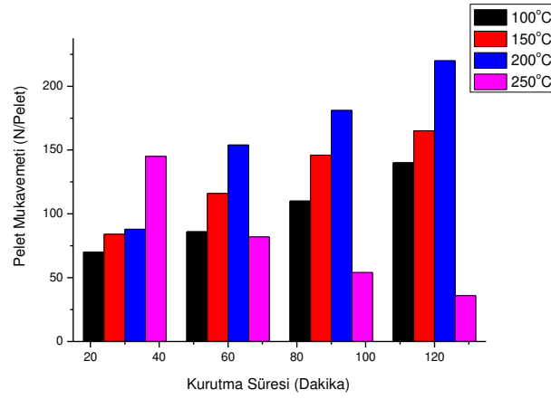
Şekil 6.4. (Melas/Su) oranı (60/100) olacak şekilde hazırlanan melas çözeltisinden toplam malzemenin %5'i kadar alınıp püskürtülerek üretilen peletlerin kurutma sıcaklığı ve süresine bağlı olarak kuru mukavemet değerlerindeki değişim.
