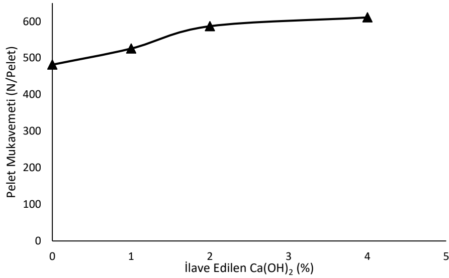
Şekil 6.8. İlave edilen \text{Ca(OH)}_2 oranına göre değişen mukavemet değerleri ((Melas/Su=0,6, Kok/ \Sigma Malzeme =0,2, T=200°C, t=120 dakika, Hazırlanan melas çözeltisinden toplam malzemenin %10'ı kadar alınıp püskürtülerek üretilen peletler)
