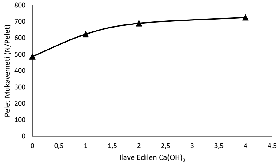
Şekil 6.14. % 2 CMC, %20 kok ve farklı oranlarda \text{Ca(OH)}_2 ilave edilerek üretilen peletlerin kuru mukavemet değerlerindeki değişim.
