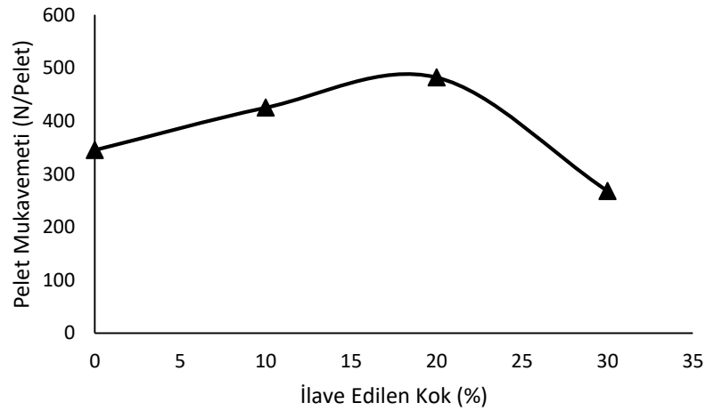
Şekil 6.7. Konsantre içerisine farklı oranlarda ilave edilen kok kömürünün pelet mukavemetine etkisi ((Melas/Su=0,6) olacak şekilde hazırlanan melas çözeltisinden toplam malzemenin %10'ı kadar alınıp püskürtülerek üretilen peletler T=200°C, t=120 dakika)
