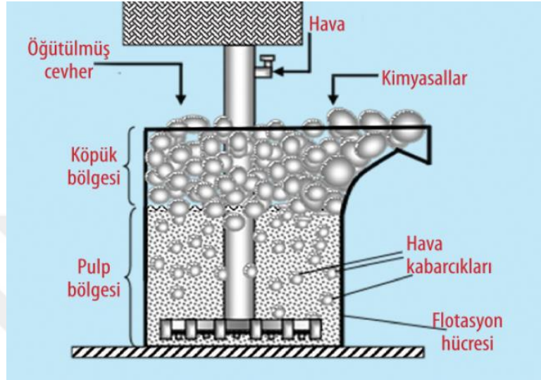
Şekil 2.6. Flotasyon hücresi
