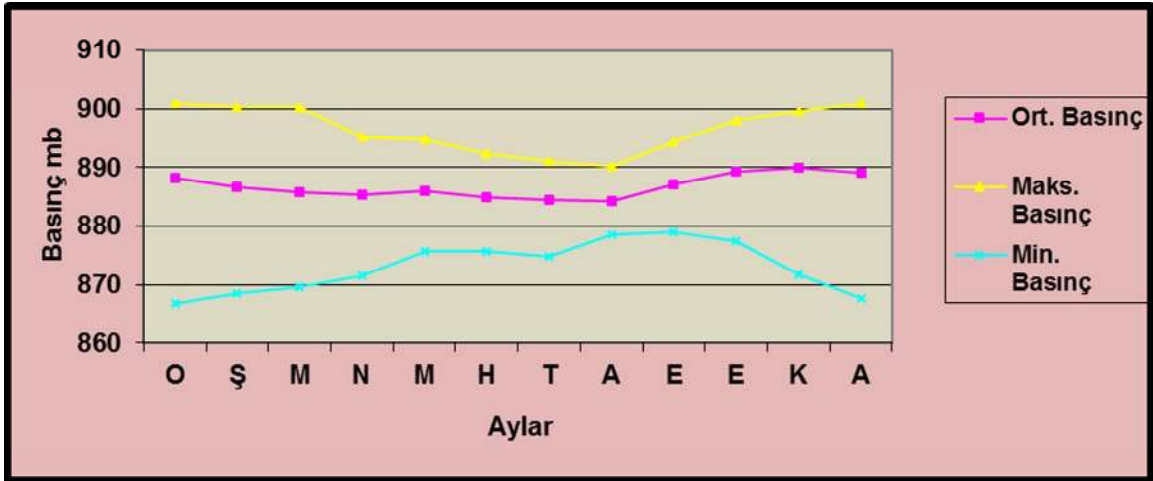
Grafik 9. Elbistan'da maksimum, ortalama ve minimum basınçların yıl içerisindeki durumu (1970-2011).
