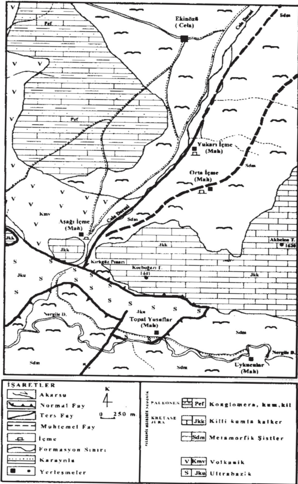
Şekil 26. Ekinözü içmeleri jeoloji haritası (Gökalp, 1972; Ölmez, 1977 ve Gürbüz ve Sandal, 2003'ten alınmıştır).
