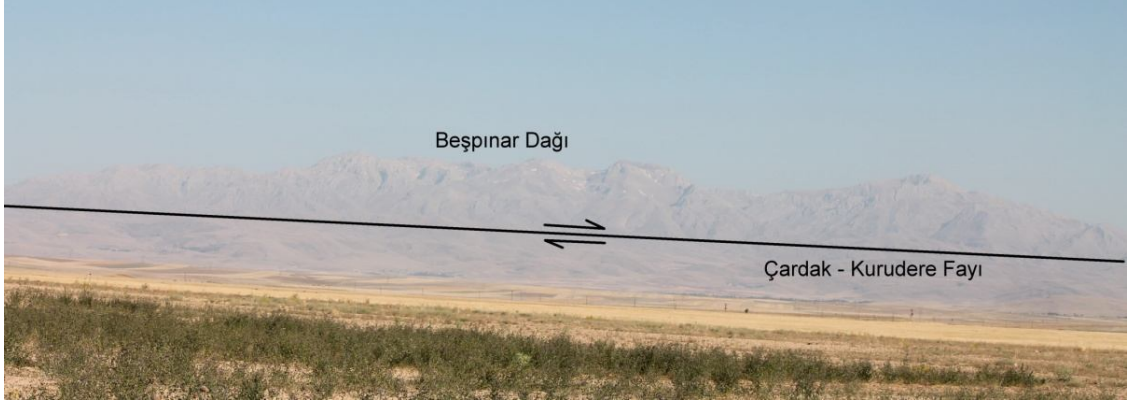
Foto 10. Elbistan Havzası'nın kuzeyindeki ploto sahasının oluşumunda etkili olan Çardak-Kurudere Fayı (Yeniköy güneyinden batıya bakış).
