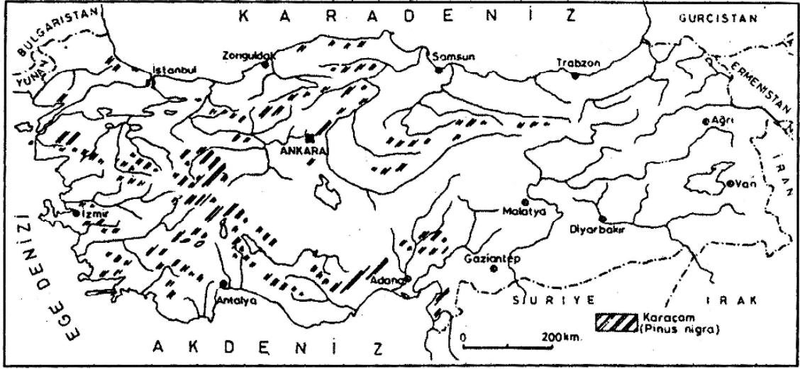
Şekil 36. Türkiye’de karaçam ormanlarının yayılış alanları (Atalay, 2008).
