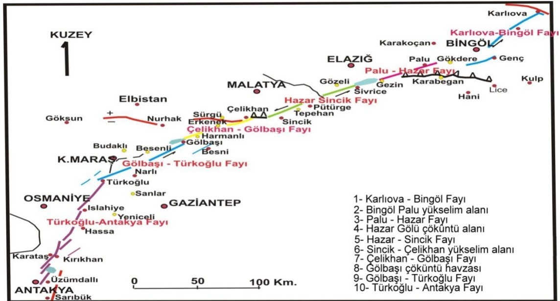
Karlıova ile Antakya Arasında Uzanan Doğu Anadolu Fayının Bölümleri
