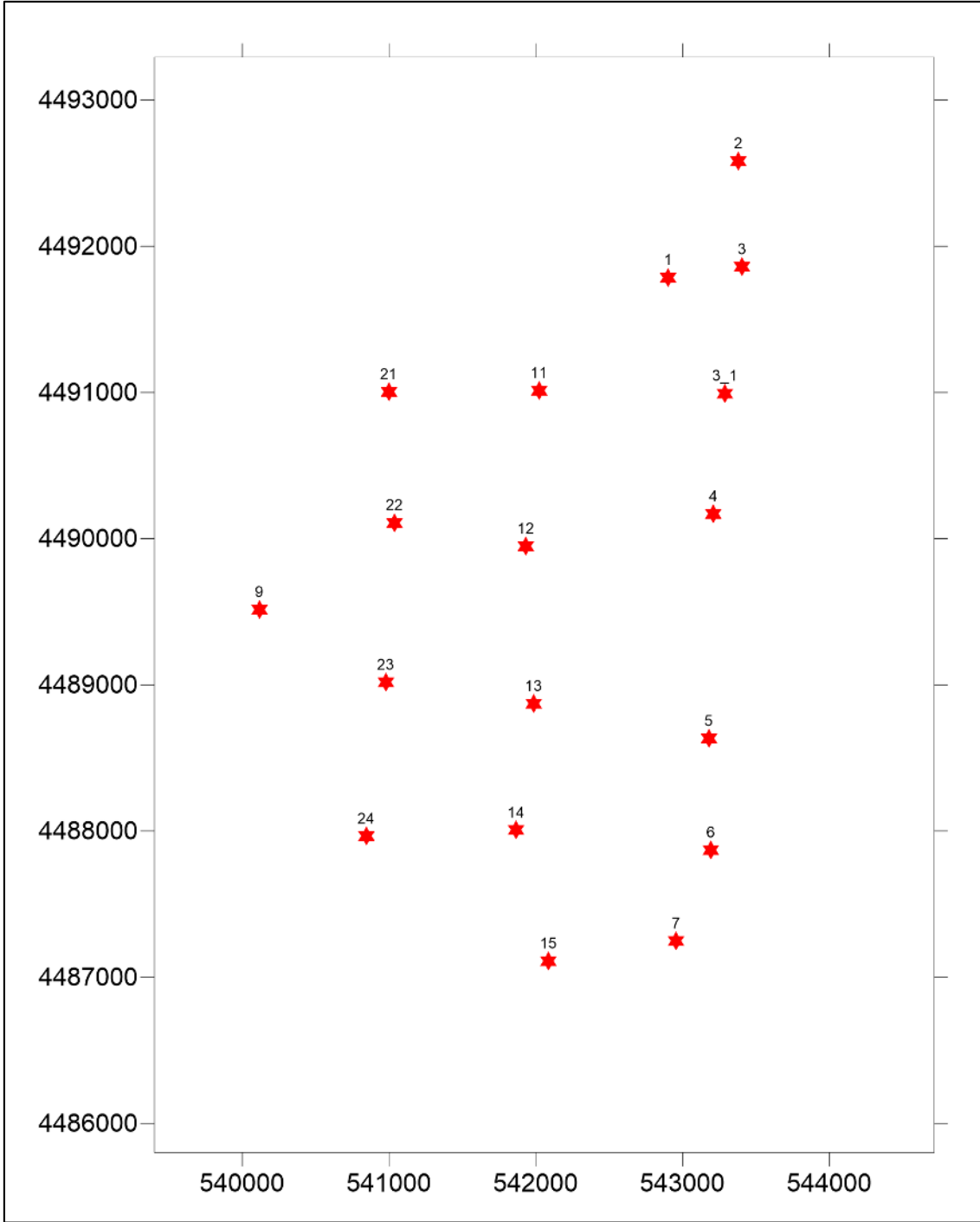
Şekil 3.2. Düşey elektrik sondajlarının lokasyonları
