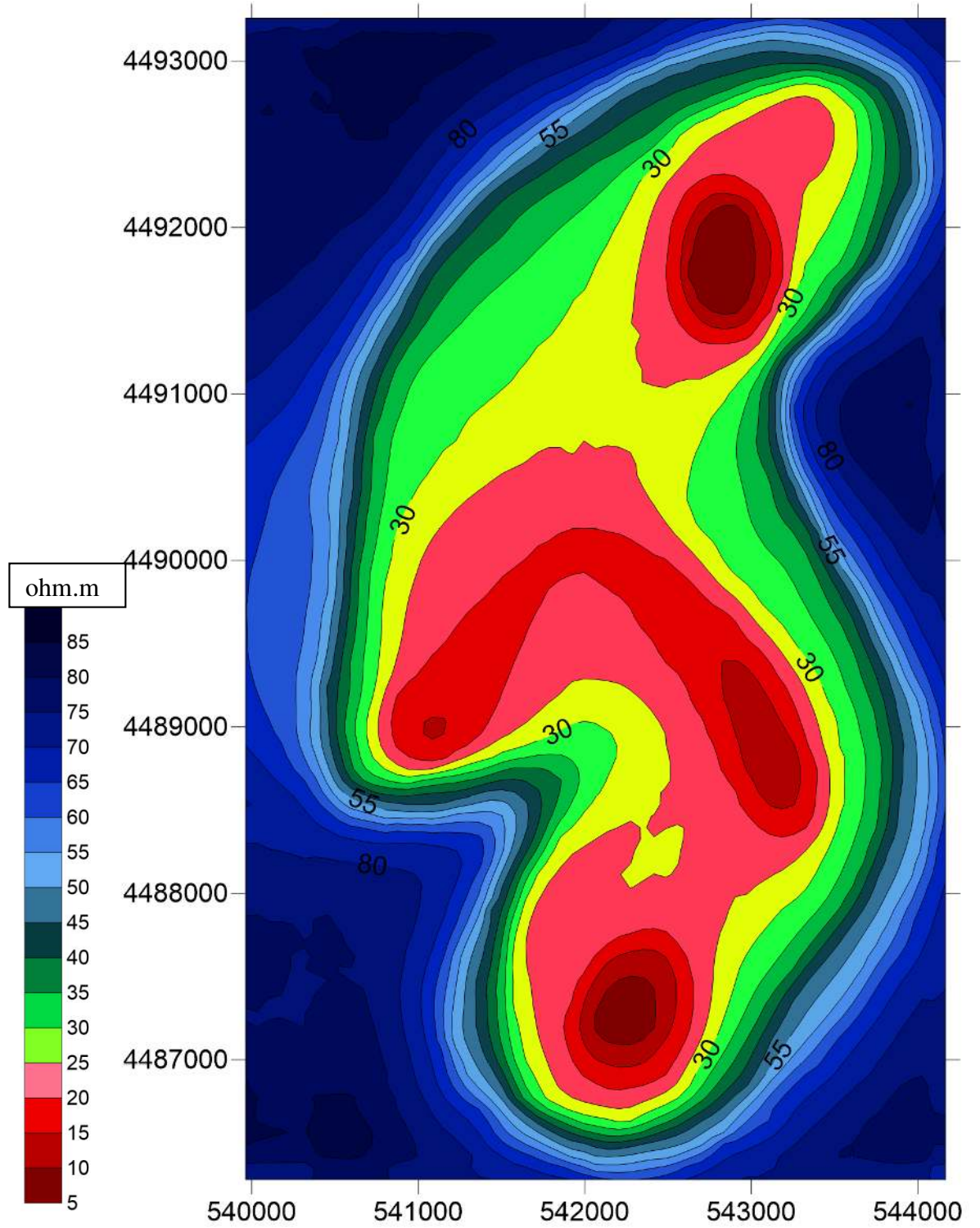
Şekil 4.20. 400 metre derinlikli eş rezistivite haritası
