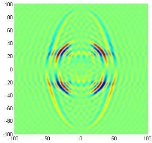
(b) H_3^3(x_1, 0, x_3, 6/c)
