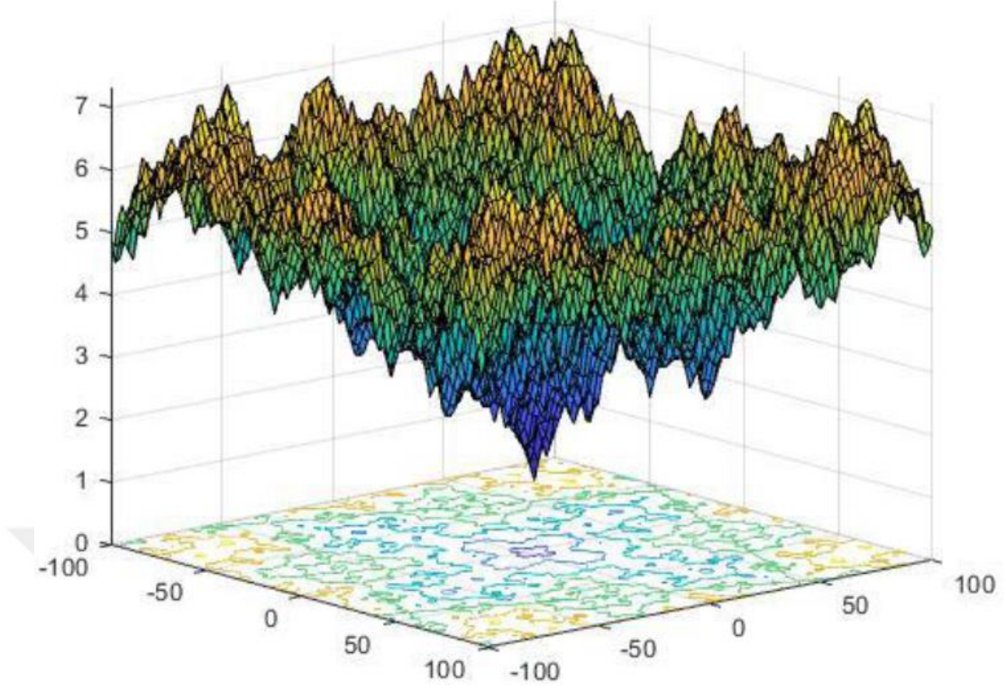
Şekil 4.7. Weierstrass fonksiyonunun 2 boyut için grafiğidir.
