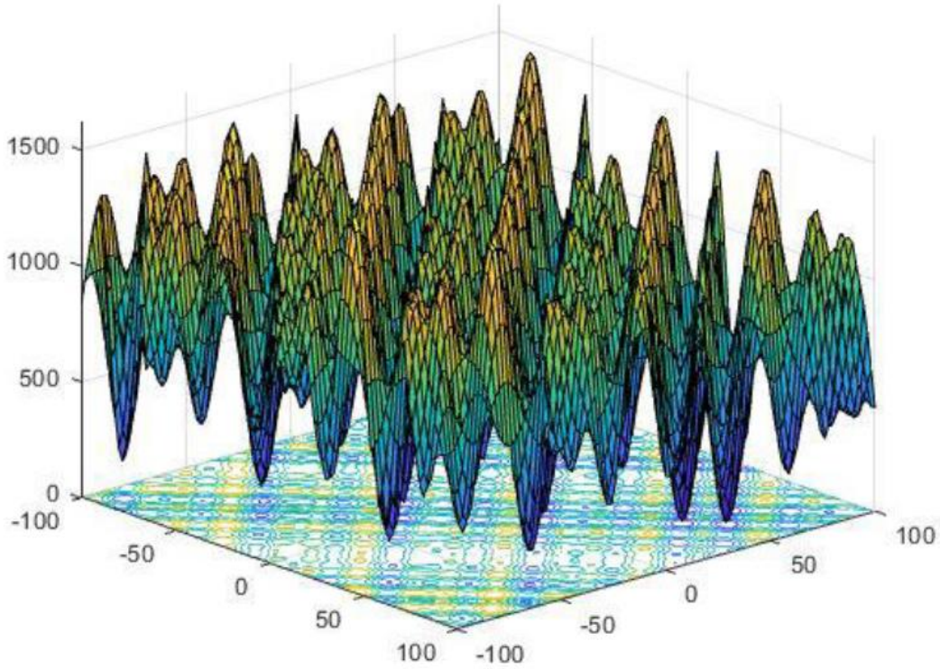
Şekil 4.8. Değiştirilmiş Schwefel fonksiyonunun 2 boyut için grafiğidir.
