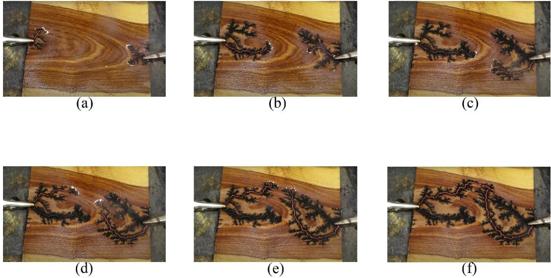
Şekil 3.2. Yüksek voltajlı elektrik kullanılarak ahşap üzerinde oluşturulan Lichtenberg figürü yanık izleridir.
