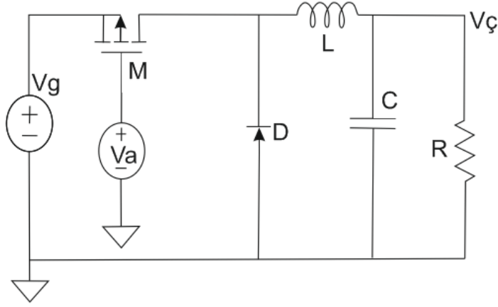
Şekil 2.1. Anahtarlamaalı Voltaj Düşürücü Devre [80'den değiştirilmiştir]
