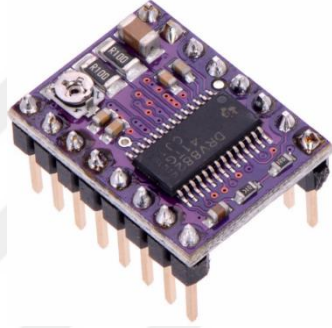
 ekil 2.11. DRV8825 Mikro Adım S r c  [88]
