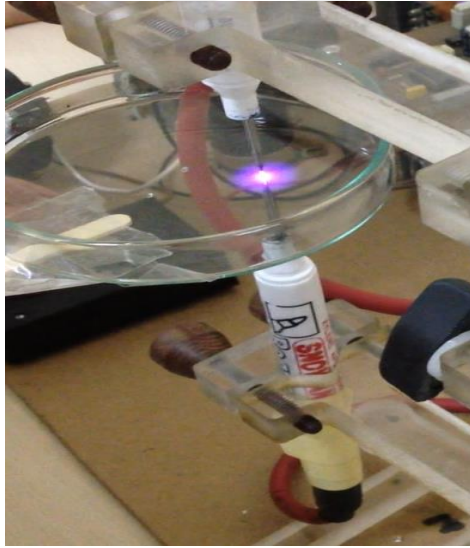
Şekil 3.12. Analog Kontrol Sistemi Cam Delme Çalışması
