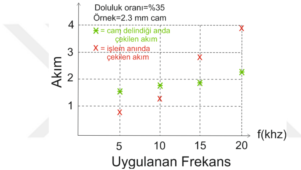
Şekil 3.20. Uygulanan Frekans ve Çekilen Akım İlişkisi
