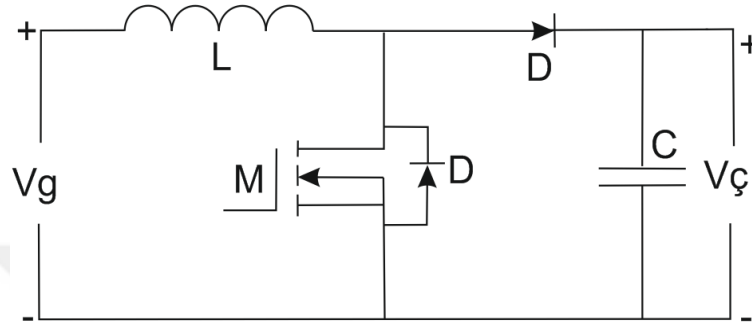
Şekil 2.3. İzolasyonsuz Anahtarlama Yükseltici Devre [82'den değiştirilmiştir]
