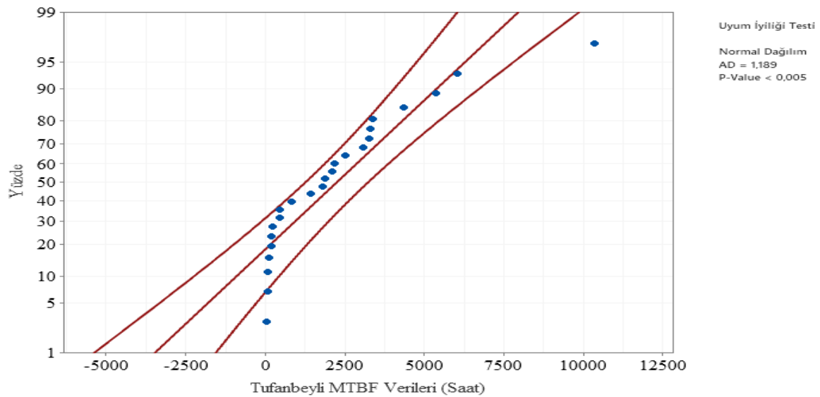
Şekil 6.10. Tufanbeyli Fideri normal dağılım Anderson- Darling uyumluluk eğrisi
