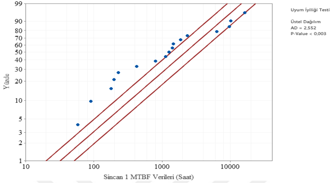
Şekil 6.43. Sincan 1 Fideri üstel dağılım Anderson- Darling uyumluluk eğrisi
