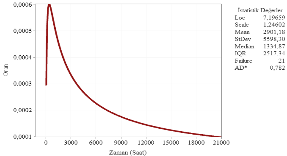
Şekil 6.127. Elbistan fideri tehlike fonksiyonu eğrisi
