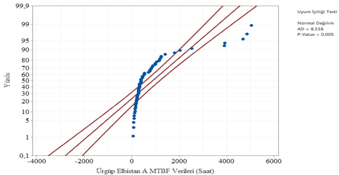
Şekil 6.34. Elbistan A Fideri normal dağılım Anderson- Darling uyumluluk eğrisi
