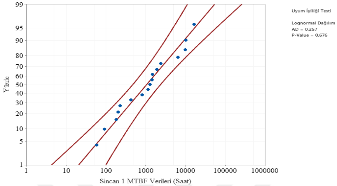
Şekil 6.45. Sincan 1 Fideri lognormal dağılımı Anderson- Darling uyumluluk eğrisi
