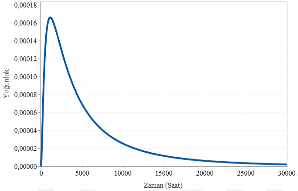
Şekil 6.116. Gölbaşı Kuzey fideri olasılık yoğunluk fonksiyonu eğrisi
