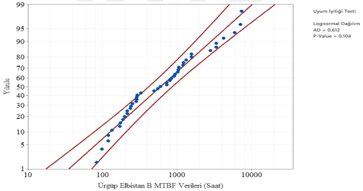
Şekil 6.41. Elbistan B Fideri lognormal dağılımı Anderson- Darling uyumluluk eğrisi
