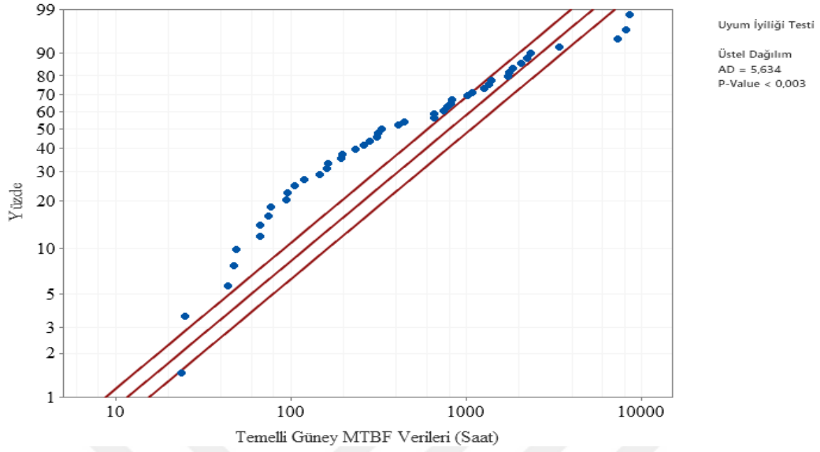
Şekil 6.27. Temelli Güney Fideri üstel dağılım Anderson- Darling uyumluluk eğrisi
