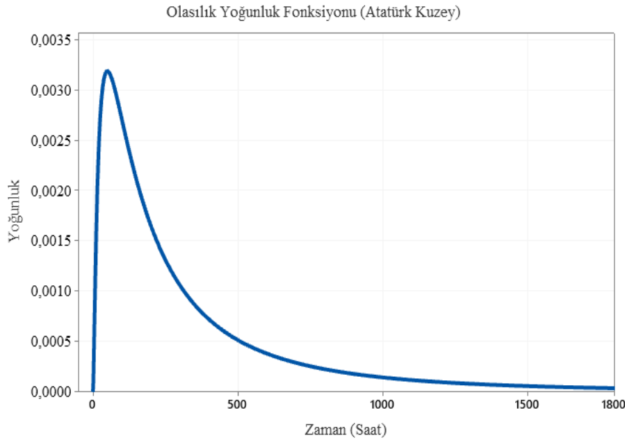
Şekil 6.83. Atatürk Kuzey fideri olasılık yoğunluk fonksiyonu eğrisi
