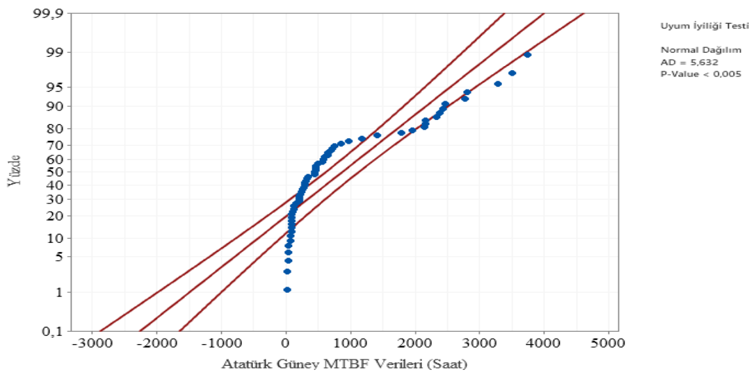
Şekil 6.2. Atatürk Güney Fideri normal dağılım Anderson- Darling uyumluluk eğrisi
