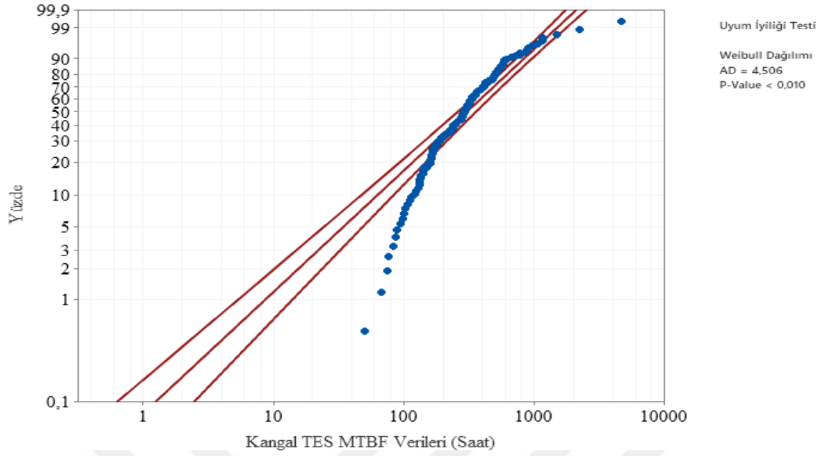
Şekil 6.72. Kangal TES Fideri weibull dağılımı Anderson- Darling uyumluluk eğrisi
