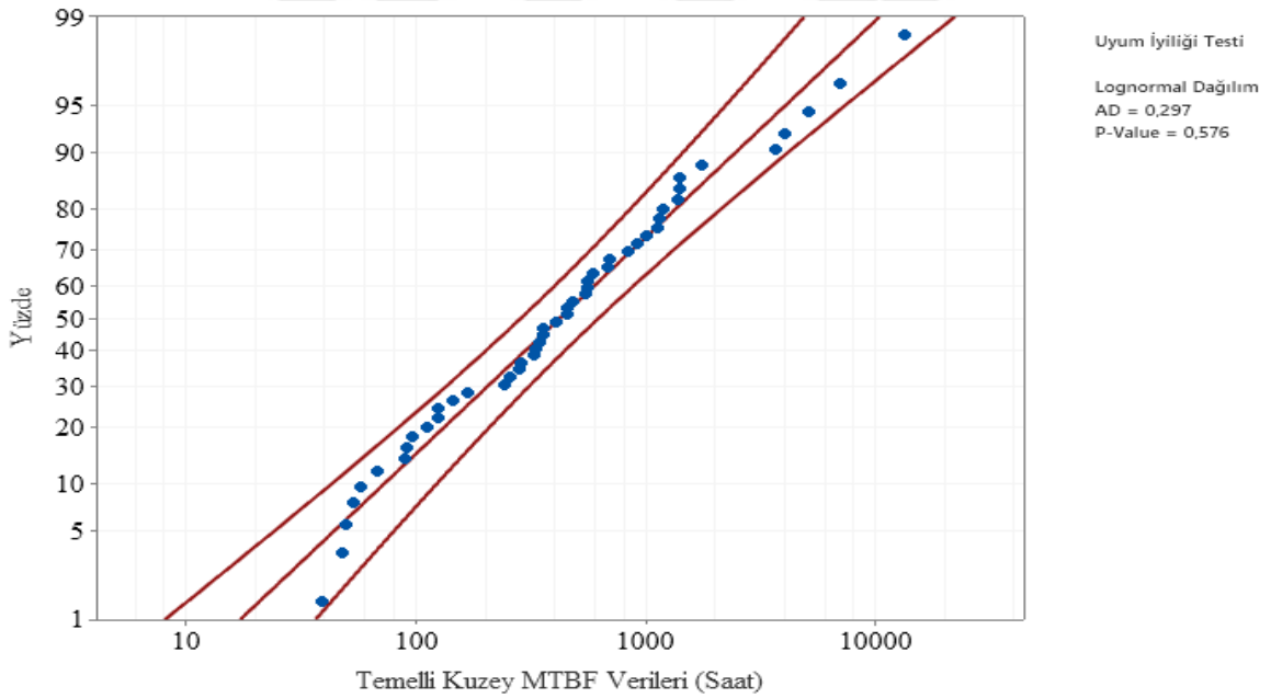
Şekil 6.33. Temelli Kuzey Fideri lognormal dağılımı Anderson- Darling uyumluluk eğrisi
