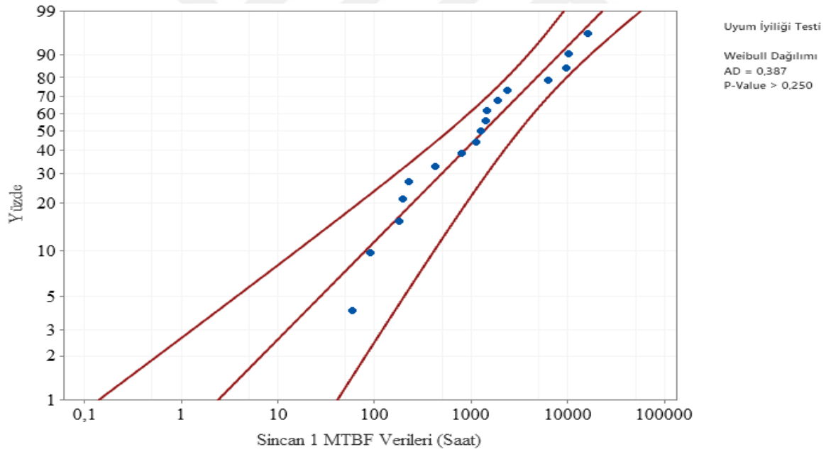
Şekil 6.44. Sincan 1 Fideri weibull dağılımı Anderson- Darling uyumluluk eğrisi
