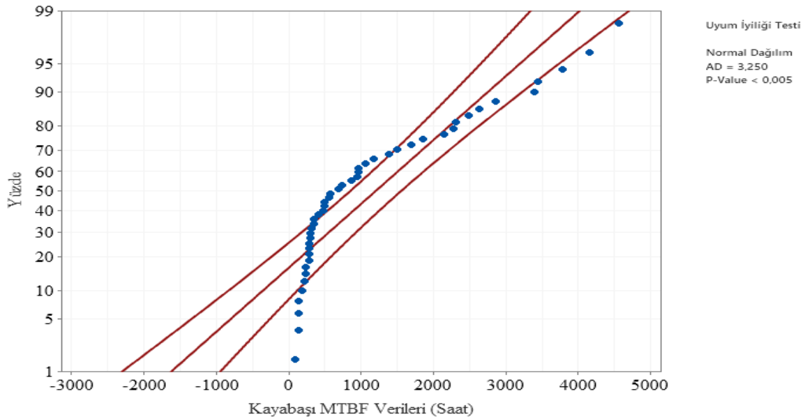
Şekil 6.74. Kayabaşı Fideri normal dağılım Anderson- Darling uyumluluk eğrisi
