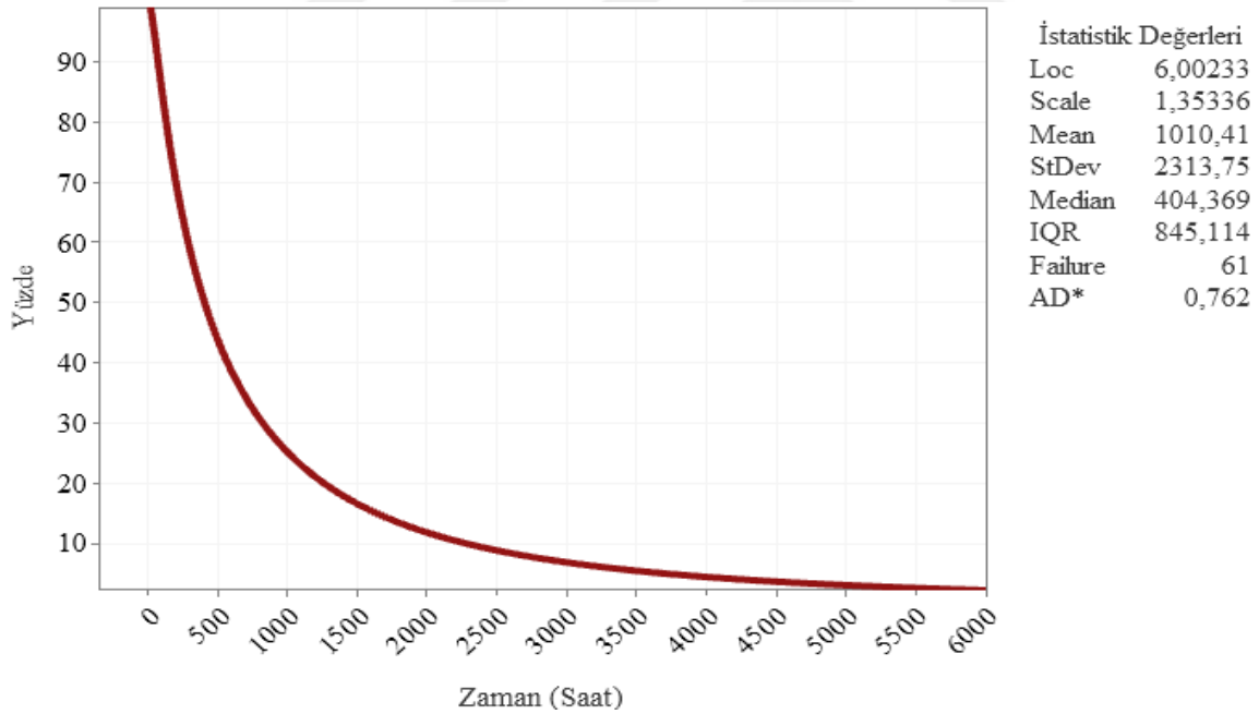
Şekil 6.78. Atatürk Güney fideri güvenilirlik fonksiyonu eğrisi
