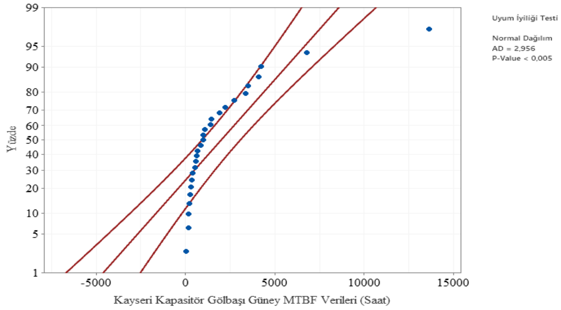
Şekil 6.54. Gölbaşı Güney Fideri normal dağılım Anderson- Darling uyumluluk eğrisi
