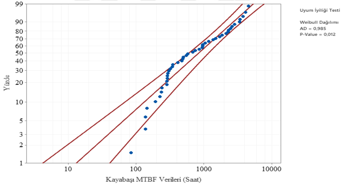
Şekil 6.76. Kayabaşı Fideri weibull dağılımı Anderson- Darling uyumluluk eğrisi
