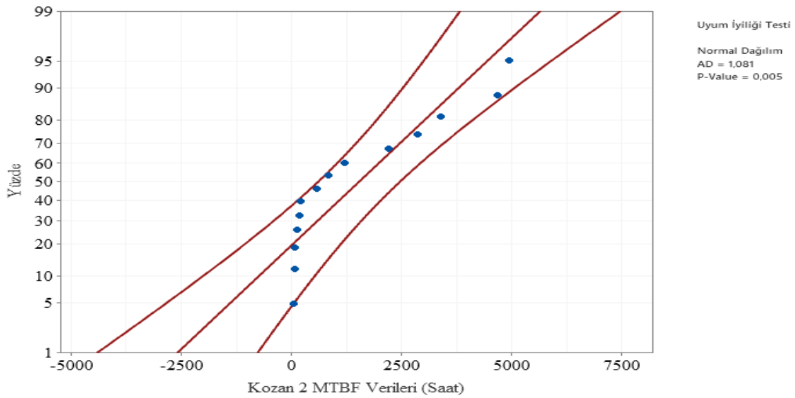
Şekil 6.18. Kozan 2 Fideri normal dağılım Anderson- Darling uyumluluk eğrisi
