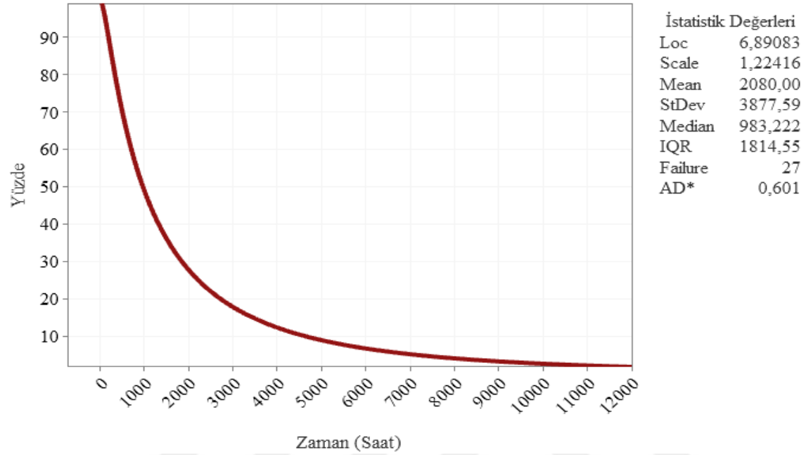
Şekil 6.117. Gölbaşı Güney fideri güvenilirlik fonksiyonu eğrisi
