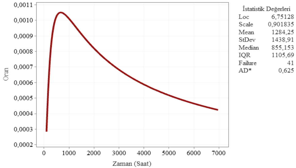
Şekil 6.124. Keban Kuzey fideri tehlike fonksiyonu eğrisi
