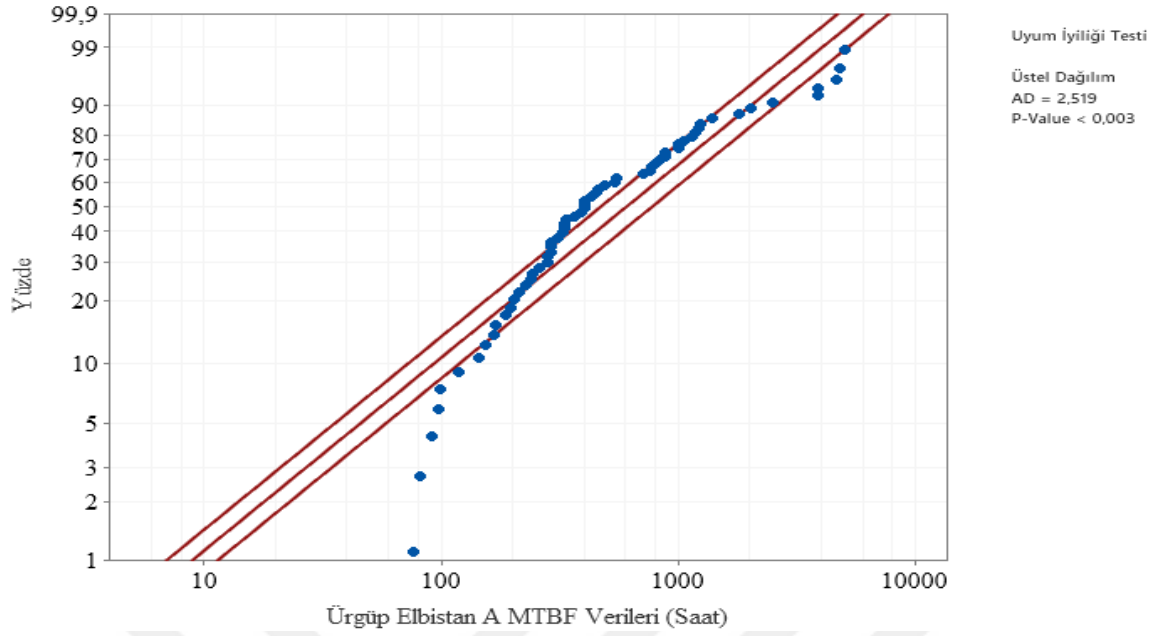
Şekil 6.35. Elbistan A Fideri üstel dağılım Anderson- Darling uyumluluk eğrisi
