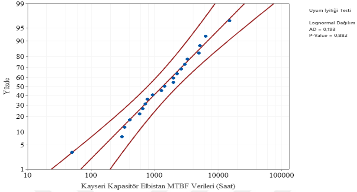
Şekil 6.69. Elbistan Fideri lognormal dağılımı Anderson- Darling uyumluluk eğrisi
