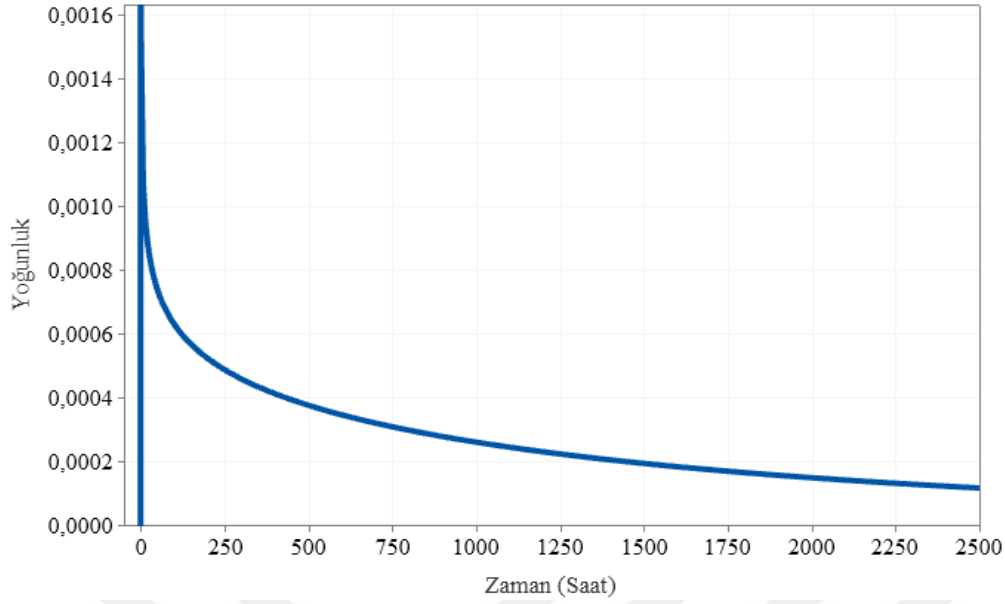
Şekil 6.86. Tufanbeyli fideri olasılık yoğunluk fonksiyonu eğrisi
