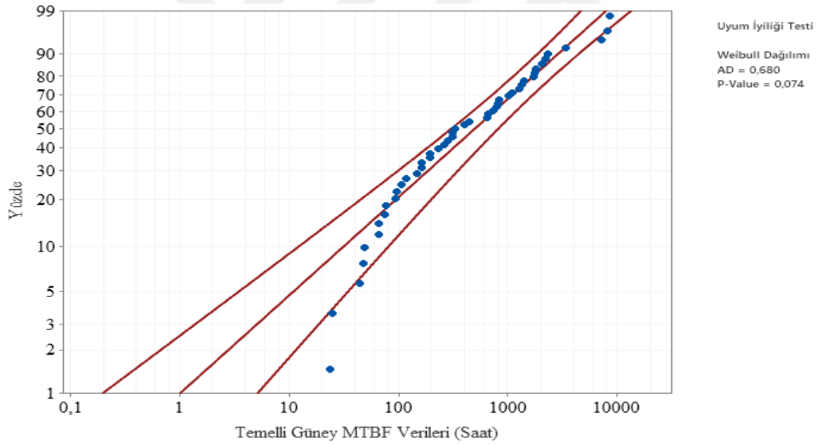
Şekil 6.28. Temelli Güney Fideri weibull dağılımı Anderson- Darling uyumluluk eğrisi
