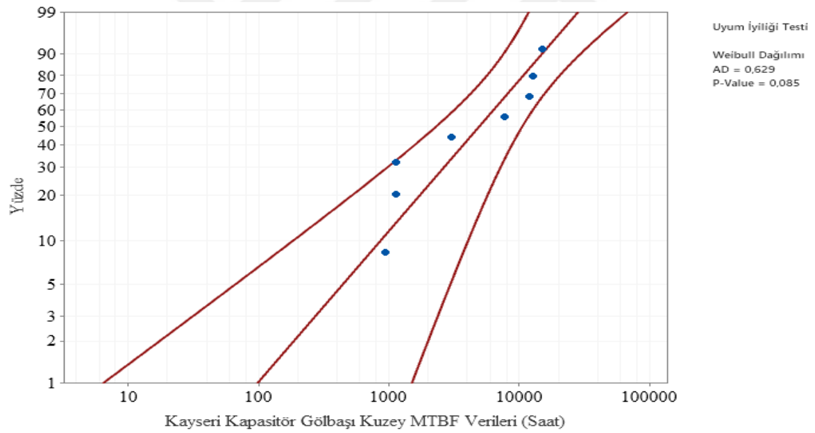
Şekil 6.52. Gölbaşı Kuzey Fideri weibull dağılımı Anderson- Darling uyumluluk eğrisi
