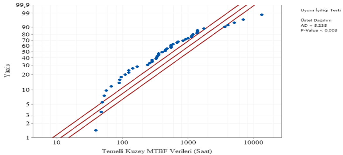
Şekil 6.31. Temelli Kuzey Fideri üstel dağılım Anderson- Darling uyumluluk eğrisi
