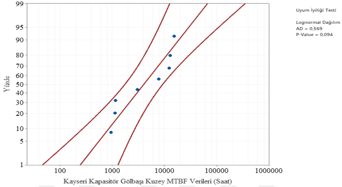
Şekil 6.53. Gölbaşı Kuzey Fideri lognormal dağılımı Anderson- Darling uyumluluk eğrisi
