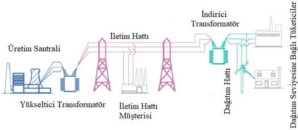
Şekil 6.1. Elektrik üretim, iletim ve dağıtım şematik gösterimi
