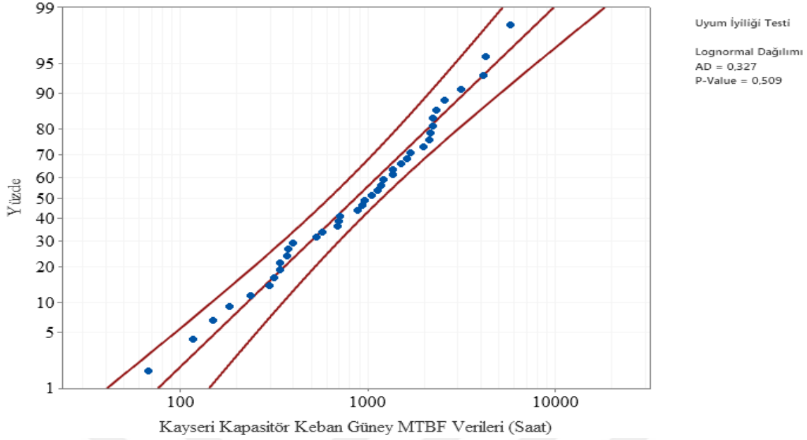
Şekil 6.61. Keban Güney Fideri lognormal dağılımı Anderson- Darling uyumluluk eğrisi
