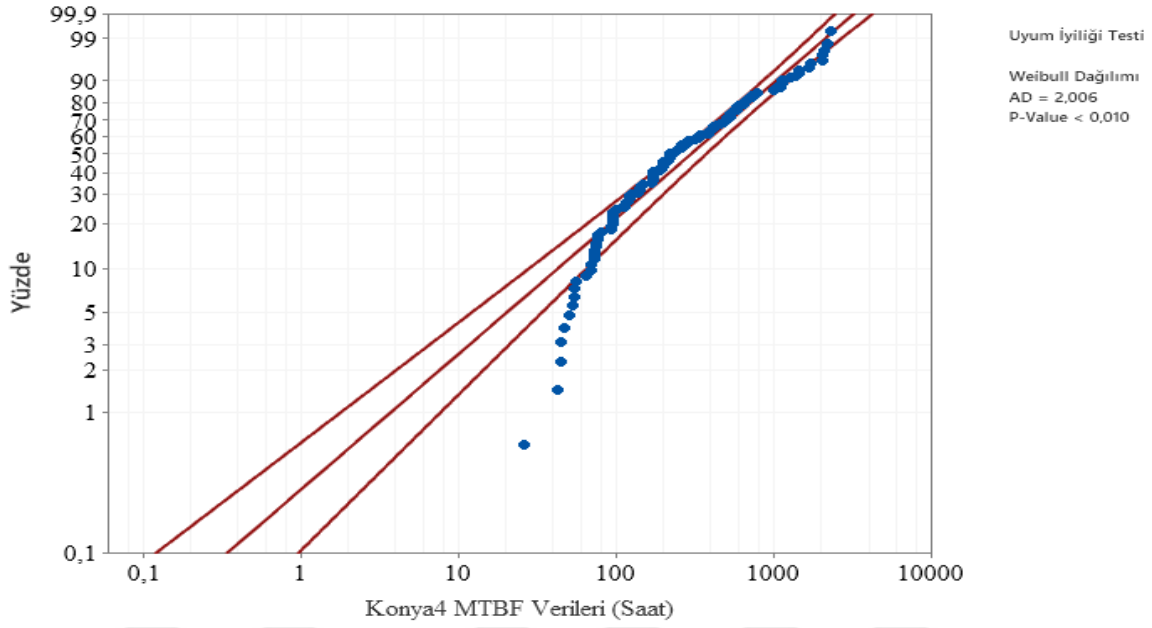
Şekil 6.24. Konya4 Fideri weibull dağılımı Anderson- Darling uyumluluk eğrisi
