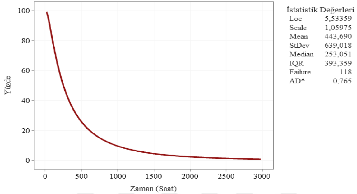
Şekil 6.93. Konya4 fideri güvenilirlik fonksiyonu eğrisi
