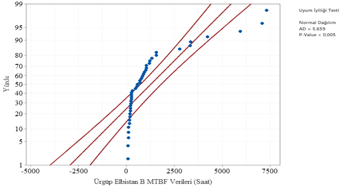
Şekil 6.38. Elbistan B Fideri normal dağılım Anderson- Darling uyumluluk eğrisi
