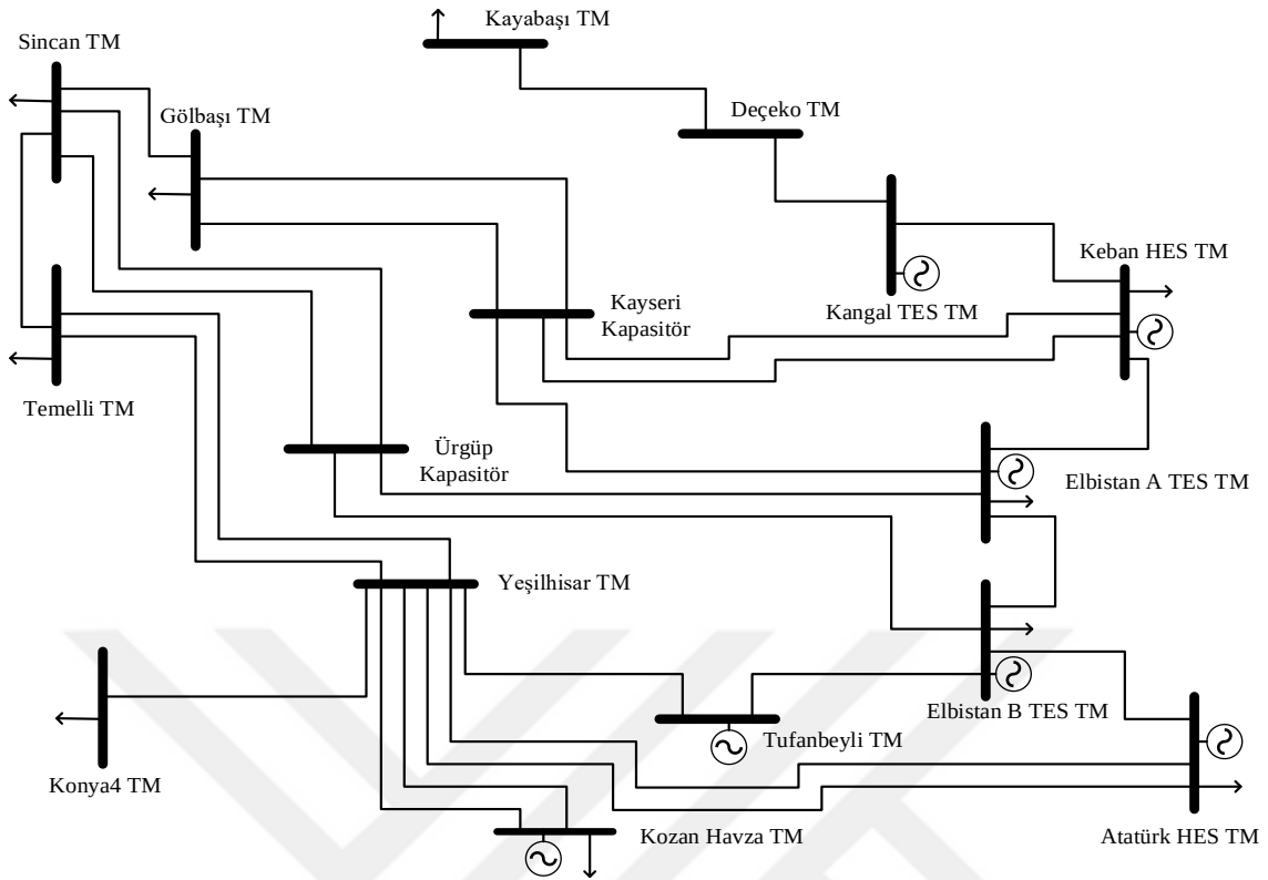
Şekil 6.135. TEİAŞ Kayseri 11. Bölge 380 kV hat şeması
