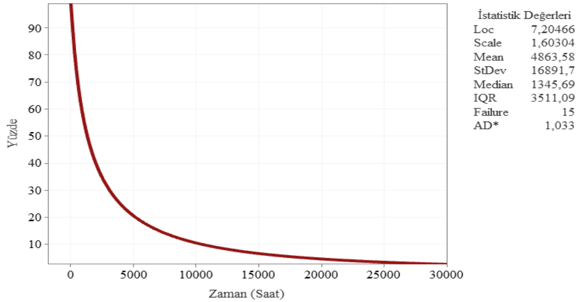
Şekil 6.111. Sincan 2 fideri güvenilirlik fonksiyonu eğrisi
