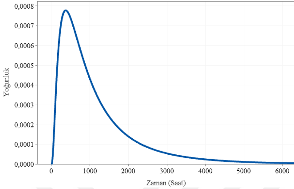
Şekil 6.125. Keban Kuzey fideri olasılık yoğunluk fonksiyonu eğrisi
