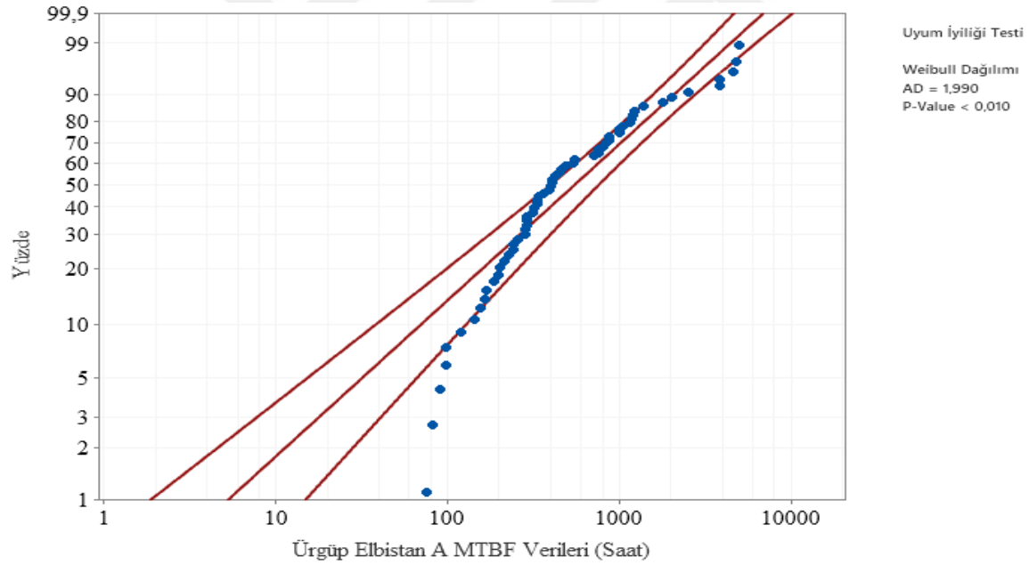
Şekil 6.36. Elbistan A Fideri weibull dağılımı Anderson- Darling uyumluluk eğrisi
