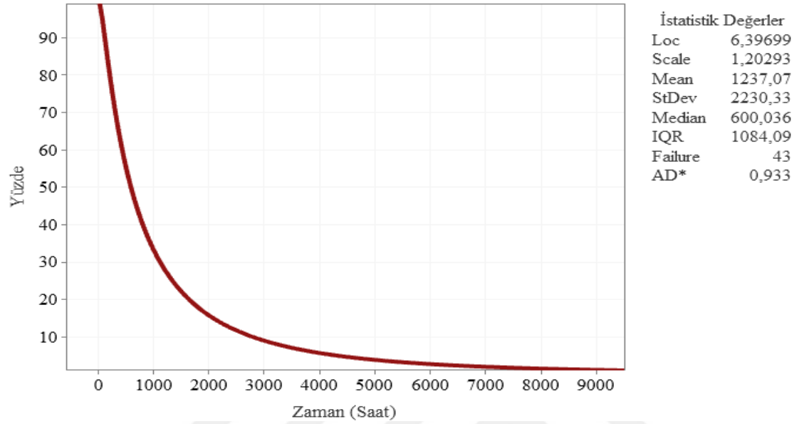
Şekil 6.105. Elbistan B fideri güvenilirlik fonksiyonu eğrisi
