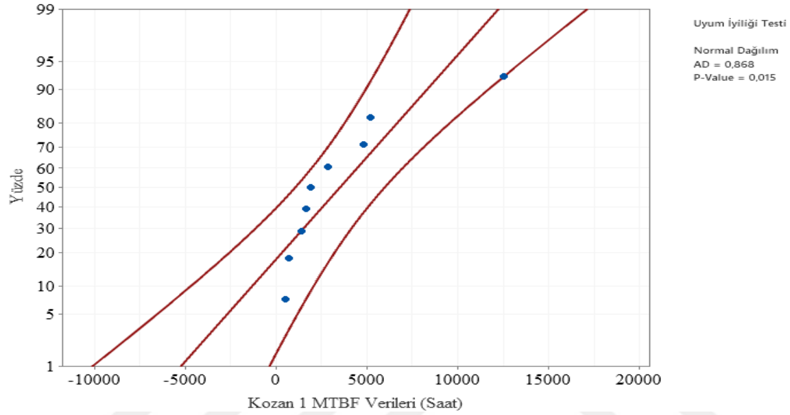
Şekil 6.14. Kozan 1 Fideri normal dağılım Anderson- Darling uyumluluk eğrisi
