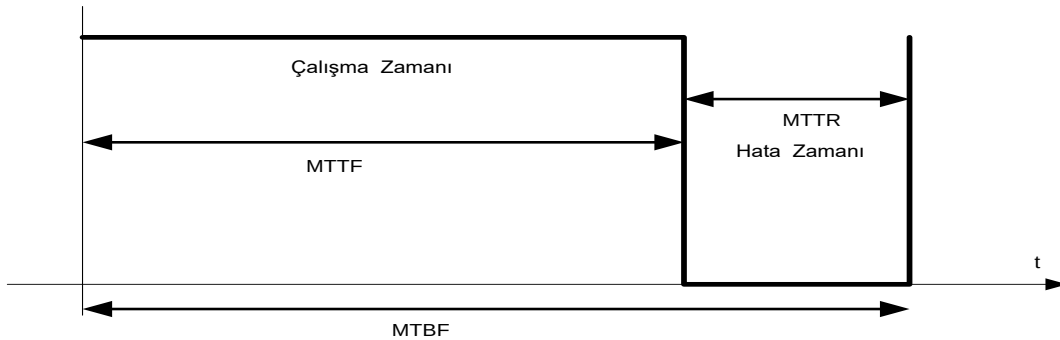
Şekil 2.3. MTTF, MTTR ve MTBF'nin vektörel gösterimi
