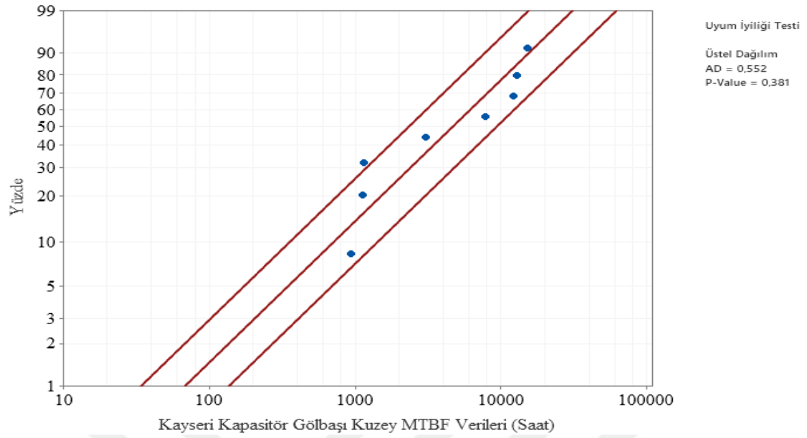
Şekil 6.51. Gölbaşı Kuzey Fideri üstel dağılım Anderson- Darling uyumluluk eğrisi
