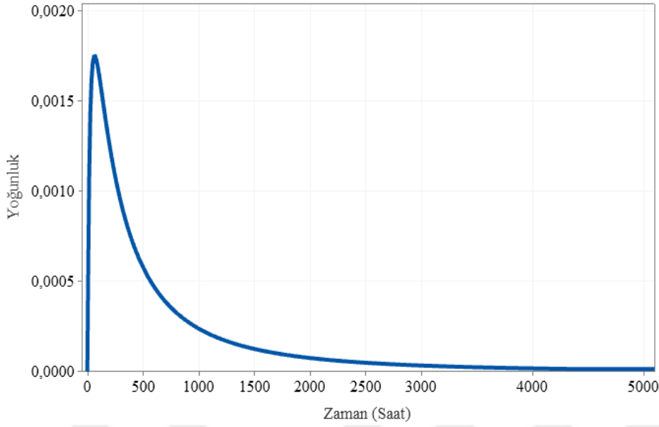
Şekil 6.101. Temelli Kuzey fideri olasılık yoğunluk fonksiyonu eğrisi
