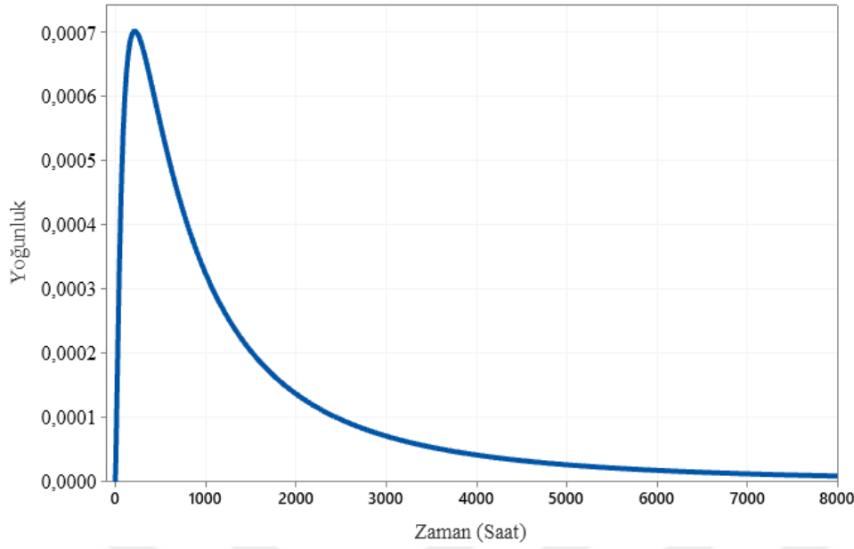
Şekil 6.119. Gölbaşı Güney fideri olasılık yoğunluk fonksiyonu eğrisi
