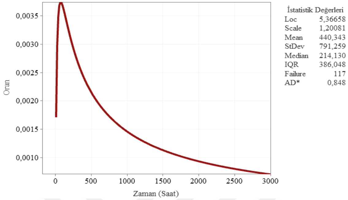
Şekil 6.82. Atatürk Kuzey fideri tehlike fonksiyonu eğrisi
