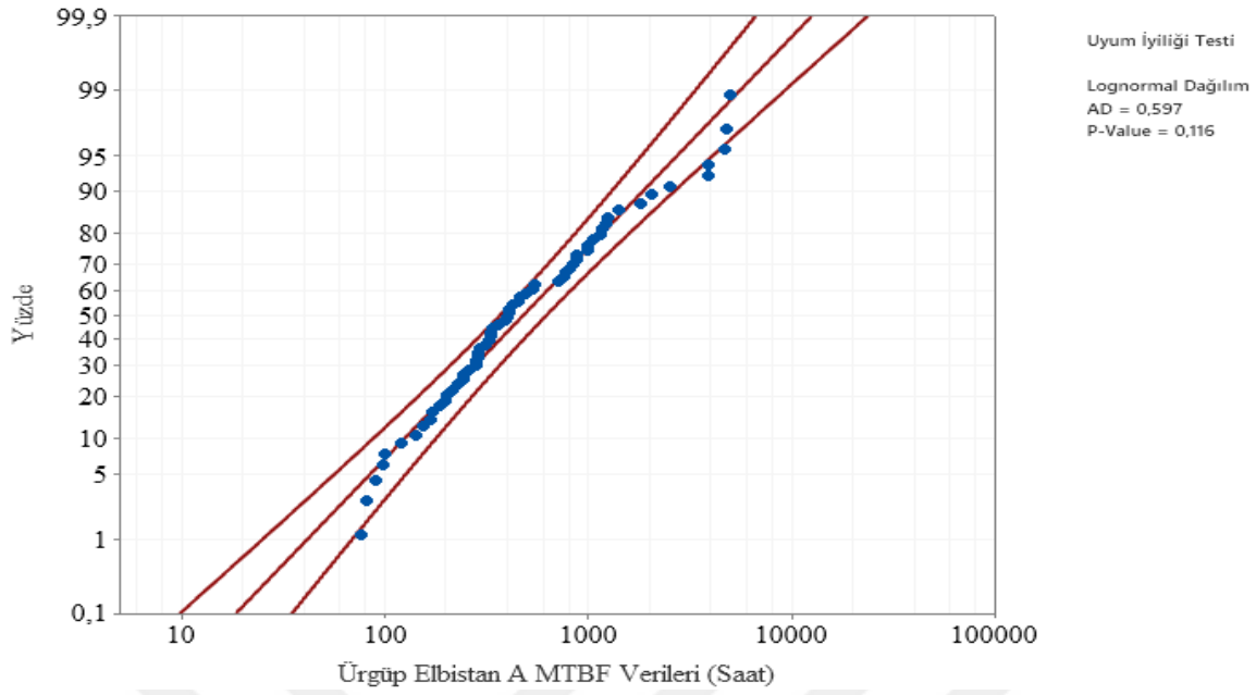
Şekil 6.37. Elbistan A Fideri lognormal dağılımı Anderson- Darling uyumluluk eğrisi
