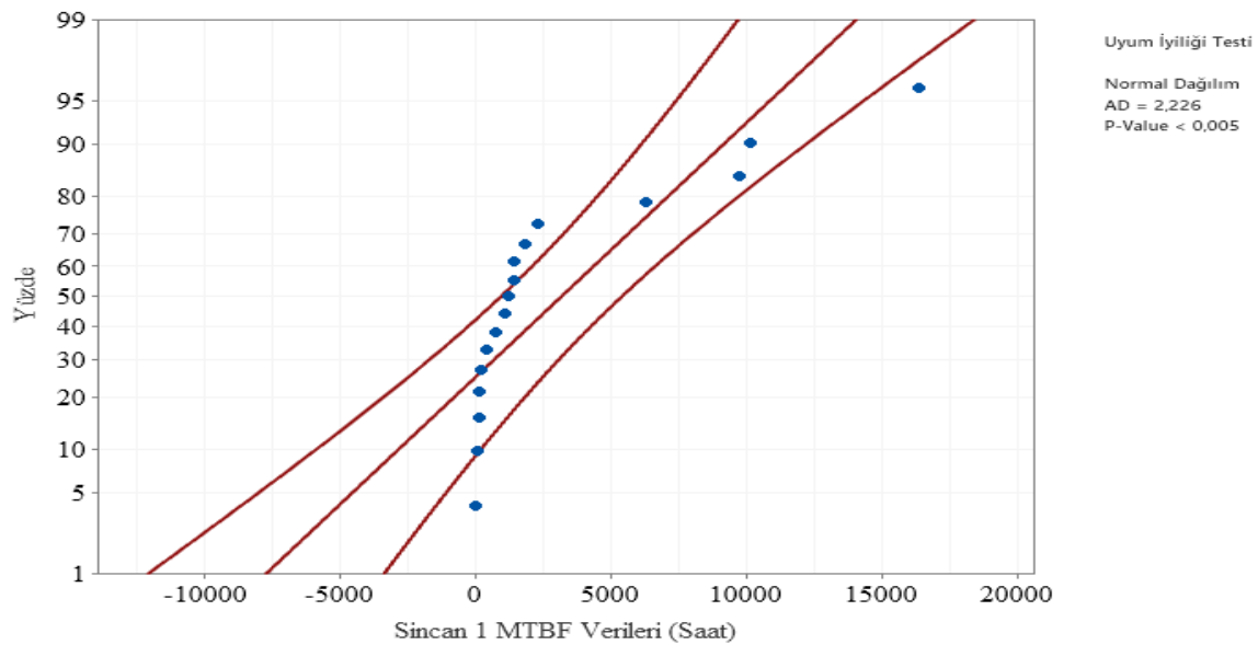
Şekil 6.42. Sincan 1 Fideri normal dağılım Anderson- Darling uyumluluk eğrisi
