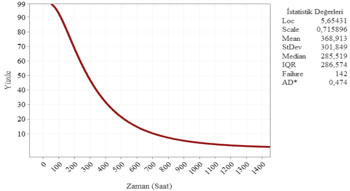
Şekil 6.129. Kangal TES fideri güvenilirlik fonksiyonu eğrisi
