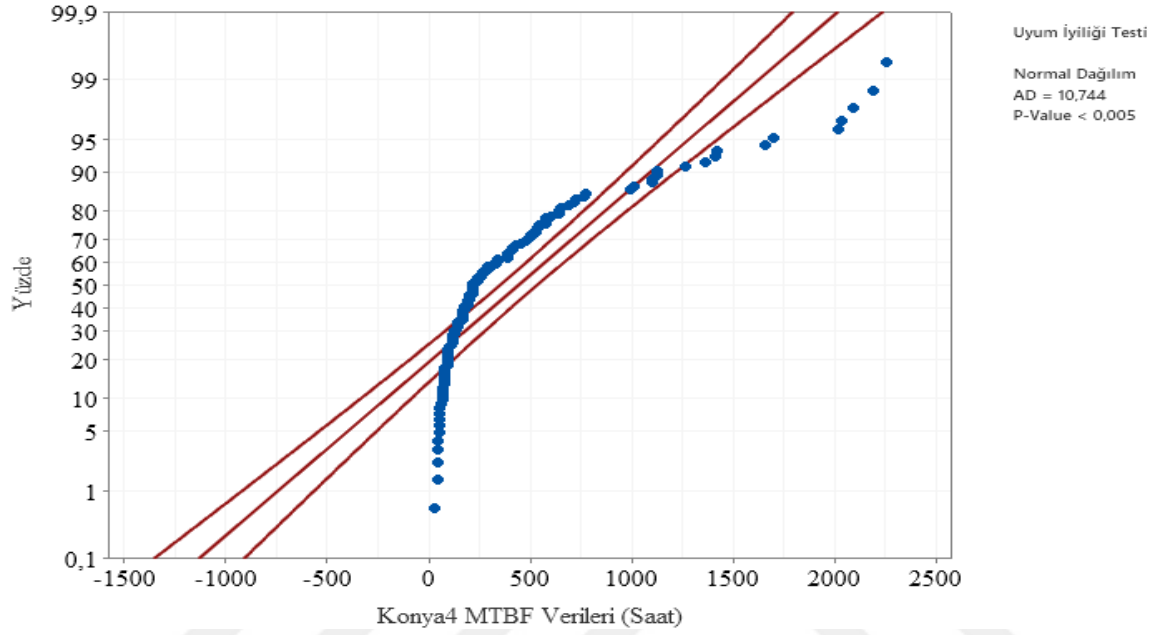
Şekil 6.22. Konya4 Fideri normal dağılım Anderson- Darling uyumluluk eğrisi
