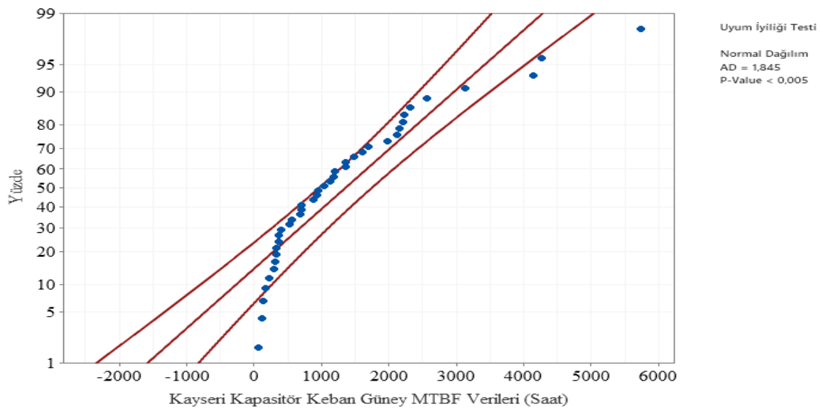
Şekil 6.58. Keban Güney Fideri normal dağılım Anderson- Darling uyumluluk eğrisi
