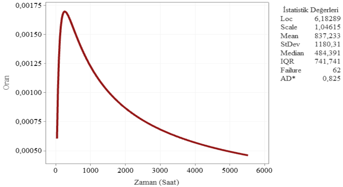
Şekil 6.103. Elbistan A fideri tehlike fonksiyonu eğrisi
