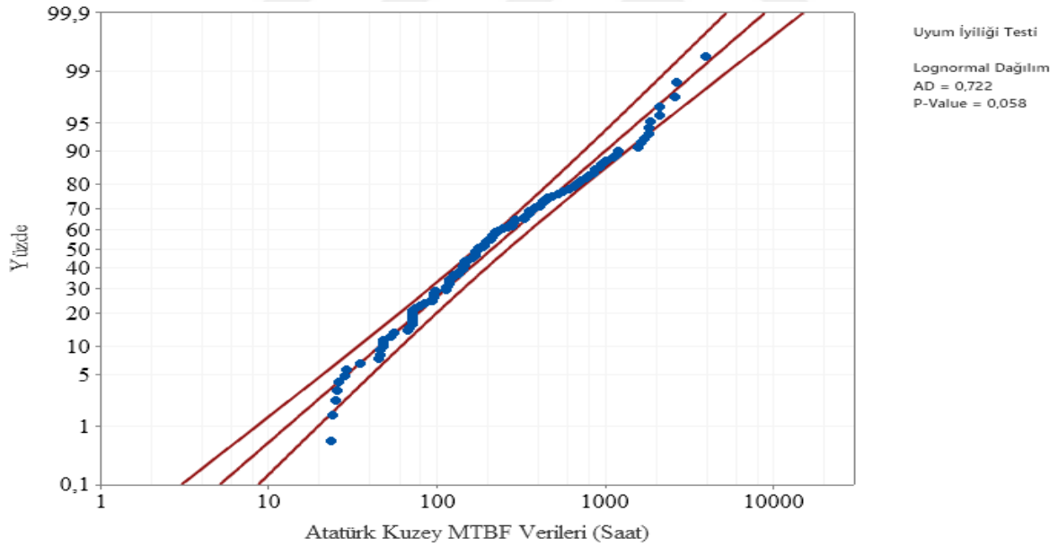
Şekil 6.9. Atatürk Kuzey Fideri lognormal dağılımı Anderson- Darling uyumluluk eğrisi
