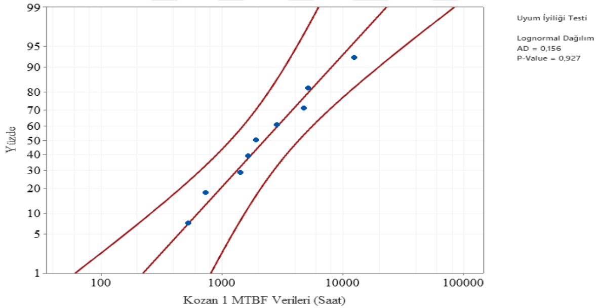
Şekil 6.17. Kozan 1 Fideri lognormal dağılımı Anderson- Darling uyumluluk eğrisi
