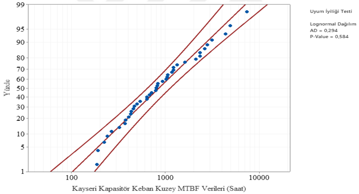
Şekil 6.65. Keban Kuzey Fideri lognormal dağılımı Anderson- Darling uyumluluk eğrisi
