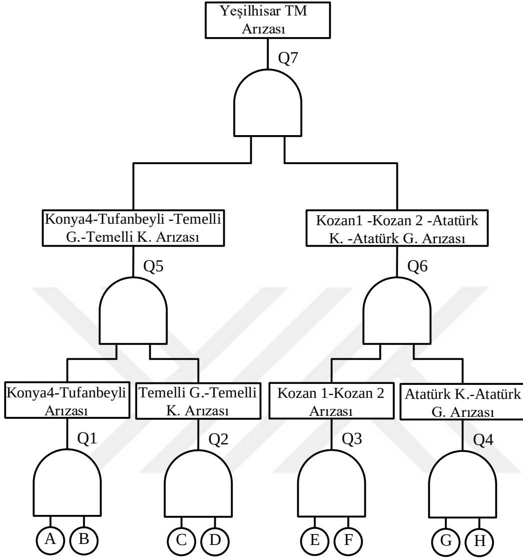
Şekil 6.1. Yeşilhisar TM hata ağacı diyagramı
