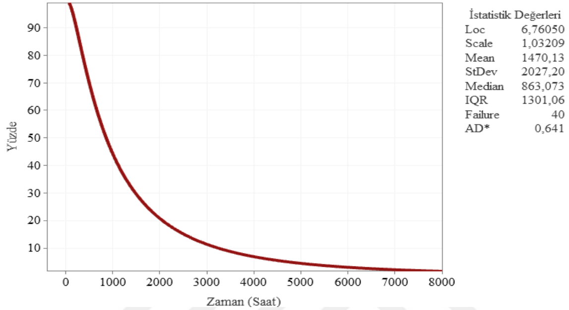
Şekil 6.120. Keban Güney fideri güvenilirlik fonksiyonu eğrisi
