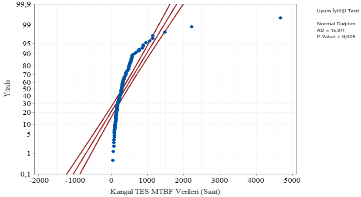
Şekil 6.70. Kangal TES Fideri normal dağılım Anderson- Darling uyumluluk eğrisi
