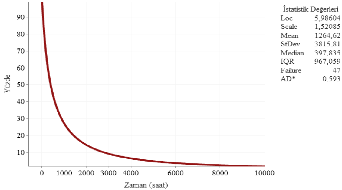
Şekil 6.96. Temelli Güney fideri güvenilirlik fonksiyonu eğrisi
