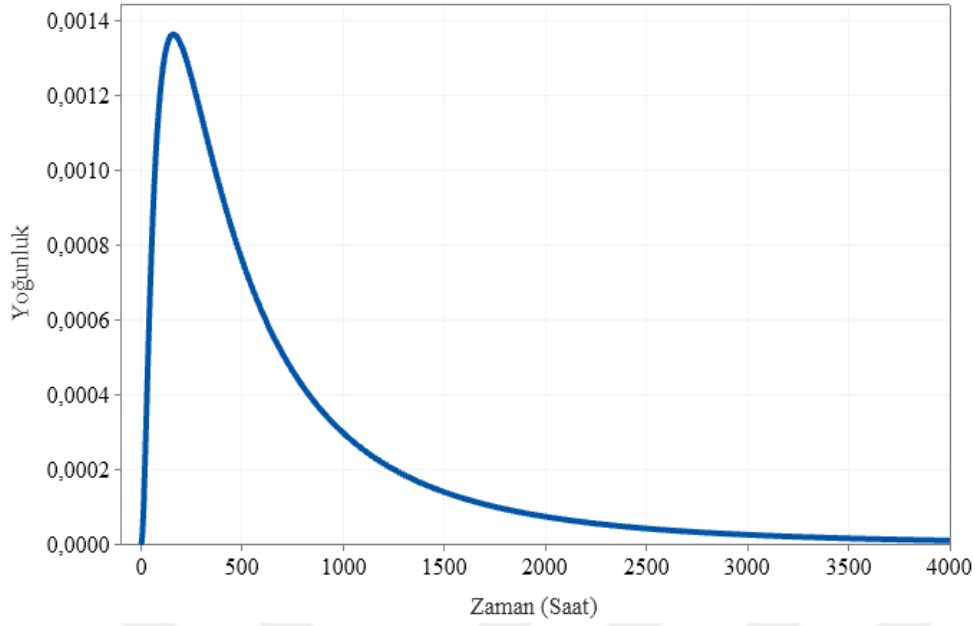
Şekil 6.104. Elbistan A fideri olasılık yoğunluk fonksiyonu eğrisi
