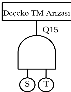
Şekil 6.22. Deçeko TM hata ağacı diyagramı
