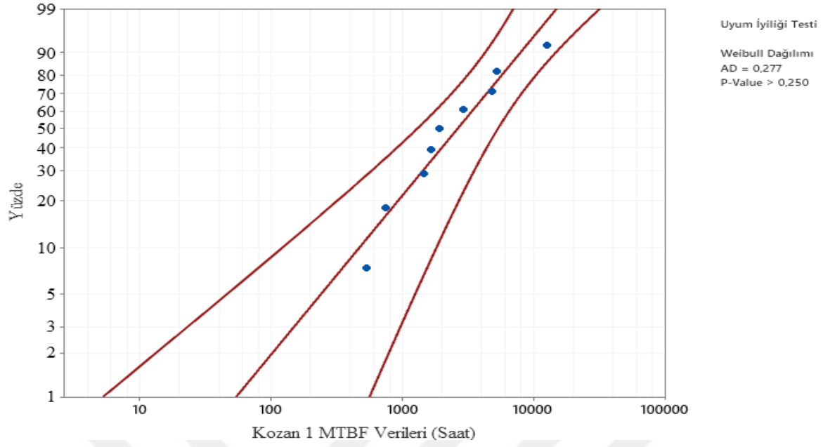
Şekil 6.16. Kozan 1 Fideri weibull dağılımı Anderson- Darling uyumluluk eğrisi
