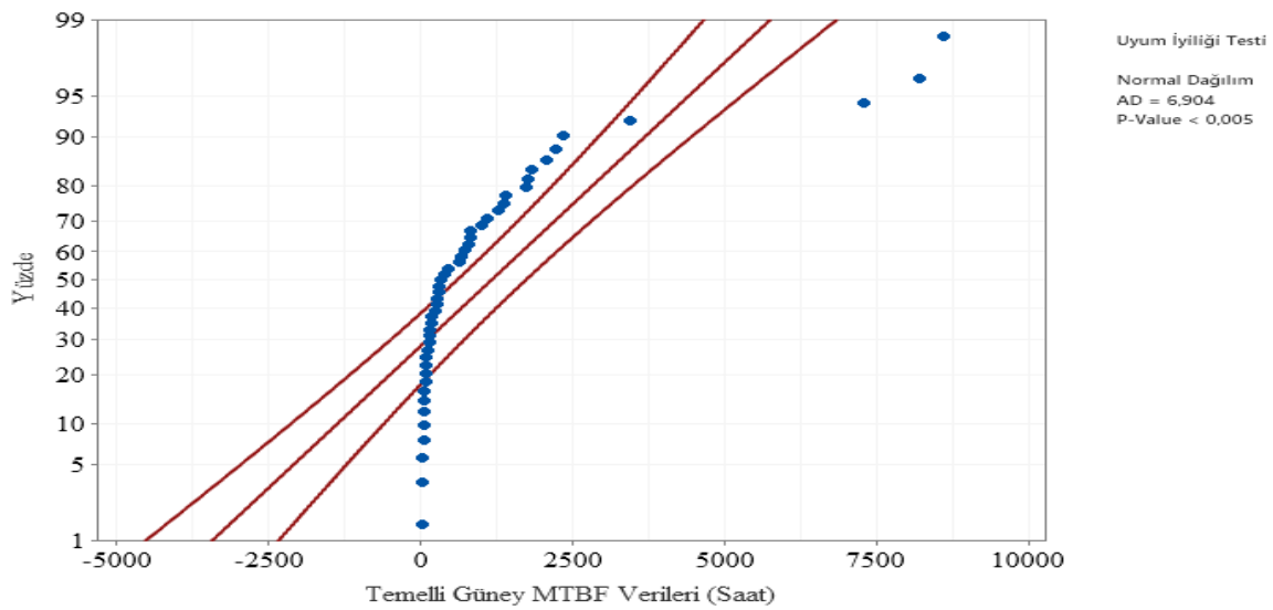
Şekil 6.26. Temelli Güney Fideri normal dağılım Anderson- Darling uyumluluk eğrisi
