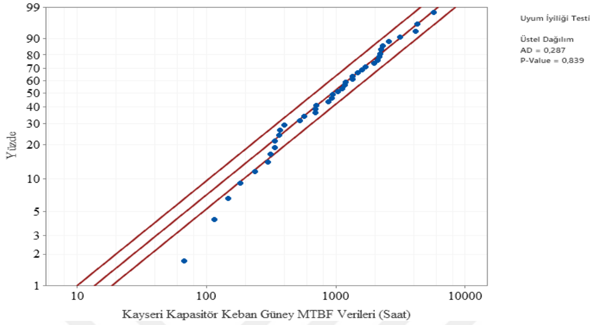
Şekil 6.59. Keban Güney Fideri üstel dağılım Anderson- Darling uyumluluk eğrisi
