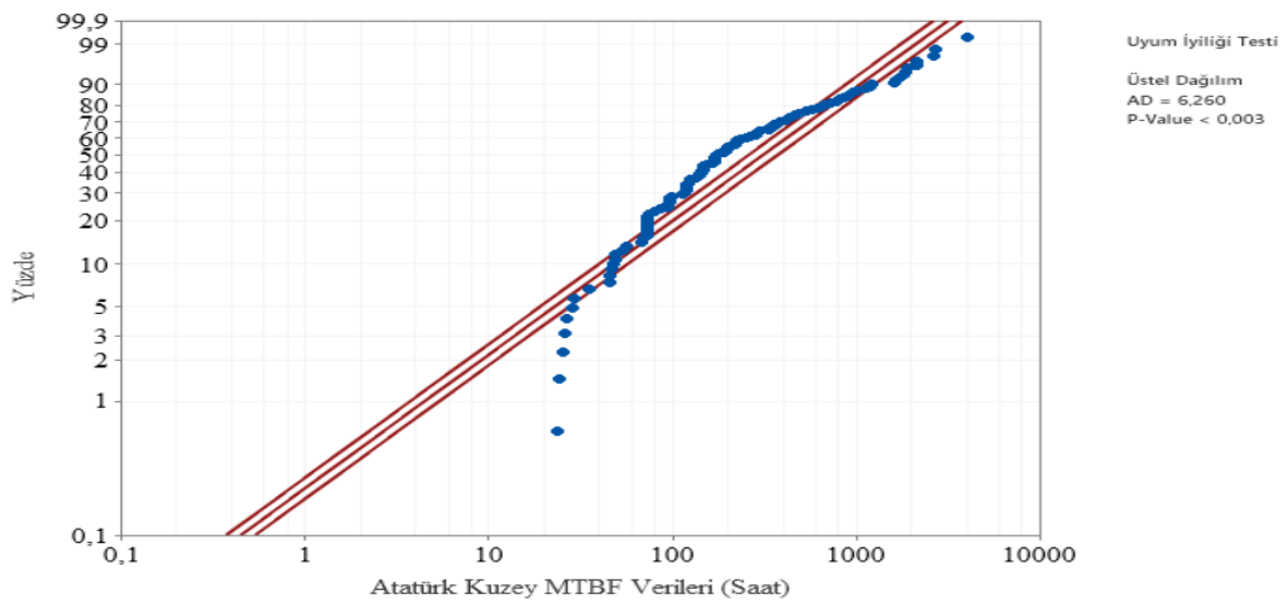
Şekil 6.7. Atatürk Kuzey Fideri üstel dağılım Anderson- Darling uyumluluk eğrisi
