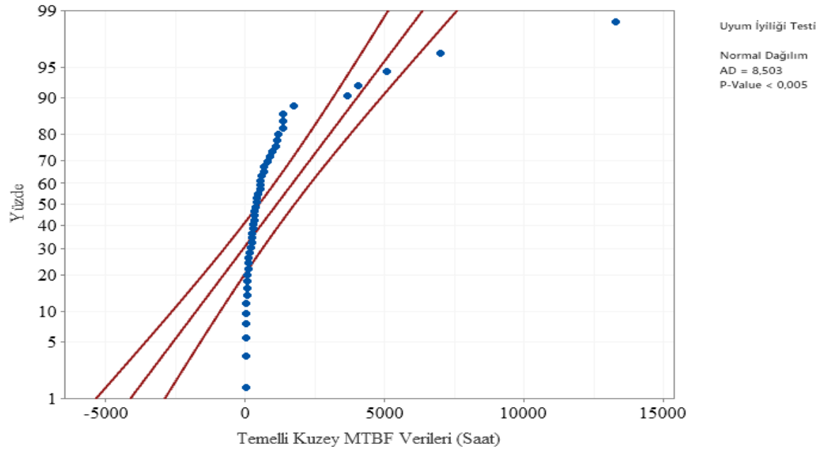
Şekil 6.30. Temelli Kuzey Fideri normal dağılım Anderson- Darling uyumluluk eğrisi
