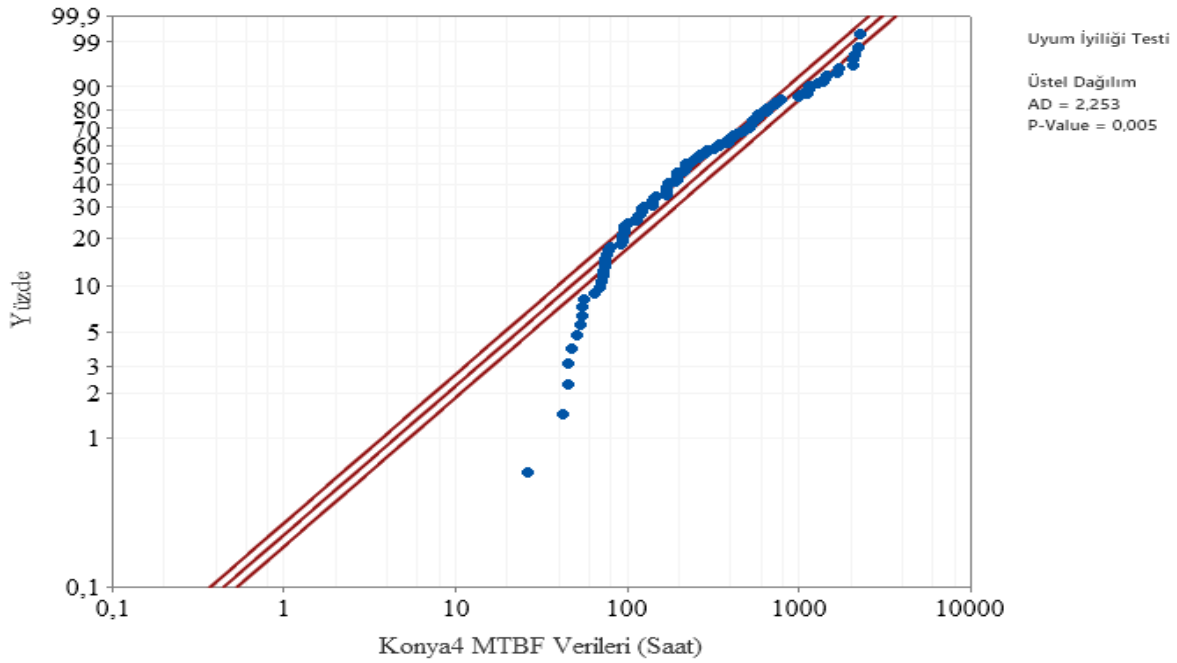
Şekil 6.23. Konya4 Fideri üstel dağılım Anderson- Darling uyumluluk eğrisi
