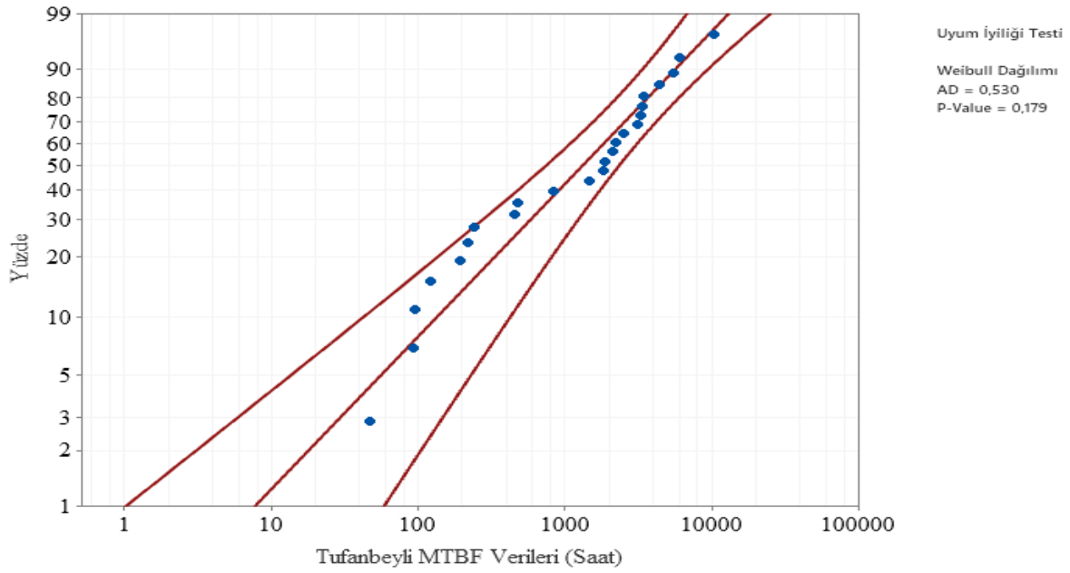
Şekil 6.12. Tufanbeyli Fideri weibull dağılımı Anderson- Darling uyumluluk eğrisi
