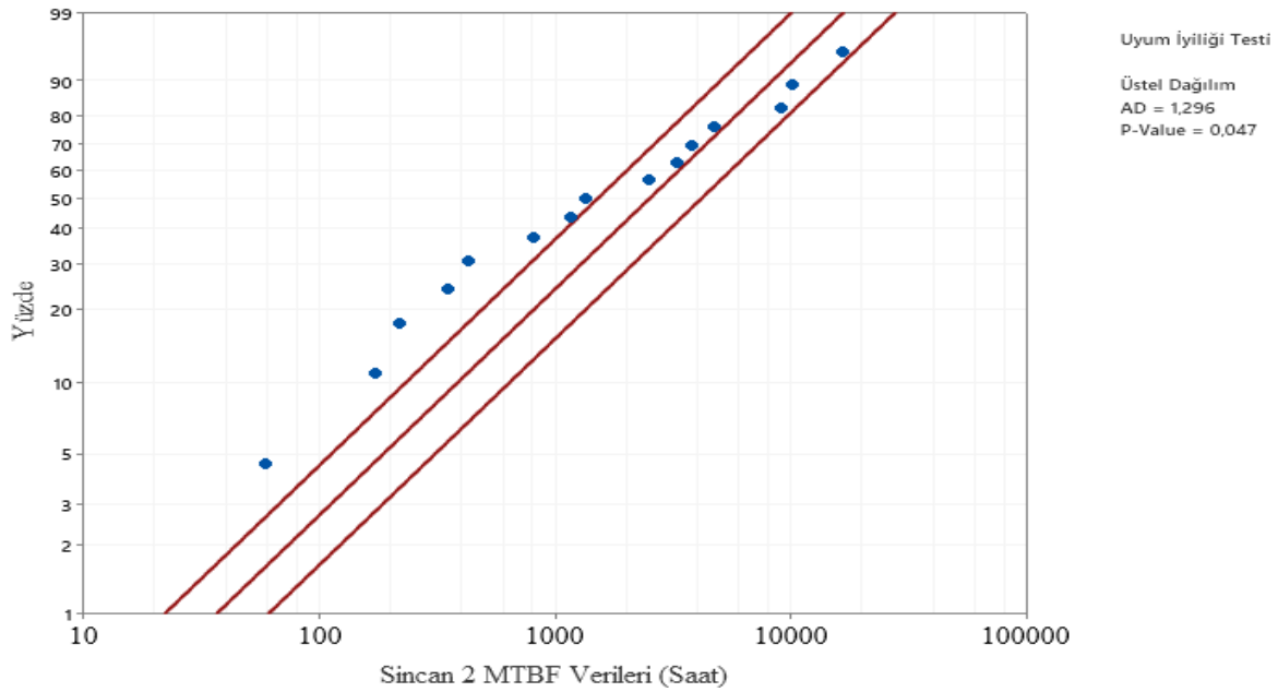
Şekil 6.47. Sincan 2 Fideri üstel dağılım Anderson- Darling uyumluluk eğrisi
