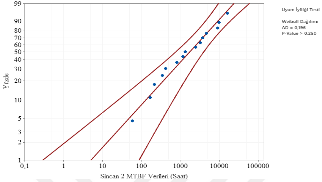
Şekil 6.48. Sincan 2 Fideri weibull dağılımı Anderson- Darling uyumluluk eğrisi
