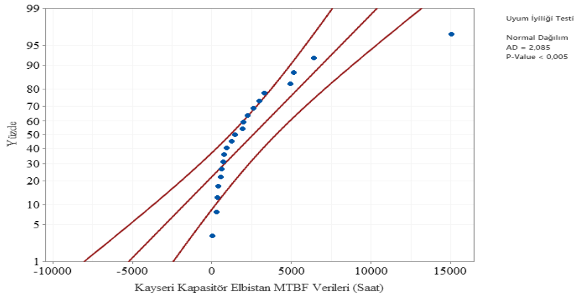
Şekil 6.66. Elbistan Fideri normal dağılım Anderson- Darling uyumluluk eğrisi
