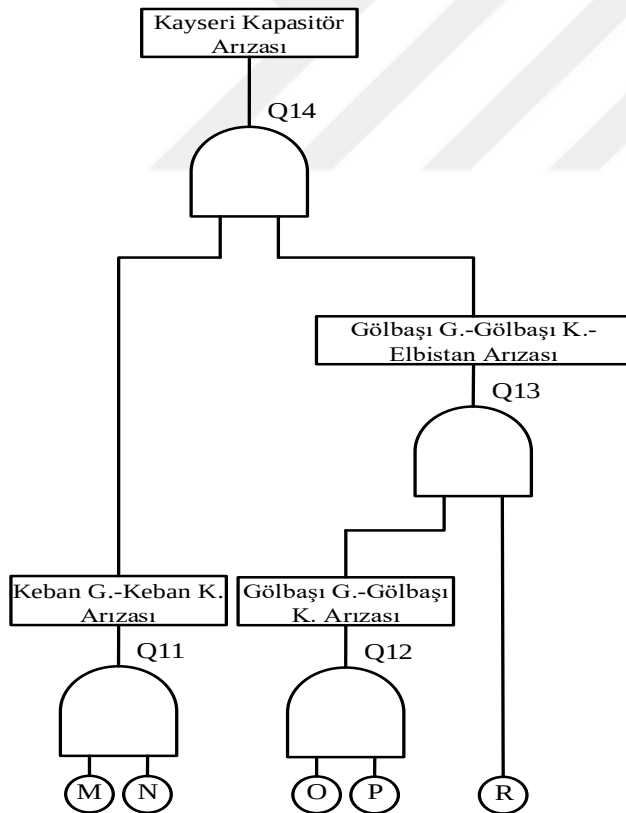
Şekil 6.141. Kayseri Kapasitör hata ağacı diyagramı
