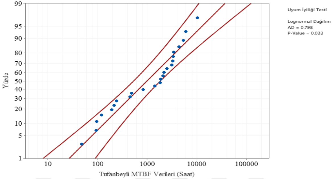
Şekil 6.13. Tufanbeyli Fideri lognormal dağılımı Anderson- Darling uyumluluk eğrisi
