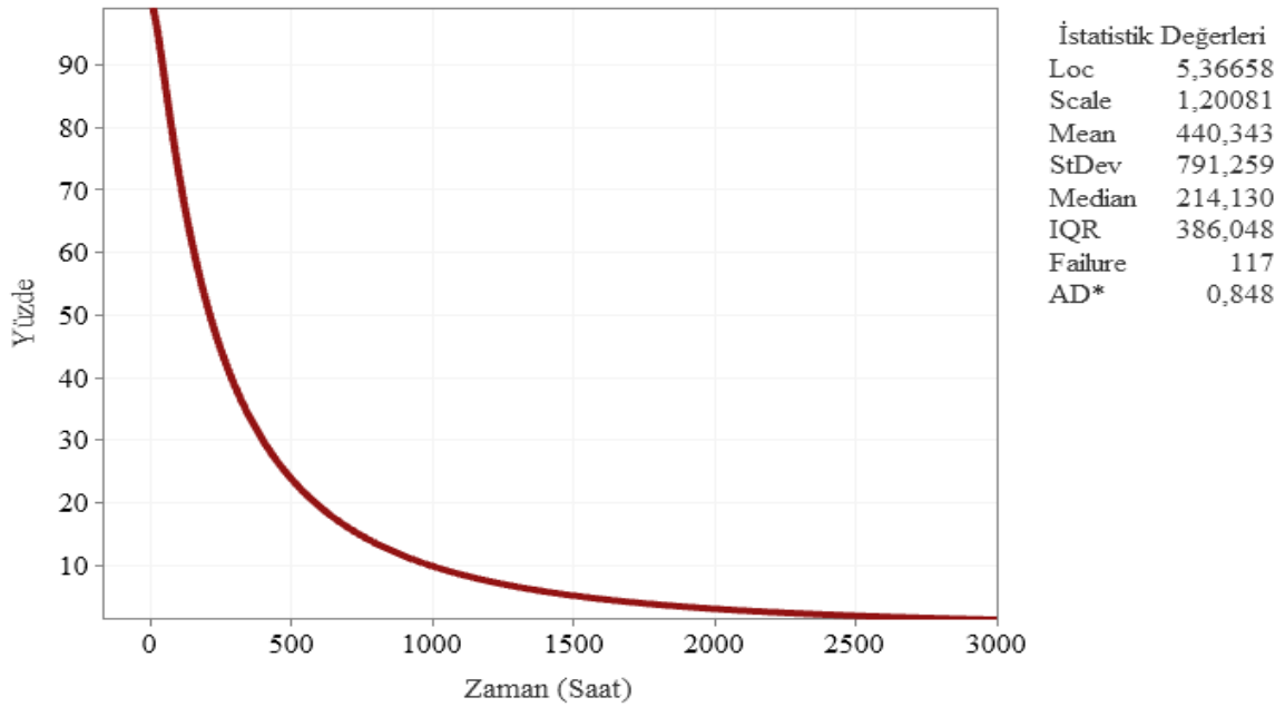
Şekil 6.81. Atatürk Kuzey fideri güvenilirlik fonksiyonu eğrisi
