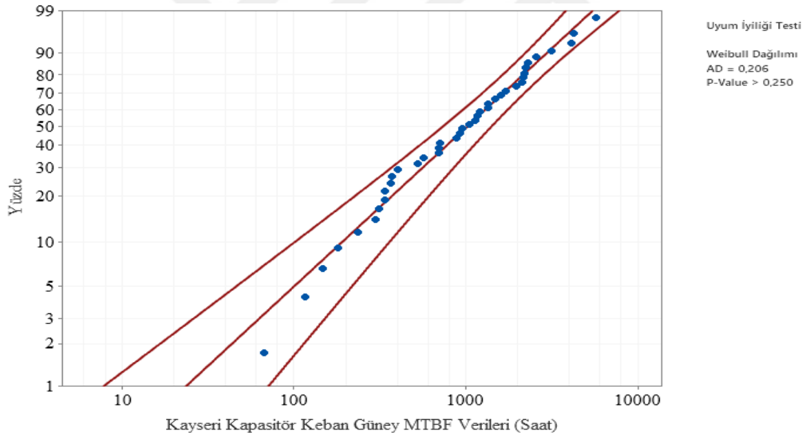
Şekil 6.60. Keban Güney Fideri weibull dağılımı Anderson- Darling uyumluluk eğrisi
