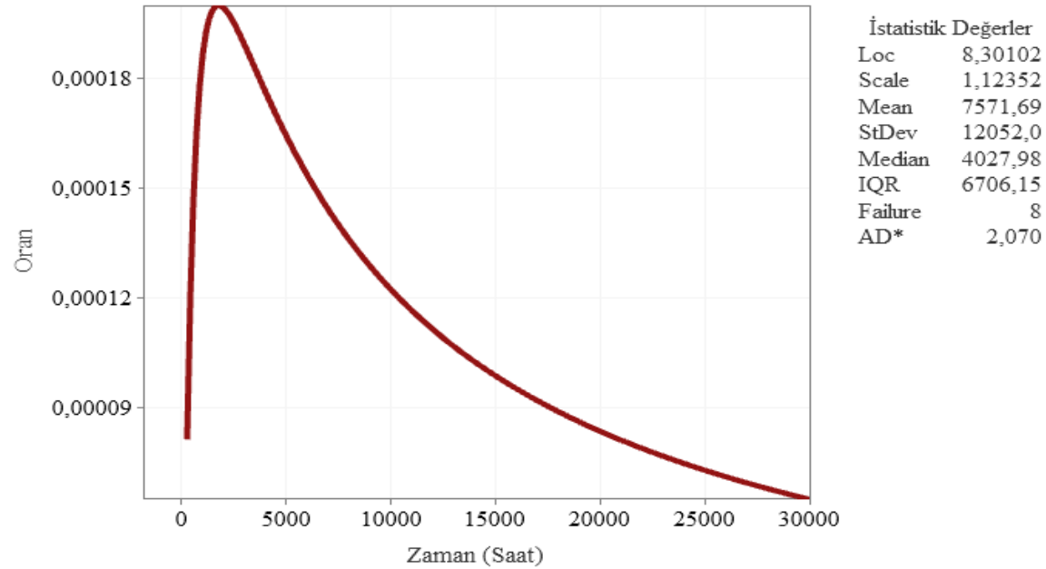
Şekil 6.115. Gölbaşı Kuzey fideri tehlike fonksiyonu eğrisi
