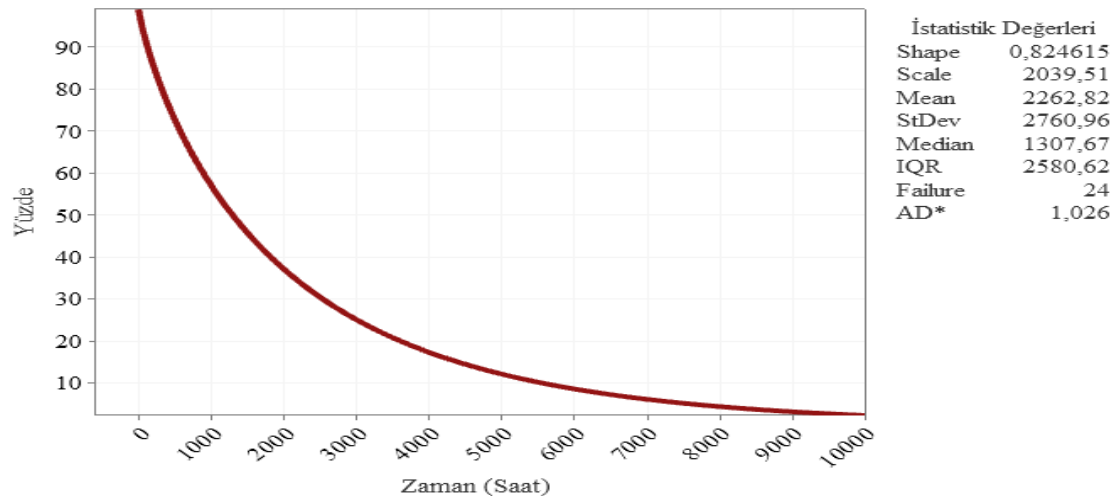
Şekil 6.84. Tufanbeyli fideri güvenilirlik fonksiyonu eğrisi
