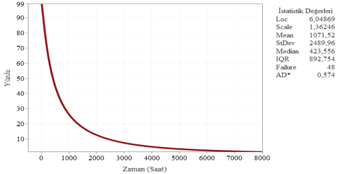
Şekil 6.99. Temelli Kuzey fideri güvenilirlik fonksiyonu eğrisi
