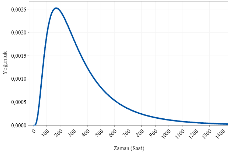
Şekil 6.131. Kangal TES fideri olasılık yoğunluk fonksiyonu eğrisi
