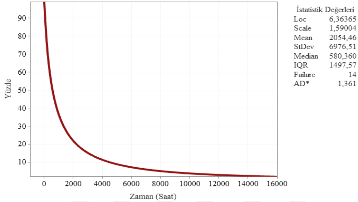
Şekil 6.90. Kozan 2 fideri güvenilirlik fonksiyonu eğrisi
