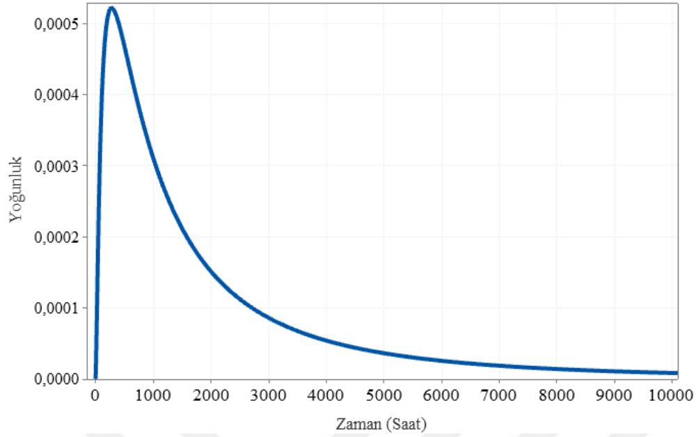
Şekil 6.128. Elbistan fideri olasılık yoğunluk fonksiyonu eğrisi
