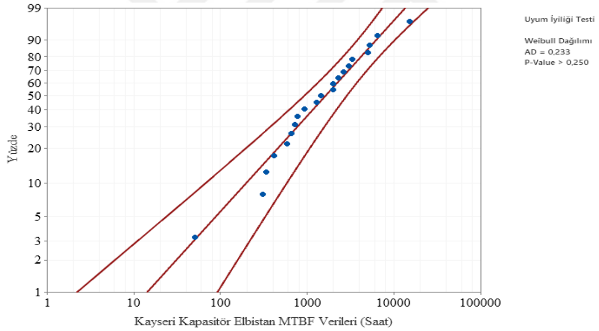
Şekil 6.68. Elbistan Fideri weibull dağılımı Anderson- Darling uyumluluk eğrisi
