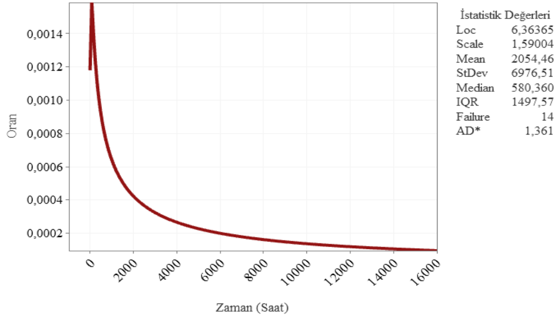
Şekil 6.91. Kozan 2 fideri tehlike fonksiyonu eğrisi
