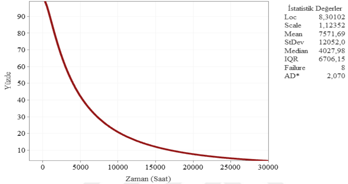
Şekil 6.114. Gölbaşı Kuzey fideri güvenilirlik fonksiyonu eğrisi
