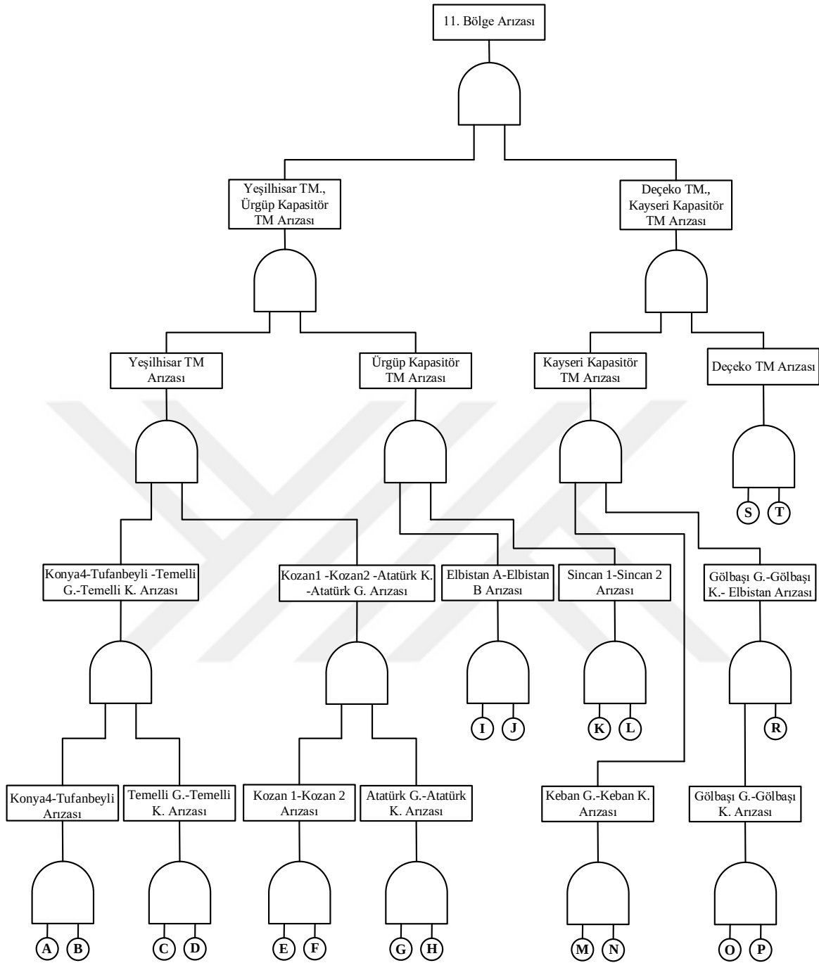
Şekil 6.136. TEİAŞ 11. Bölgesine ait hata ağacı diyagramı
