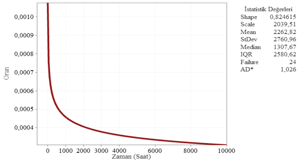
Şekil 6.85. Tufanbeyli fideri tehlike fonksiyonu eğrisi
