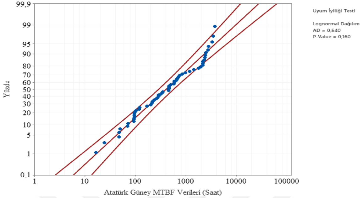
Şekil 6.5. Atatürk Güney Fideri lognormal dağılımı Anderson- Darling uyumluluk eğrisi
