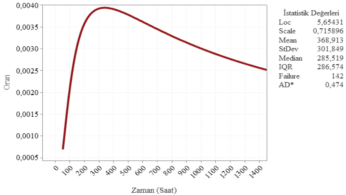
Şekil 6.130. Kangal TES fideri tehlike fonksiyonu eğrisi
