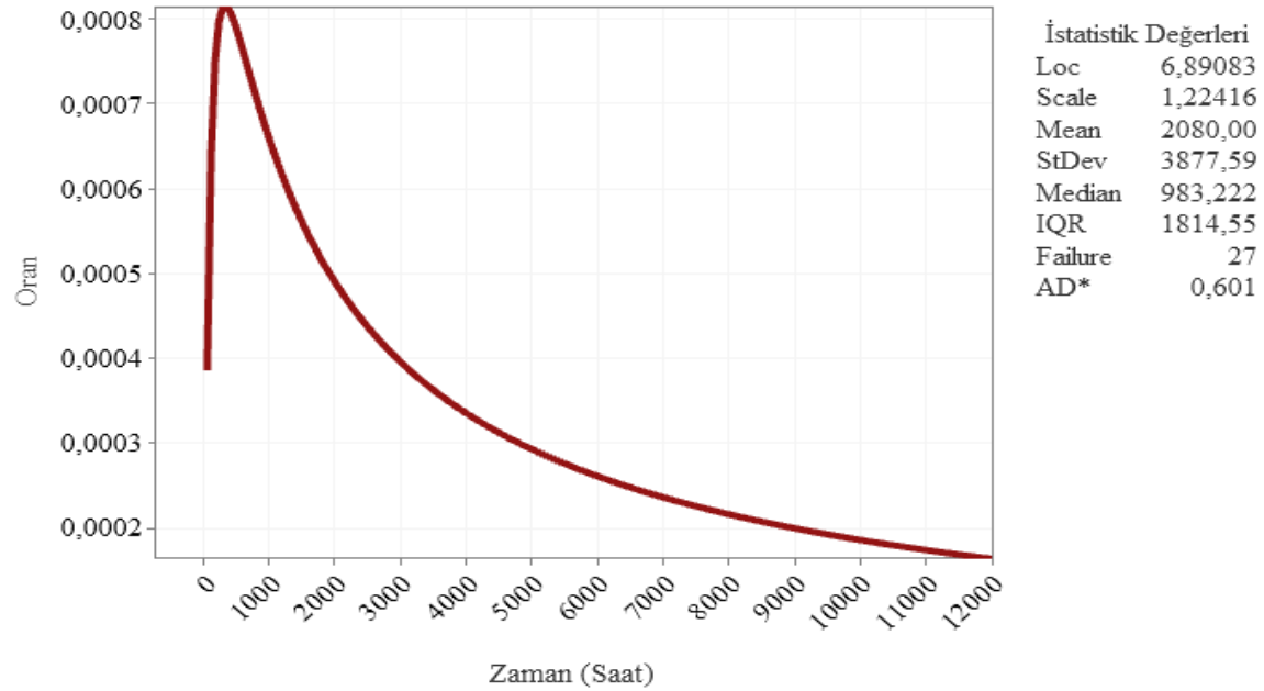
Şekil 6.118. Gölbaşı Güney fideri tehlike fonksiyonu eğrisi
