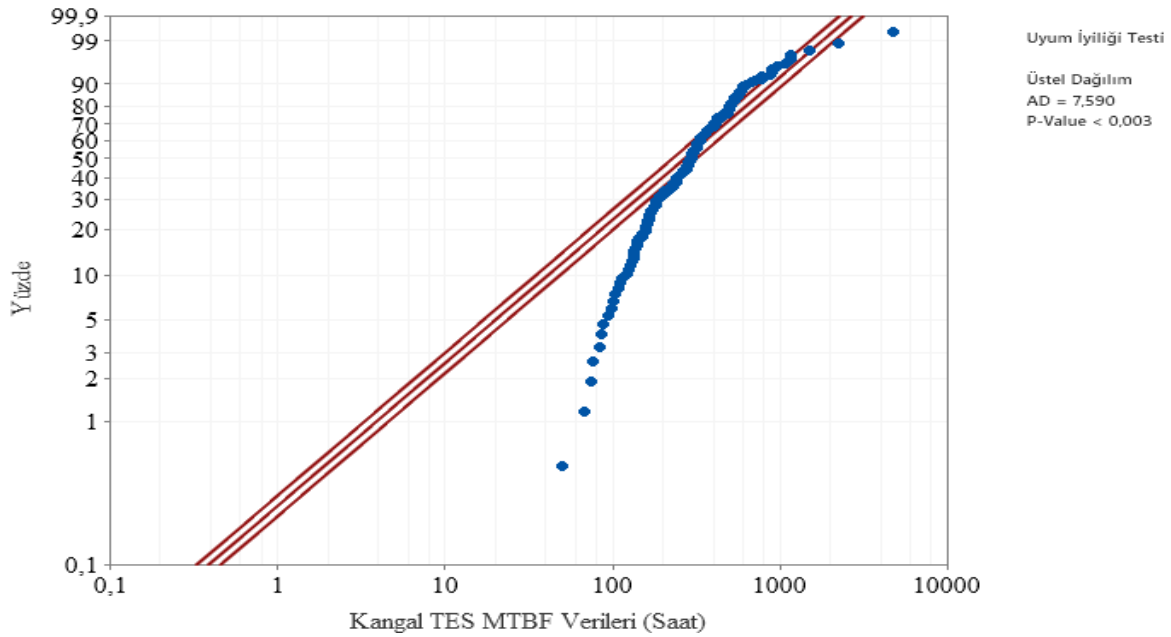
Şekil 6.71. Kangal TES Fideri üstel dağılım Anderson- Darling uyumluluk eğrisi
