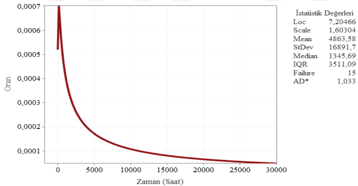
Şekil 6.112. Sincan 2 fideri tehlike fonksiyonu eğrisi
