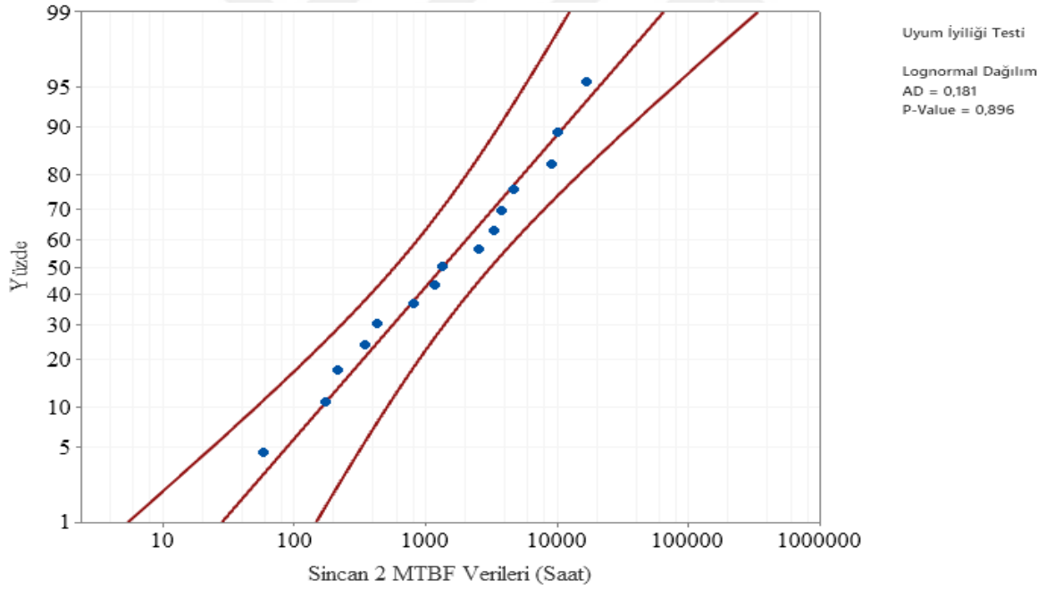
Şekil 6.49. Sincan 2 Fideri lognormal dağılımı Anderson- Darling uyumluluk eğrisi
