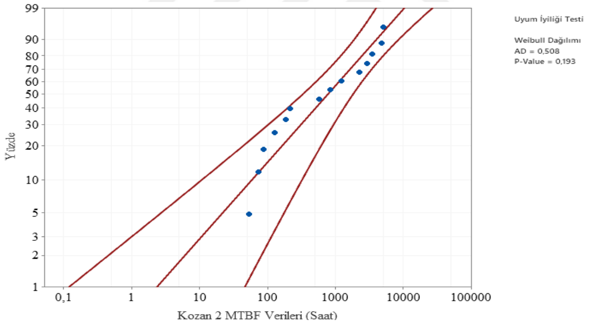
Şekil 6.20. Kozan 2 Fideri weibull dağılımı Anderson- Darling uyumluluk eğrisi
