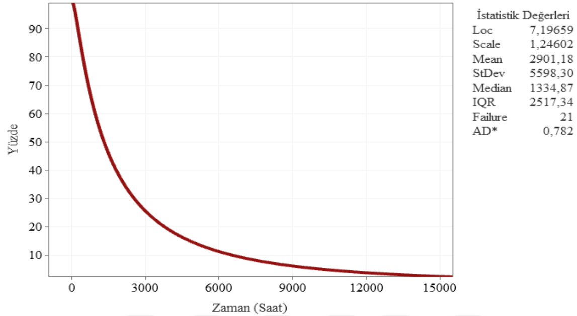
Şekil 6.126. Elbistan fideri güvenilirlik fonksiyonu eğrisi
