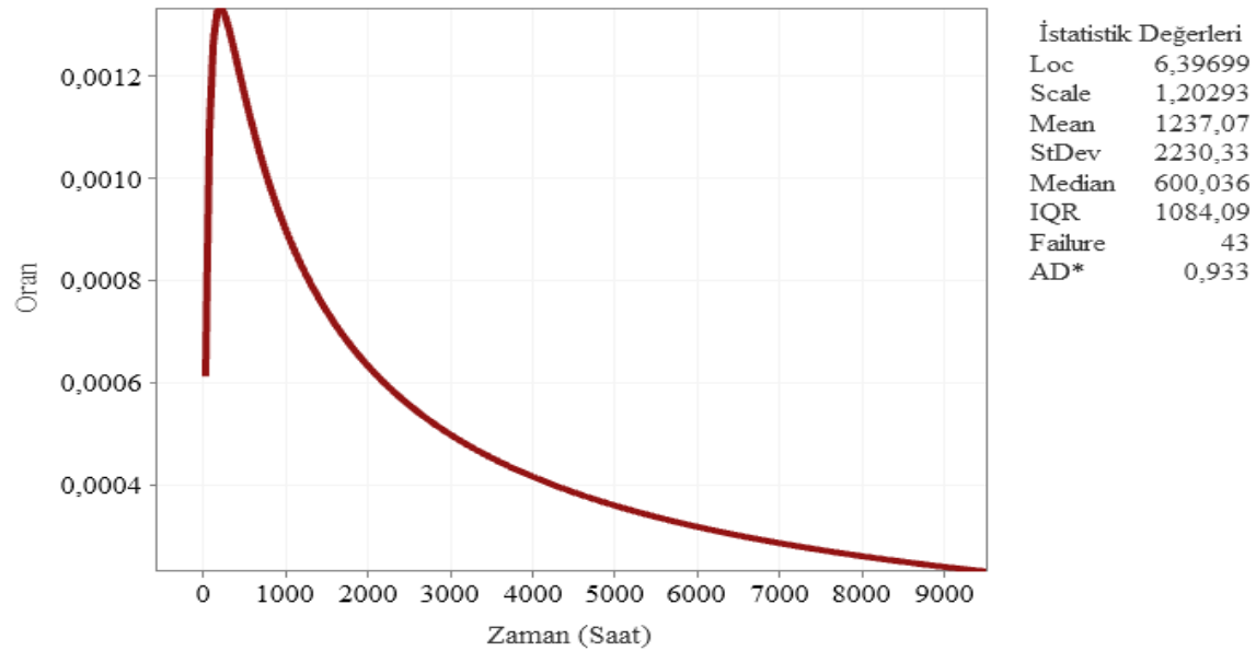
Şekil 6.106. Elbistan B fideri tehlike fonksiyonu eğrisi
