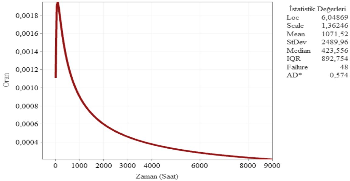
Şekil 6.100. Temelli Kuzey fideri tehlike fonksiyonu eğrisi
