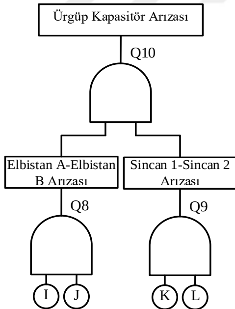
Şekil 6.140. Ürgüp Kapasitör hata ağacı diyagramı
