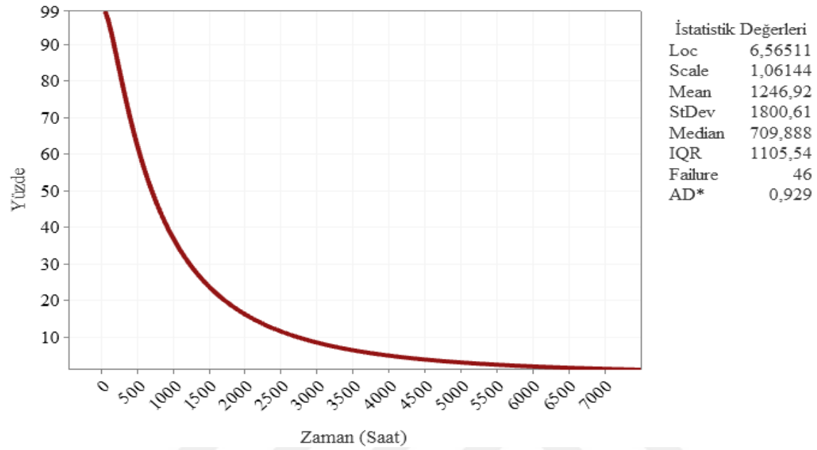
Şekil 6.132. Kayabaşı fideri güvenilirlik fonksiyonu eğrisi
