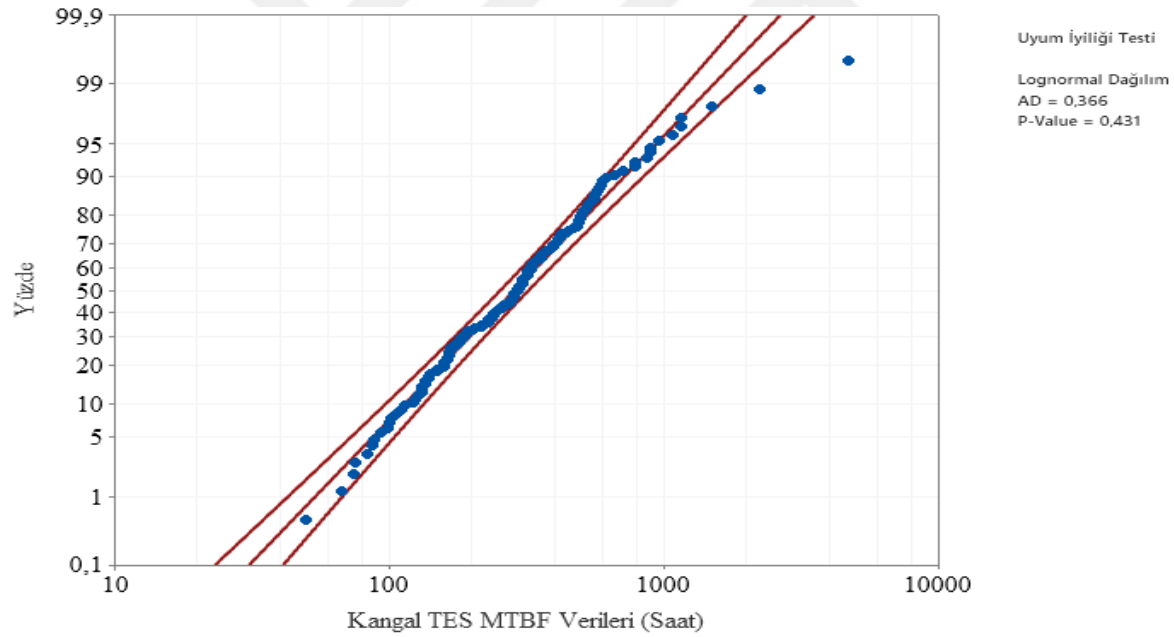
Şekil 6.73. Kangal TES Fideri lognormal dağılımı Anderson- Darling uyumluluk eğrisi
