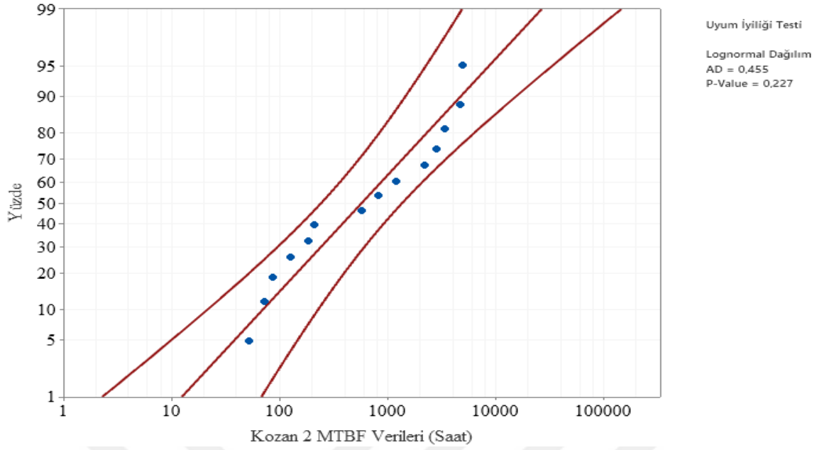
Şekil 6.21. Kozan 2 Fideri lognormal dağılımı Anderson- Darling uyumluluk eğrisi
