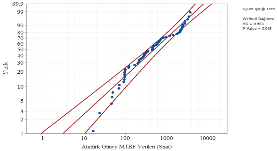
Şekil 6.4. Atatürk Güney Fideri weibull dağılımı Anderson- Darling uyumluluk eğrisi
