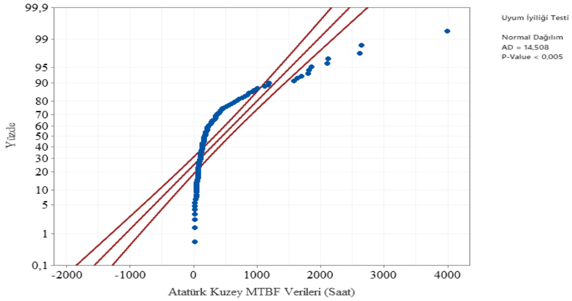
Şekil 6.6. Atatürk Kuzey Fideri normal dağılım Anderson- Darling uyumluluk eğrisi
