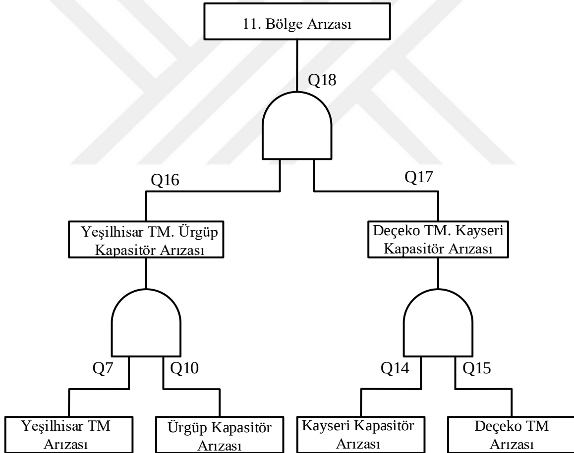
Şekil 6.143. Tepe olay ara olay hata ağacı diyagramı
