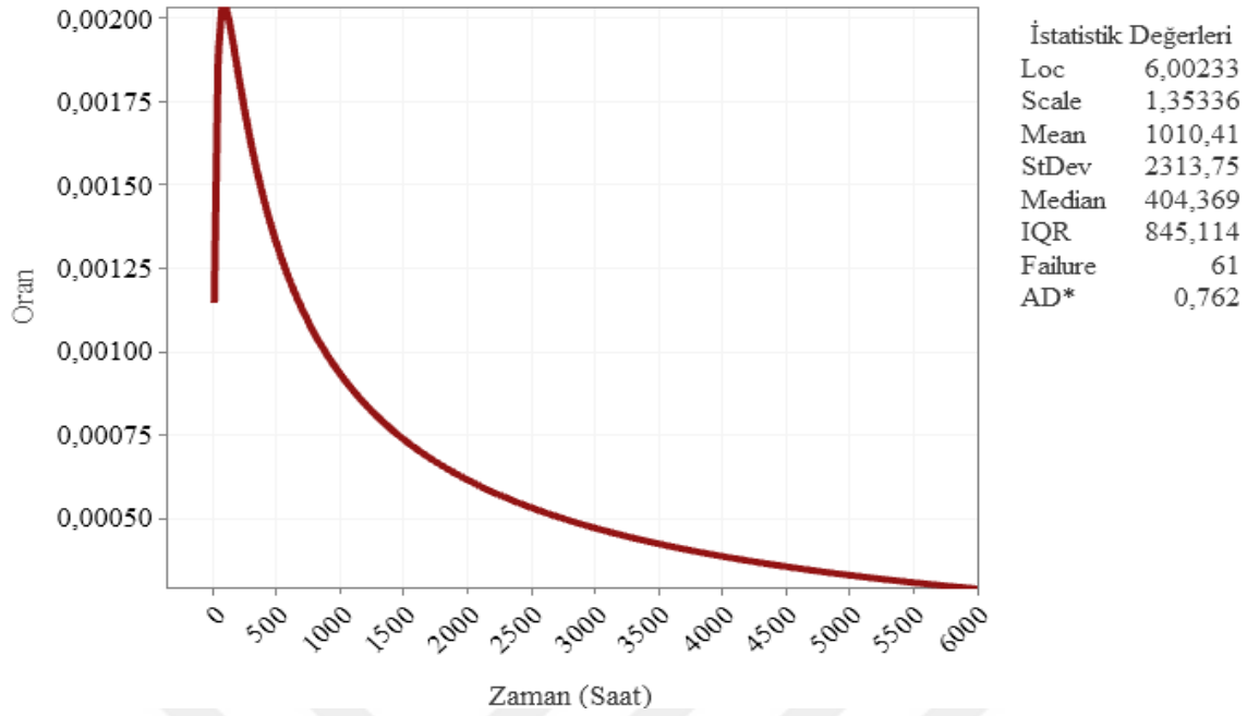
Şekil 6.79. Atatürk Güney fideri tehlike fonksiyonu eğrisi
