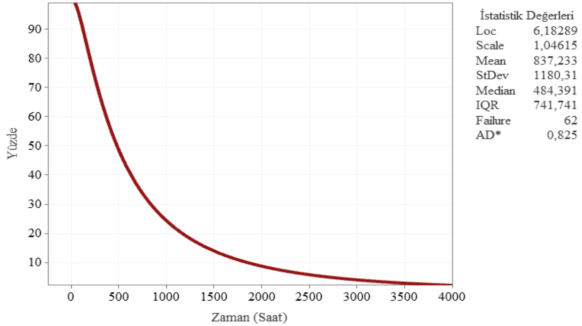
Şekil 6.102. Elbistan A fideri güvenilirlik fonksiyonu eğrisi
