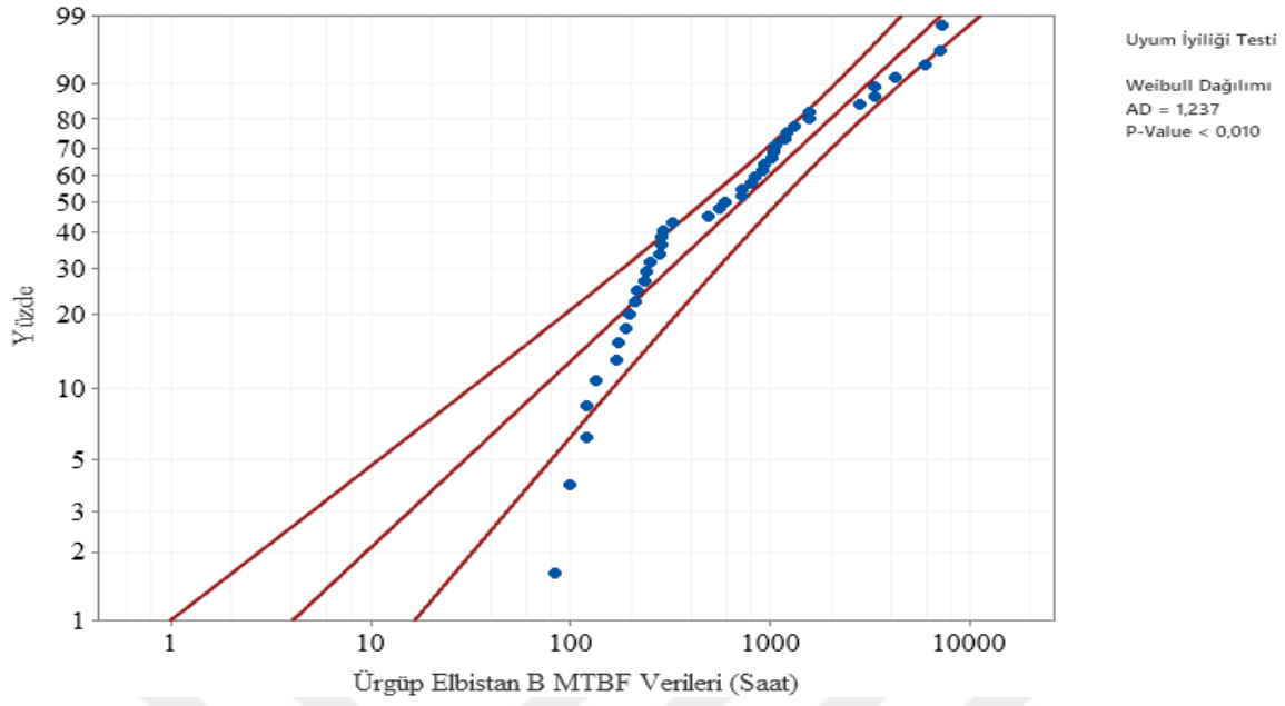
Şekil 6.40. Elbistan B Fideri weibull dağılımı Anderson- Darling uyumluluk eğrisi
