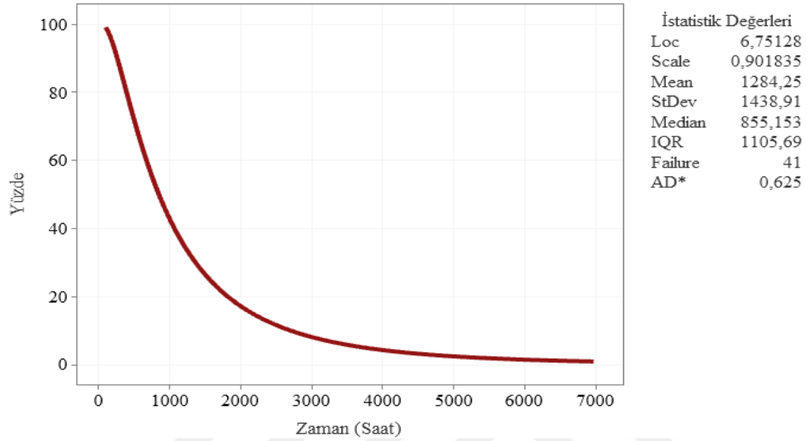
Şekil 6.123. Keban Kuzey fideri güvenilirlik fonksiyonu eğrisi
