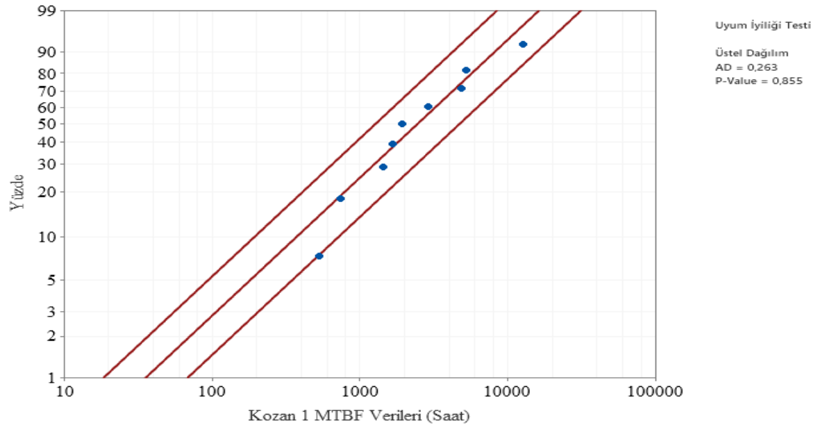
Şekil 6.15. Kozan 1 Fideri üstel dağılım Anderson- Darling uyumluluk eğrisi
