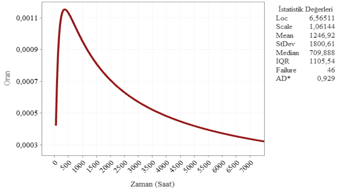
Şekil 6.133. Kayabaşı fideri tehlike fonksiyonu eğrisi
