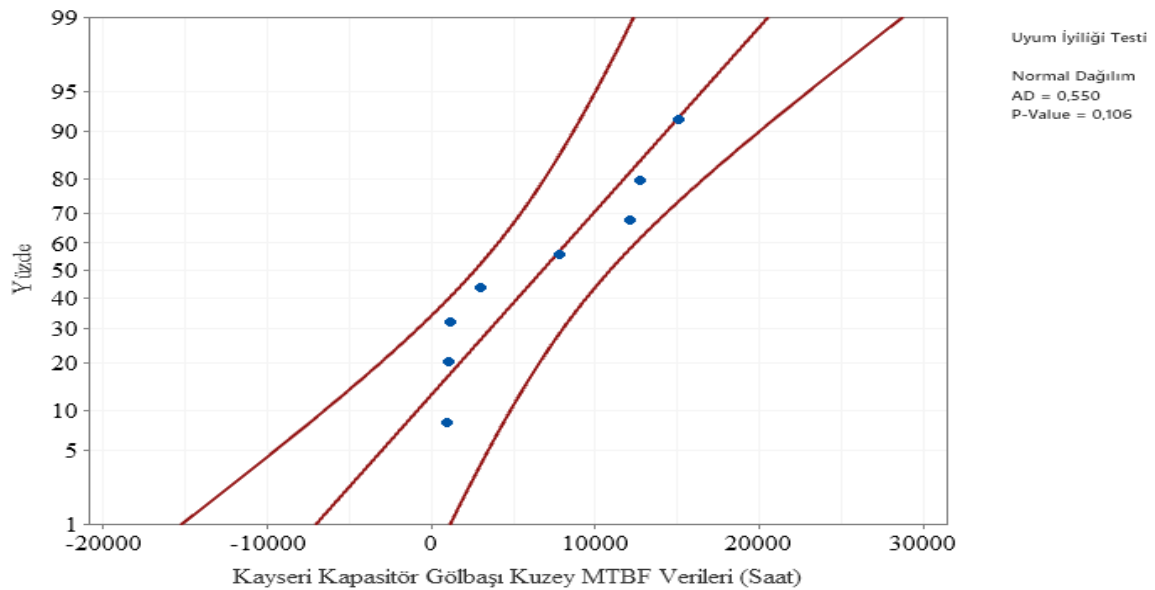
Şekil 6.50. Gölbaşı Kuzey Fideri normal dağılım Anderson- Darling uyumluluk eğrisi
