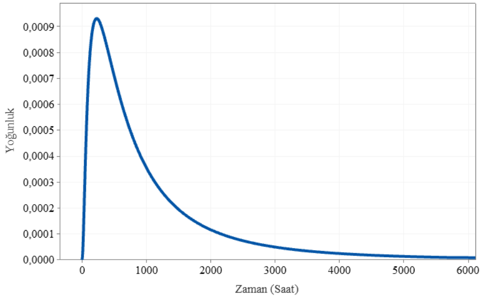
Şekil 6.134. Kayabaşı fideri olasılık yoğunluk fonksiyonu eğrisi
