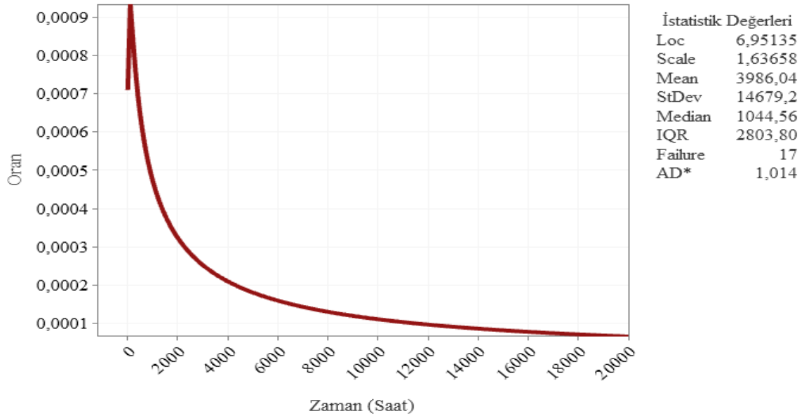
Şekil 6.109. Sincan 1 fideri tehlike fonksiyonu eğrisi
