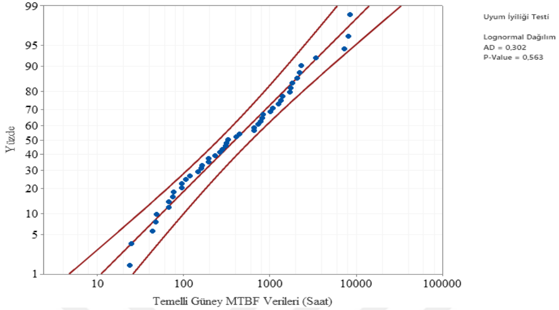
Şekil 6.29. Temelli Güney Fideri lognormal dağılımı Anderson- Darling uyumluluk eğrisi
