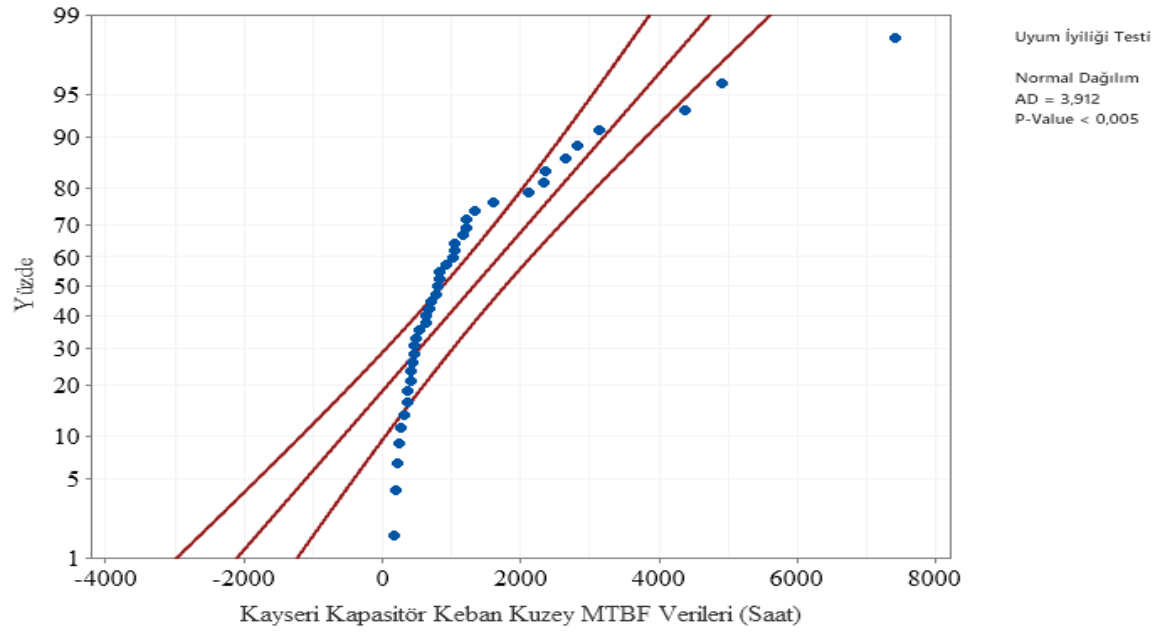
Şekil 6.62. Keban Kuzey Fideri normal dağılım Anderson- Darling uyumluluk eğrisi
