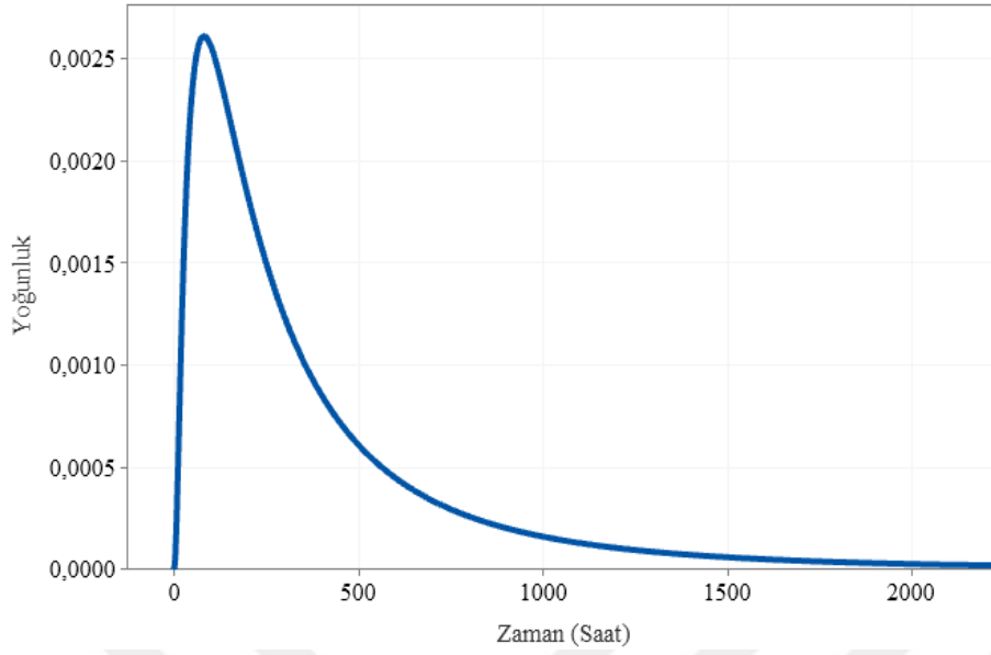
Şekil 6.95. Konya4 fideri olasılık yoğunluk fonksiyonu eğrisi
