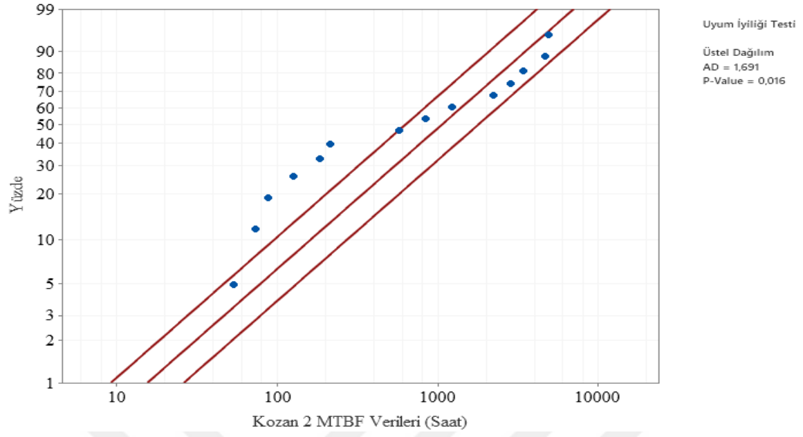
Şekil 6.19. Kozan 2 Fideri üstel dağılım Anderson- Darling uyumluluk eğrisi
