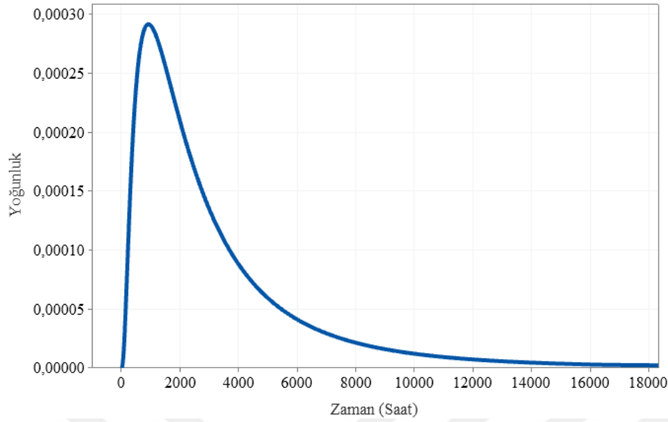
Şekil 6.89. Kozan 1 fideri olasılık yoğunluk fonksiyonu eğrisi
