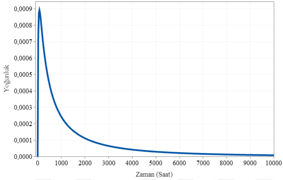
Şekil 6.110. Sincan 1 fideri olasılık yoğunluk fonksiyonu eğrisi
