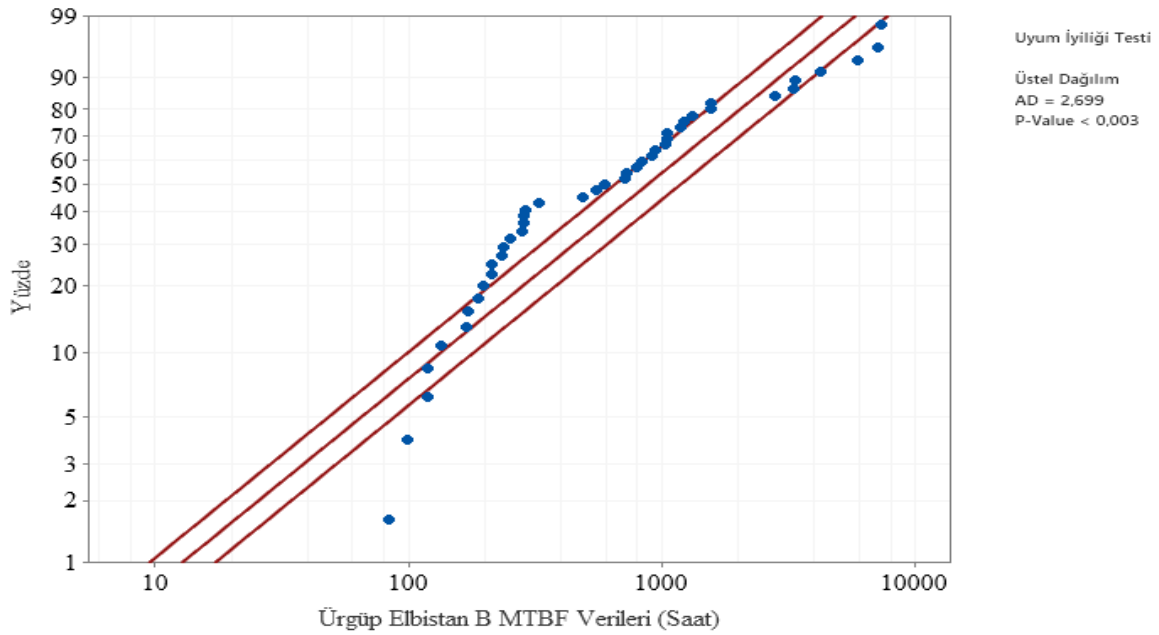
Şekil 6.39. Elbistan B Fideri üstel dağılım Anderson- Darling uyumluluk eğrisi
