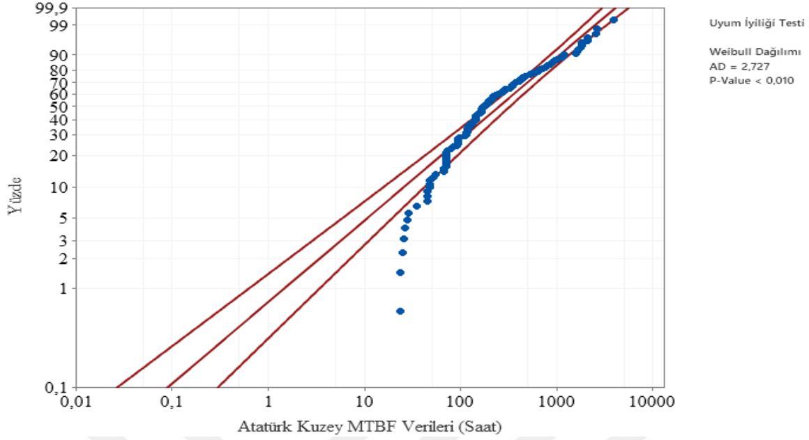
Şekil 6.8. Atatürk Kuzey Fideri weibull dağılımı Anderson- Darling uyumluluk eğrisi
