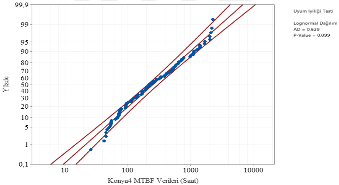
Şekil 6.25. Konya4 Fideri lognormal dağılımı Anderson- Darling uyumluluk eğrisi
