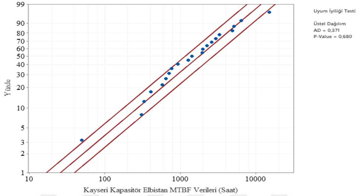
Şekil 6.67. Elbistan Fideri üstel dağılım Anderson- Darling uyumluluk eğrisi
