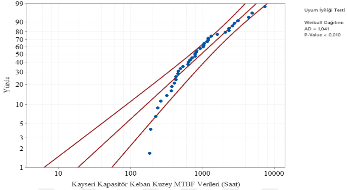
Şekil 6.64. Keban Kuzey Fideri weibull dağılımı Anderson- Darling uyumluluk eğrisi
