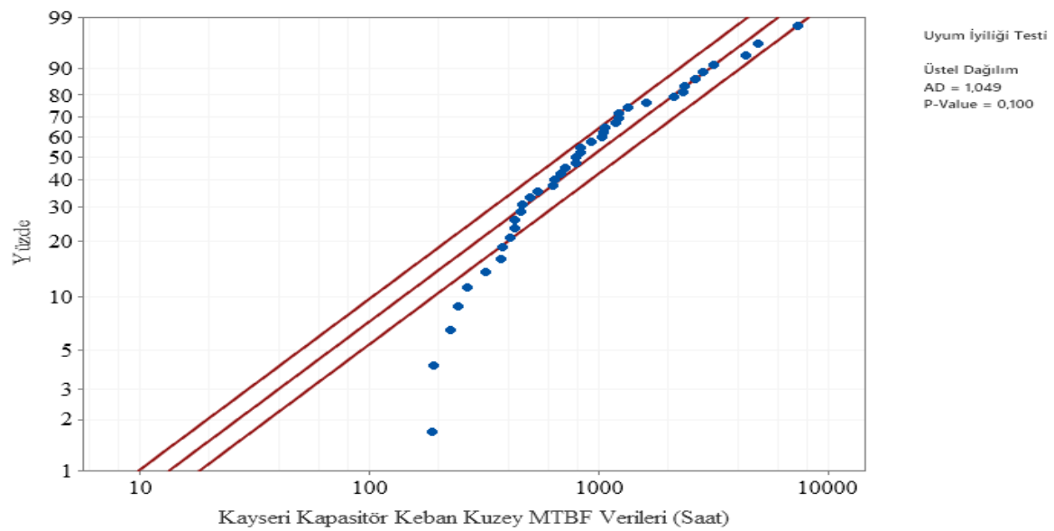
Şekil 6.63. Keban Kuzey Fideri üstel dağılım Anderson- Darling uyumluluk eğrisi
