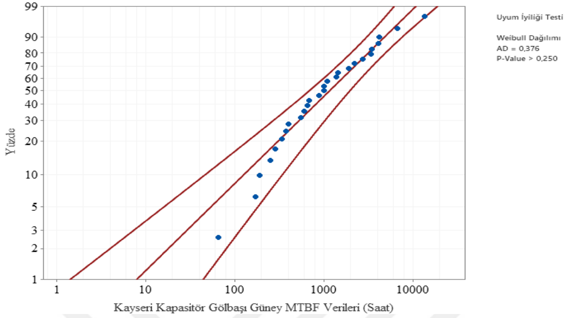
Şekil 6.56. Gölbaşı Güney Fideri weibull dağılımı Anderson- Darling uyumluluk eğrisi
