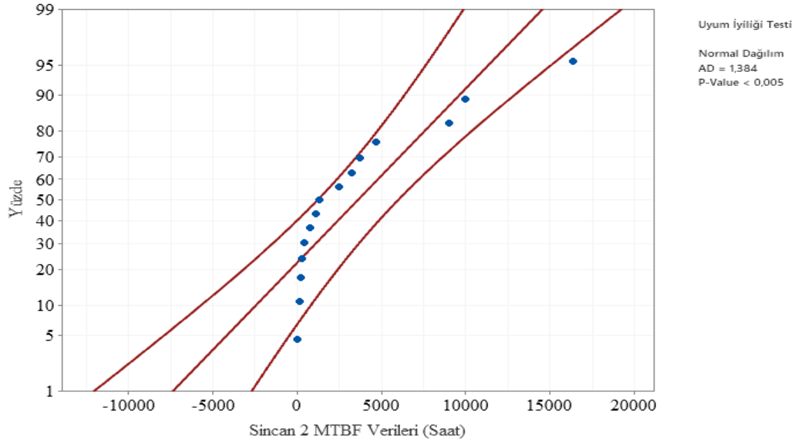
Şekil 6.46. Sincan 2 Fideri normal dağılım Anderson- Darling uyumluluk eğrisi
