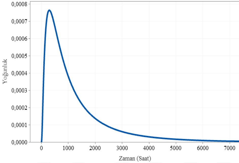
Şekil 6.122. Keban Güney fideri olasılık yoğunluk fonksiyonu eğrisi
