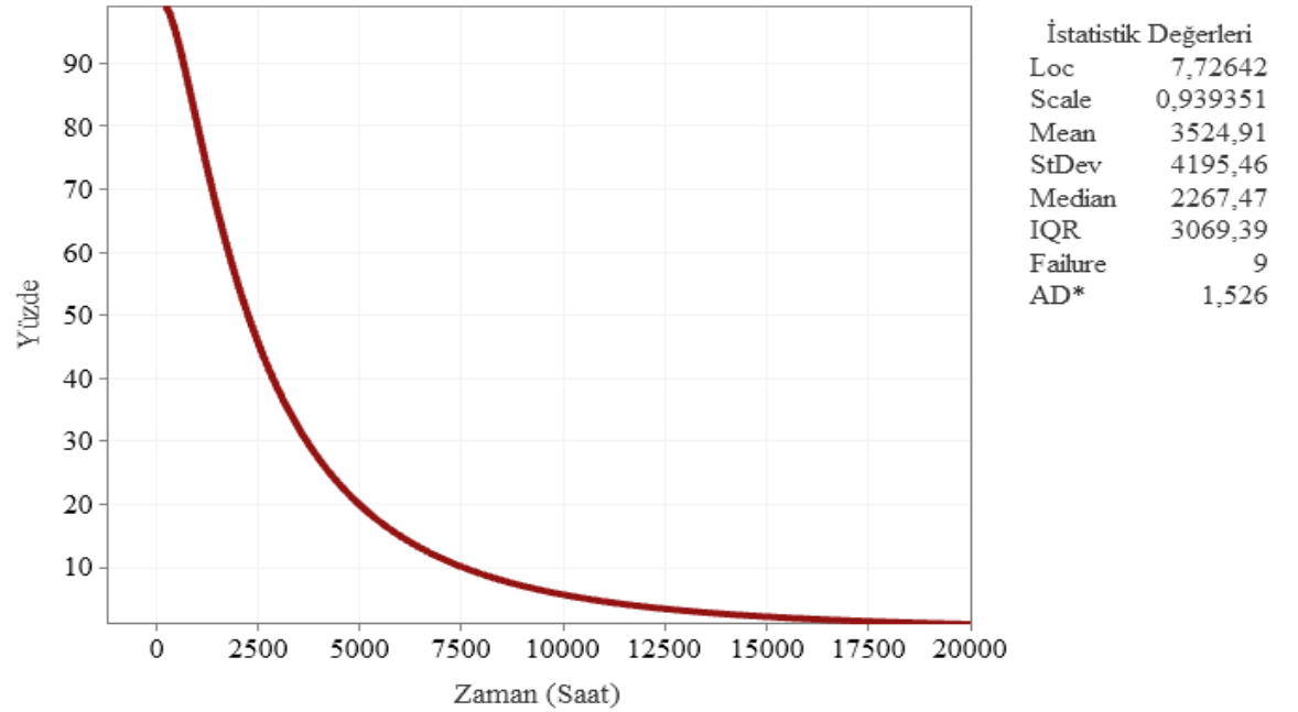
Şekil 6.87. Kozan 1 fideri güvenilirlik fonksiyonu eğrisi
