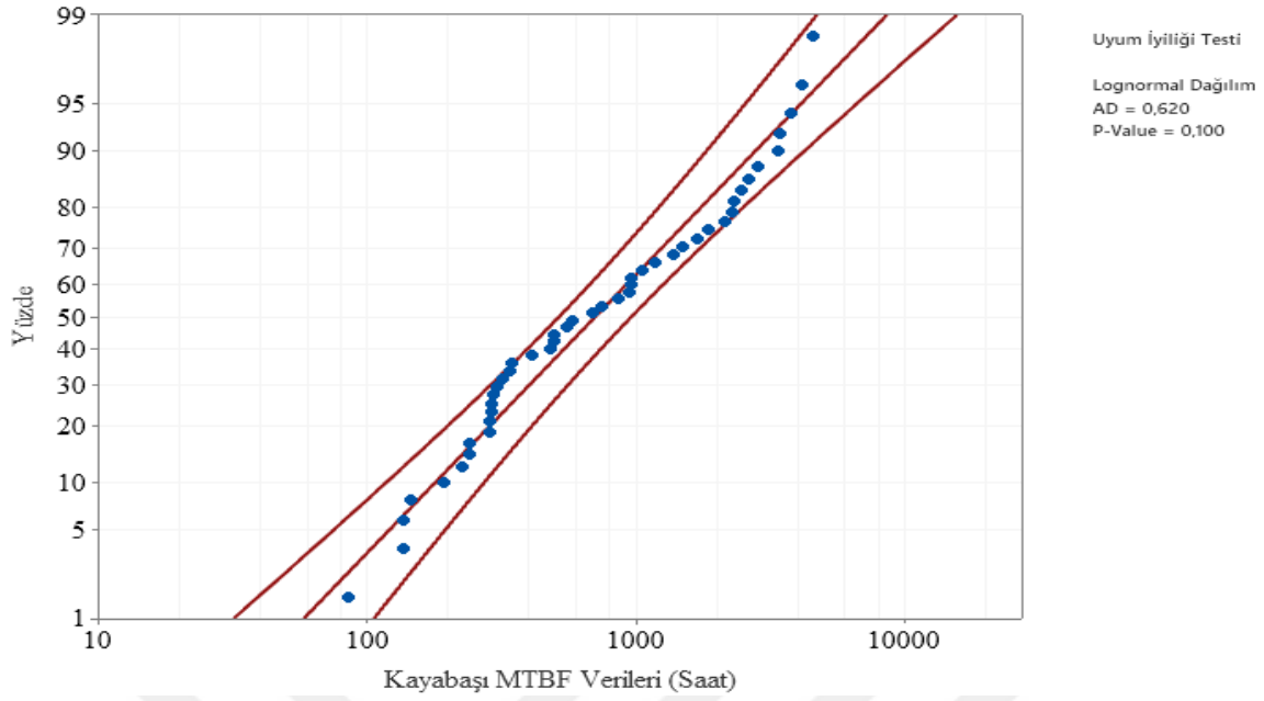
Şekil 6.77. Kayabaşı Fideri lognormal dağılımı Anderson- Darling uyumluluk eğrisi
