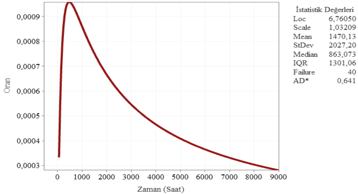
Şekil 6.121. Keban Güney fideri tehlike fonksiyonu eğrisi
