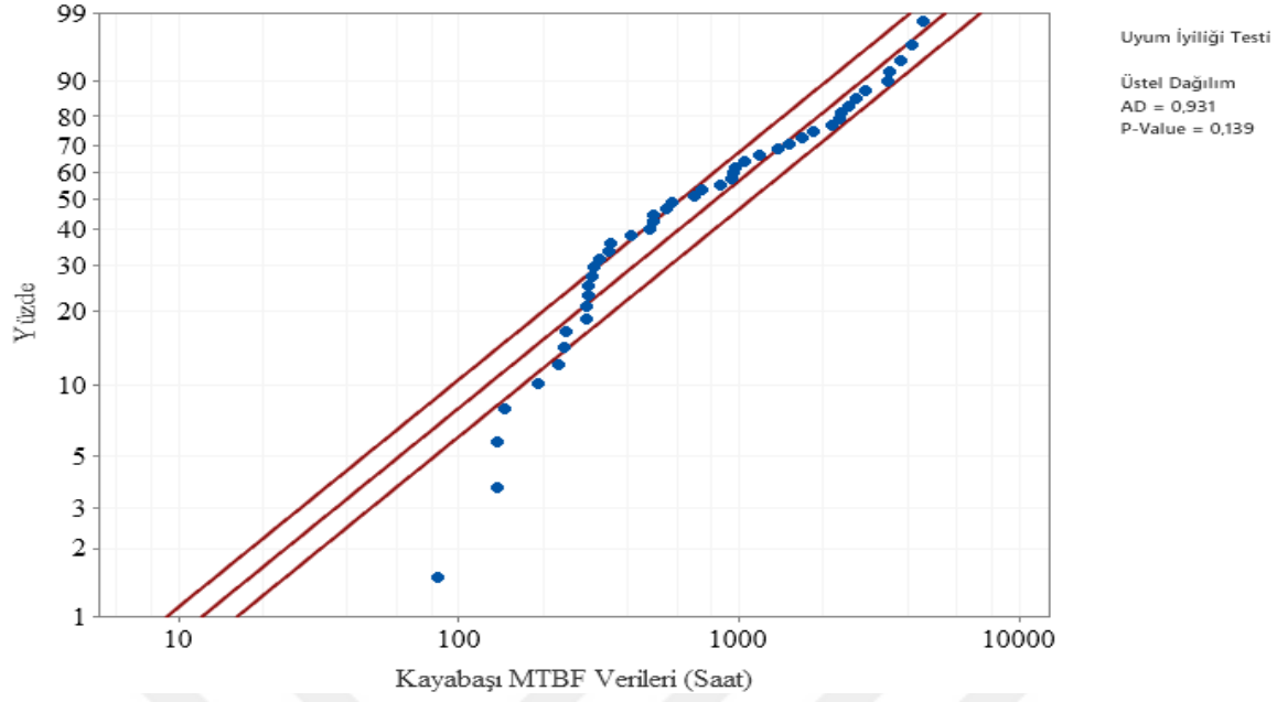
Şekil 6.75. Kayabaşı Fideri üstel dağılım Anderson- Darling uyumluluk eğrisi
