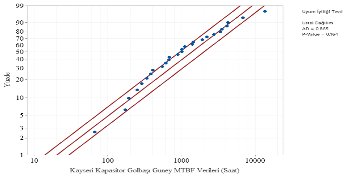
Şekil 6.55. Gölbaşı Güney Fideri üstel dağılım Anderson- Darling uyumluluk eğrisi
