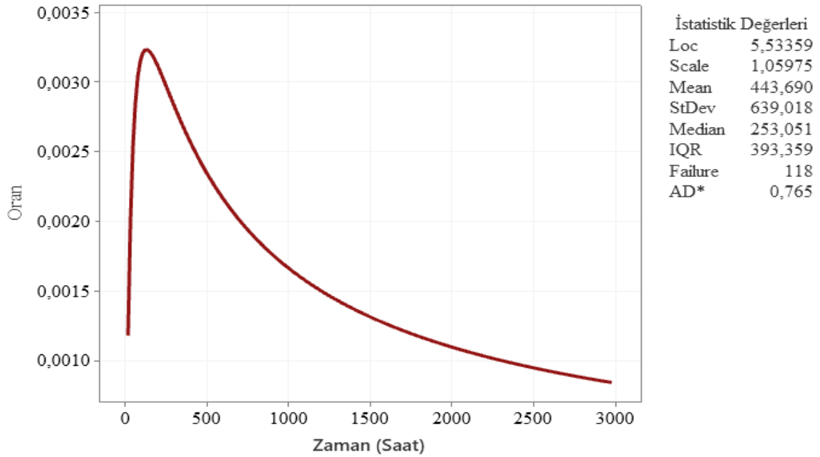
Şekil 6.94. Konya4 fideri tehlike fonksiyonu eğrisi
