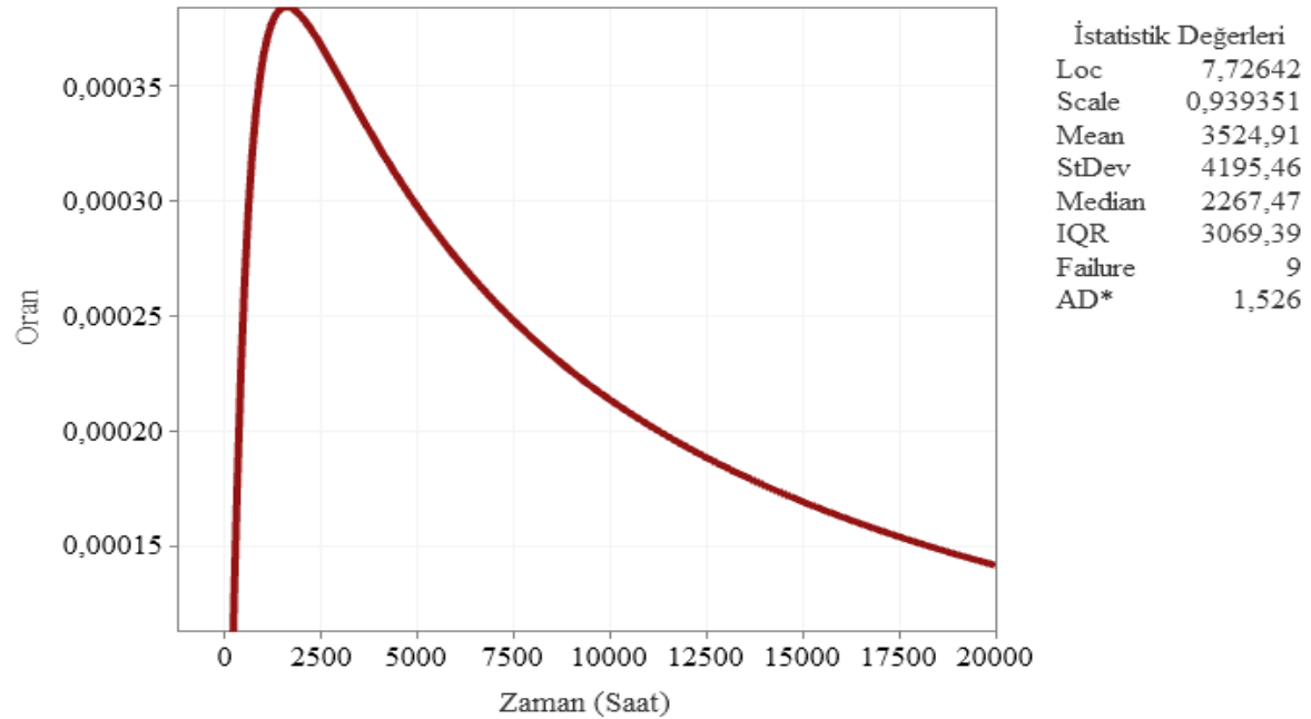
Şekil 6.88. Kozan 1 fideri tehlike fonksiyonu eğrisi
