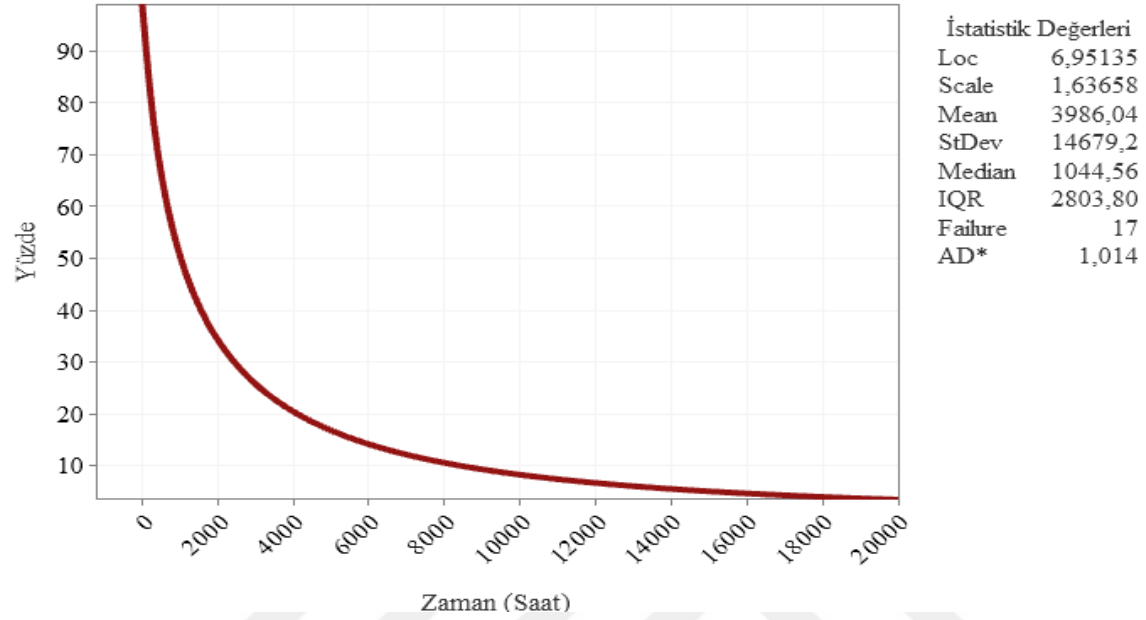
Şekil 6.108. Sincan 1 fideri güvenilirlik fonksiyonu eğrisi
