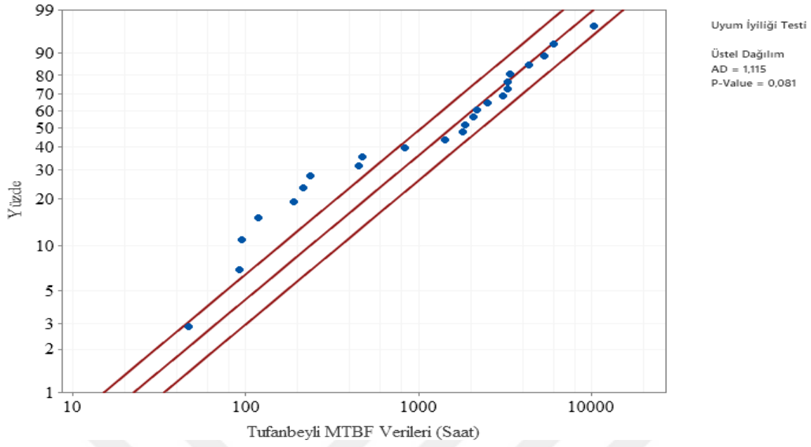
Şekil 6.11. Tufanbeyli Fideri üstel dağılım Anderson- Darling uyumluluk eğrisi
