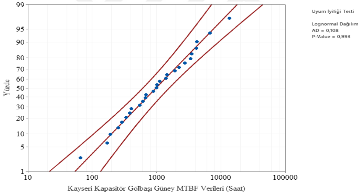
Şekil 6.57. Gölbaşı Güney Fideri lognormal dağılımı Anderson- Darling uyumluluk eğrisi
