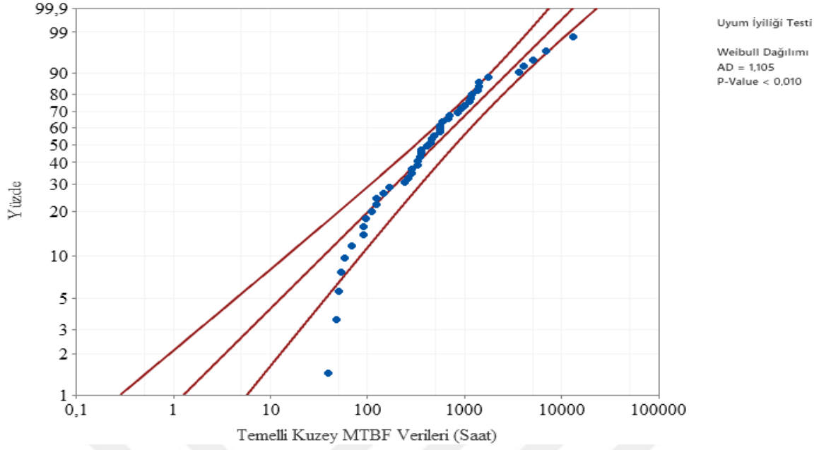
Şekil 6.32. Temelli Kuzey Fideri weibull dağılımı Anderson- Darling uyumluluk eğrisi
