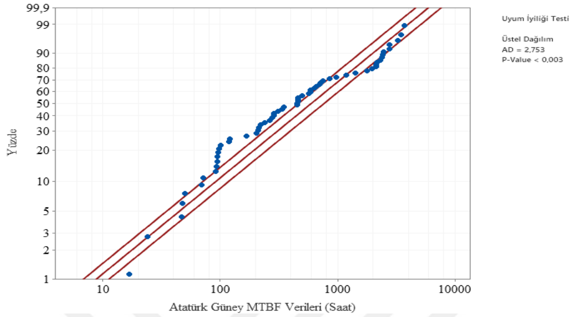
Şekil 6.3. Atatürk Güney Fideri üstel dağılım Anderson- Darling uyumluluk eğrisi
