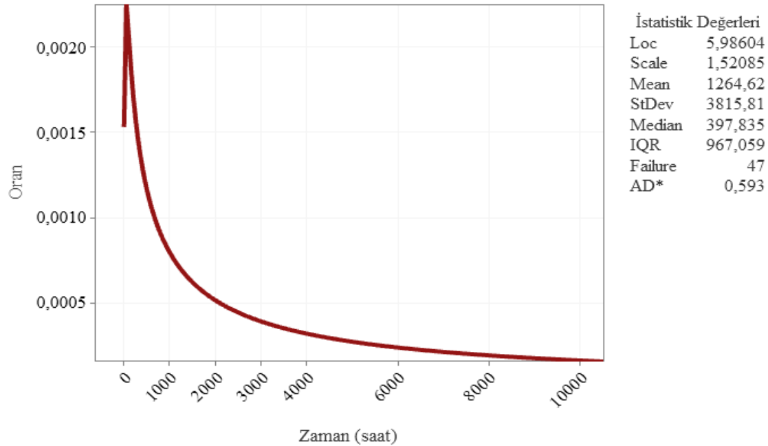
Şekil 6.97. Temelli Güney fideri tehlike fonksiyonu eğrisi
