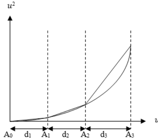
Şekil 4.15. Parçalı doğrusallaştırma
