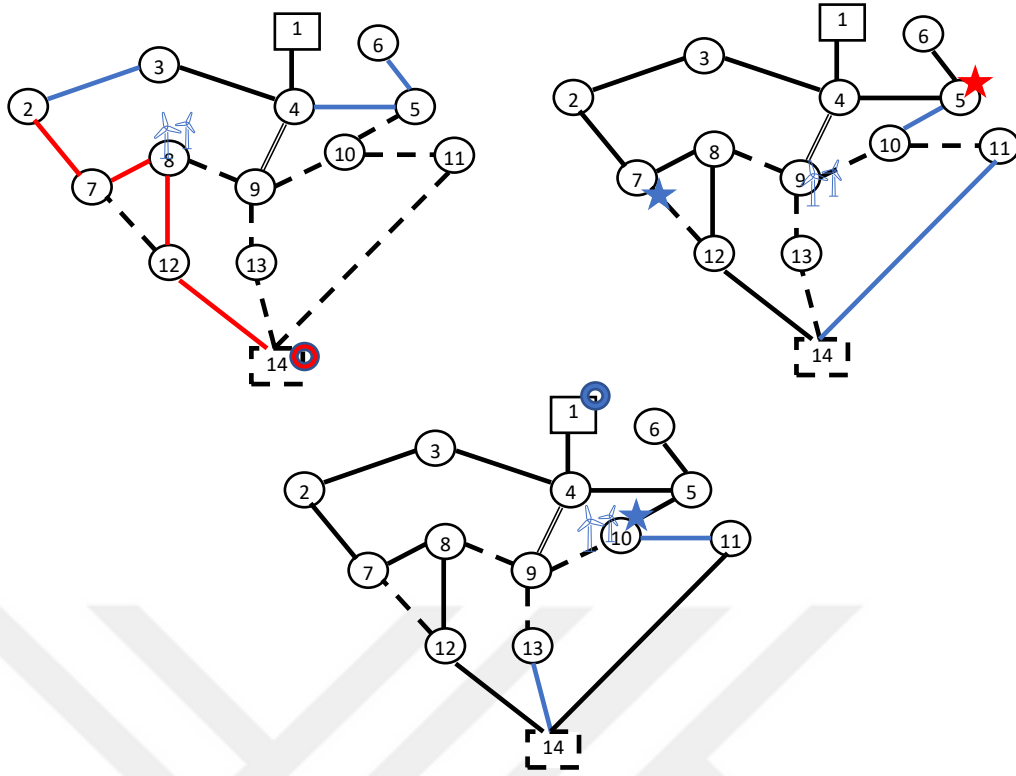
Şekil 4.16. 2 ve 6 numaralı düğümün güvenilirlik kısıtı içermesi durumunda genişleme planı
