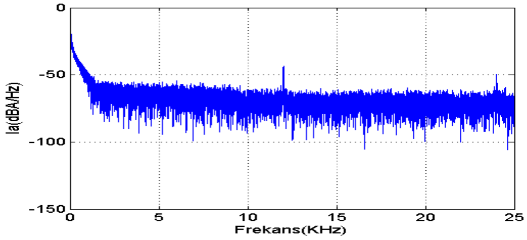
b) Şekil 8.9 Ia (stator akımı) güç spektral yoğunluğu (PSD) a) RAS-YRDKM (rastgele sinyal) b) KAO-YRDKM (kaotik sinyal)
