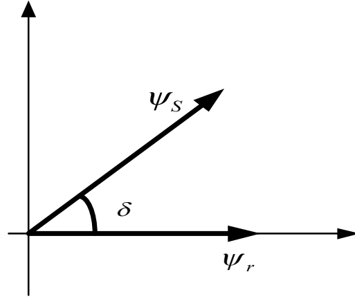
Şekil 5.1 DMK yönteminde stator akısı ile rotor akısı konumu
