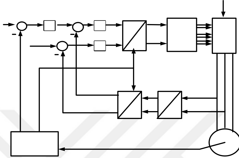
Şekil 7.2 KSDGM modülasyonlu vektör kontrol blok diyagramı
