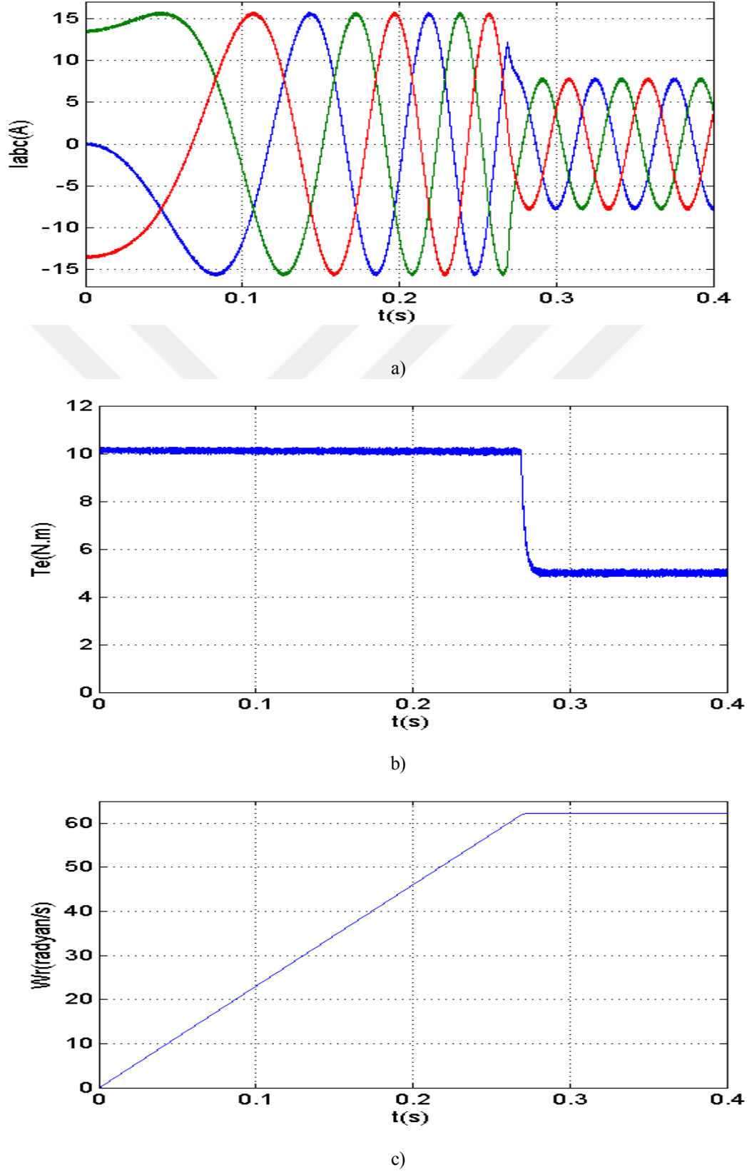
Şekil 7.3 Klasik SDGM a) stator akımları b)moment c) motor açısal hızı
