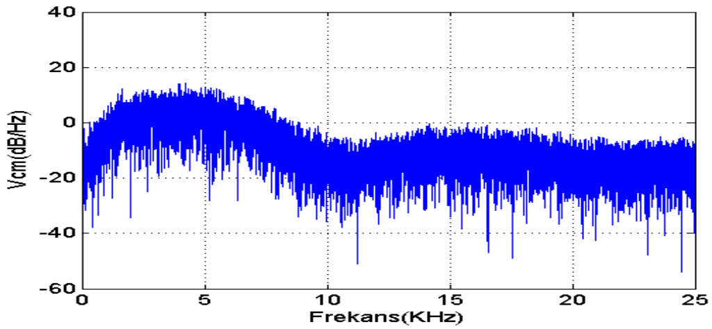
b) Şekil 8.10 V_{cm} (OMG) güç spektral yoğunluğu (PSD) a) RAS-YKDKM (rastgele sinyal) b) KAO-YKDKM (kaotik sinyal)
