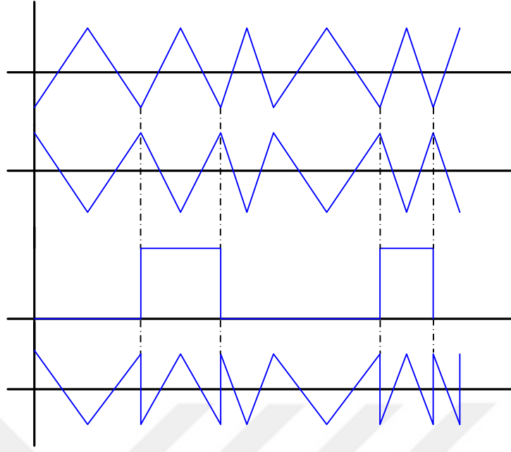
Şekil 8.16 KAO-KAM yönteminde a) taşıyıcı dalga b) taşıyıcı dalga tersi c) kaotik bit d) seçici çıkışındaki taşıyıcı dalga
