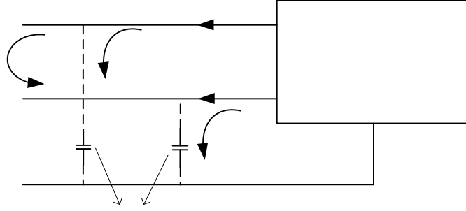
Şekil 4.1 Ortak mod ve fark mod iletim gürültüleri[2]
