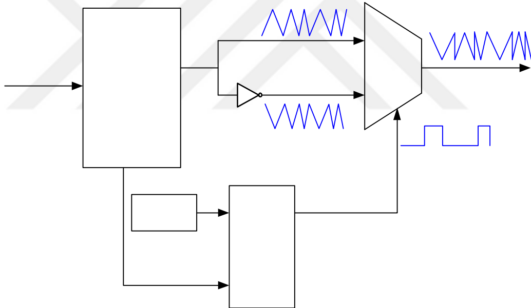
Şekil 8.15 KAO-KAM yöntemi prensip şeması
