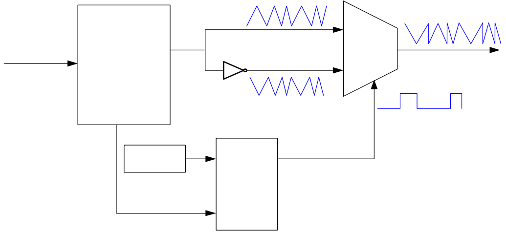
Şekil 8.13 KAO-RAM yöntemi prensip şeması
