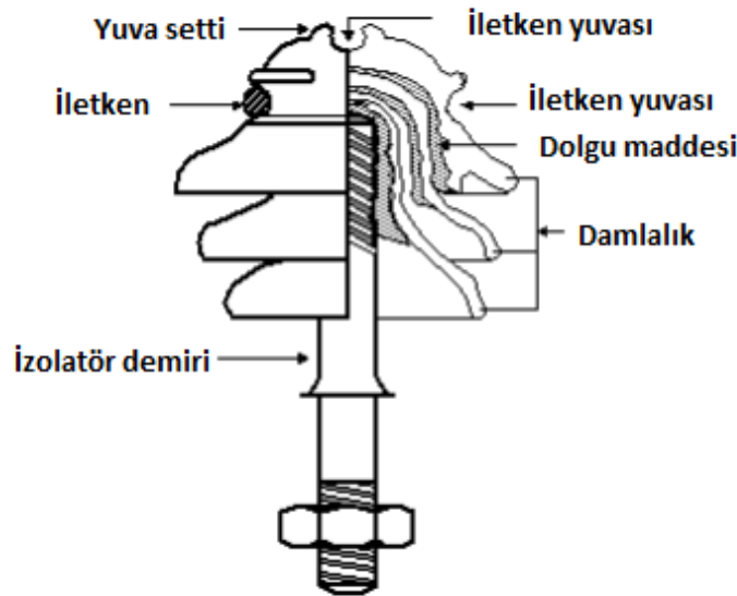
Şekil 3.7. İzolatör kısımları
