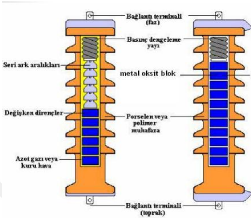
Şekil 3.9. Parafudr yapısı
