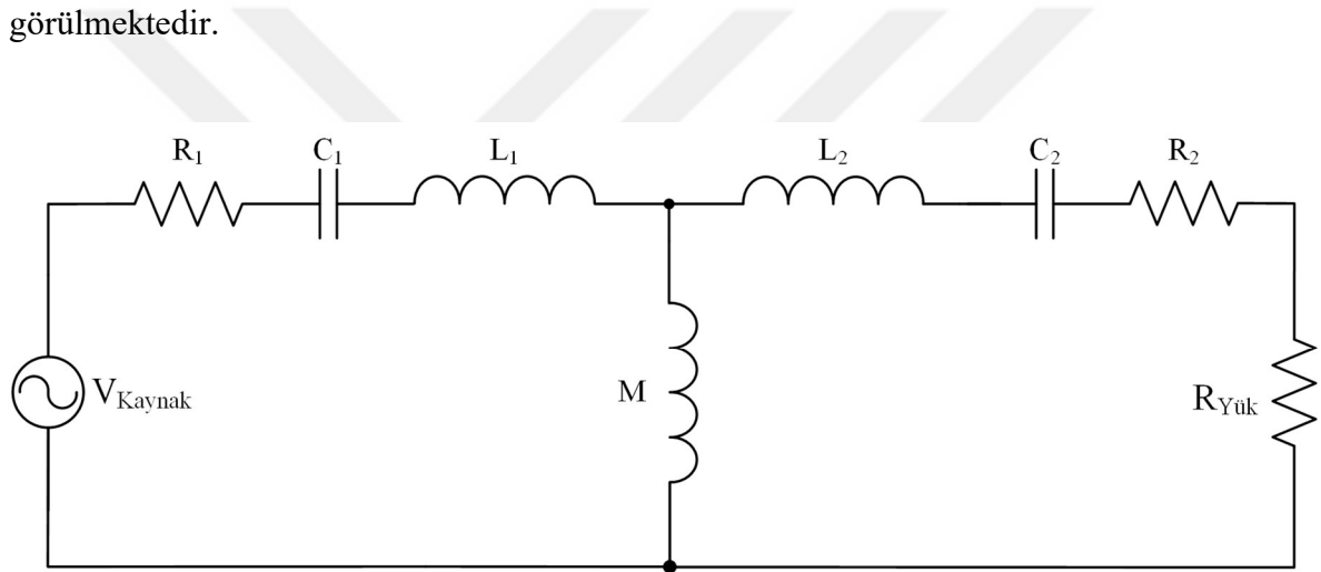
Şekil 3.2. MRKKA eşdeğer devresi
