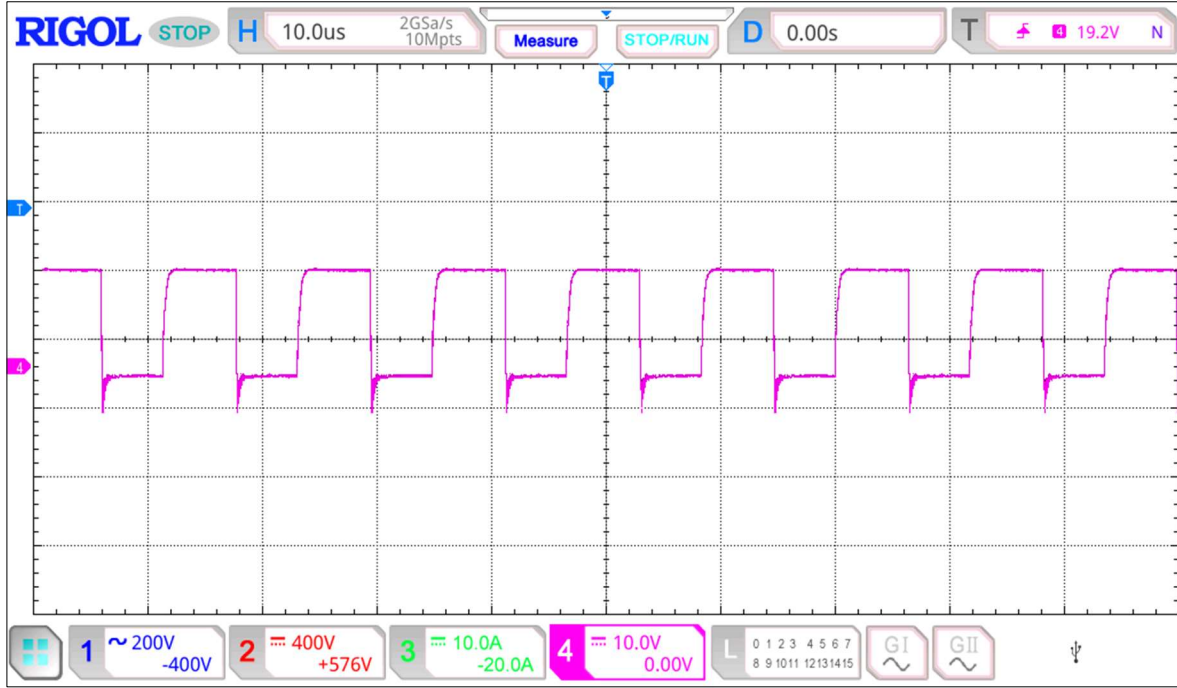
Şekil 4.10. MOSFET sürücü çıkış sinyali
