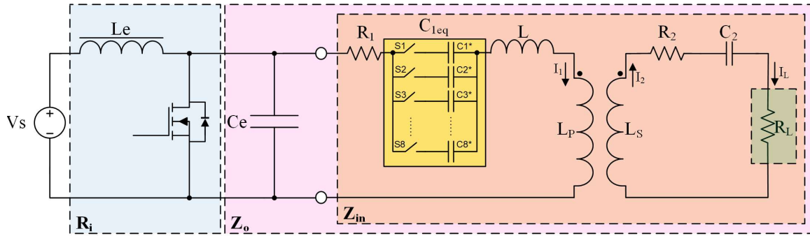
Şekil 4.6. Tümlleşik E-sınıfı evirici ve KGA sistemine ait devre topolojisi
