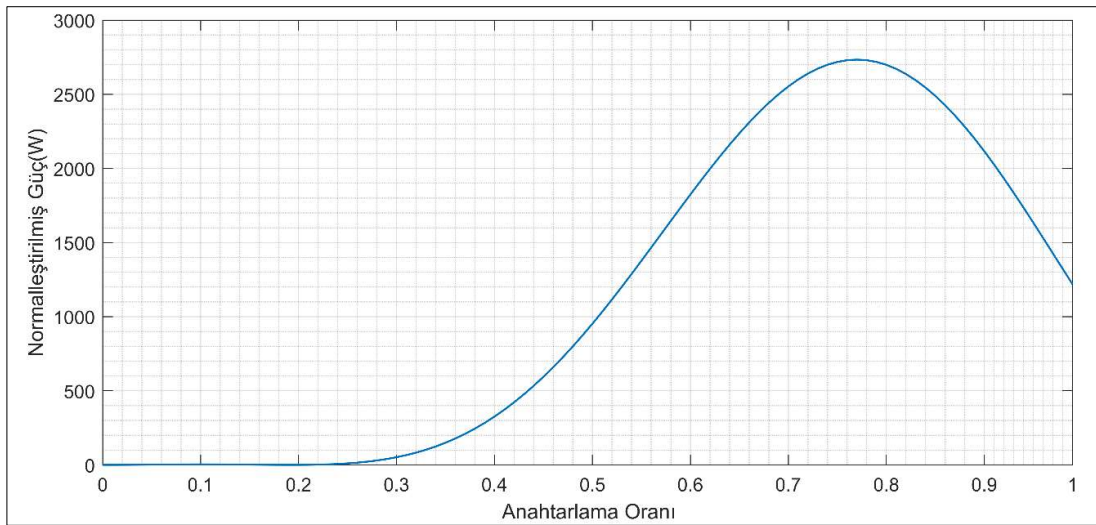
Şekil 4.14. Normalleştirilmiş güç ve anahtarlama doluluk oranı ilişkisi
