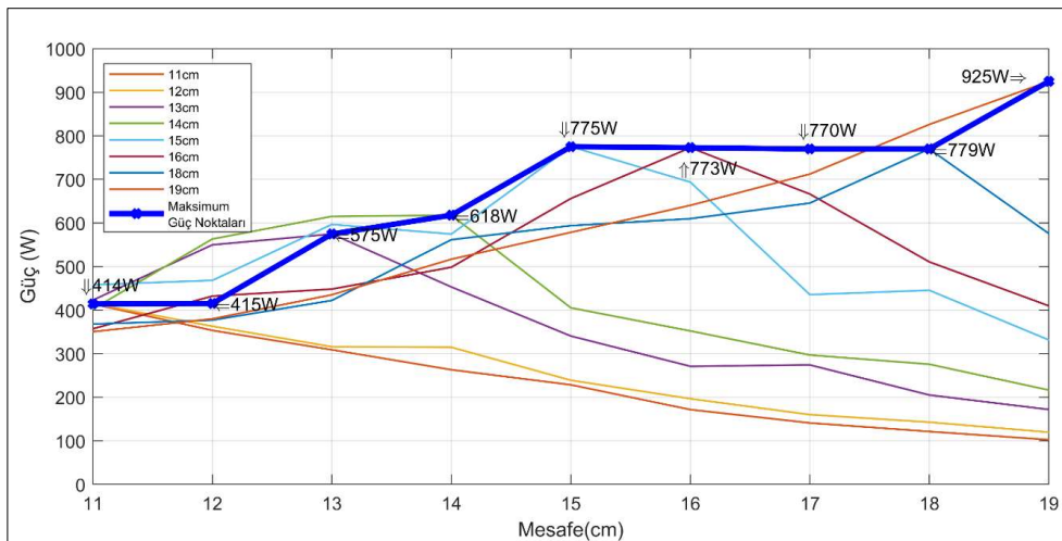
Şekil 7.42. 11-19 cm mesafe aralığında empedans uyumunun ve rezonans şartının sağlanması ile elde edilen güç değerleri
