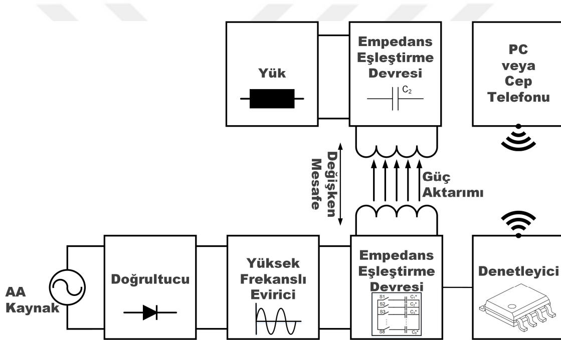
Şekil 5.7. Elektrikli aracın kablosuz şarjı için tasarlanan sisteme ait blok diyagramı
