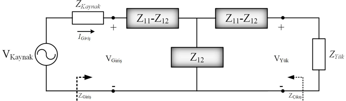
Şekil 5.5. Kablosuz enerji aktarım sistemi iki kapı eşdeğeri
