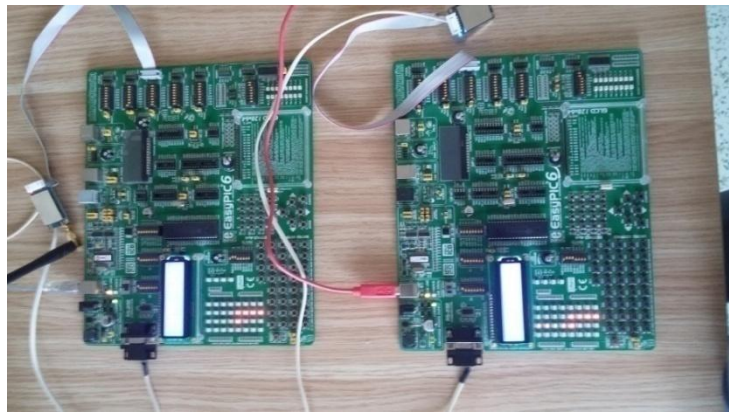
Resim 3.1 Mikro denetleyici tabanlı telemetry geliştirme bordu.
