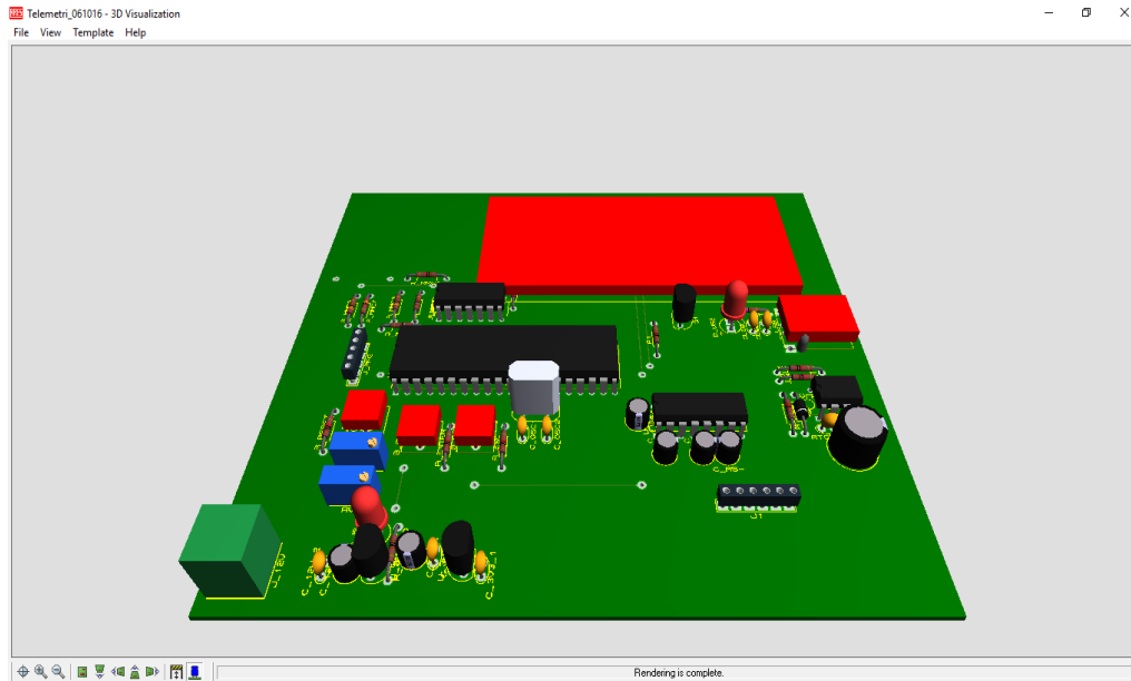
Şekil 3.6 Tasarlanan telemetry kartlarının üç boyutlu görünümü.
