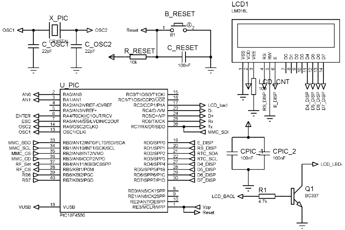
Şekil 3.3 Telemetry ana kart şeması.
