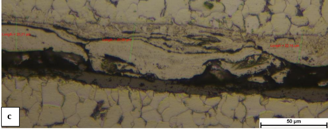
Resim 4.5 (Devam) c) 6'ncı Numune 160 V 890 Hz 500x Büyütme Mikroyapısı.
