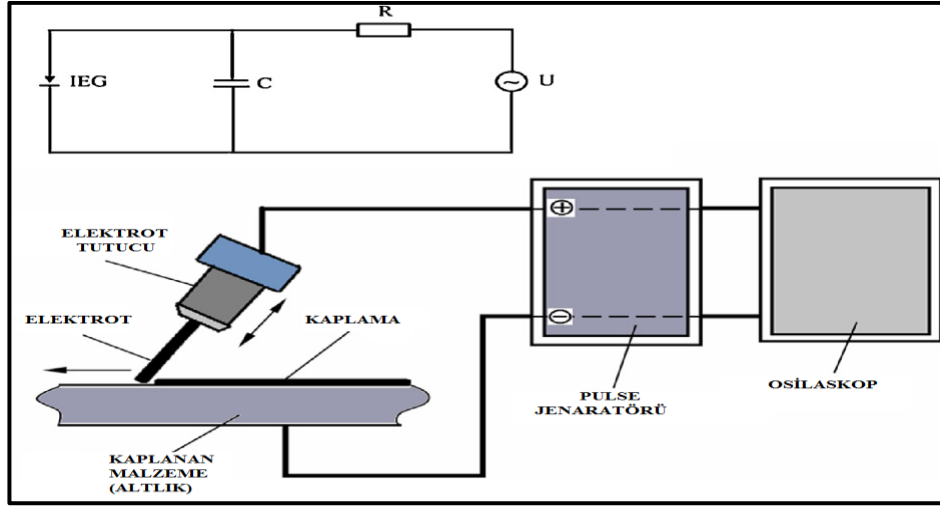
Şekil 2.2 ESD Kaplama Sisteminin Şematik Gösterimi (Bozkurt 2018).
