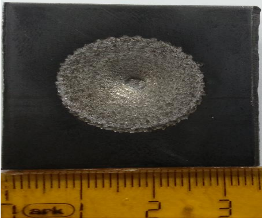
Resim 4.18 AISI 1008 Çeliği Üzerine Alaşımli Çelik Kaplama Serbest Deformasyon İzi.
