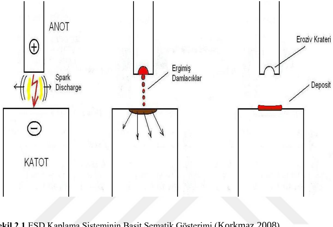
Şekil 2.1 ESD Kaplama Sisteminin Basit Şematik Gösterimi (Korkmaz 2008).
