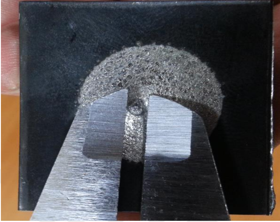
Resim 4.21 AISI 1008 Çeliği Kaplama Yüzeyi Serbest Deformasyon İndent Genişliği.
