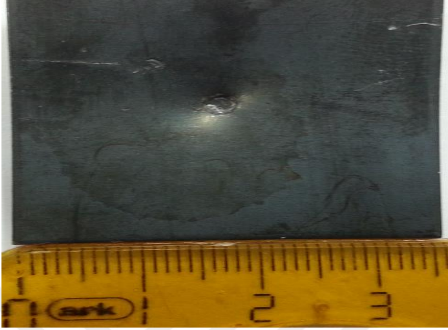
Resim 4.17 AISI 1008 Çeliği Üzerine Kaplamasız Serbest Deformasyon İzi.
