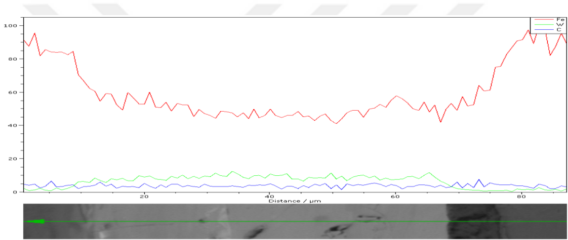
Şekil 4.12 Yüzeyi 160V ve 890 Hz ile Tungsten Karbür ile Kaplanan Alaşımının Çizgi Analizi.
