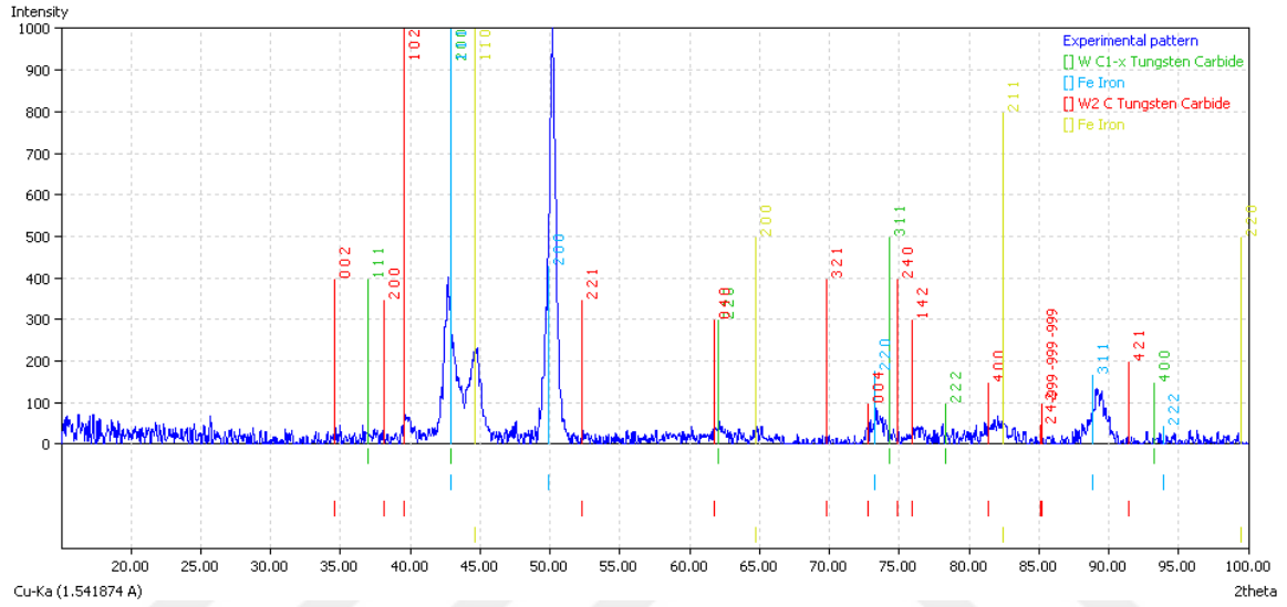
Şekil 4.10 Yüzeyi 160V ve 890 Hz ile Tungsten Karbür Kaplanan Alaşımın XRD Sonucu.
