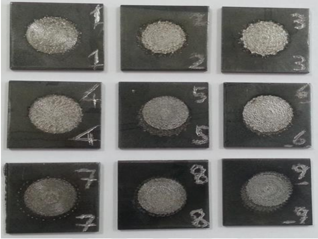
Resim 4.2 Yüzeyleri Alaşımlı Çelik ile Kaplanan Numuneler.
