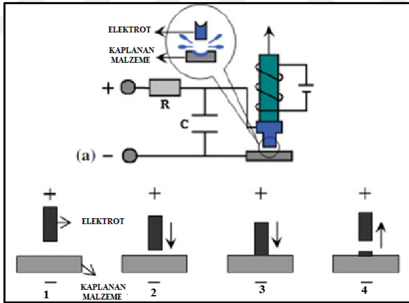
Şekil 2.3 ESD Prosesinin Kapanmak İstenen Malzemeye Parça Bırakımı (Bozkurt 2018).
