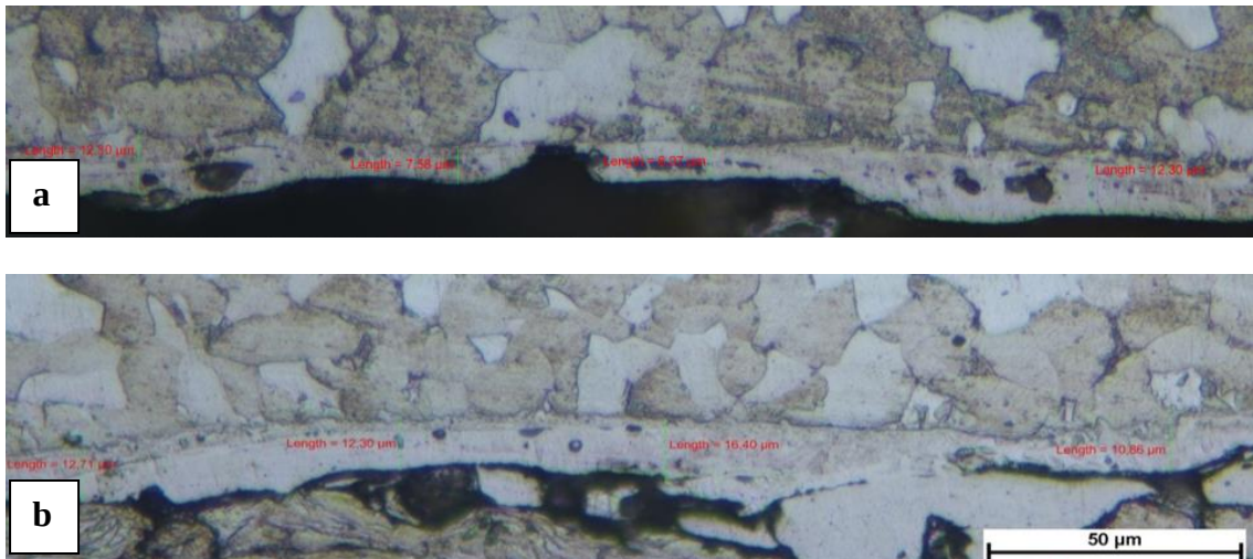
Resim 4.10 a) Alaşımlı Çelik Kaplama 1’inci Numune 48 V 210 Hz, b) 2’nci Numune 104 V 210 Hz 500x Büyütme Mikroyapıları.
