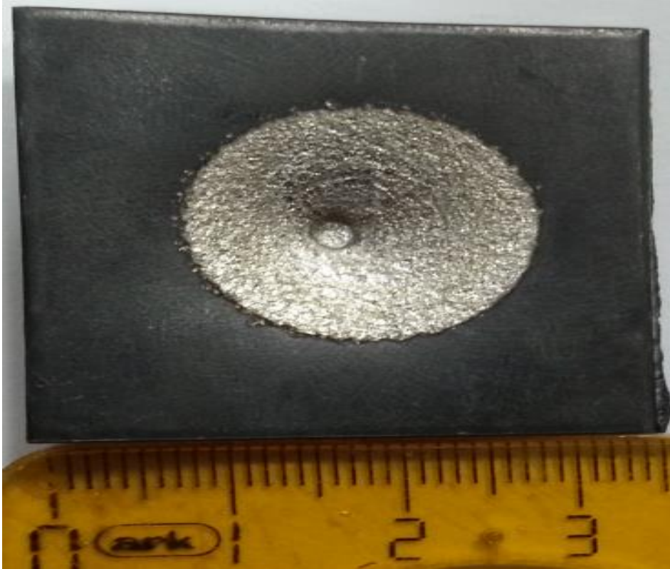
Resim 4.20 AISI 1008 Çeliği Üzerine WC Kaplama Serbest Deformasyon İzi.
