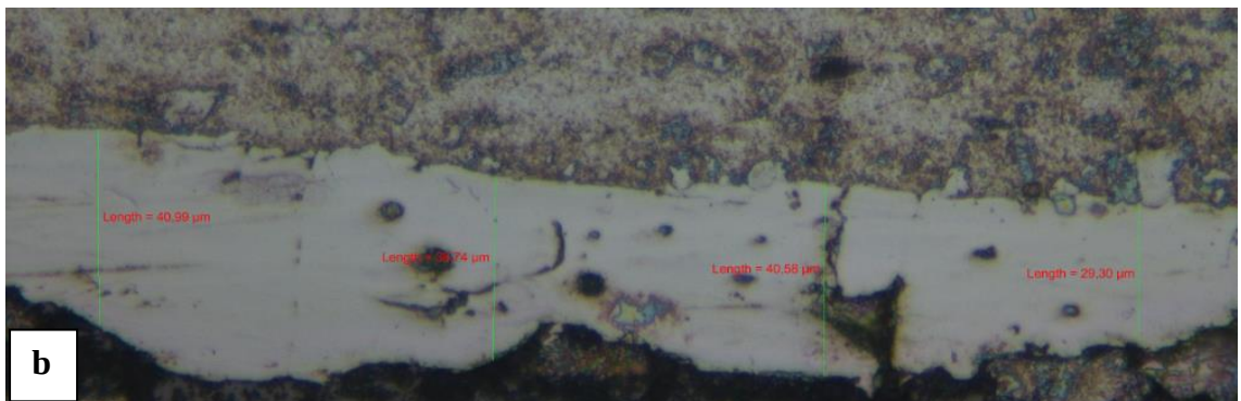
Resim 4.9 a) Tungsten Karbür(WC) Kaplama 7'nci Numune 48 V 1570 Hz, b) 8'inci Numune 104 V 1570 Hz 500x Büyütme Mikroyapıları.
