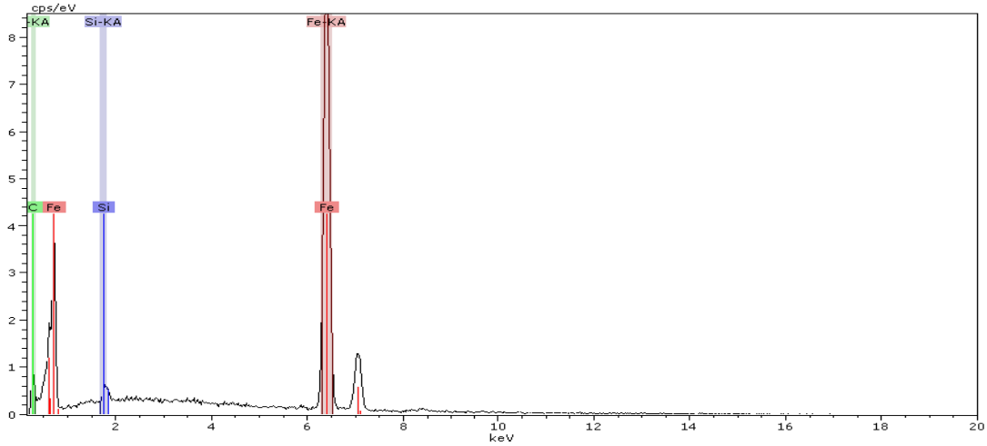
Şekil 4.5 Yüzeyi 160V ve 1570 Hz ile Alaşımlı Çelik Kaplamanın EDX Sonucu.
