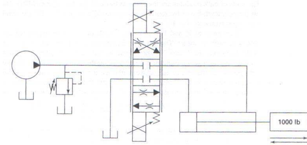
Şekil 5.47 Örnek devre (Norvelle, 2000)
