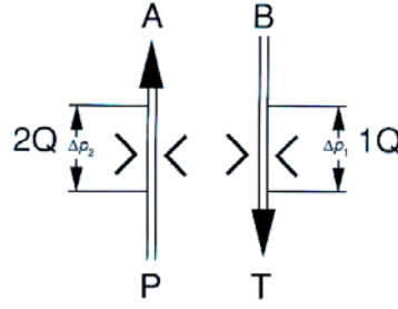
Şekil 3.22 E1 sürgüsü içindeki kısma noktalarını
