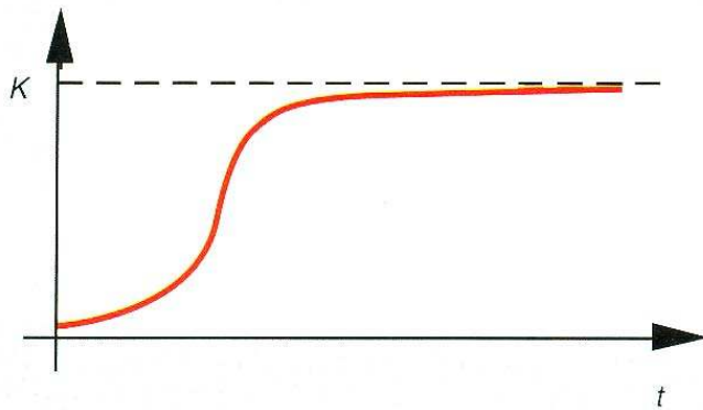
Şekil 5.22 D > 1 için ikinci dereceli orantı elemanının step giriş cevabı
