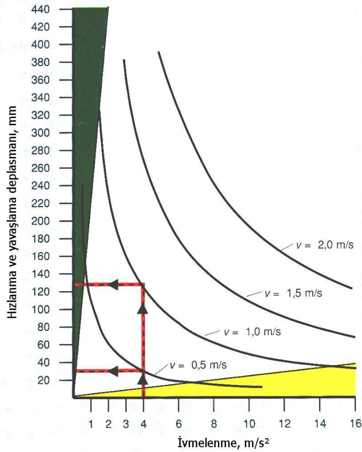
Şekil 5.28 Sabit ivmede hızlanma ve yavaşlama deplasmanı (Rexroth, 1989)
