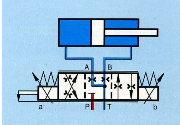
Şekil 3.24 W sürgülü oransal valf ile kontrol edilen silindir (Rexroth, 1989)
