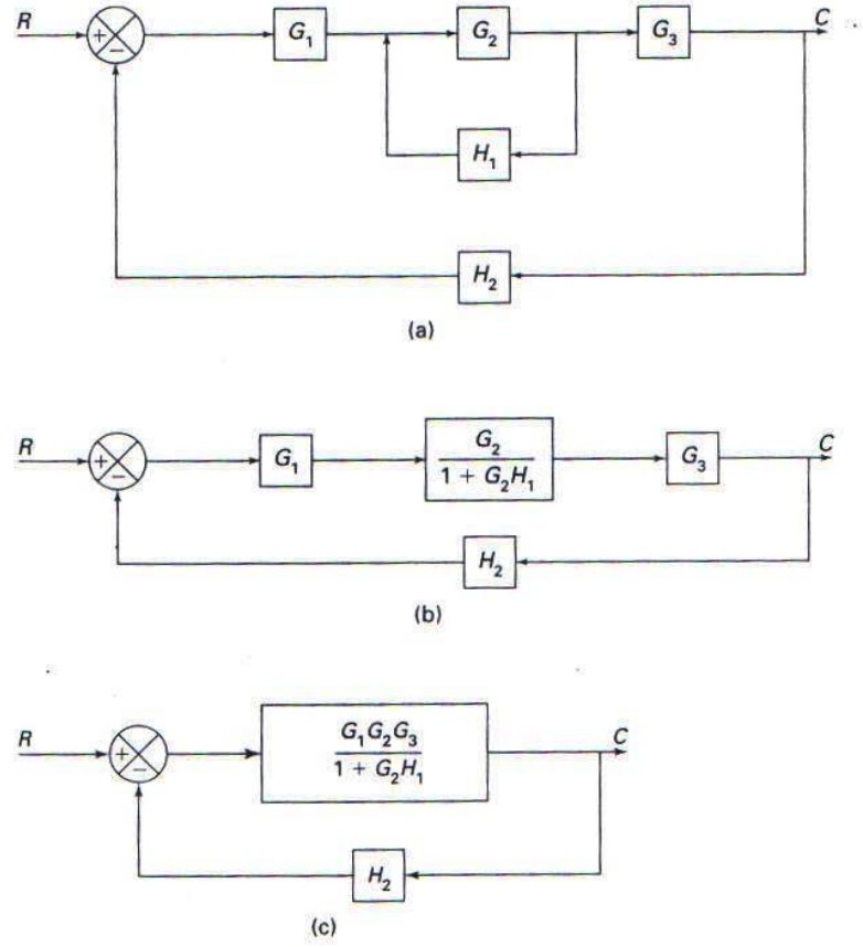
Şekil 5.10 Çoklu geri beslemeli sistemin blok diyagramı
