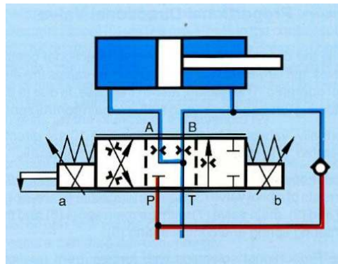
Şekil 3.25 W3 sürgülü oransal valf ile kontrol edilen silindir (Rexroth, 1989)
