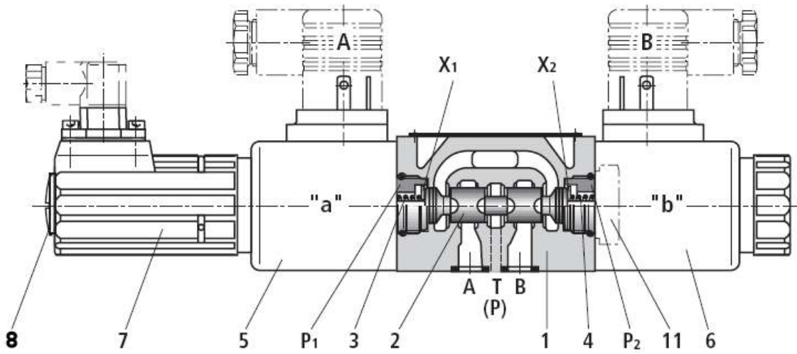
Şekil 3.7 Direk uyarılı oransal yön kontrol valfi
