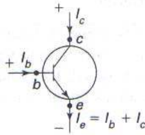
Şekil 5.14 Transistorun sembolik gösterimi
