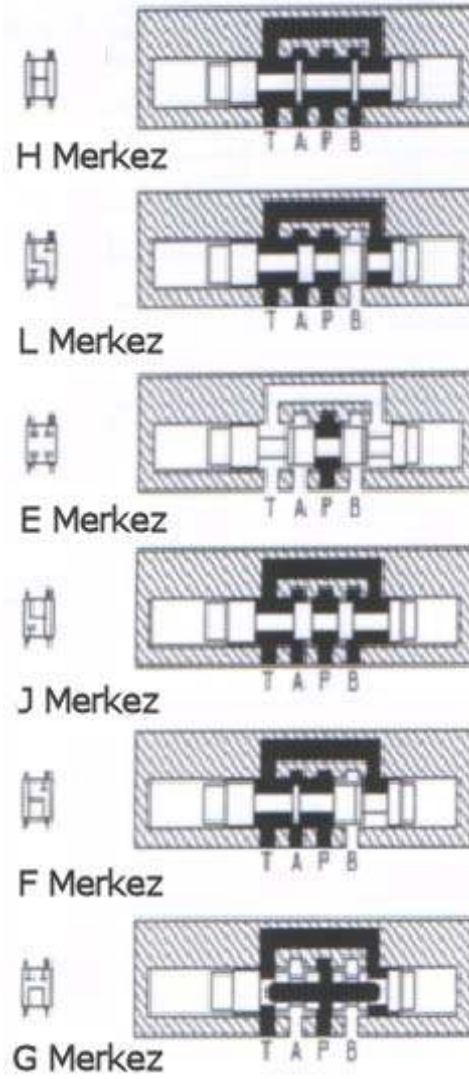
Şekil 3.6 Sürgü Tipleri (Johnson 2000)
