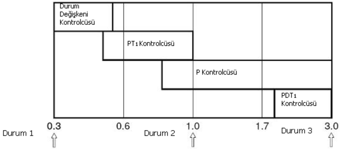
Şekil 5.50 Silindir ve valfin doğal frekans oranlarına göre kontrolcü tipi
