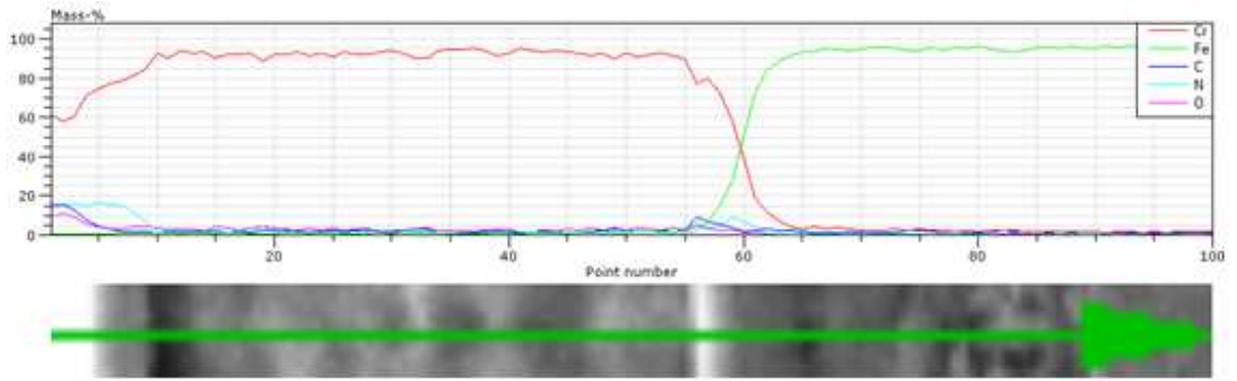
Şekil 6.18 600 °C’ de plazma nitrüleme işlemine tabi tutulan krom kaplanmış AISI 1040 çeliğinin mikroyapı görüntüsü ve Çizgi Tarama (Line Scan) analizi
