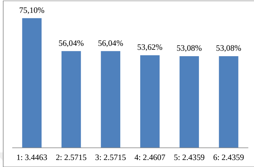
Şekil 32. Dosyalama
