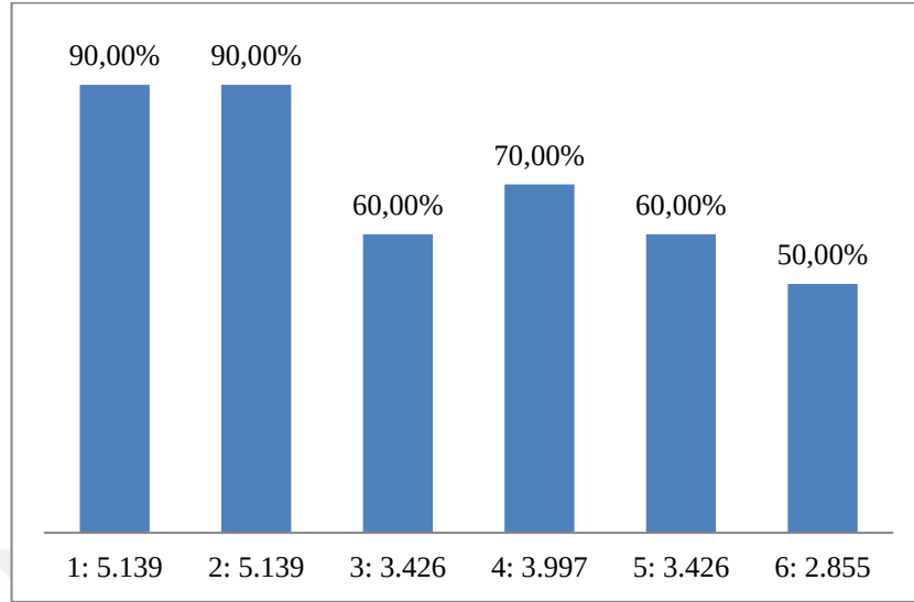
Şekil 36. Log Kayıtları
