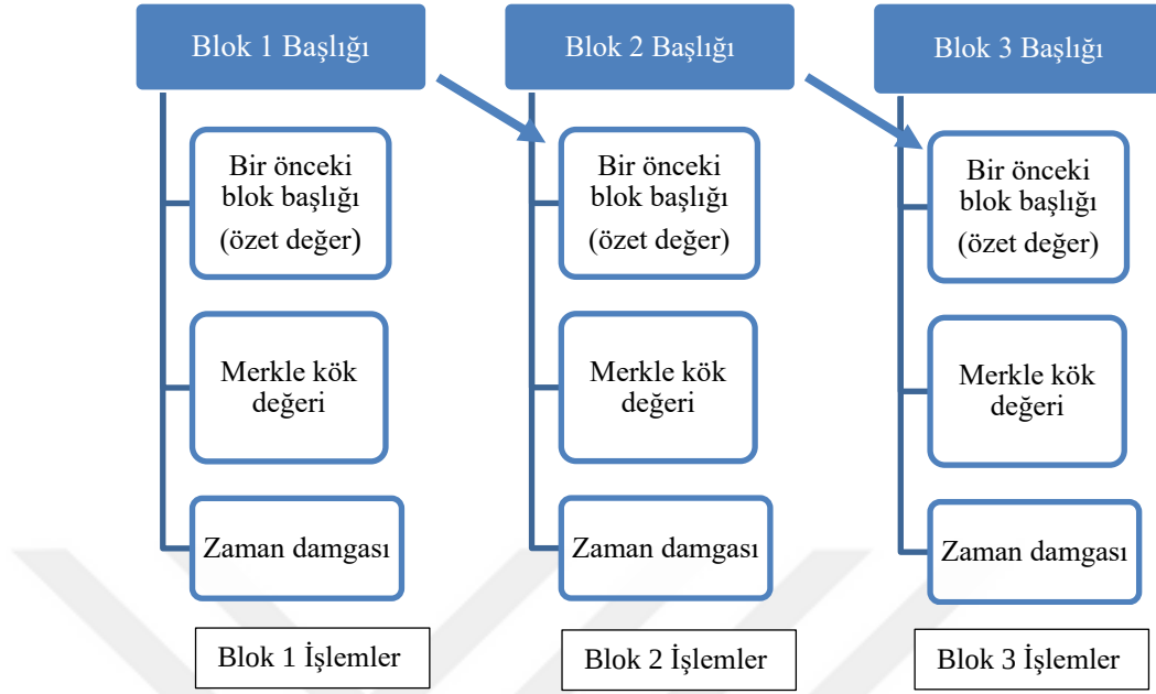
Şekil 4. Blok Yapısı
