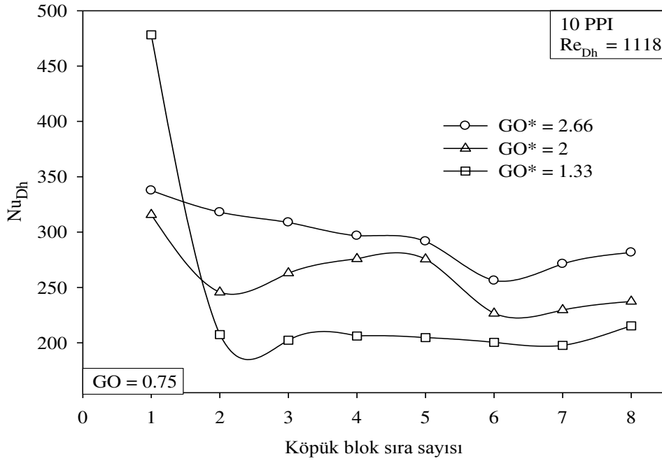
Şekil 4.29. Re_{Dh} = 1118 , GO = 0.75 ve 10 PPI'da laminar akış şartlarında kanal yüksekliğine bağlı olarak köpük blok sıra sayısına göre ortalama Nusselt dağılımı
