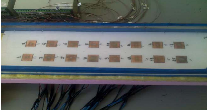
Şekil 3.4. Bakır plakaların teflon malzemeye montajı
