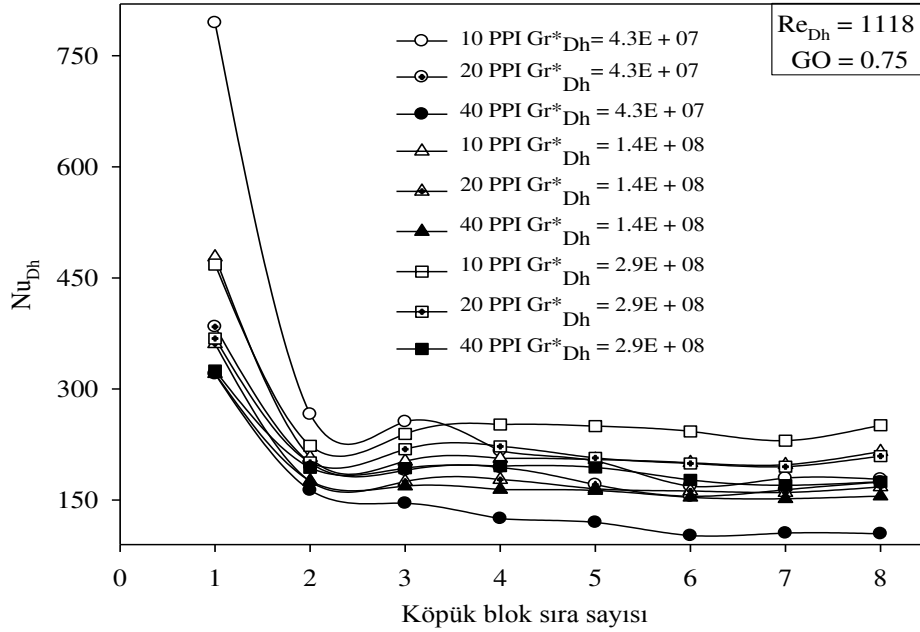
Şekil 4.8. Re_{Dh} = 1118 ve GO = 0.75 'te laminar akış şartlarında farklı gözenek yoğunluğuna ve Gr_{Dh}^* sayısına sahip alüminyum köpüklerin blok sıra sayısına göre Nu_{Dh} değişimi
