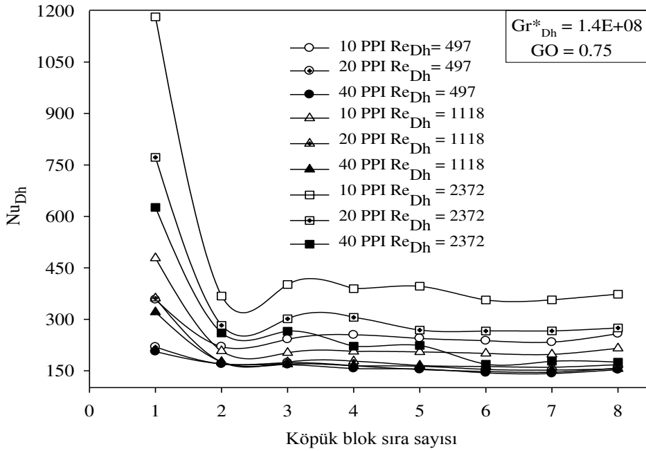
Şekil 4.7. Gr_{Dh}^* = 1.4E+08 ve GO = 0.75 'te laminar akış şartlarında farklı gözenek yoğunluğuna ve Re_{Dh} sayısına sahip alüminyum köpüklerin blok sıra sayısına göre Nu_{Dh} değişimi
