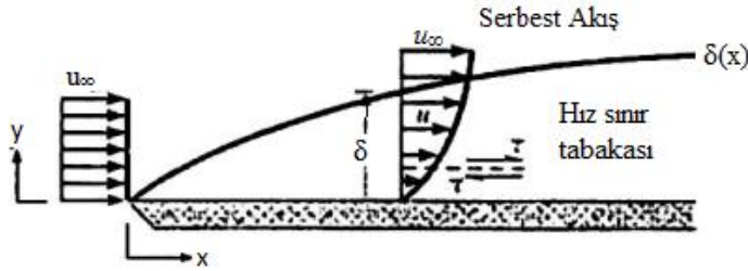
Şekil 2.1. Düzlem levha üzerinde hız (hidrodinamik) sınır tabakanın gelişimi (Incropera ve DeWitt 2006)
