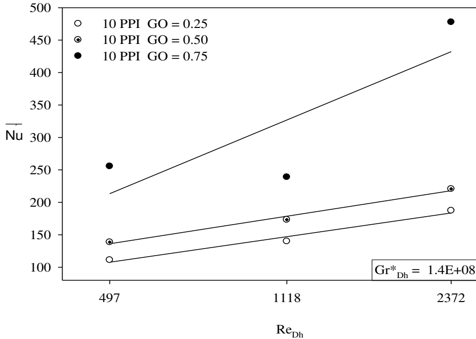
Şekil 4.20. Gr_{Dh}^* = 1.4E+08 ve 10 PPI’da laminar akış şartlarında geometrik orana bağlı olarak köpük blok sıra sayısına göre ortalama Nusselt değişimi
