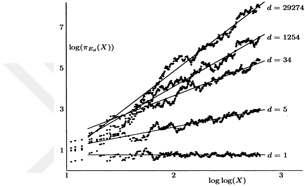
Şekil 6.1. Belli d değerleri için y^2 = x^3 - d^2x için Birch ve Swinnerton-Dyer datası.
