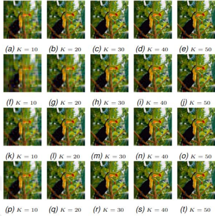
Şekil 5.11 Test görüntülerinin seçilmiş kısmı toplamları (Ayrılabilir metod: a-e, QSVD: f-j, RBSVD: k-o ve ESVD: p-t).
