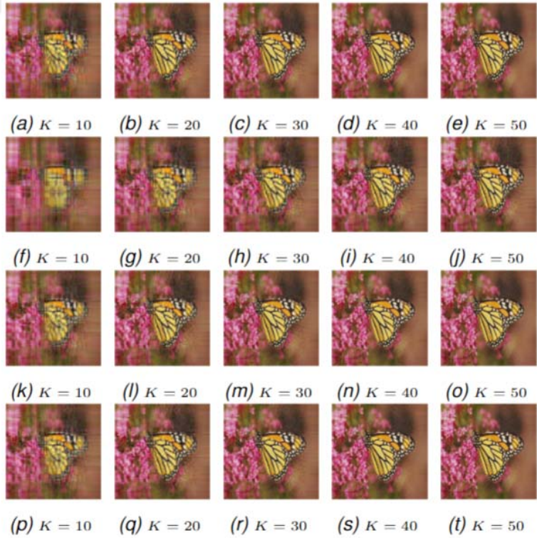
Şekil 5.12 Test görüntülerinin seçilmiş kısmı toplamları (Ayrılabilir metod: a-e, QSVD: f-j, RBSVD: k-o ve ESVD: p-t).
