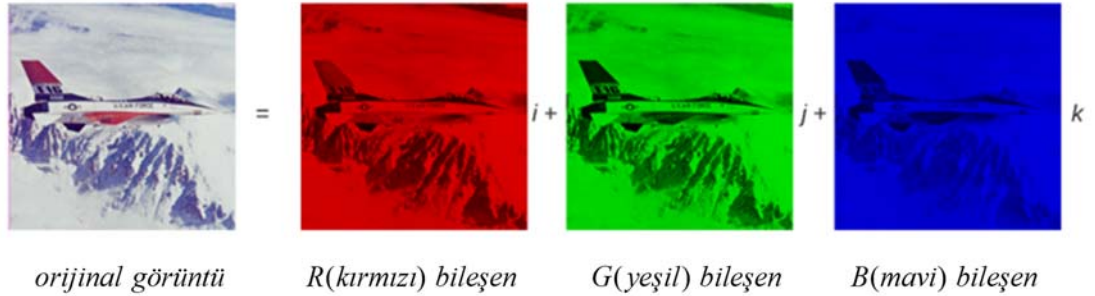
Şekil 5.1 Renkli görüntünün eliptik kuaterniyon matris gösterimi.
