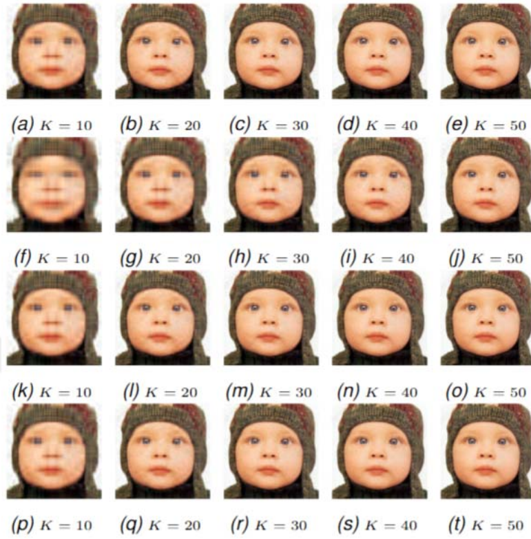
Şekil 5.8 Test görüntülerinin seçilmiş kısmi toplamaları (Ayrılabilir metod: a-e, QSVD: f-j, RBSVD: k-o ve ESVD: p-t).
