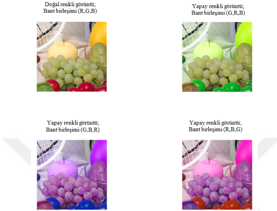
Şekil 2.4 RGB uzayında elde edilmiş yapay renkli görüntüler.
