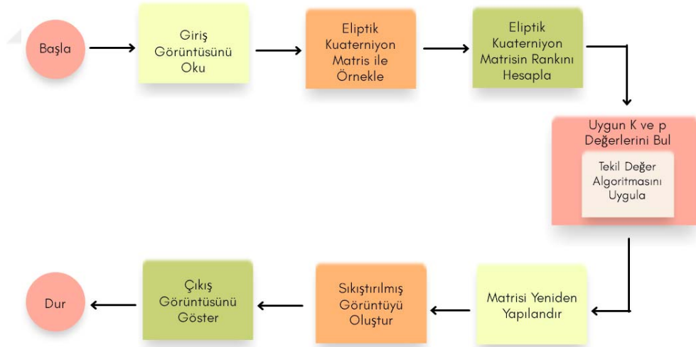
Şekil 5.4 ESVD ile görüntü sıkıştırma adımları.
