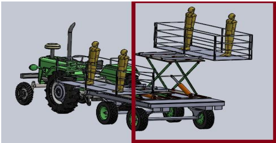
Şekil 4.20. Hidrolik silindirin sistemdeki konumuna ilişkin bir görüntü
