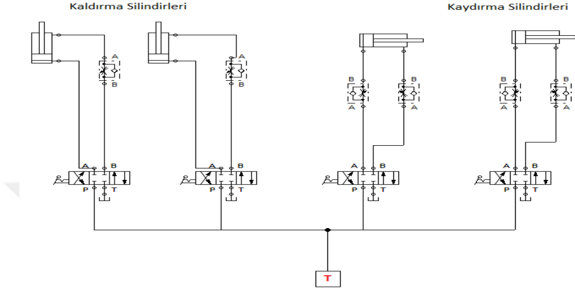
Şekil 4.18. Hidrolik devre tasarımının şematik görünümü
