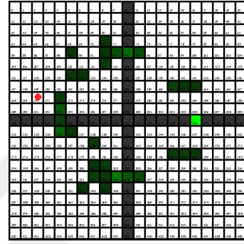
(d) EMDD-RL result on STEPPOSITIVE
