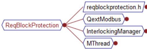
řekil 5.5 : Ray devresi koruma talebi sınıf statik baęımlılık grafięi.
