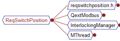
řekil 5.3 : Makas pozisyon deęiřtirme talebi sınıf statik baęımlılık grafięi.
