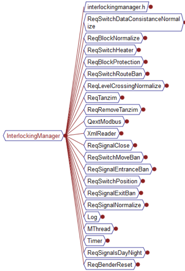
Şekil 5.1 : InterlockingManager sınıf statik bağımlılık grafiği.
