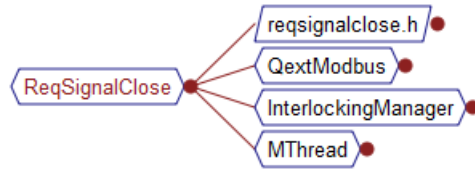
řekil 5.4 : Sinyal kapama talebi sınıf statik baęımlılık grafięi.
