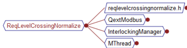
řekil 5.6 : Hemzemin geit arıza normalize talebi sınıf statik baęımlılık grafięi.
