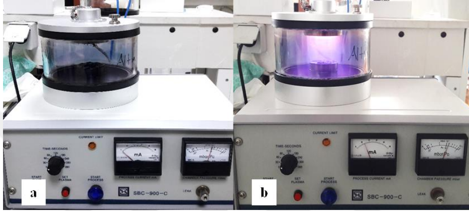
Şekil 3.8. a) SBC-900 Tek hedefli plazma (altın) saçtırmalı ince film kaplama cihazı b) Altın kaplama sırasında oluşan ışıma
