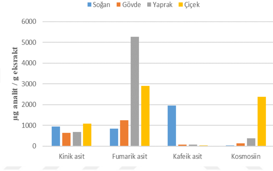
Şekil 4.6. B.sasonii ekstrelerinde yüksek miktarda bulunan fitokimyasal bileşikler
