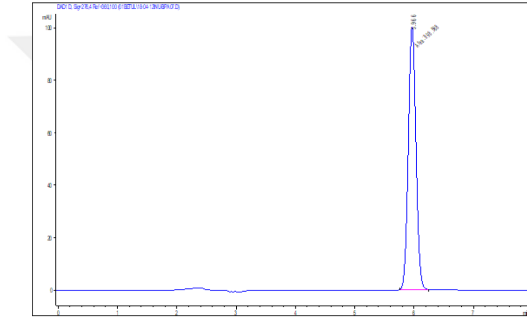
Şekil 4.14. BPA çözeltisinin HPLC kromatogramı
