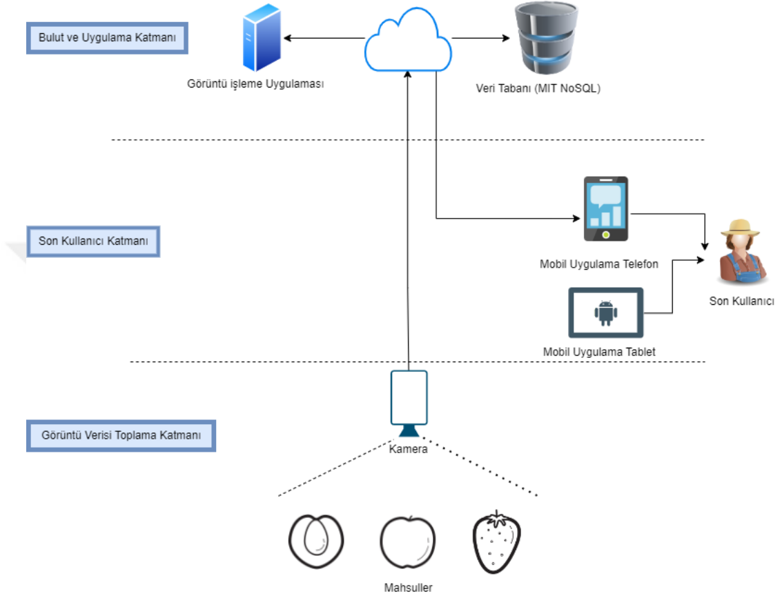
Şekil 4.1. Akıllı tarım görüntü işleme uygulaması genel akış
