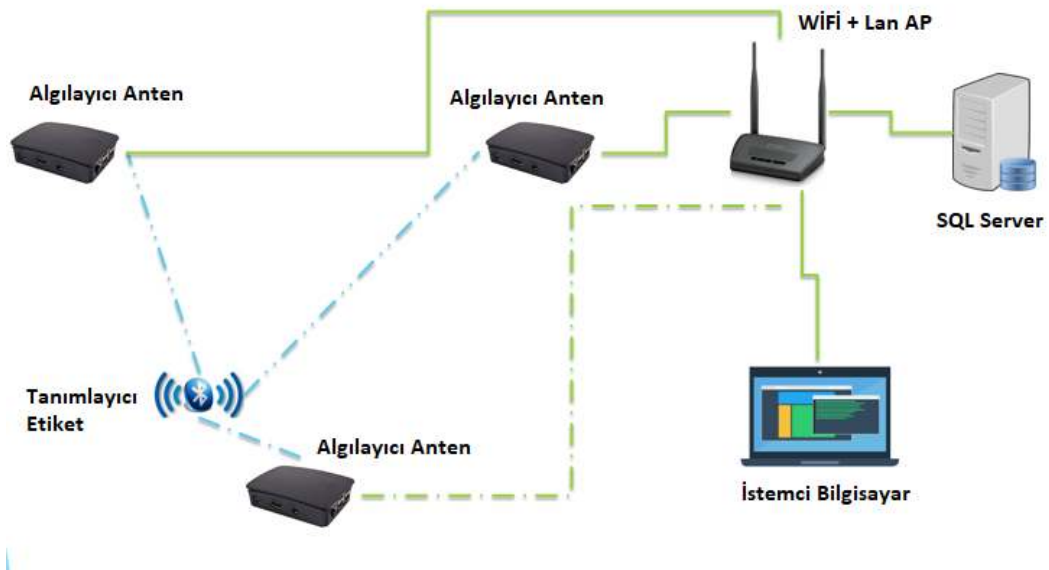
Şekil 3.11. Sistem topolojisi
