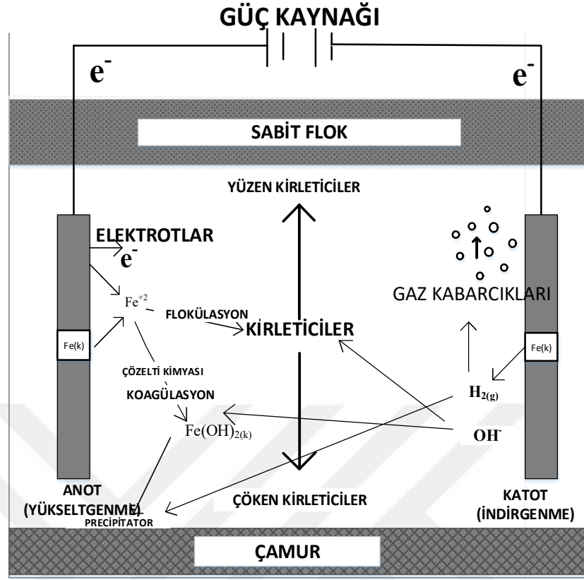
Şekil 3.3. Elektrokoagülasyon mekanizması [54]
