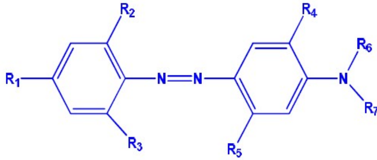
Şekil 2.1. Monoazo dispers boyar maddenin kimyasal yapısı [17].
