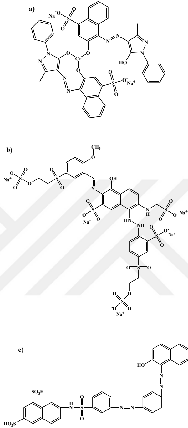
Şekil 3.1. a) Isolan Bordeaux, b) Remazol Red ve c) Erionyl Red boyalarının kimyasal bağ yapısı.
