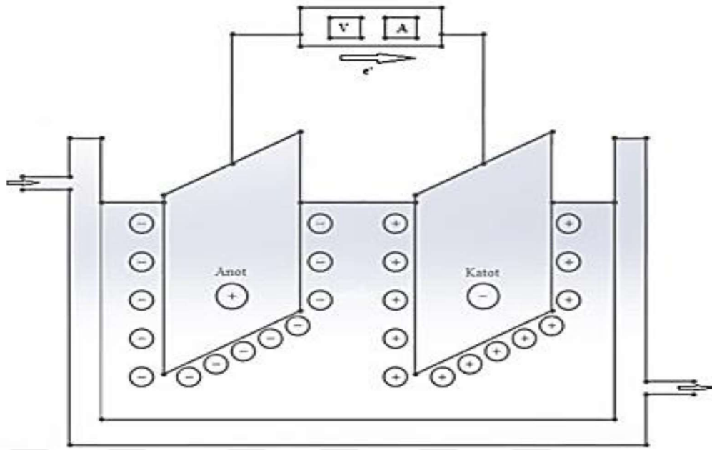
Şekil 2.4. Elektrokimyasal hücrenin şematik gösterimi [56].
