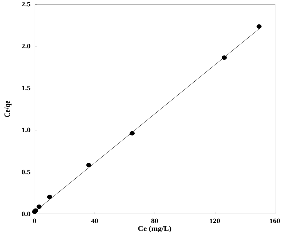
Şekil 4.9. YKHK-MB Langmuir Grafiği
