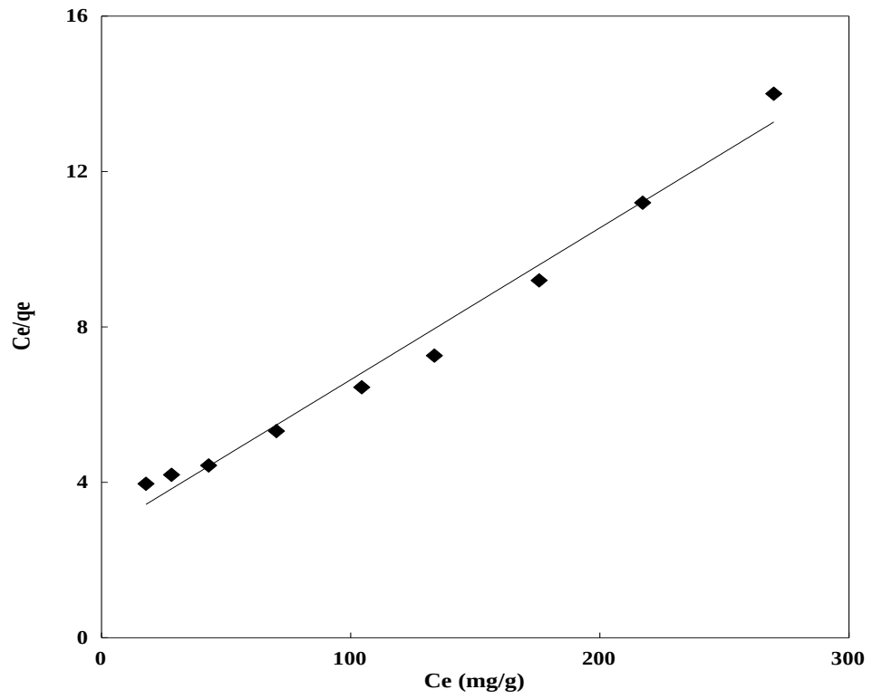
Şekil 4.12 YKHK-MO Langmuir Grafiği
