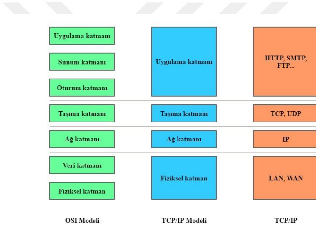
Şekil 3.15. OSI ve TCP/IP katman yapılarının kıyaslanması
