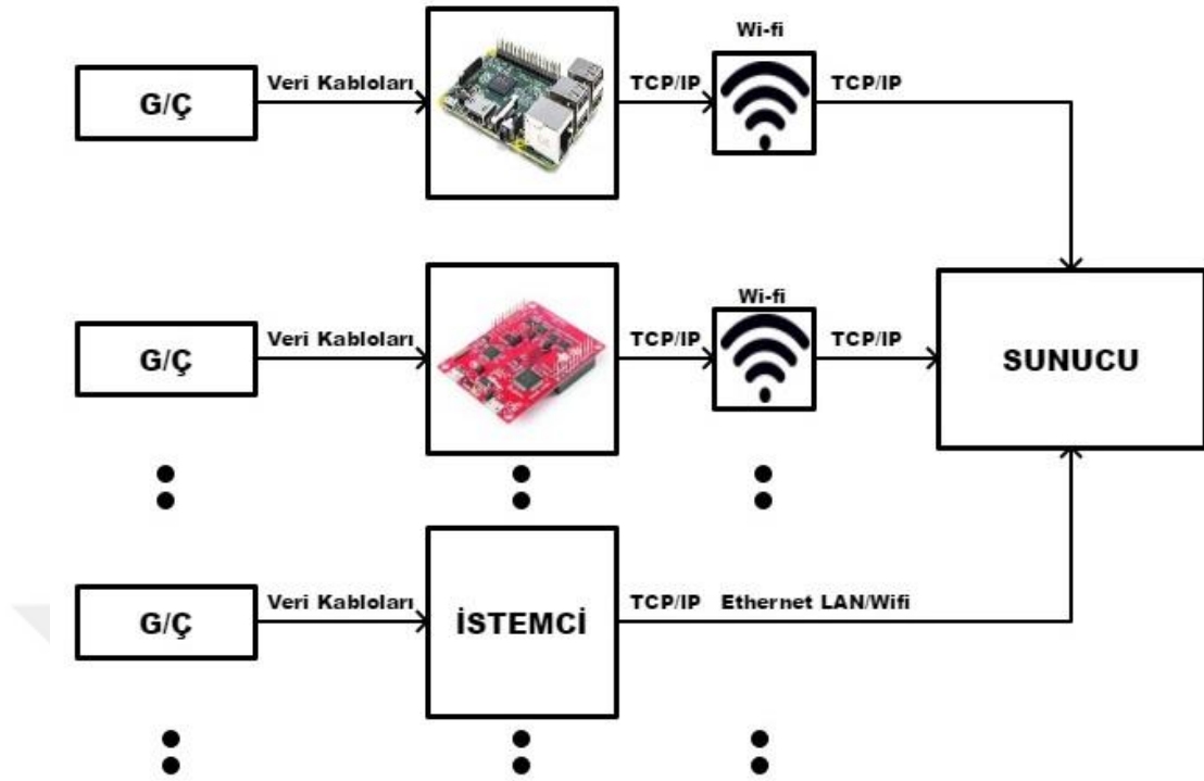
Şekil 1.1. Oluşturulan IoT sisteminin şeması
