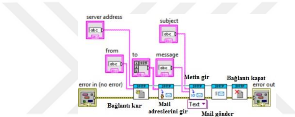
Şekil 3.19. SMTP yazılım kodu uygulaması
