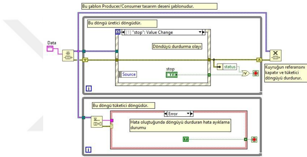
Şekil 3.3. Producer/Consumer tasarım deseni şablonu [18]
