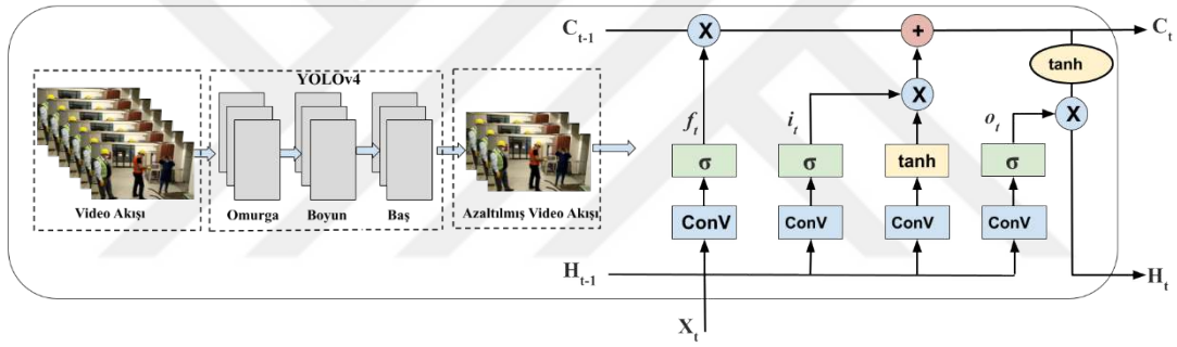
Şekil 3.7. Güvensiz davranış tespiti için YOLOv4 ve ConvLSTM tabanlı önerilen Unsafe-Net derin öğrenme modelinin mimarisi
