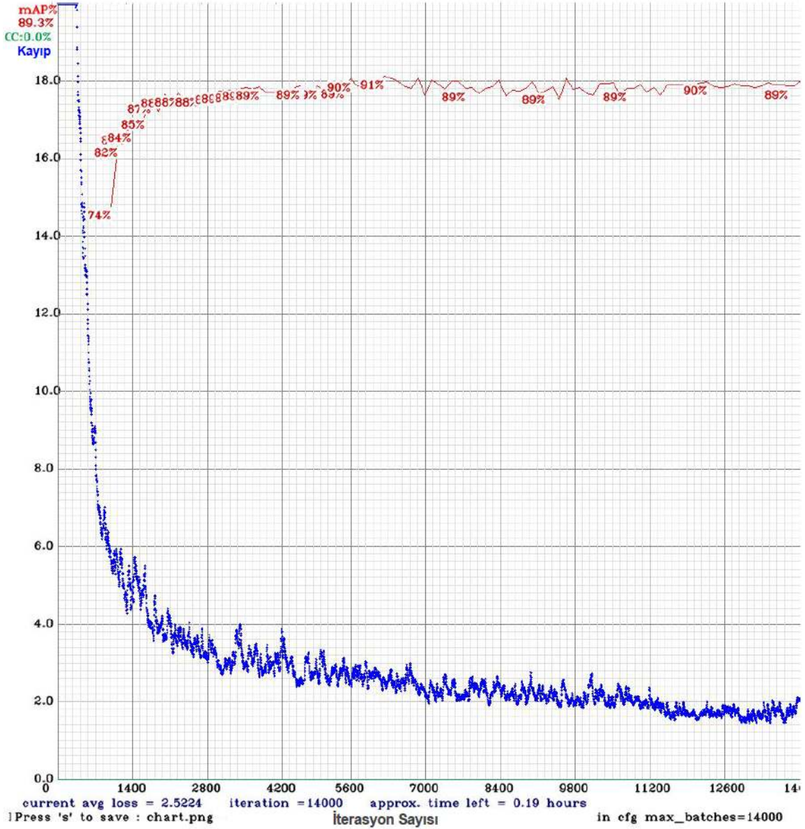
Grafik 4.1. Önerilen YOLOv4 ağının 5 numaralı eğitim için ortalama kayıp ve mAP değerlerinin iterasyon sayısına göre değişimi
