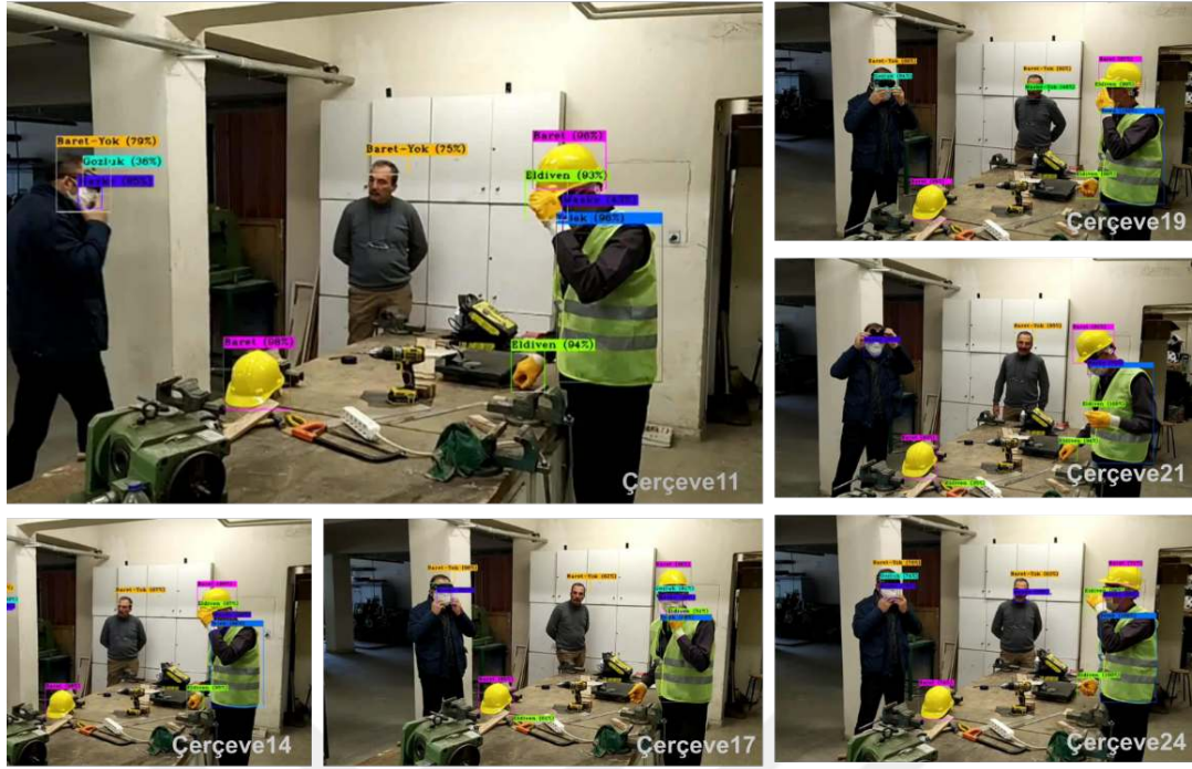
Şekil 4.1. Önerilen YOLOV4 modeli ile video çerçeveleri üzerinde çalışma ortamında KKD tespiti yapılması
