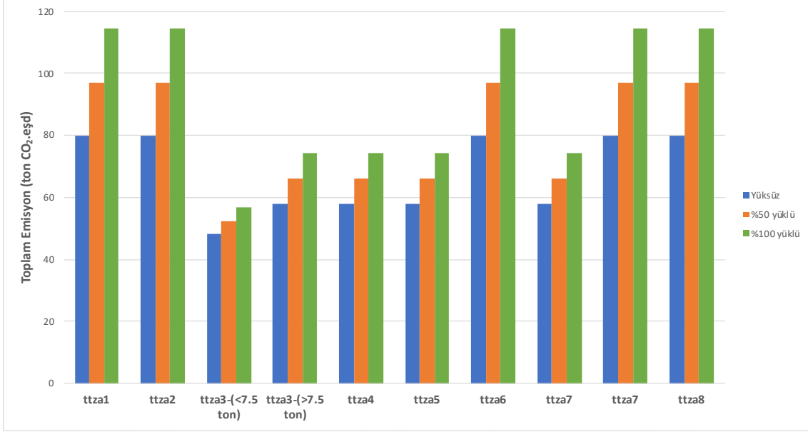
Grafik 8.7. TTZA Araçların Klima Kullanılması ve Taşıdığı Yük Durumlarına Bağlı Toplam Emisyon Değerleri
