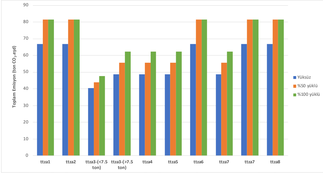
Grafik 8.6. TTZA Araçların Taşıdığı Yük Durumlarına Bağlı Toplam Emisyon Değerleri
