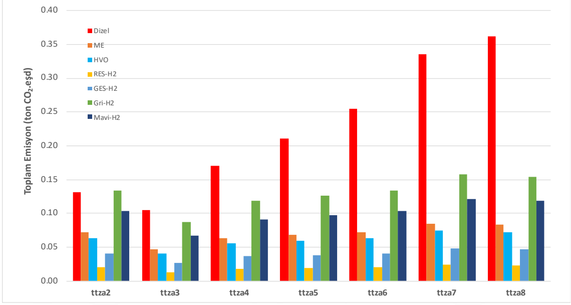
Grafik 8.5. TTZA Araçlara Ait Farklı Yakıt Türlerinin Tüketimine Bağlı Toplam Emisyon Değerleri
