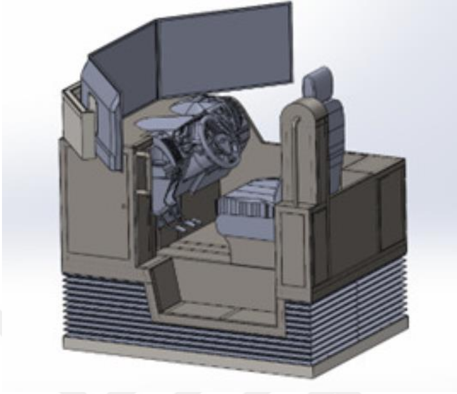
Şekil 7.10. Açık Kabin Simülatörü
