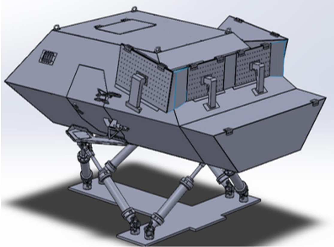
Şekil 7.9. Kapalı Kabin Simülatörü
