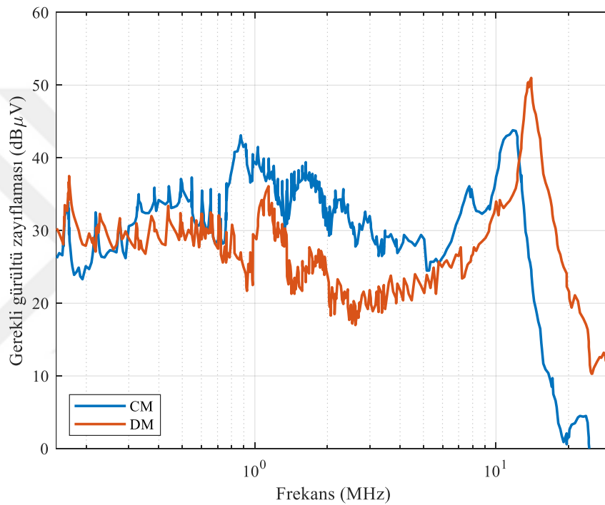
Şekil 4.5. EMI filtreden beklenen gerekli gürültü zayıflatması grafiği.
