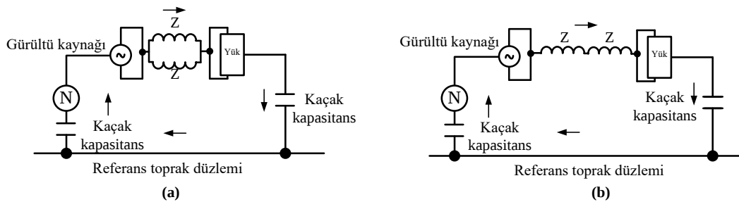
Şekil 1.4. Bobin ve CMC kullanımının karşılaştırılması [2].
