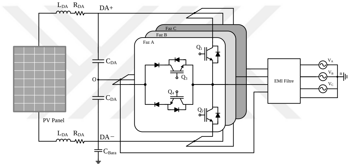
Şekil 3.1. T-tipi şebeke bağlantılı evirici devre şeması.
