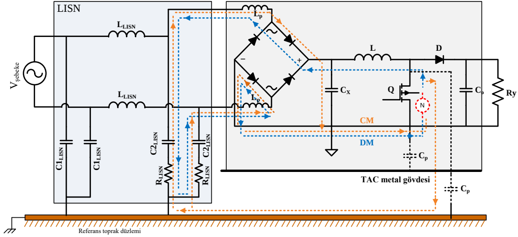
Şekil 4.1. Yükselten PFC devresi ve EMI gürültü yolları.
