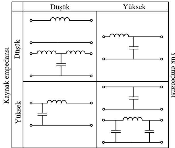
Şekil 3.6. EMI filtre yapısının seçimi için empedans uyumsuzluğu değerlendirmesi.
