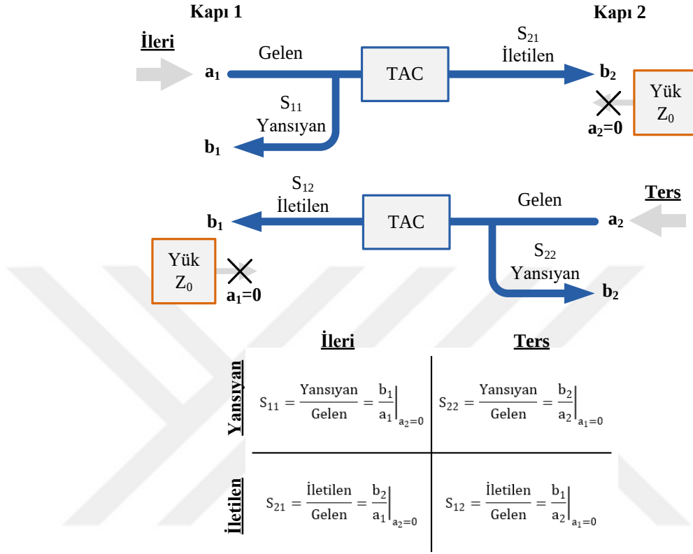
Şekil 4.15. İki kapılı devre için S-parametrelerinin gösterimi [104].
