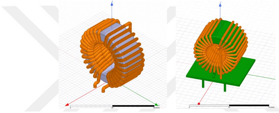
Şekil 4.8. EMI filtrede kullanılan CMC1 ve CMC2 bobinleri.
