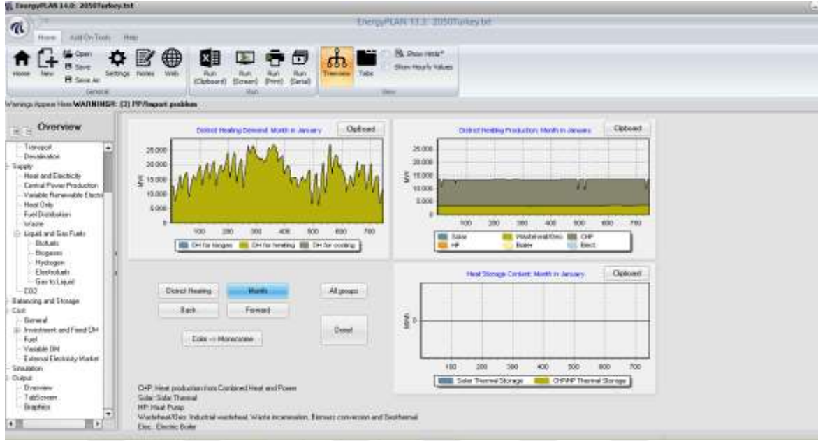
Resim 4.20. 2050 yılı Ocak ayı bölgesel ısıtma sonuçları (Düşük kapasite)
