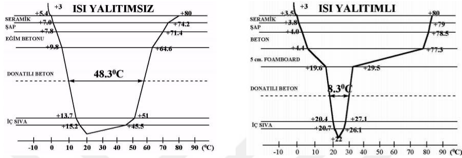
Şekil 6.46. Yaz ve kış mevsimlerinde ısı yalıtımsız çatı plağı kesitindeki sıcaklıklar. Dağsöz ve Ark., 1999
