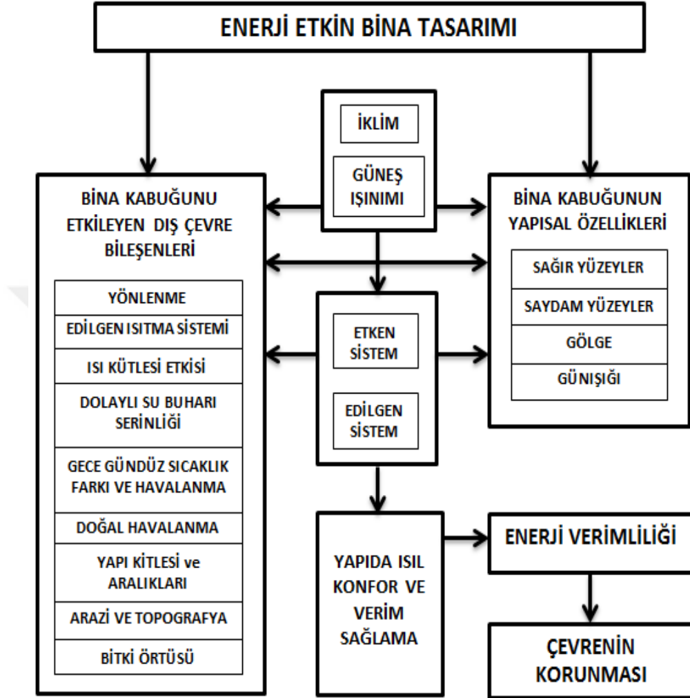
Şekil 5.1. Enerji etkin bina tasarımı (Yüceer, 2015).
