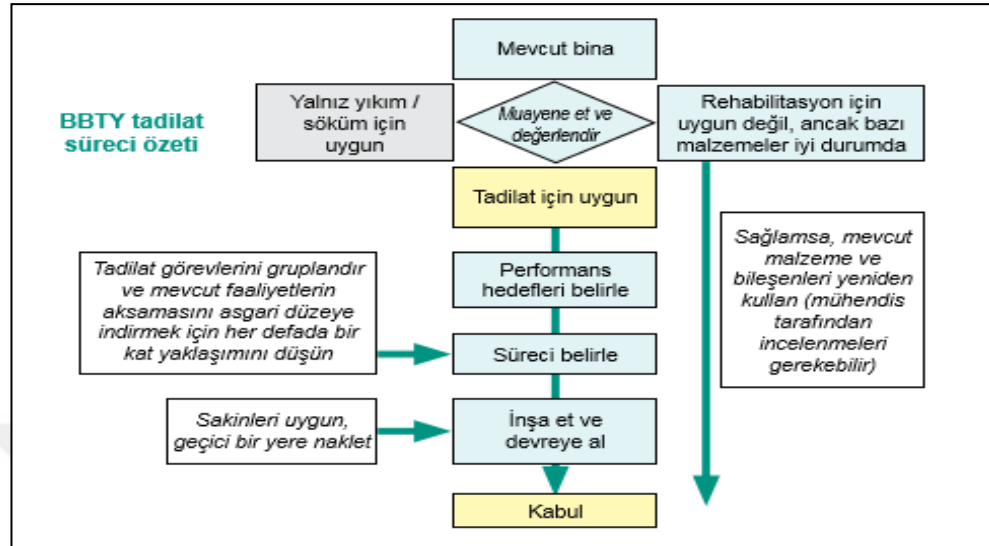
Şekil 5.3. Mevcut Binalar için bütünsel bina tadilat süreci özeti. (Bütünsel Bina Tasarımı Yaklaşımı İle Proje Geliştirme Süreci Uygulama Kılavuzu ISBN: 978-605-5310-87-5)
