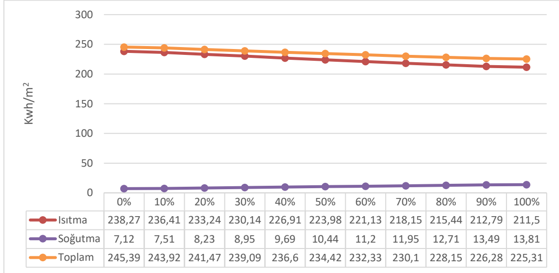
Şekil 4.135. Batı cephe pencere oranının enerji tüketimindeki etkisi
