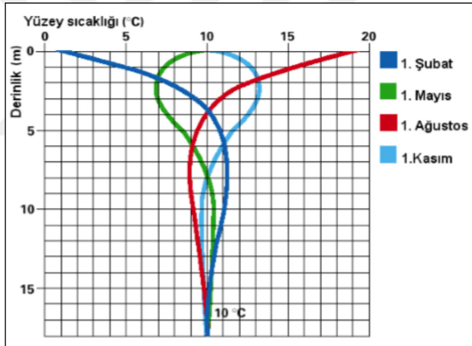
Şekil 2.23. Yıllık toprak altı sıcaklık değişimi [47]
