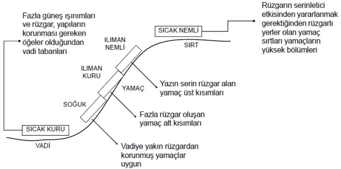
Şekil 3.8. Binaların iklim bölgesine göre konumlandırılması [55]
