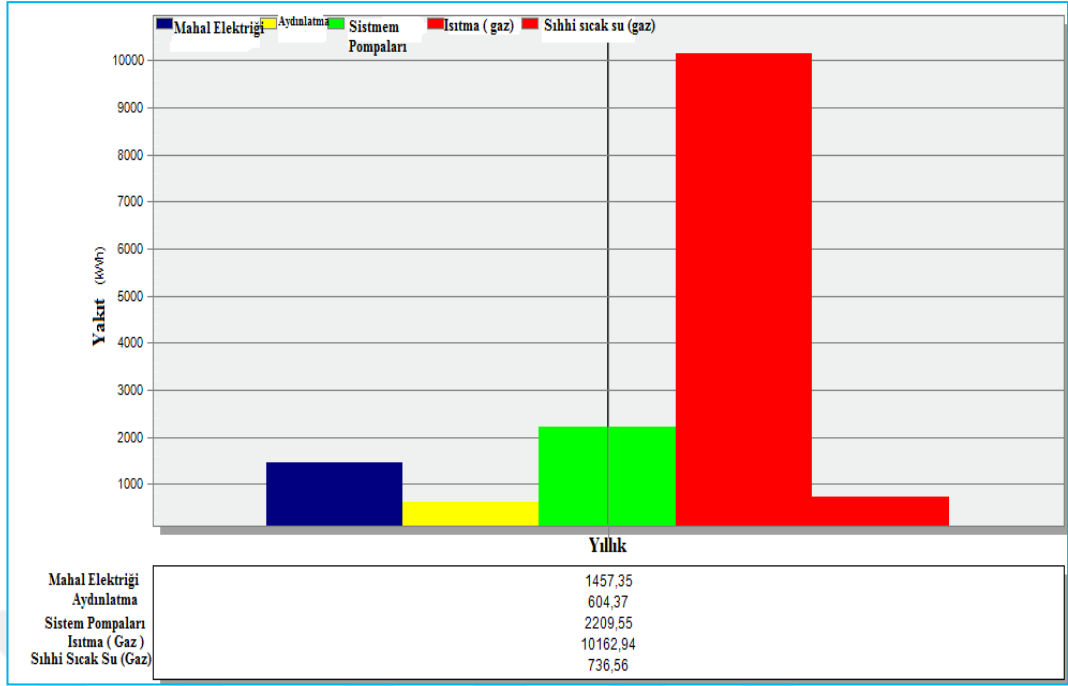
Şekil 5.7. Referans bina yıllık enerji tüketim değerleri
