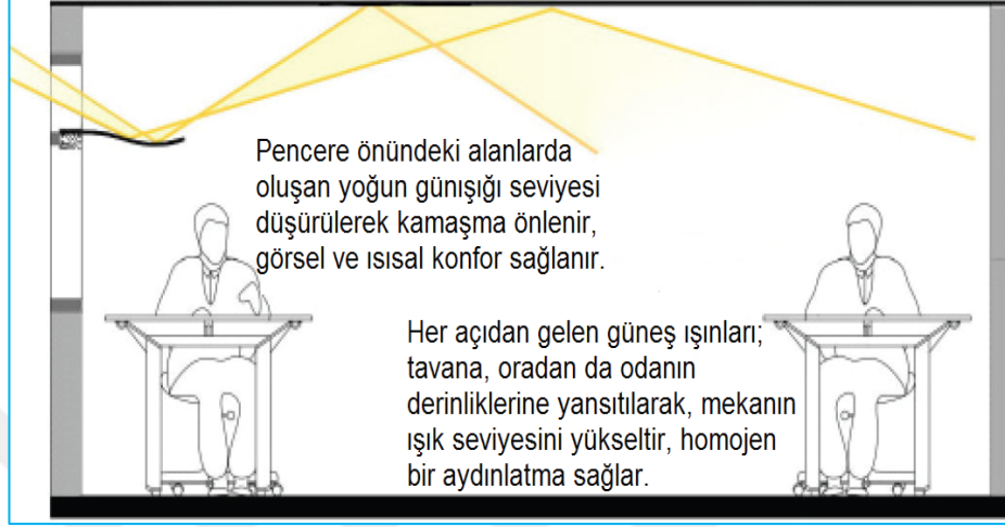
Şekil 2.16. Işık rafları [34]
