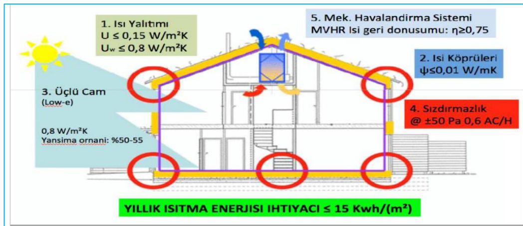
Şekil 2.2. Pasif ev temel tasarım kriterleri [30]
