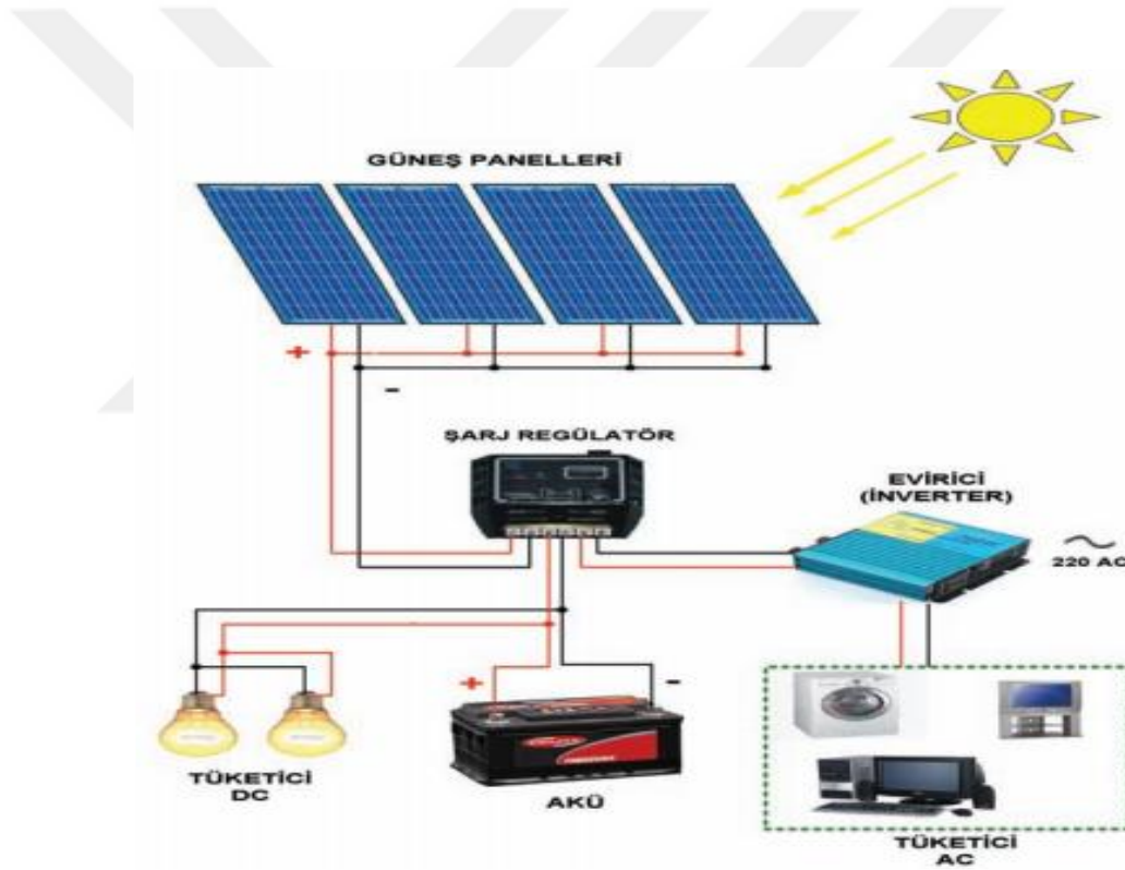
Şekil 2.13. Güneş panel sistemini oluşturan temel donanımlar [39]
