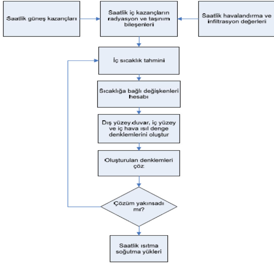
Şekil 4.7. ASHRAE ısıl denge metodu akış şeması [64]
