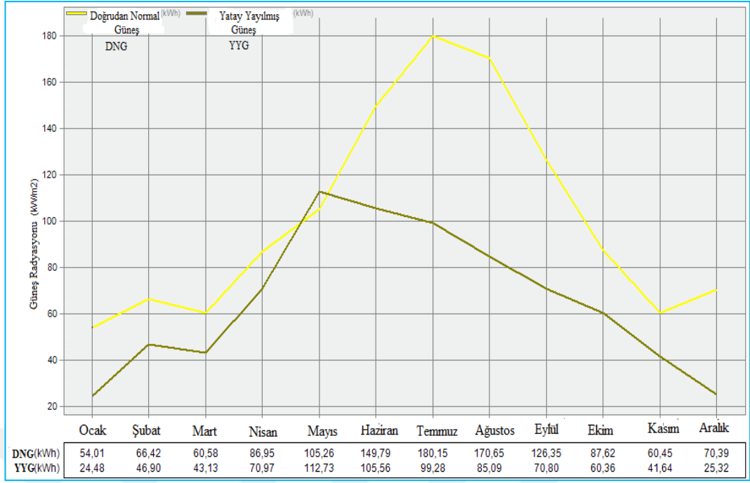
Şekil 5.4. Malatya iline ait aylık ortalama doğrudan normal güneş ve yatay difüz güneş miktarı
