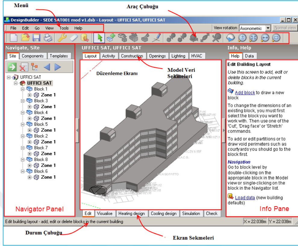
Şekil 4.3. DesignBuilder kullanıcı ara yüzü [62]
