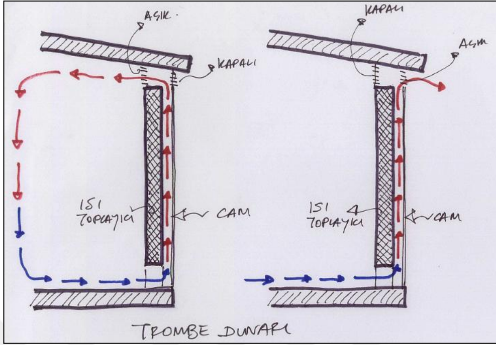
Şekil 2.6. Trombe duvar ısıtma ve havalandırma çalışma sistemi [34]
