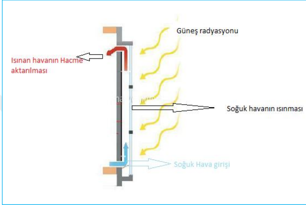
Şekil 4.16. Trombe duvardaki hava döngüsü [75]
