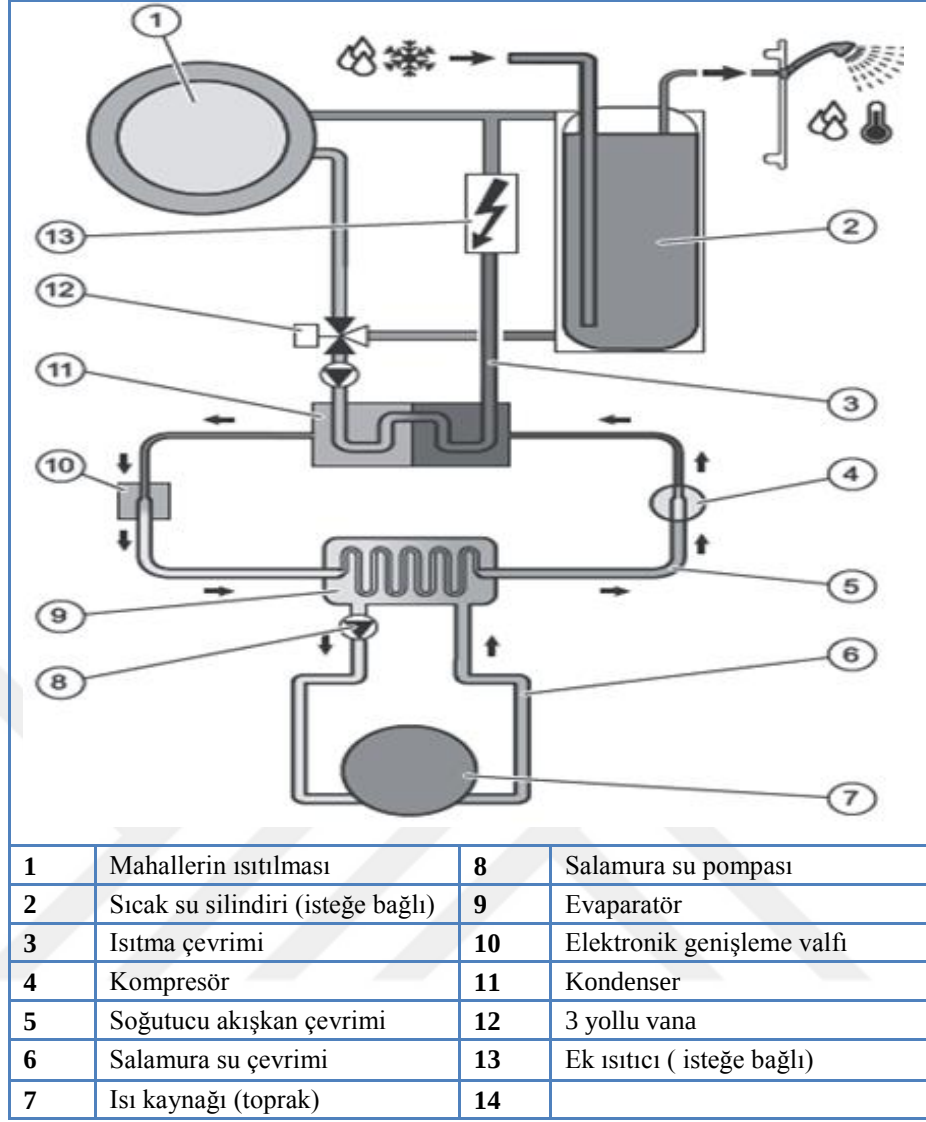
Şekil 4.13. Isı pompası ile ısıtma ve sıcak temini şematik gösterimi [68]
