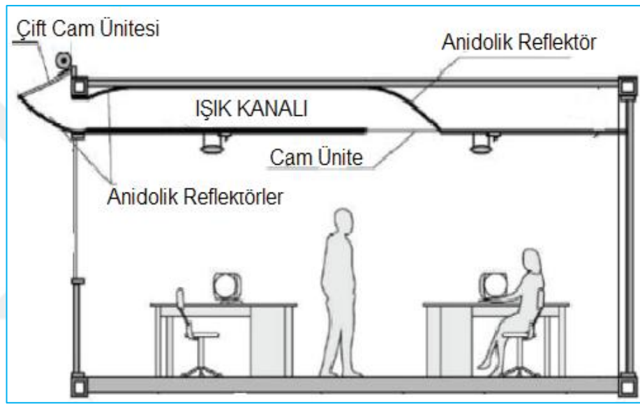
Şekil 2.18. Andolik tavan sistemi [34]
