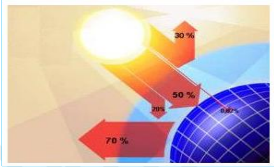
Şekil 2.4. Güneş ışınlam değerlerinin dünyaya ulaşan ve ulaşamayan değerleri
