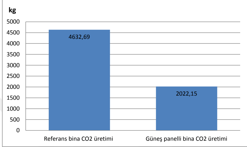
Şekil 5.12. Referans bina ve Güneş panelli bina CO 2 üretim değerleri
