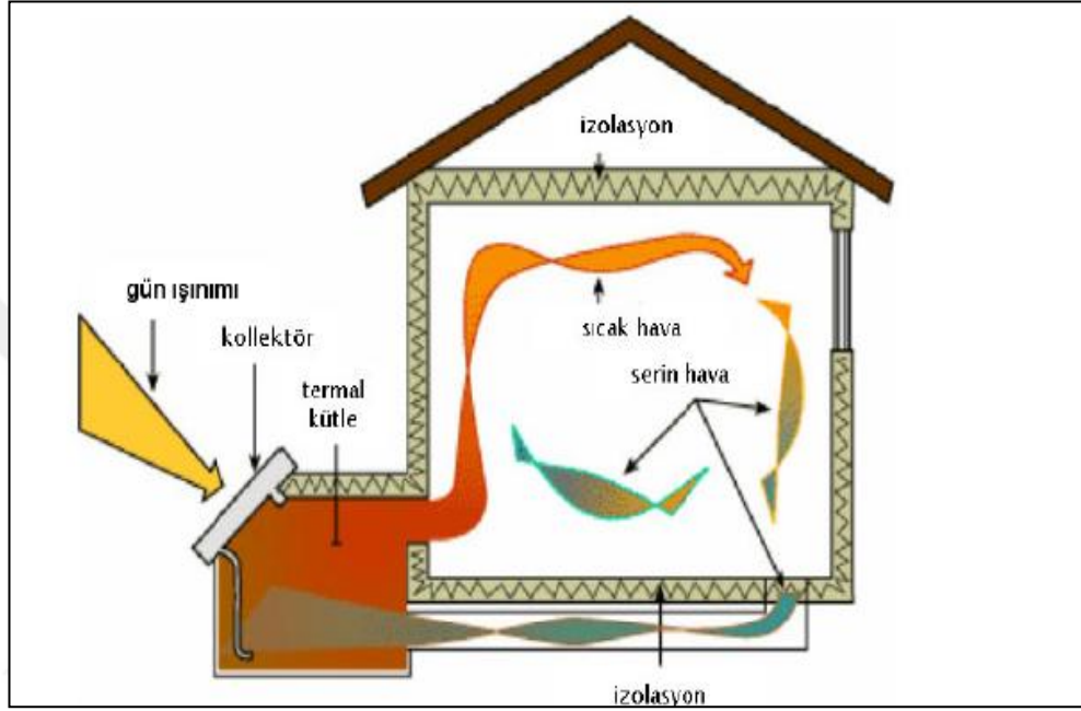
Şekil 2.9. Termosifon sistemler [12, 34]
