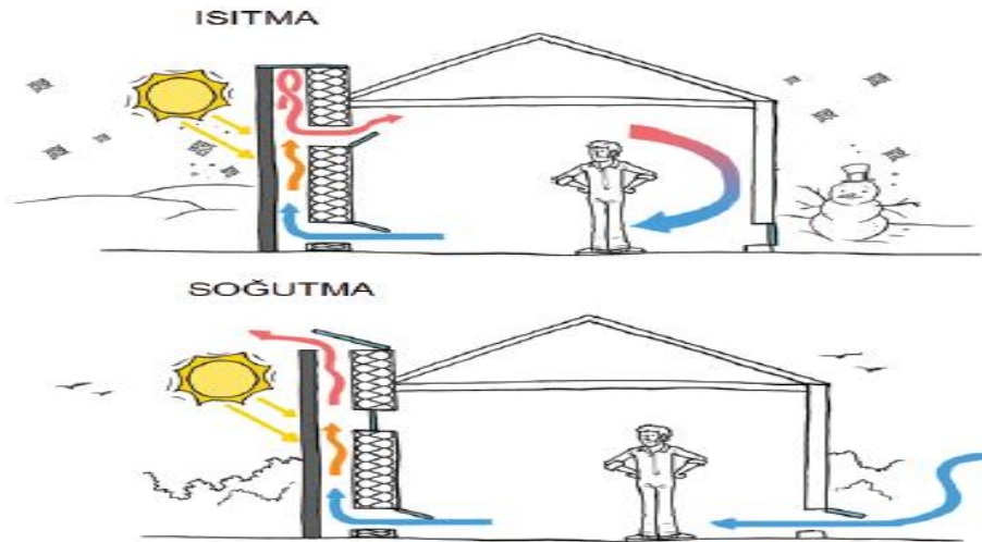
Şekil 2.11. Güneş baca sistemi [34]
