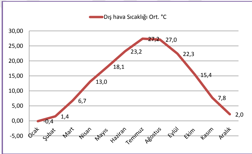
Şekil 4.2. Malatya ortalama dış hava sıcaklıkları [60]
