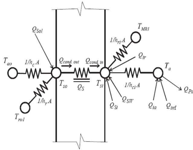
Şekil 4.6. ASHRAE Isıl denge metodu direnç şeması [65]
