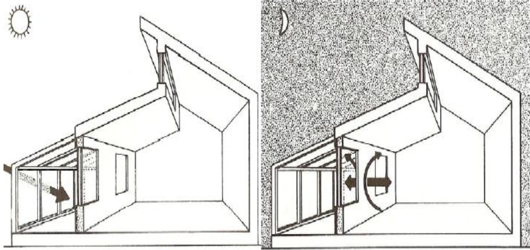
Şekil 2.10. Sera sistemi [34]
