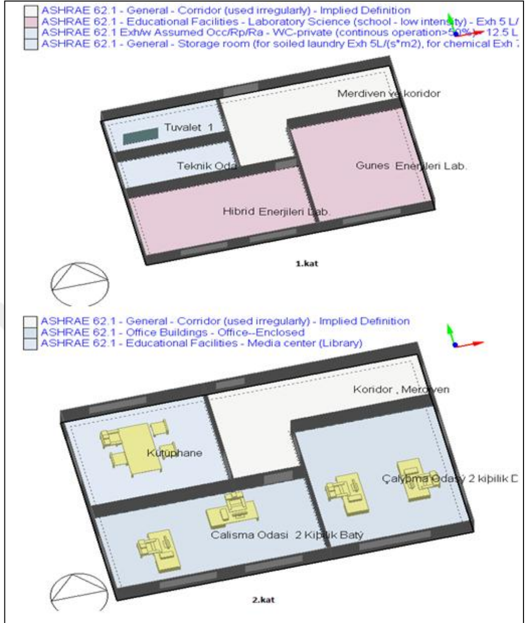
Şekil 4.12. Bina hacim organizasyonu
