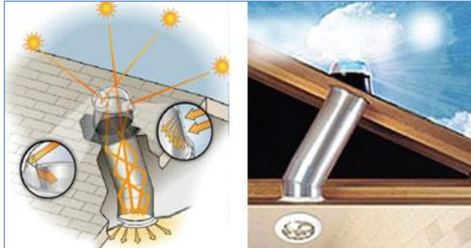
Şekil 2.17. Işık tüpleri [34]
