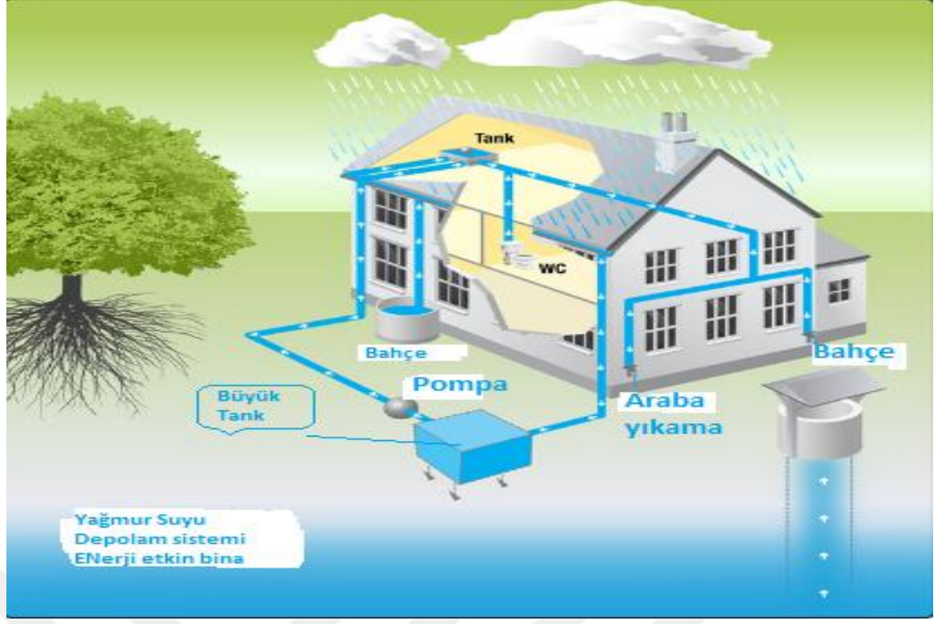
Şekil 4.21. Yağmur suyu depolama ve dağıtım sistemi örneği [79]
