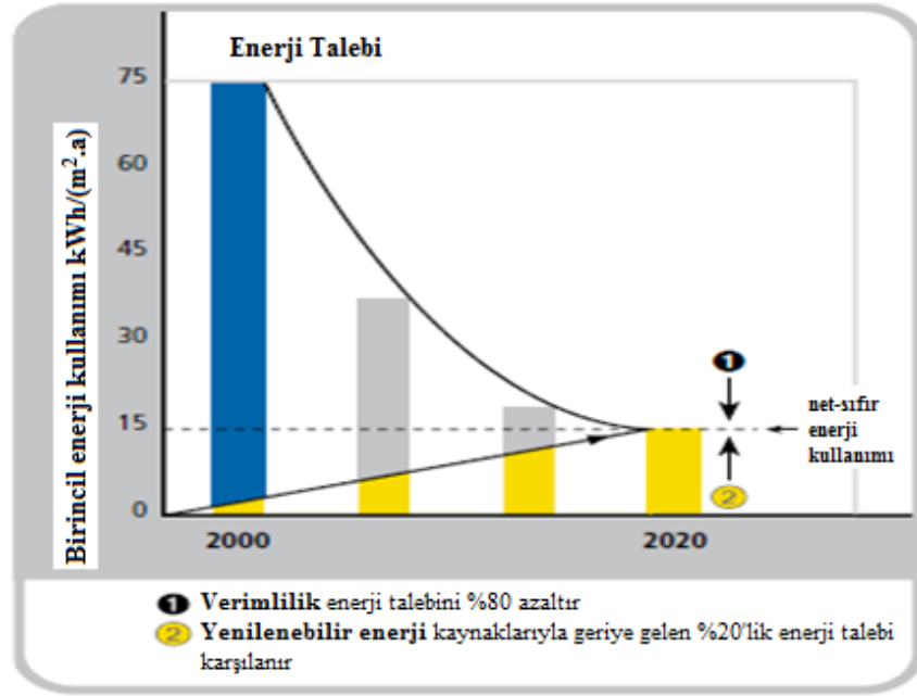
Şekil 2.3. Net-sıfır enerji tüketimin başarılması
