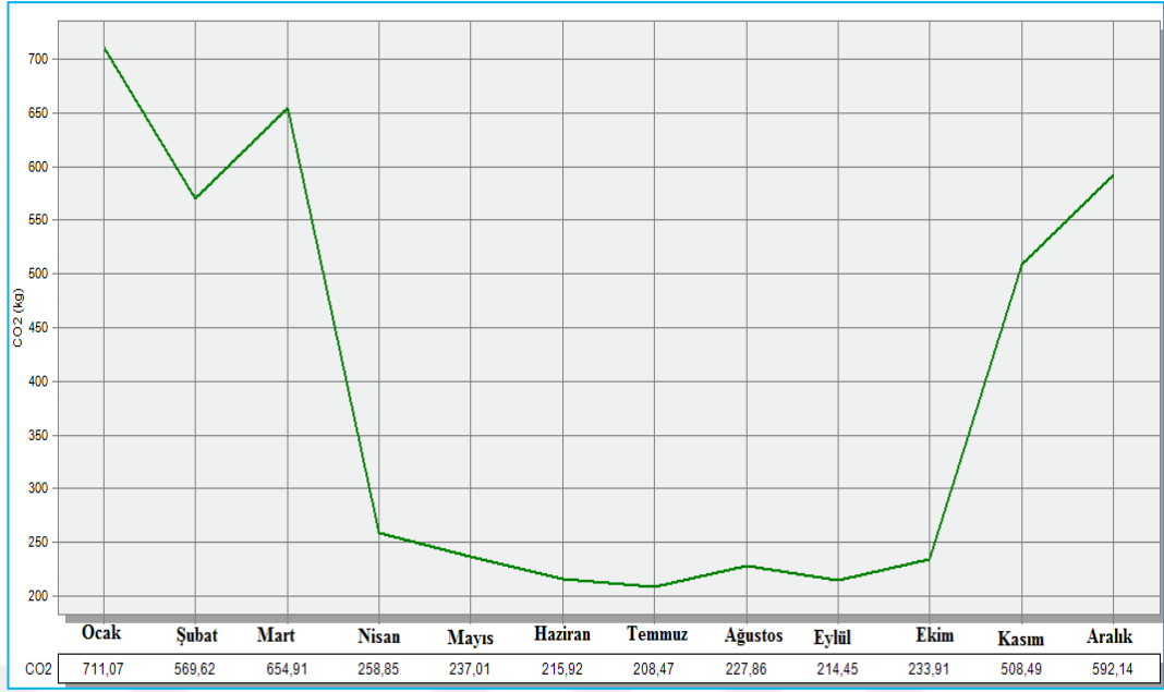
Şekil 5.9. Referans bina aylık ortalama CO 2 üretim miktarları
