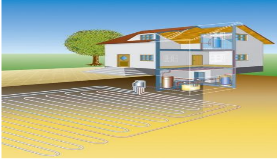
Şekil 2.24. Düz yatay tip toprak kaynaklı ısı pompası [48]
