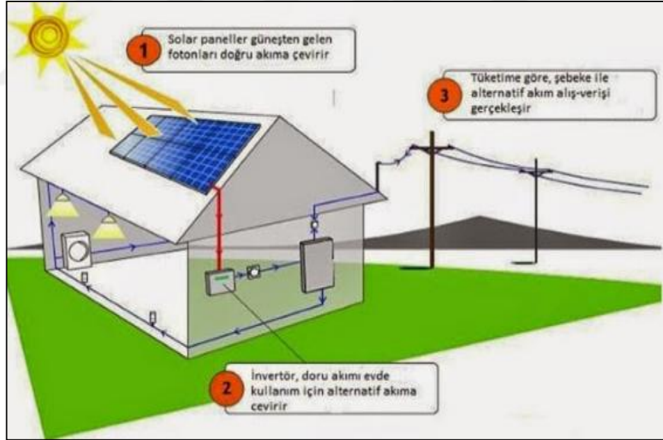
Şekil 2.15. Şebeke bağlantılı sistemler (on grid) [42]
