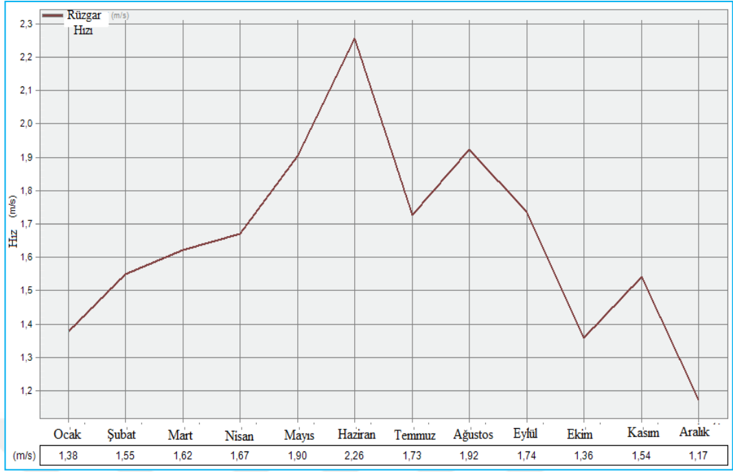
Şekil 5.2. Malatya ili aylık ortalama rüzgâr hızı değerleri
