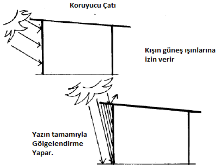
Şekil 4.18. Trombe duvar koruyucu komponent bileşeni [75]
