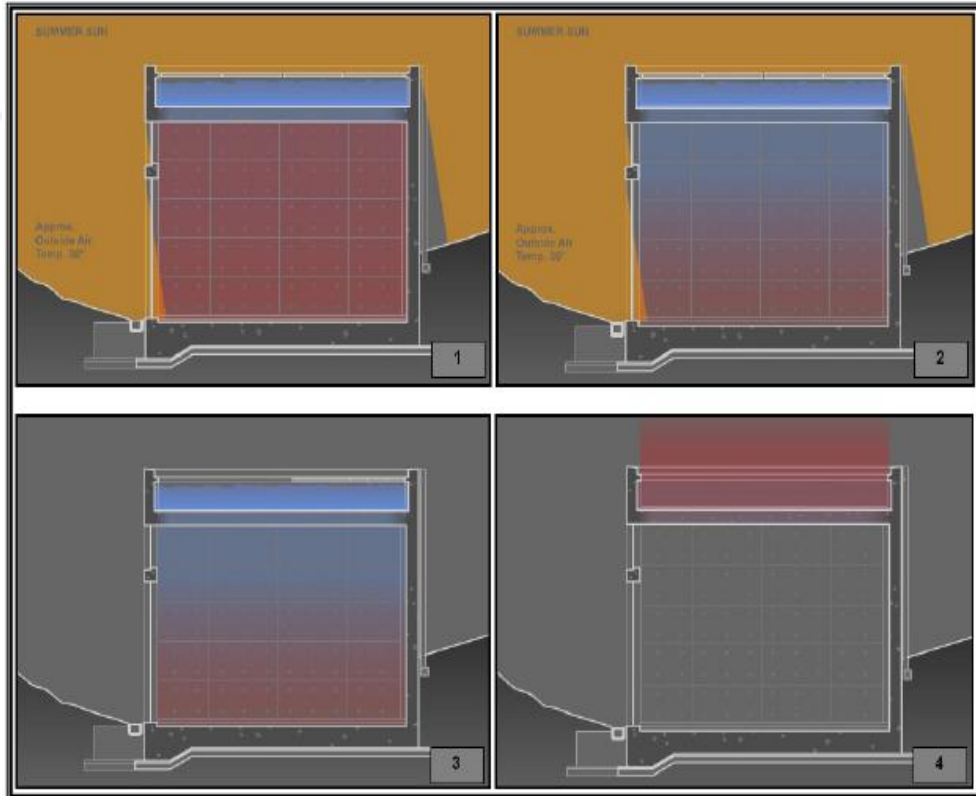
Şekil 2.8. Çatı havuz sistemi [12]
