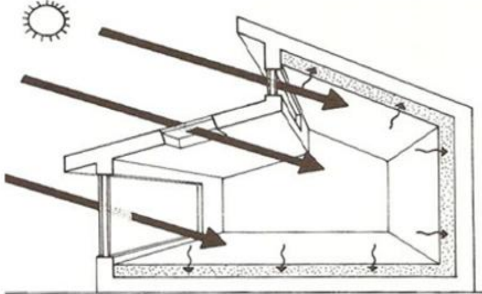
Şekil 2.5. Doğrudan kazanım sistemleri [34]
