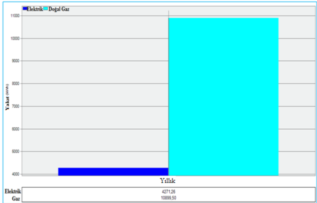
Şekil 5.8. Referans bina yıllık doğal gaz ve elektrik enerji tüketim değerleri
