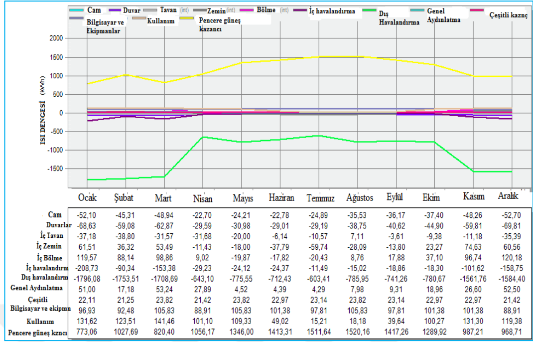
Şekil 5.5. Referans bina aylık ısı kayıpları ve kazançları
