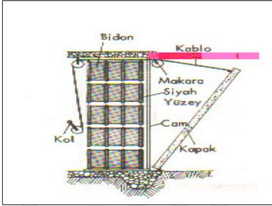
Şekil 2.7. Bidon duvar sistemi [12]
