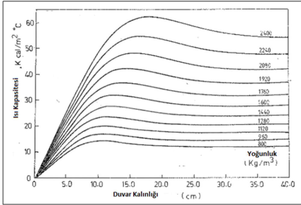
Şekil 4.17. Beton bloğun gündüzleri ısı depolama kapasitesinin duvar yoğunluğu ve duvar kalınlığına göre değişimi [75]
