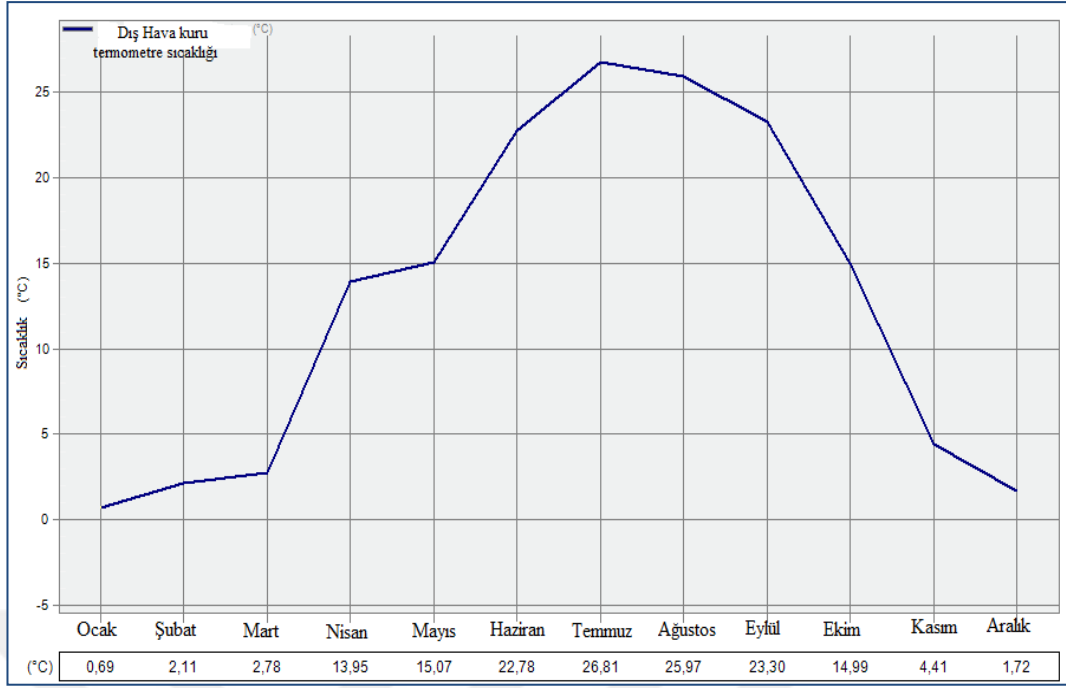
Şekil 5.1. Malatya ili aylık dış hava kuru termometre sıcaklığı
