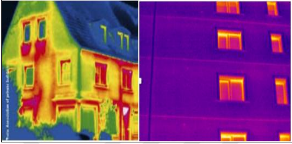
Şekil 3.11. Yalıtımlı ve yalıtımsız bir binada termal ısı kaybı karşılaştırılması
