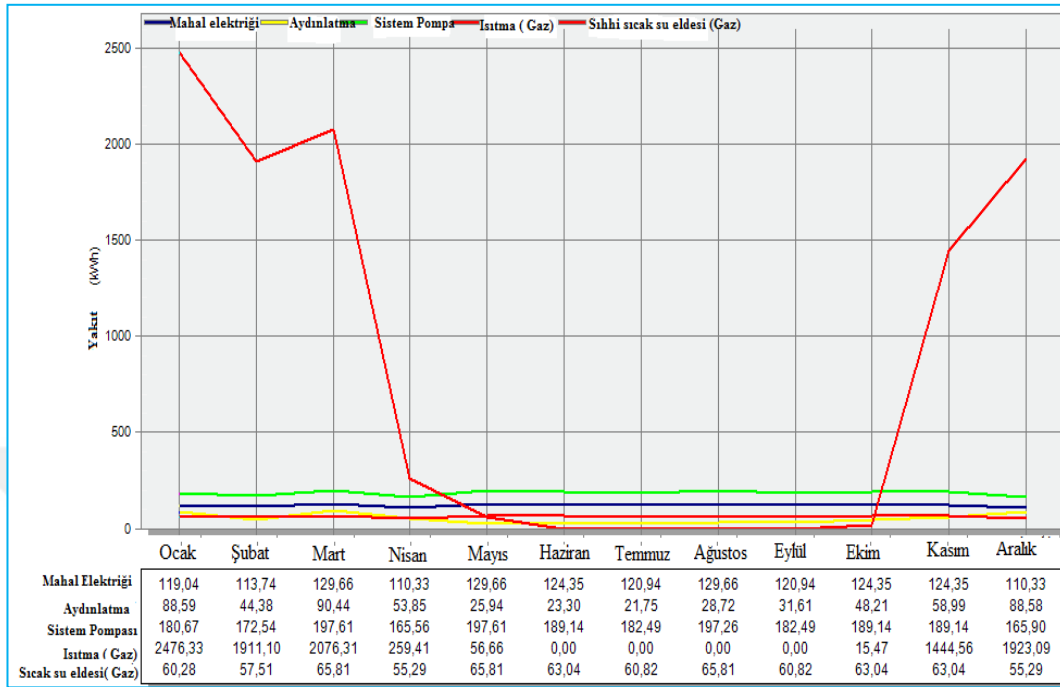
Şekil 5.6. Referans bina aylık enerji tüketim değerleri
