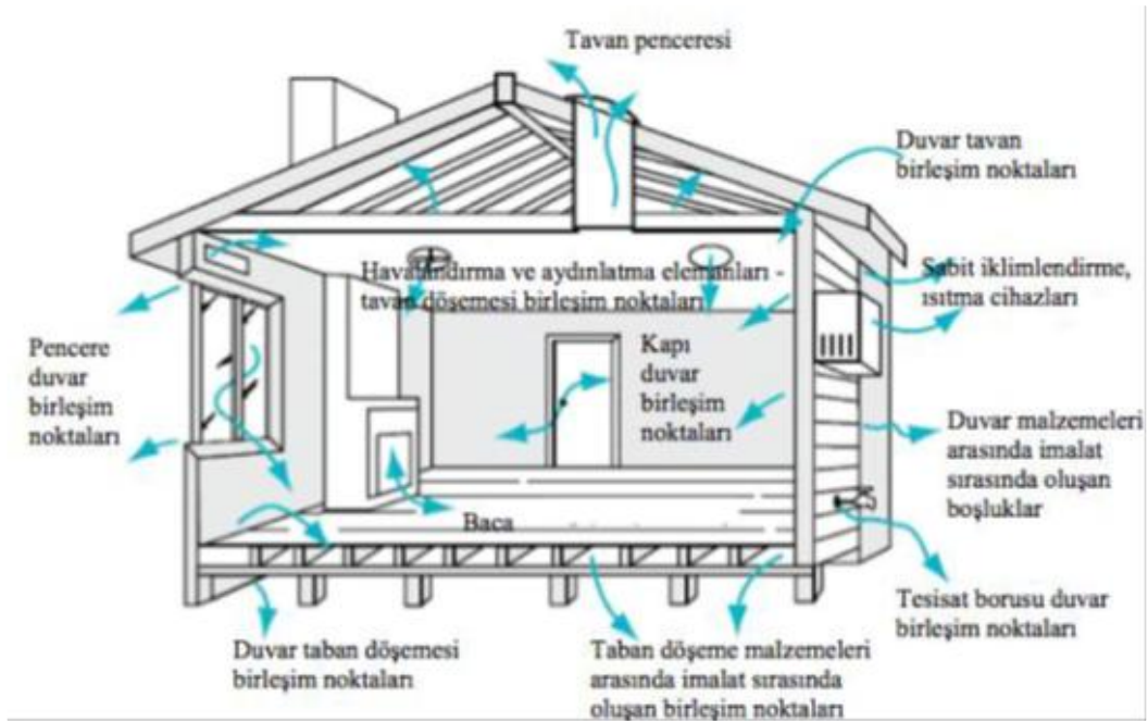
Şekil 3.13. Binalarda hava sızdırma oluşabilecek yerler [25]
