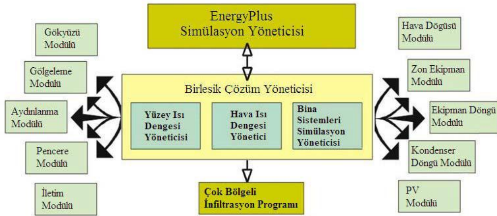
Şekil 4.5. Simülasyon yöneticisi yapısı [63]
