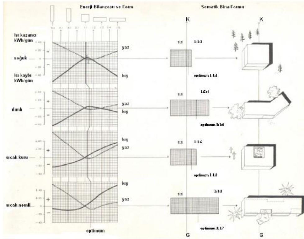
Şekil 3.9. Bina formu enerji etkileşimi [30]
