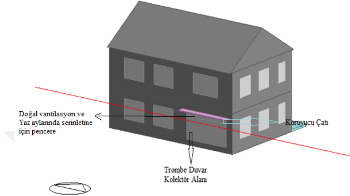
Şekil 4.19. Enerji etkin binada Trombe duvar görünümü
