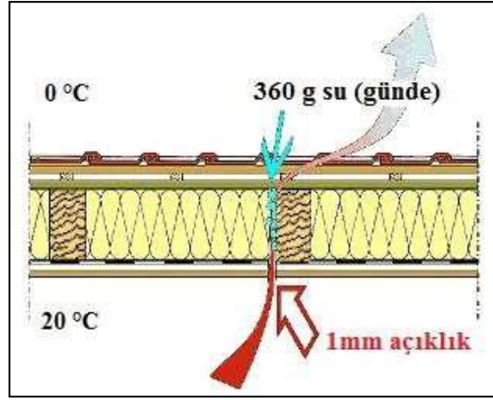
Şekil 3.14. Hava boşluklarında su buharının geçişi [25]
