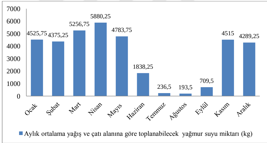
Şekil 4.22. Çatı yatay alanı ve ilin yağış miktarına göre toplanabilecek yağmur suyu
