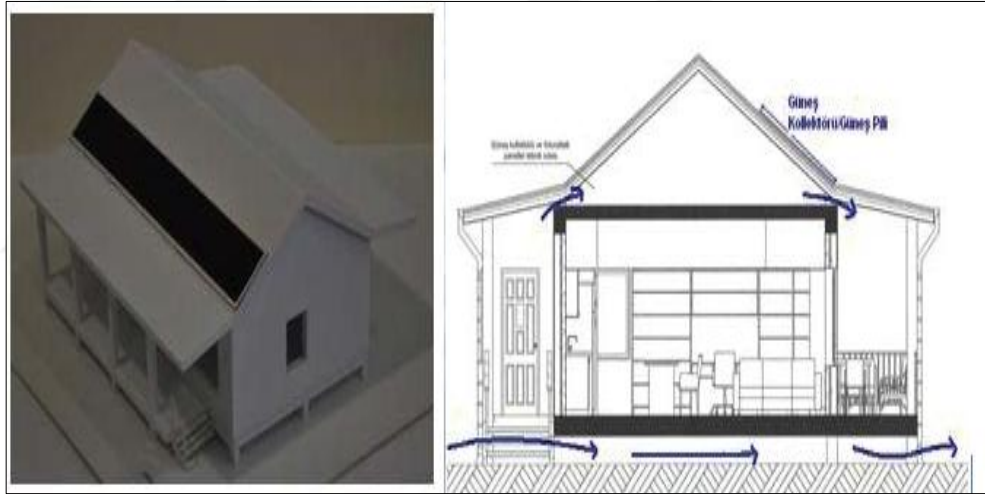
Şekil 3.4. Sıcak-nemli iklim bölgesinde tasarlanmış ev örneği [54]
