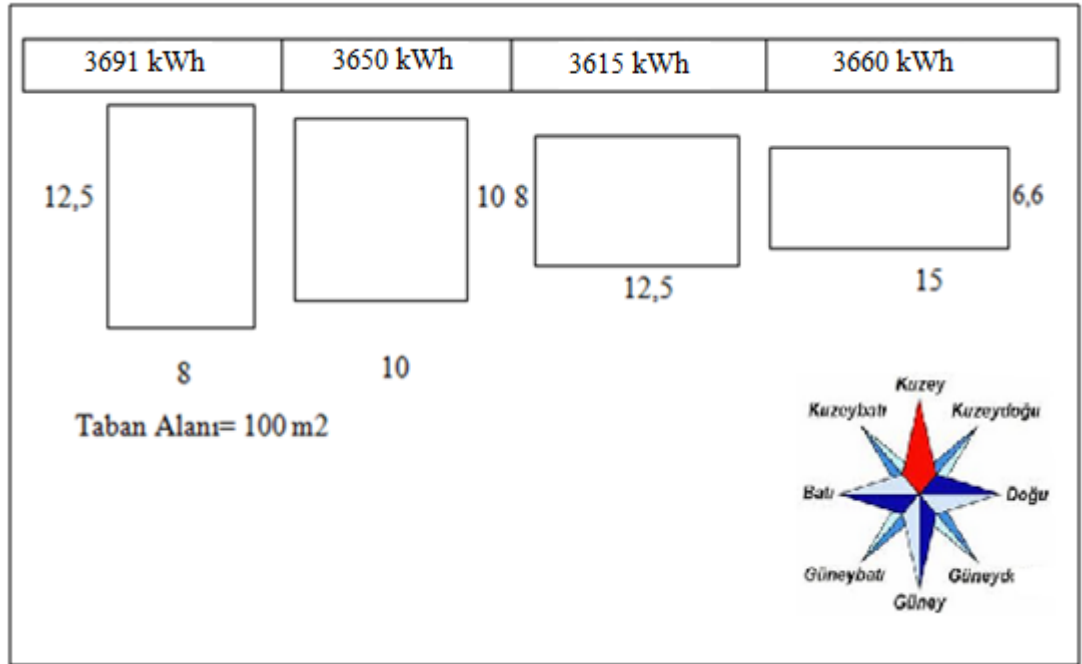
Şekil 4.10. Bina yön ve formuna bağlı ısıtma enerji tüketimi
