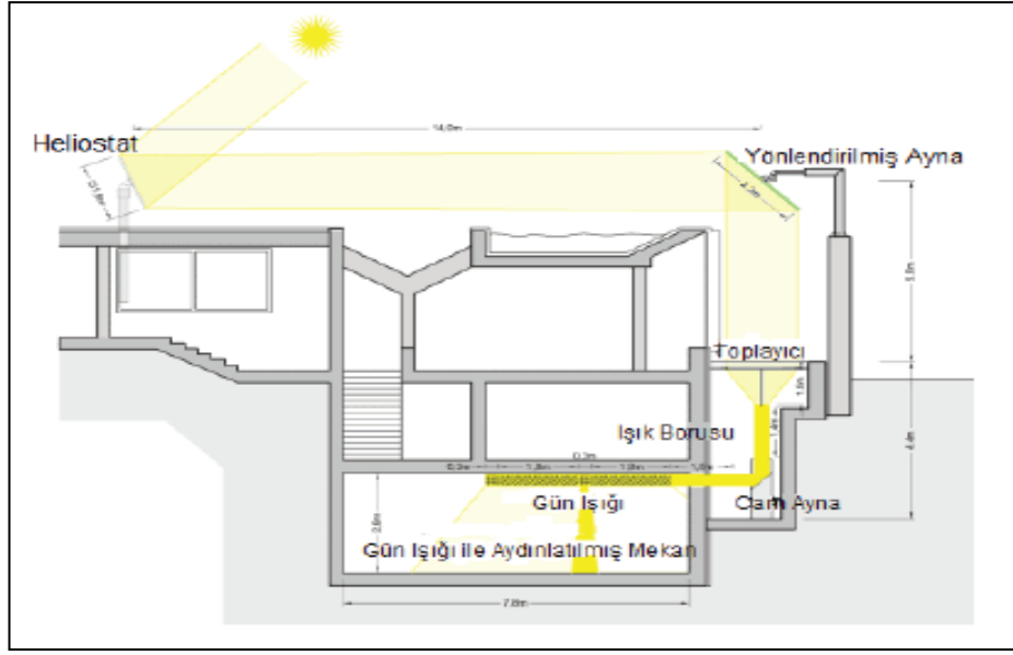
Şekil 2.19. Heliostat sistemi [34]
