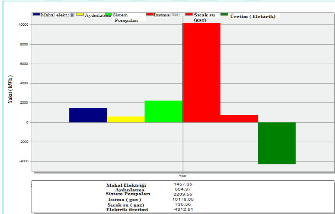
Şekil 5.11. Fotovoltaik sistemli binanın enerji üretim ve tüketim değerleri
