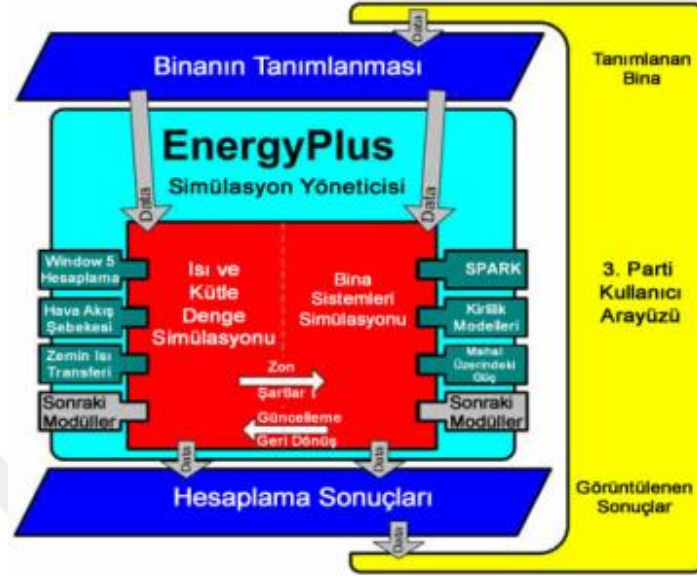
Şekil 4.4. EnergyPlus programı çalışma prensibi [63]
