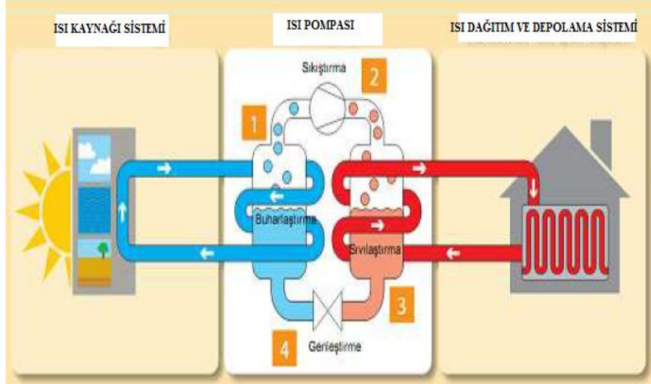
Şekil 2.22. Isı pompası çalışma sistemi [47]
