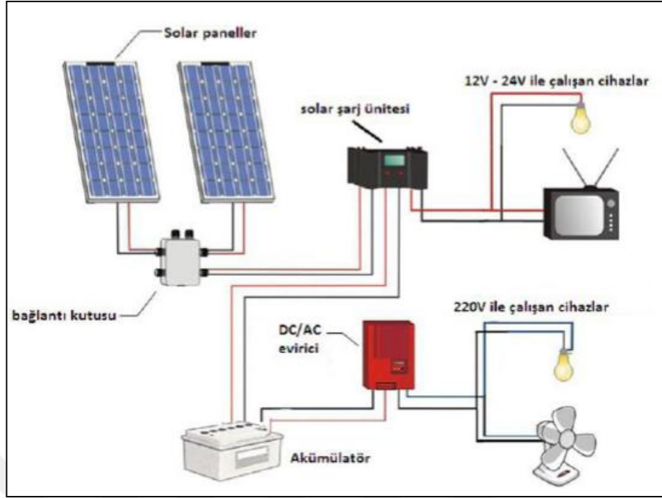
Şekil 2.14. Şebekeden bağımsız sistemler (off grid) [41]
