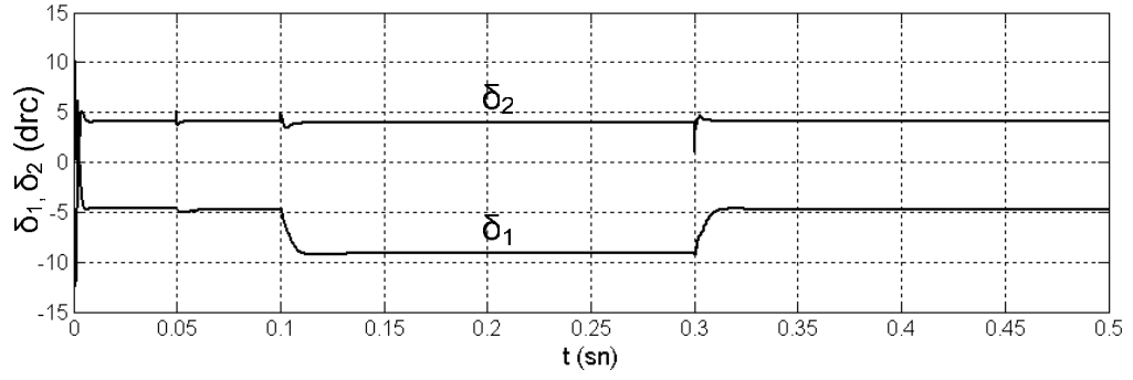
Şekil 7.44 Bara1 ve bara 2 gerilim açılarının zamana göre değişimleri.
