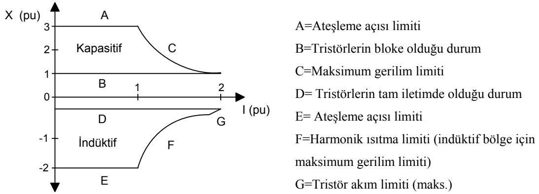
Şekil 2.6 TCSC’nin X-I karakteristiği
