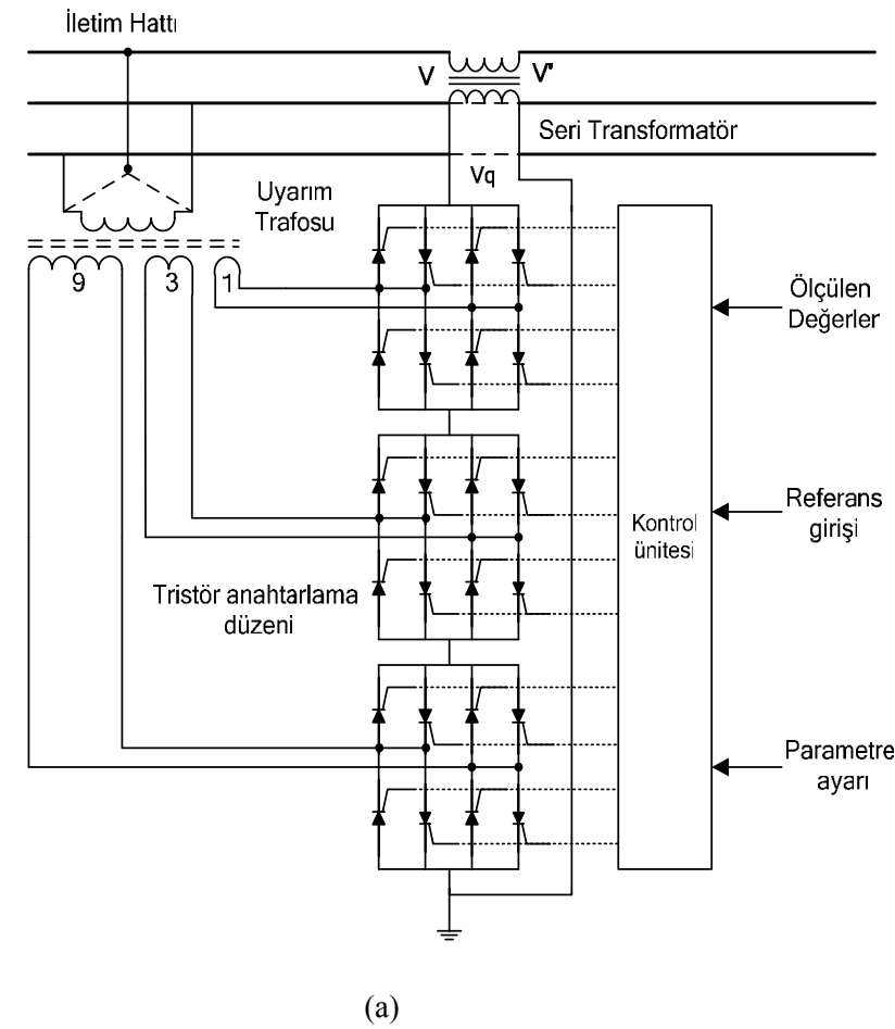
Şekil 2.10 a) TCPAR devre konfigürasyonu b) Faz kayması
