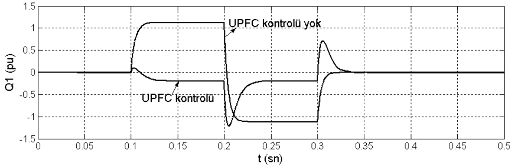
Şekil 7.37 UPFC kontrolü ve UPFC kontrolü olmadan bara 1 reaktif güç akışının karşılaştırmalı olarak zamana göre değişimi.
