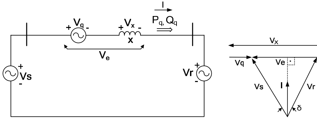
Şekil 2.21 SSSC eşdeğer devresi ve fazör diyagramı
