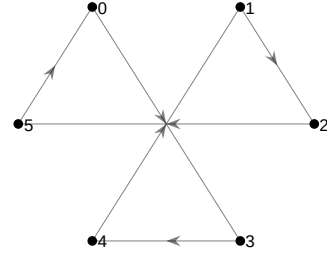
(d) Tour: 0-3-4-1-2-5
