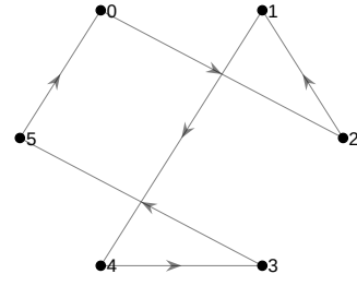
(b) Tour: 0-2-1-4-3-5
