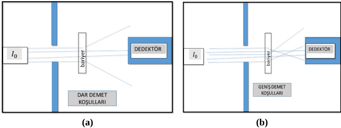
Şekil 3.2. Işınlanma koşulları (a) dar-demet; (b) geniş-demet
