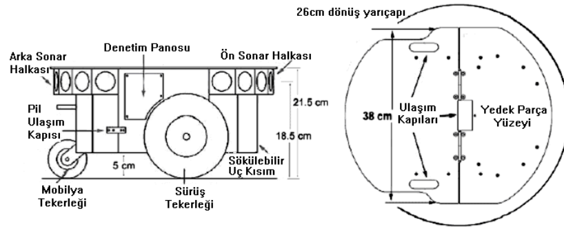
Şekil 5.2 Pioneer 3-DX’in fiziksel boyutu ve dönüş yarıçapı
