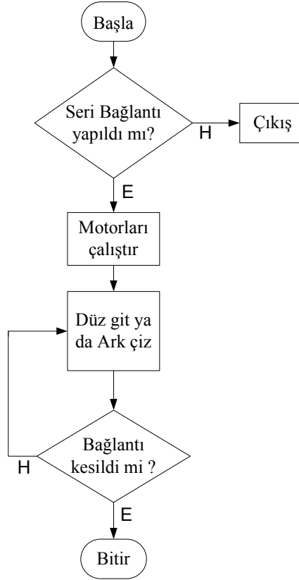
Şekil 6.2 C++ tabanlı programın akış diyagramı
