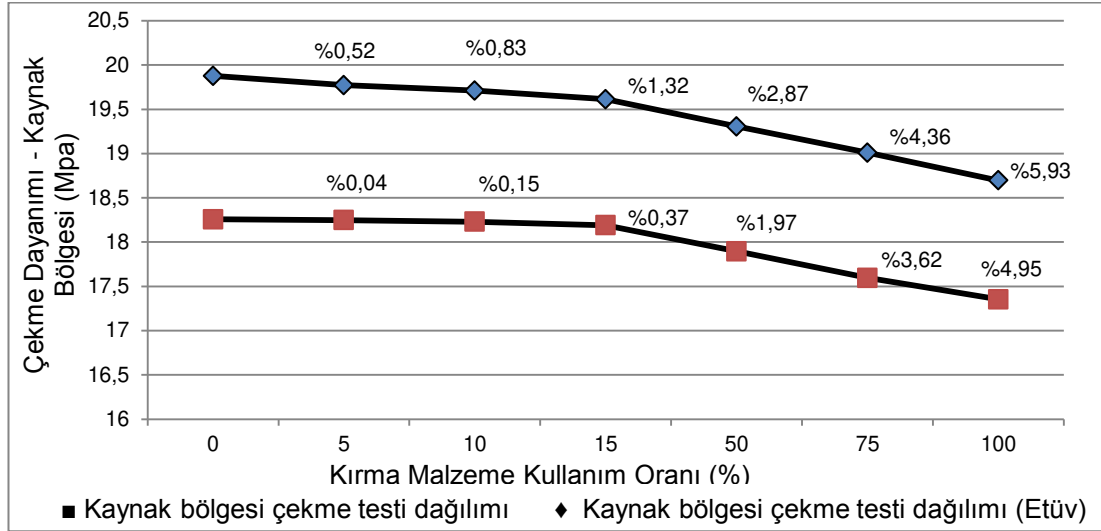
Şekil 6.3. Kıрма malzeme kullanımına göre kaynak bölgesi çekme dayanımı değişimi
