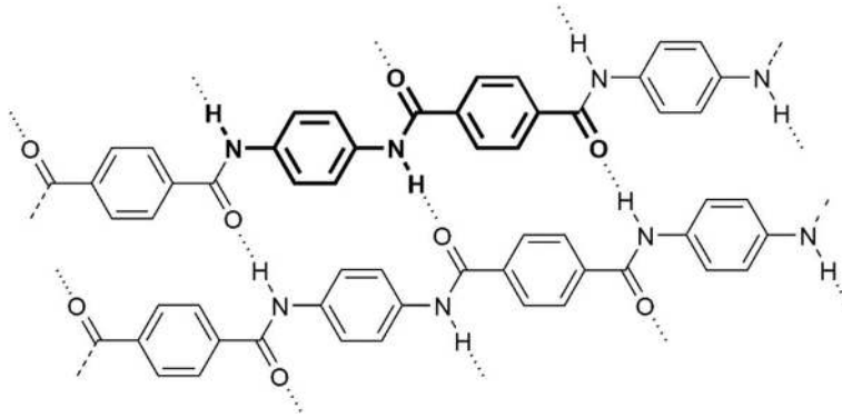
Şekil 3.10. Poliamidlerin kimyasal olarak gösterimi [13, 27].
