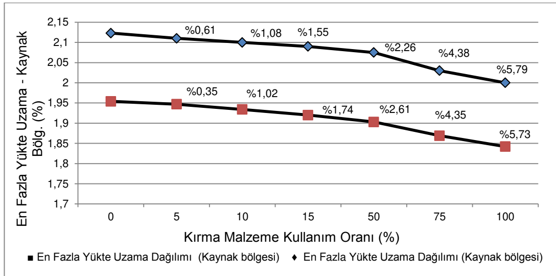
Şekil 6.4. Kıрма malzeme kullanımına göre kaynak bölgesi çekme-yükte uzama değişimi
