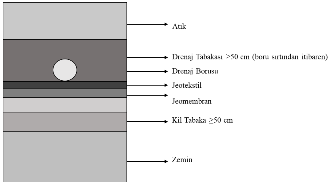
Şekil 3.14. Depo tabanı teşkili.
