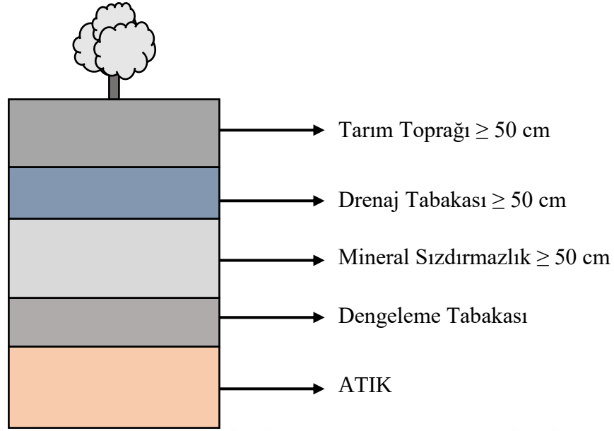
Şekil 3.15. II. Sınıf düzenli depolama tesisi üst geçirimsizlik sistemi.
