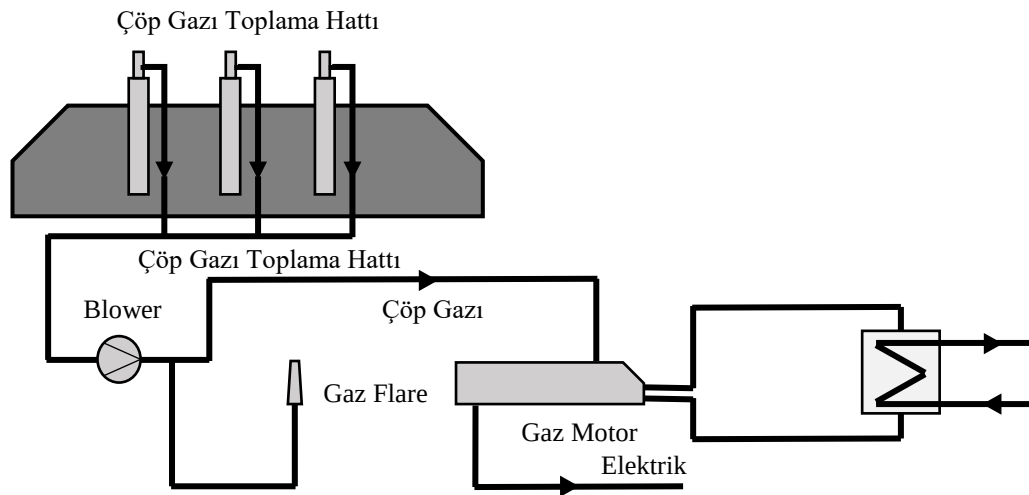
Şekil 3.17. Biyogaz tesisi iş akış şeması.
