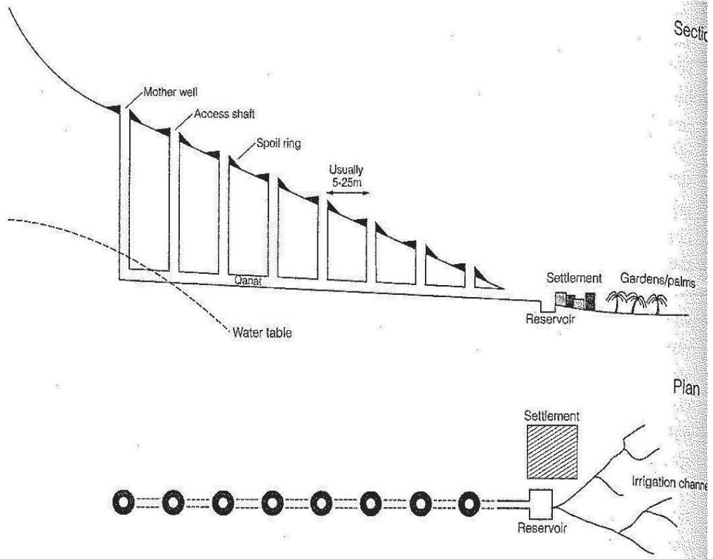
Figür 4: Bir Kehriz Şeması
