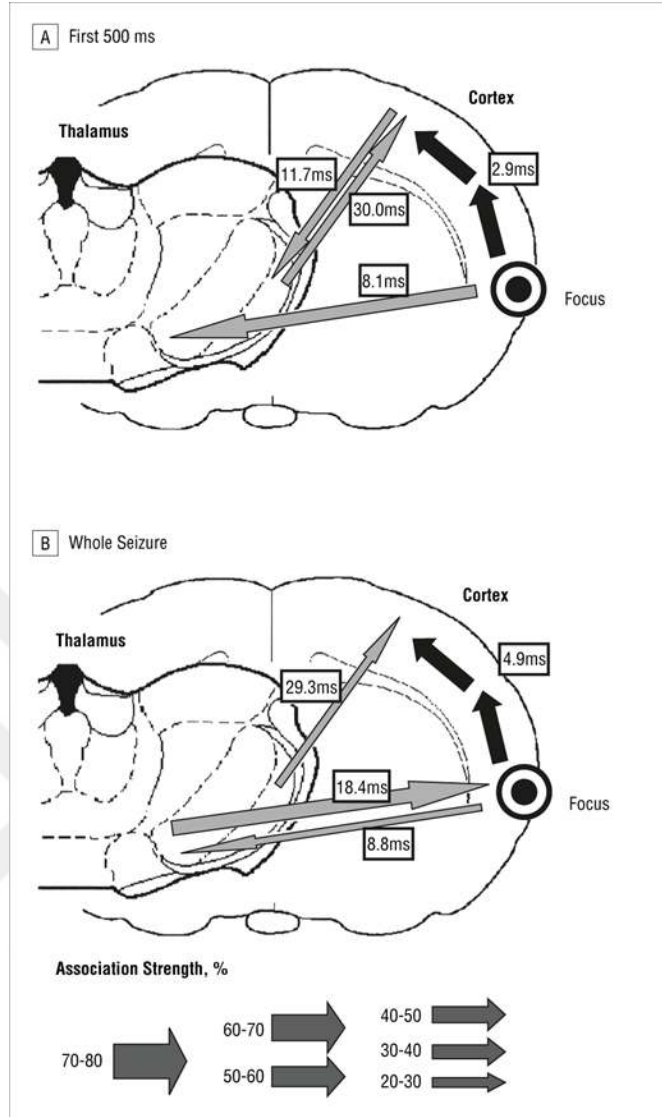
Şekil 26. Kortikokortikal ve kortikotalamik bağlantılar. Meeren ve ark.'ın 2002'deki çalışmalarında nonlinear assosiasyon analizi ile WAG/riz sıçanlarda saptadıkları spontan absans nöbetler süresince kortikokortikal (siyah oklar) ve kortikotalamik (gri oklar) karşılıklı bağlantıların şematik ifadesi. Okların kalınlığı bağlantının ağırlığını, yönü lagging tarafa yönelimi göstermektedir. A: nöbetin ilk 500 msn'si. Somato sensoriyal korteksin üst dudak ve burun bölgesinde (perioral bölge) bir kortikal odak bulundu. Bu fokal alana sırası ile arka ayak alanı 2,9 ms gecikme ile bulundu. İlgili talamo kortikal bağlantı ile ilişkili olarak, kortikal odak 8,1 msn lik bir gecikme ile talamik ventroposterior medial çekirdek ile bağlantı kurdu. B, tüm nöbet. İlk 500 msn süresince de olduğu gibi aynı kortikal odak bulundu. İlk 500 msn ile karşılaştırıldığında, kortikotalamik eşleşmenin yönü değişiyorken, aynı zamanda kortikal odaktan nonfokal kortikal bölgelere doğru zamansal gecikme arttı (74).
