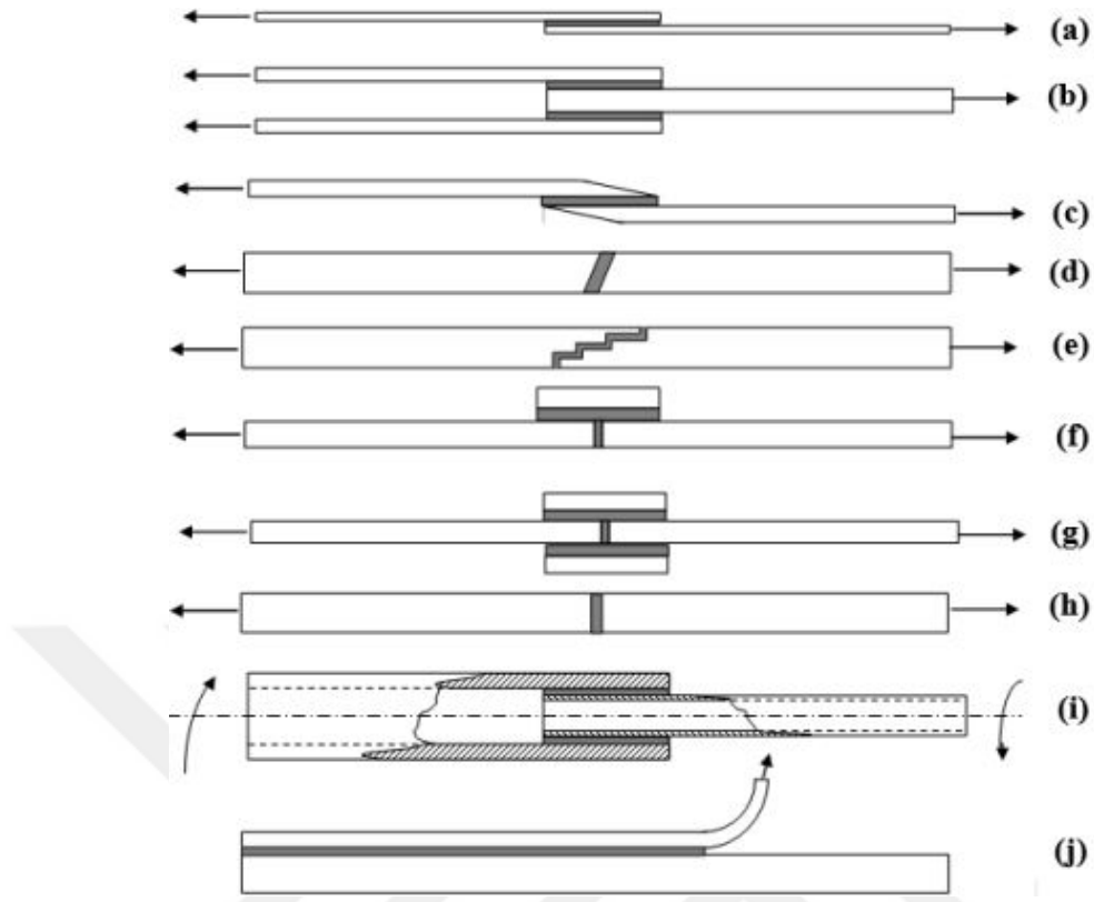
Şekil 2.7. Genel olarak kullanılan yapıştırma bağlantı tipleri, (a) tek tesirli bindirme, (b) çift tesirli bindirme, (c) boyun bindirme, (d) açılı bindirme, (e) teraslama, (f) tek takviyeli bindirme, (g) çift takviyeli bindirme, (h) alın bağlantı, (i) silindir bağlantı, (j) soyulma bağlantı (Adin, 2007)
