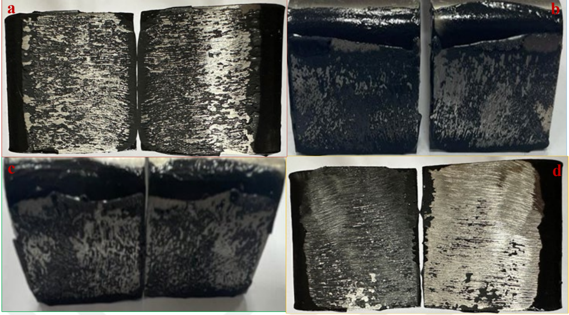
Şekil 4.11. DP490 yapıştırıcısı ve farklı takviye oranlarında Al_2O_3 ile yapılan yapıştırırmaların çekme kopma sonrası yüzey görüntüleri ( a:DP490, b:DP490-%2, c:DP490-%4, d:DP490-%6)
