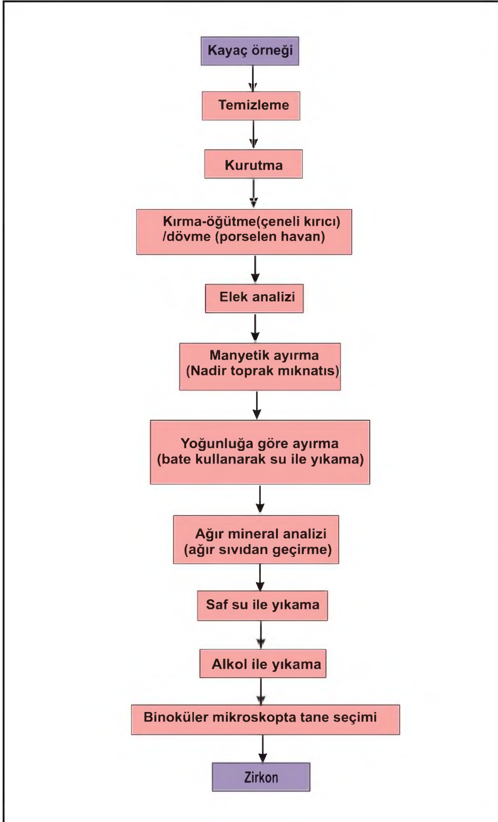
Şekil 2.2. Zirkon minerali ayırma işlemi akış şeması.
